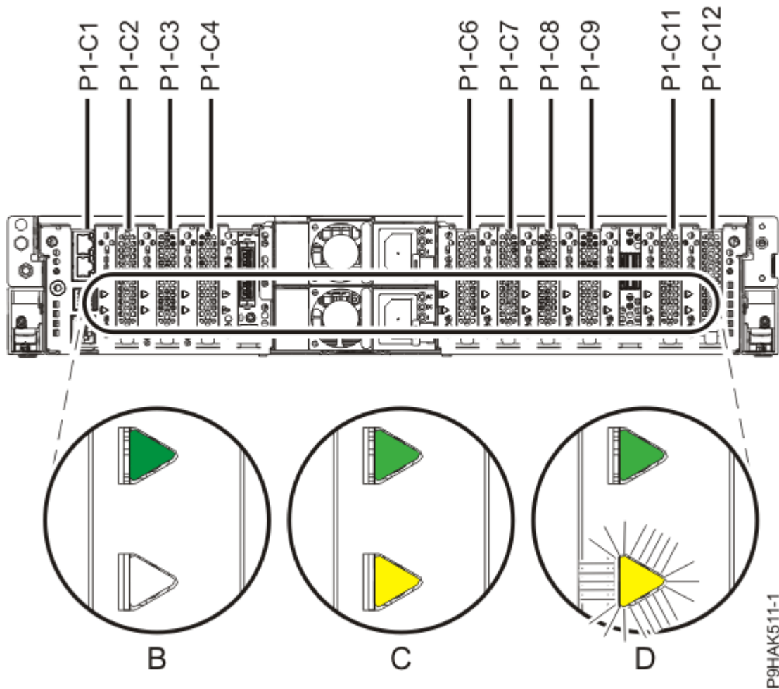
그림 1. 5105-22E, 9008-22L, 9009-22A, 9009-22G, 9223-22H, 또는 9223-22S 시스템에서 어댑터 슬롯 위치 및 LED 위치
