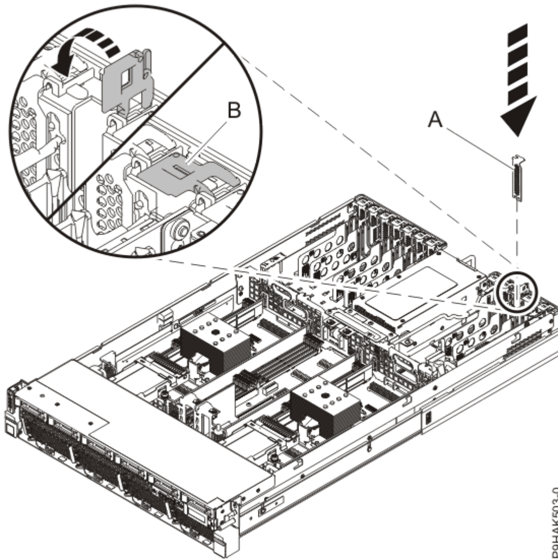
그림 39. 5105-22E, 9008-22L, 9009-22A, 9009-22G, 9223-22H, 또는 9223-22S 시스템에서 슬롯에 필터 설치
