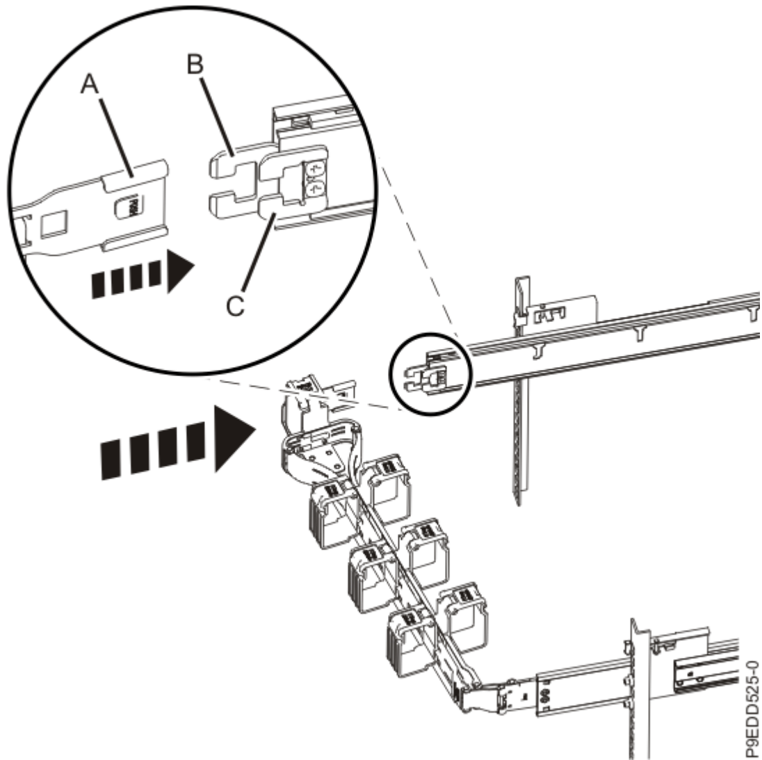
그림 31. 케이블 관리 암( arm ) 닫기
