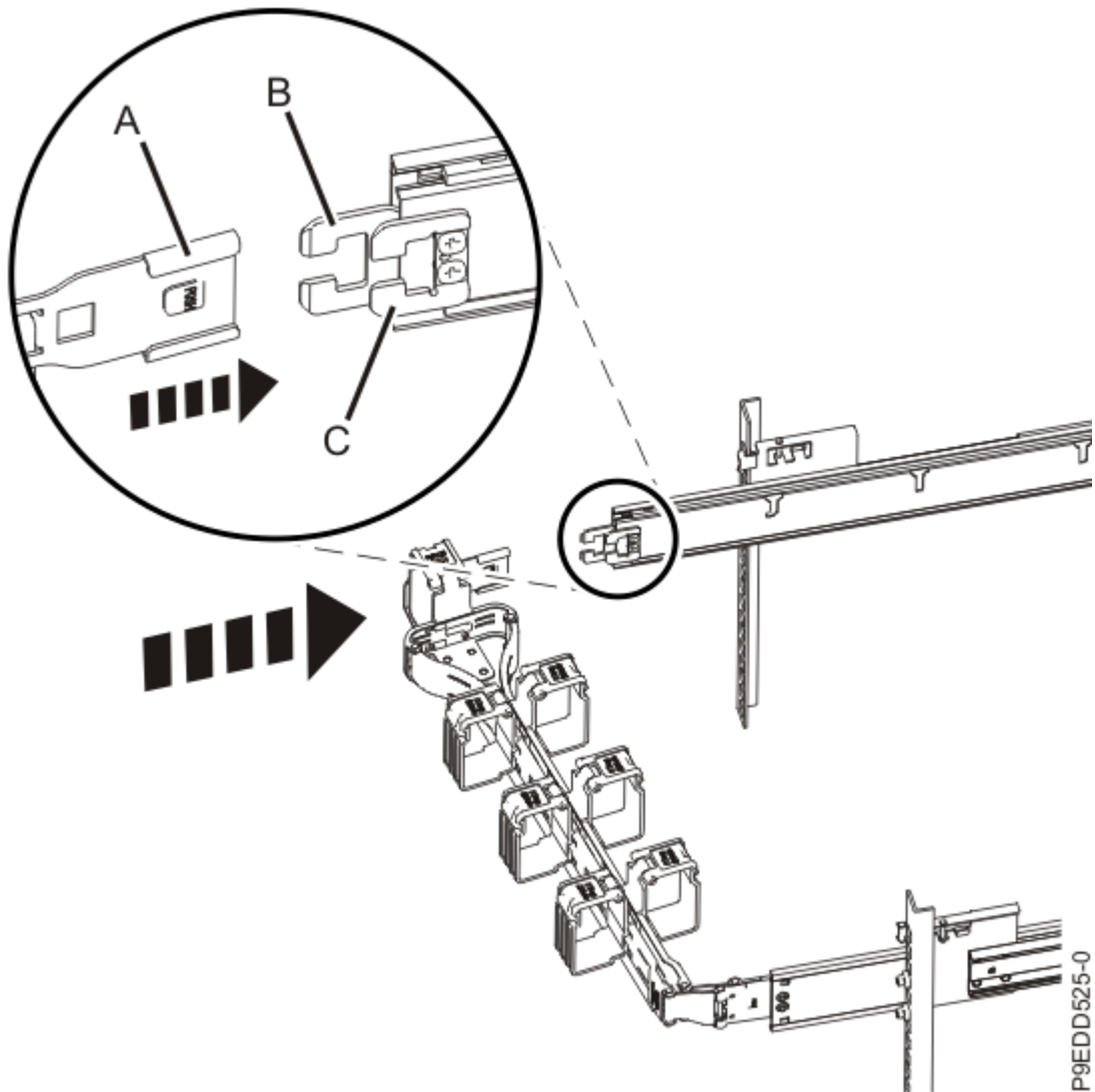
그림 35. 케이블 관리 암(arm) 닫기
