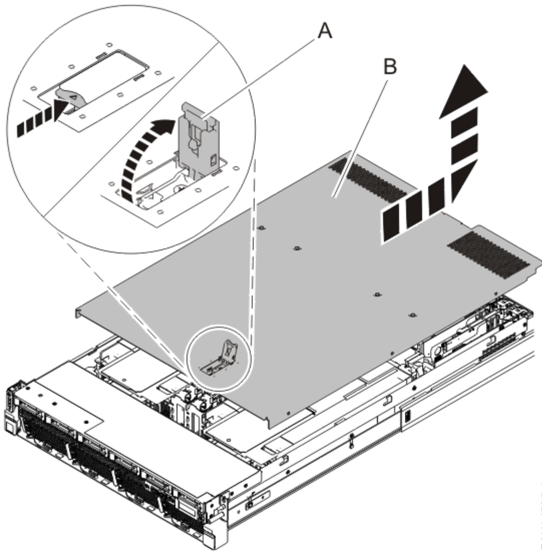
그림 37. 서비스 액세스 커버 제거
