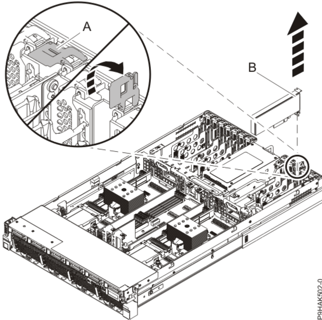
그림 38. 5105-22E, 9008-22L, 9009-22A, 9009-22G, 9223-22H, 또는 9223-22S 시스템에서 어댑터 제거
