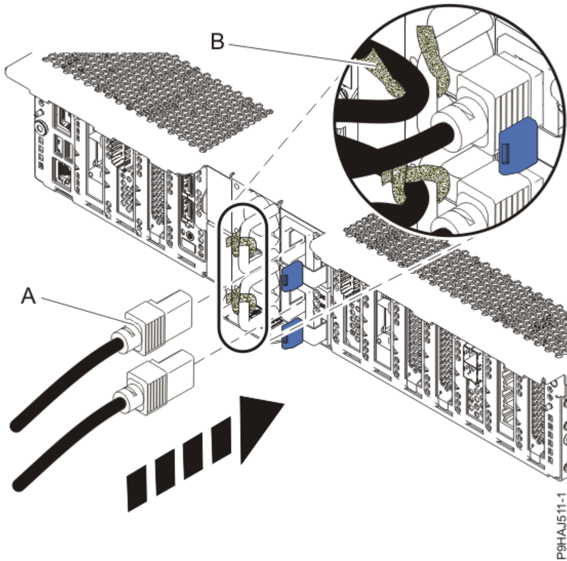
그림 14. 전원 코드 연결
