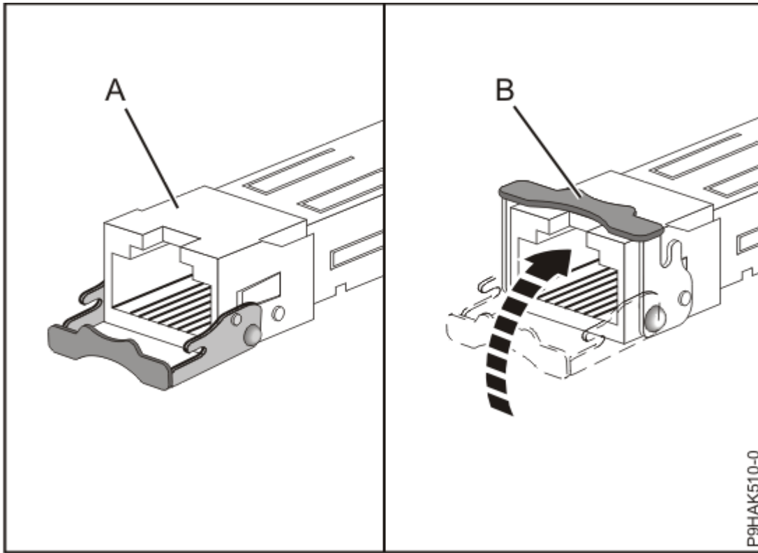
그림 49. 어댑터에서 SFP 트랜시버 교체
