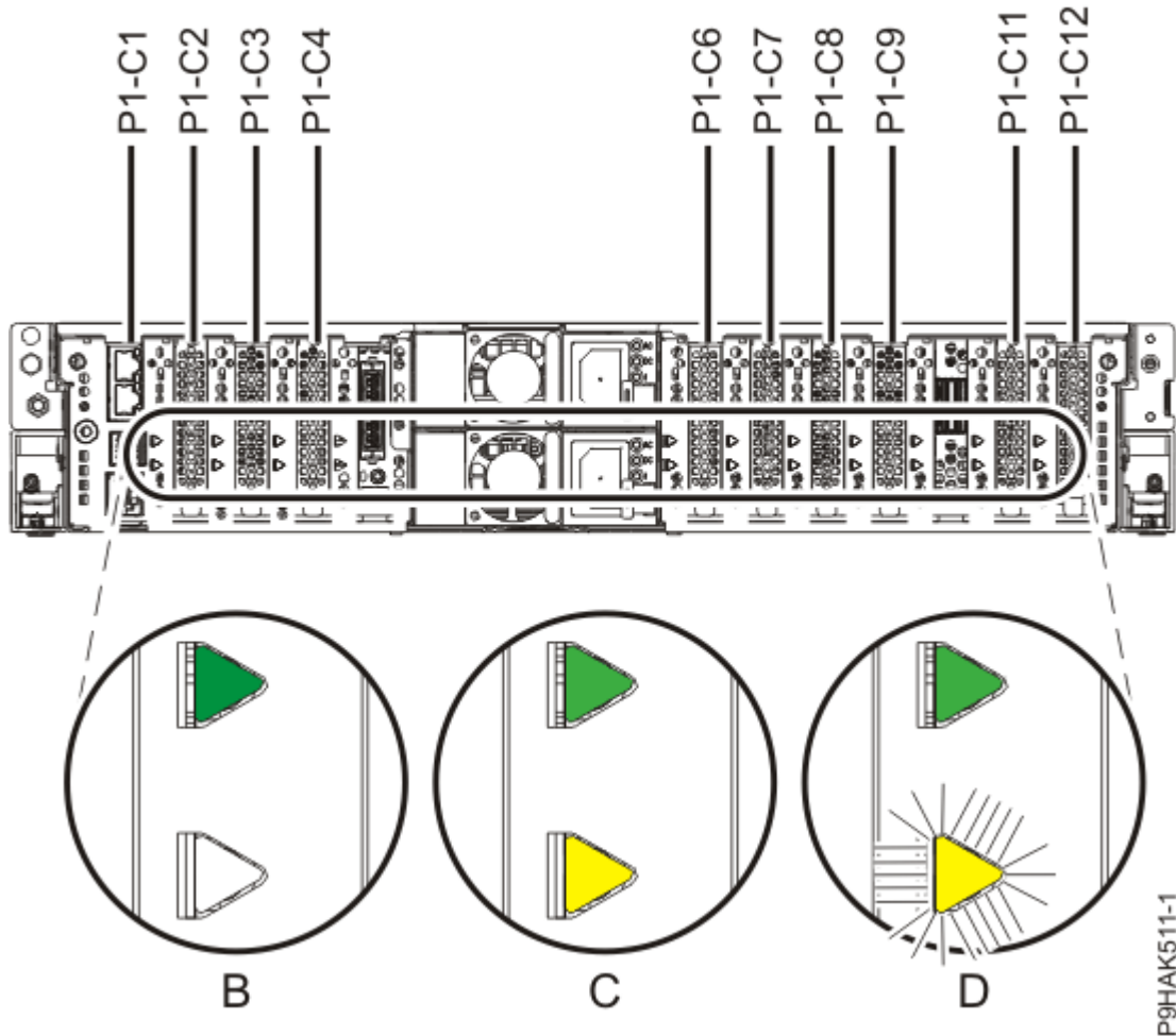
그림 16. 5105-22E, 9008-22L, 9009-22A, 9009-22G, 9223-22H, 또는 9223-22S 시스템에서 어댑터 슬롯 위치 및 LED 위치
