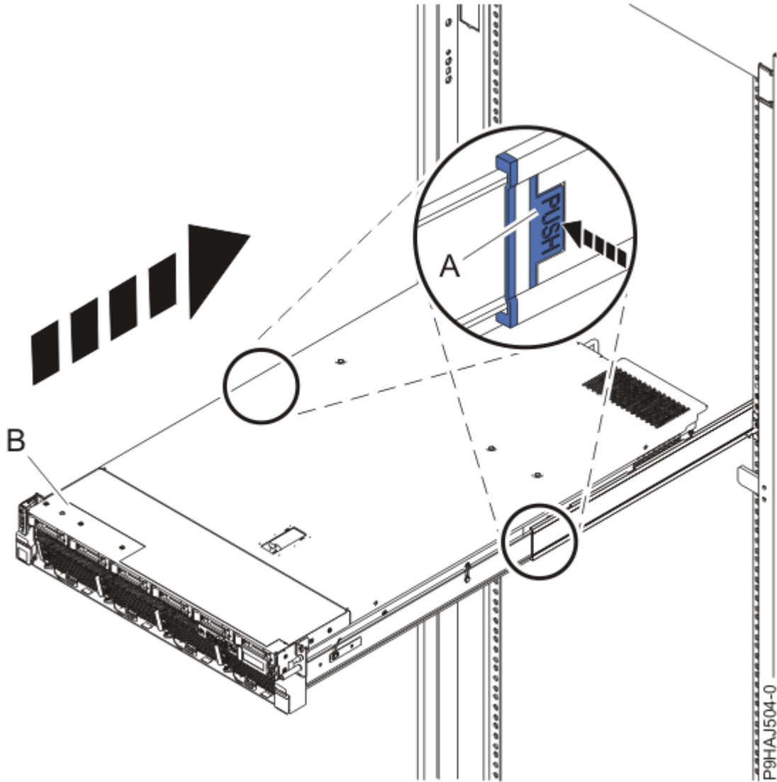
그림 28. 시스템을 작동 위치에 배치
