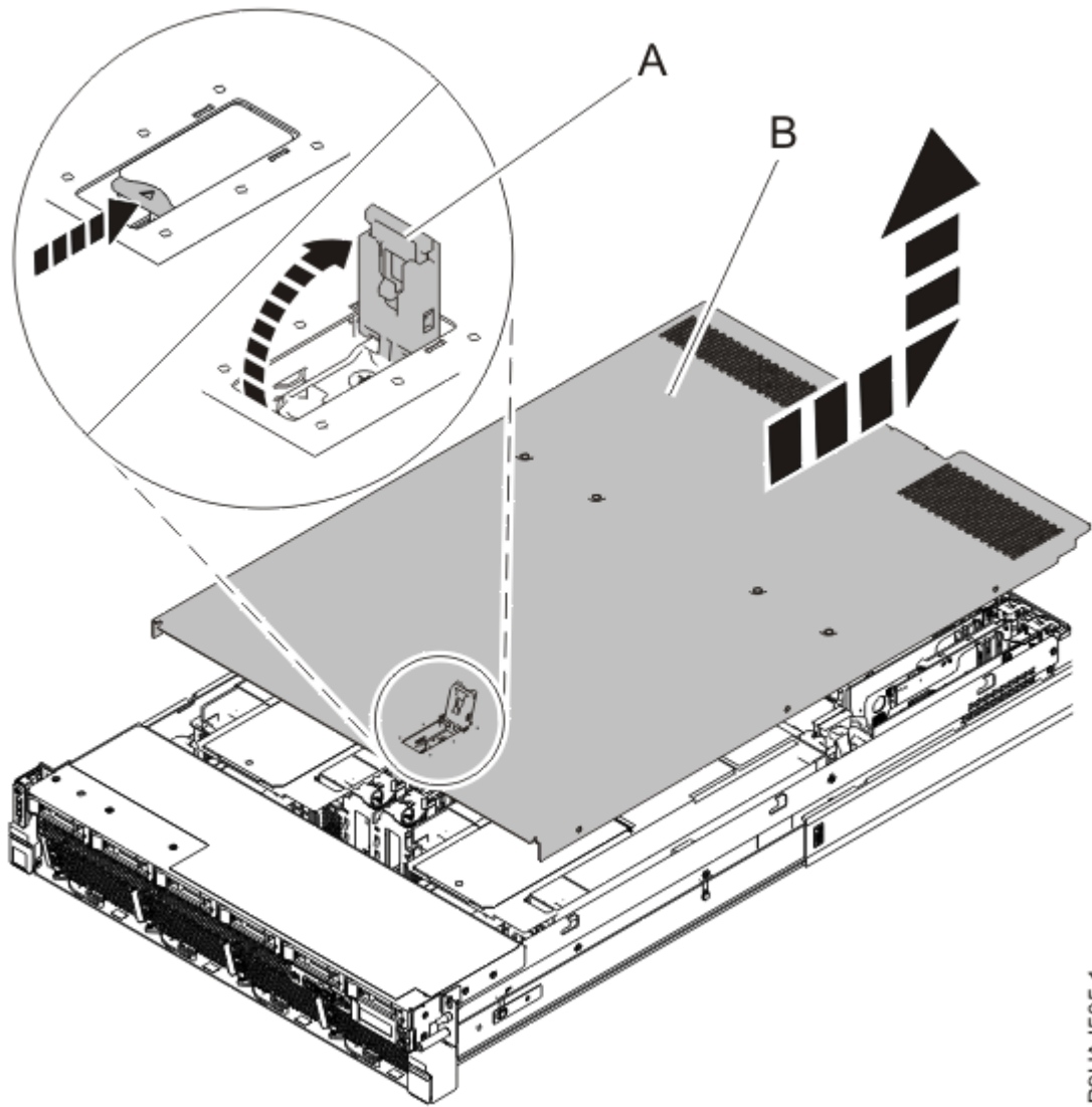
그림 24. 서비스 액세스 커버 제거
