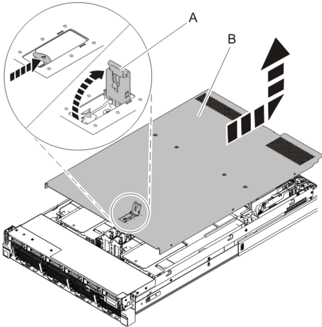
그림 10. 서비스 액세스 커버 제거
