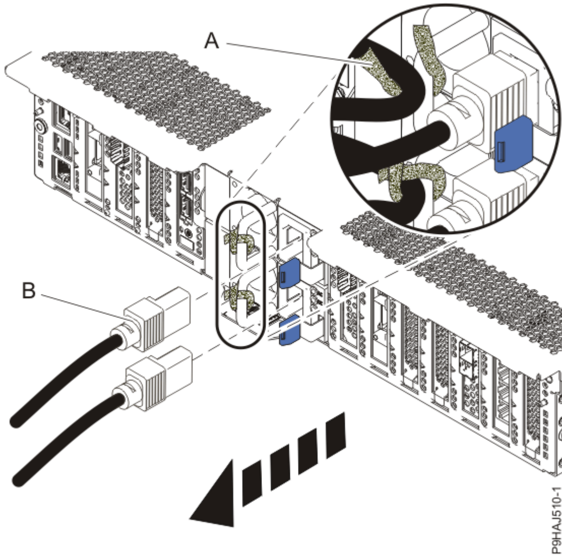
그림 34. 전원 코드 제거
