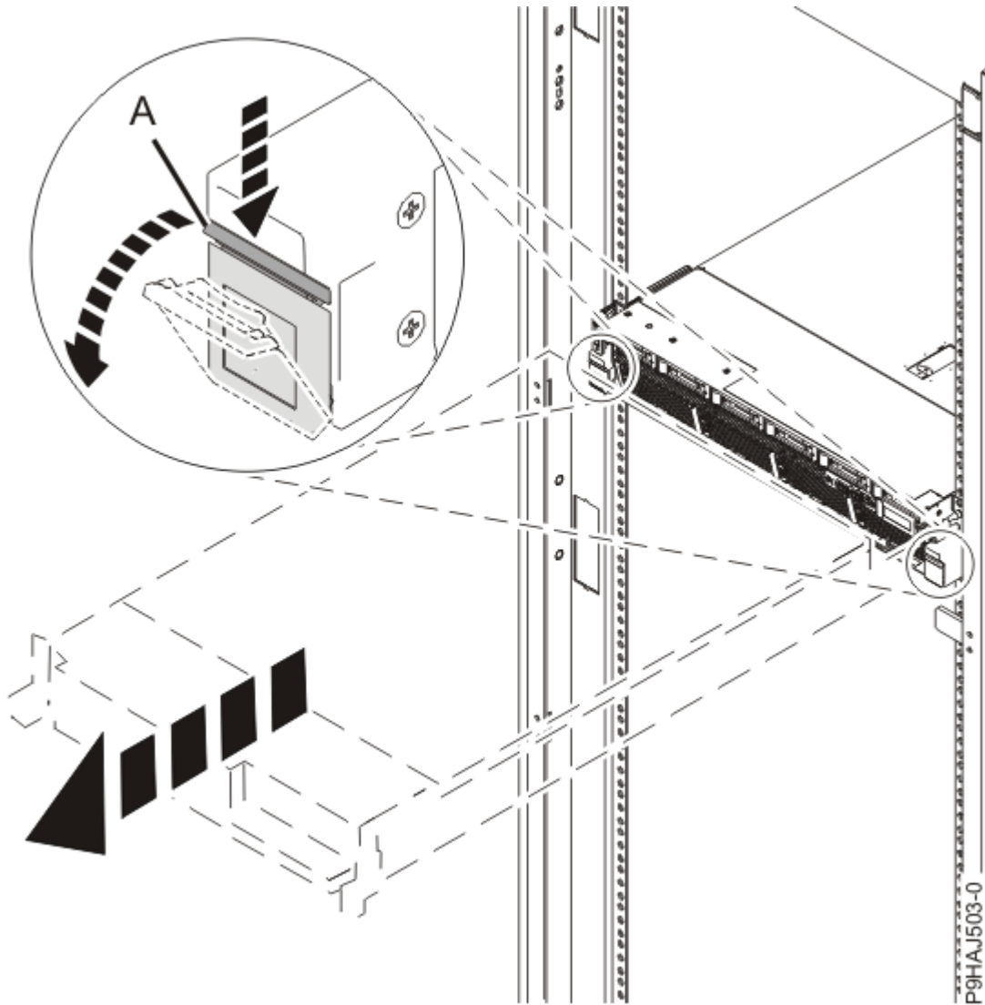
그림 8. 측면 걸쇠 해제
