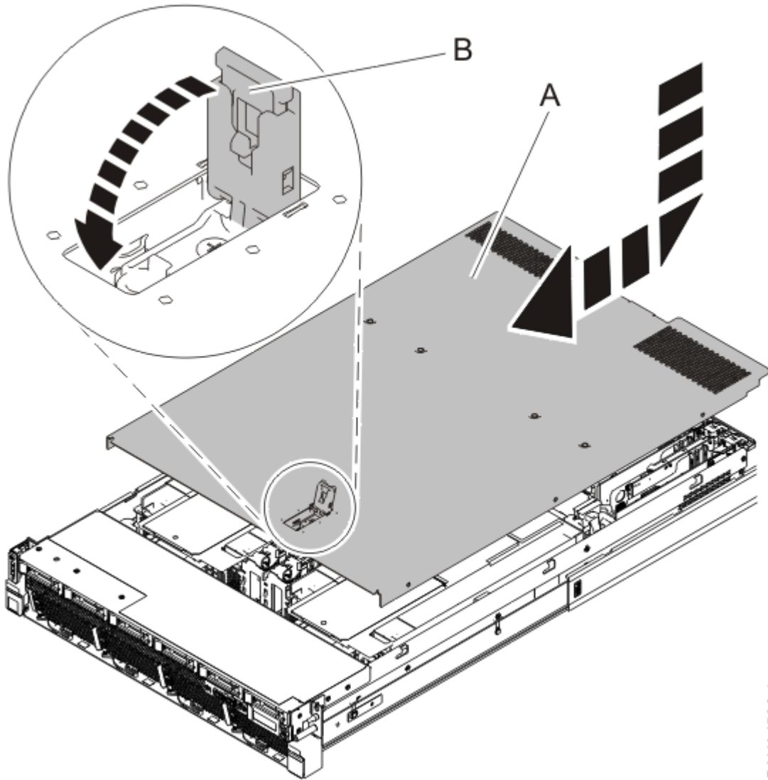
그림 12. 서비스 액세스 커버 설치
