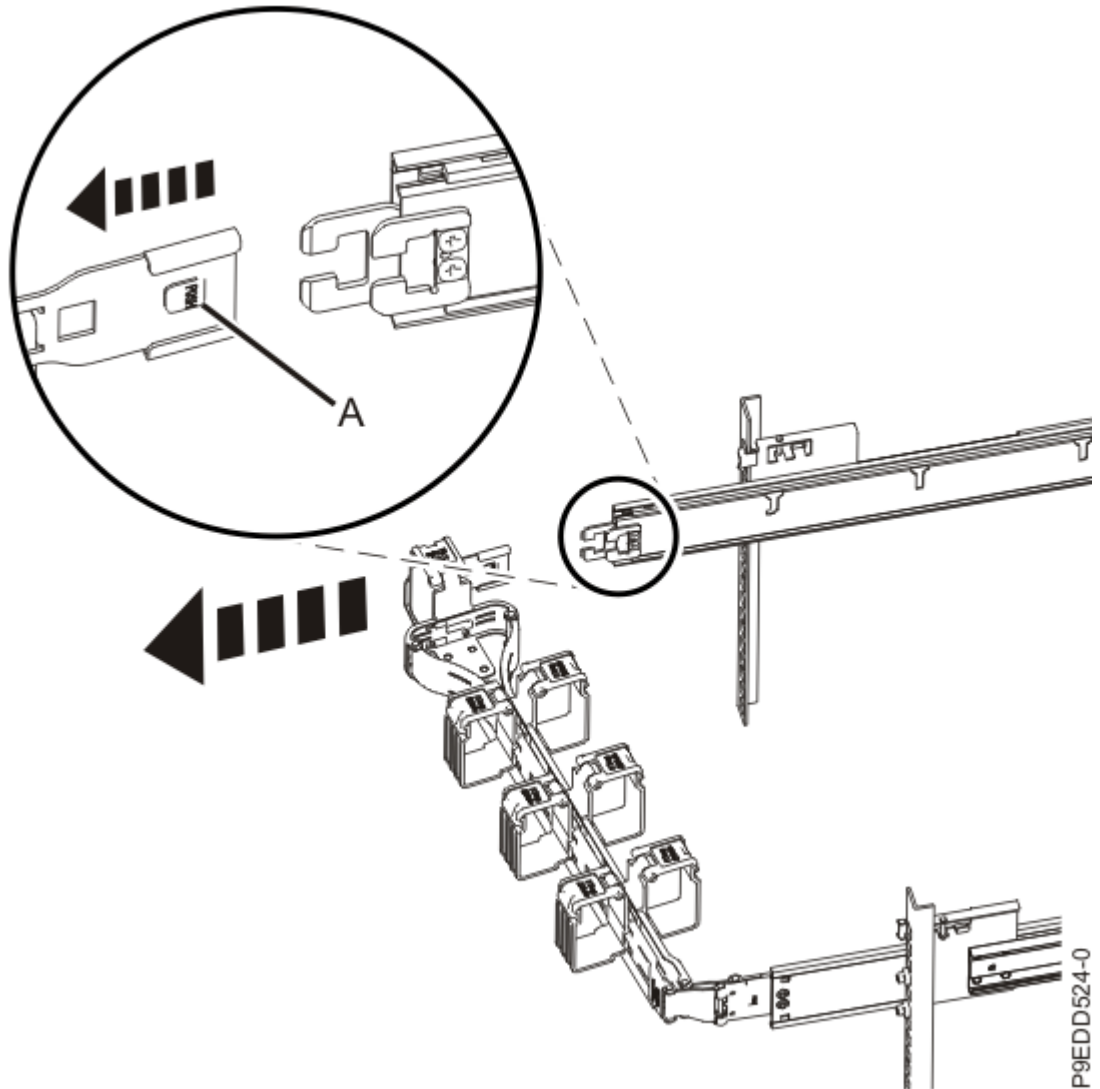
그림 2. 장착 브래킷 해제
