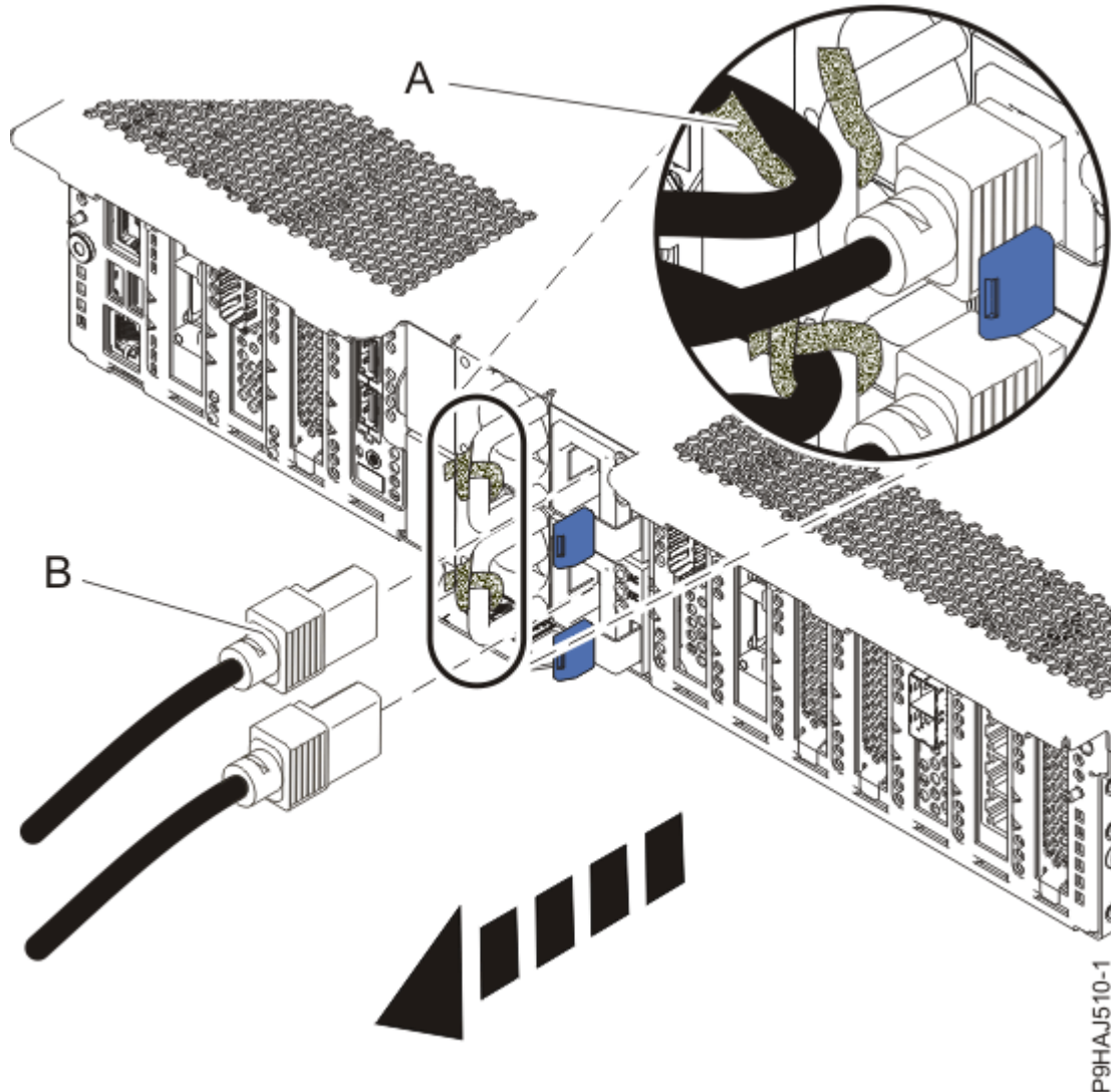
그림 3. 전원 코드 제거
