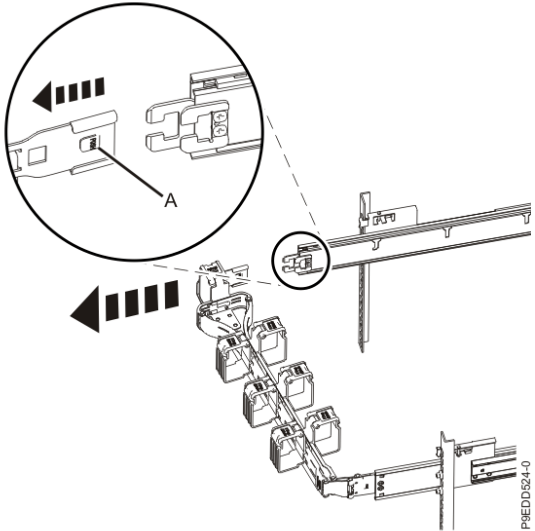
그림 17. 장착 브래킷 해제
