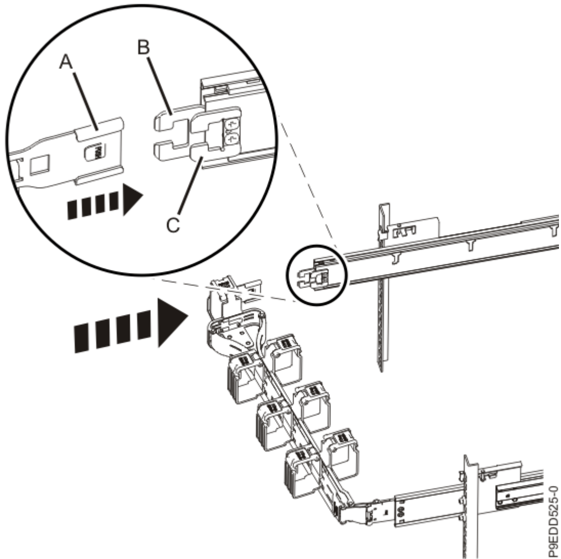
그림 7. 케이블 관리 암( arm ) 닫기
