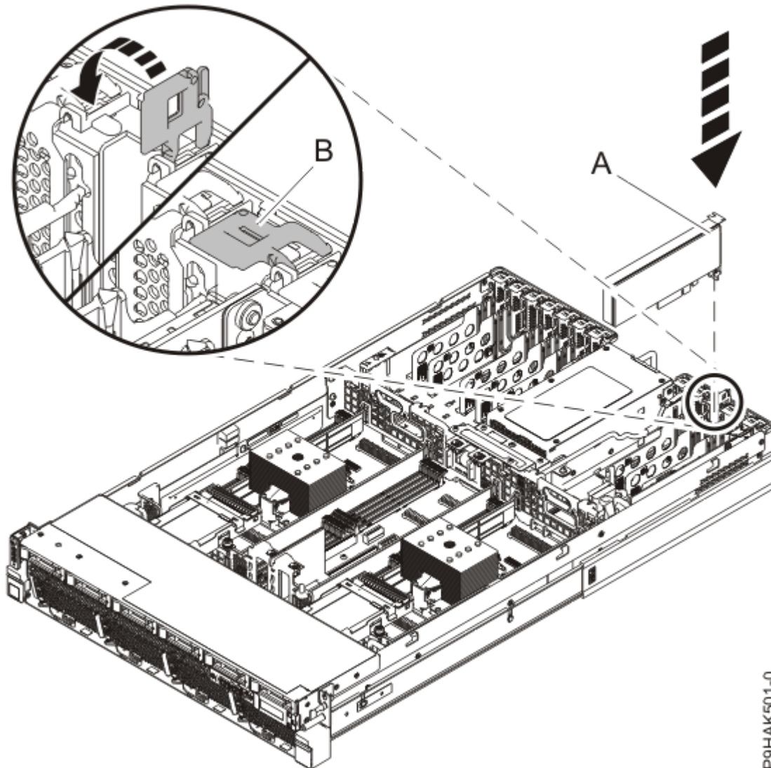
그림 11. 5105-22E, 9008-22L, 9009-22A, 9009-22G, 9223-22H, 또는 9223-22S에서 어댑터 설치 또는 교체
