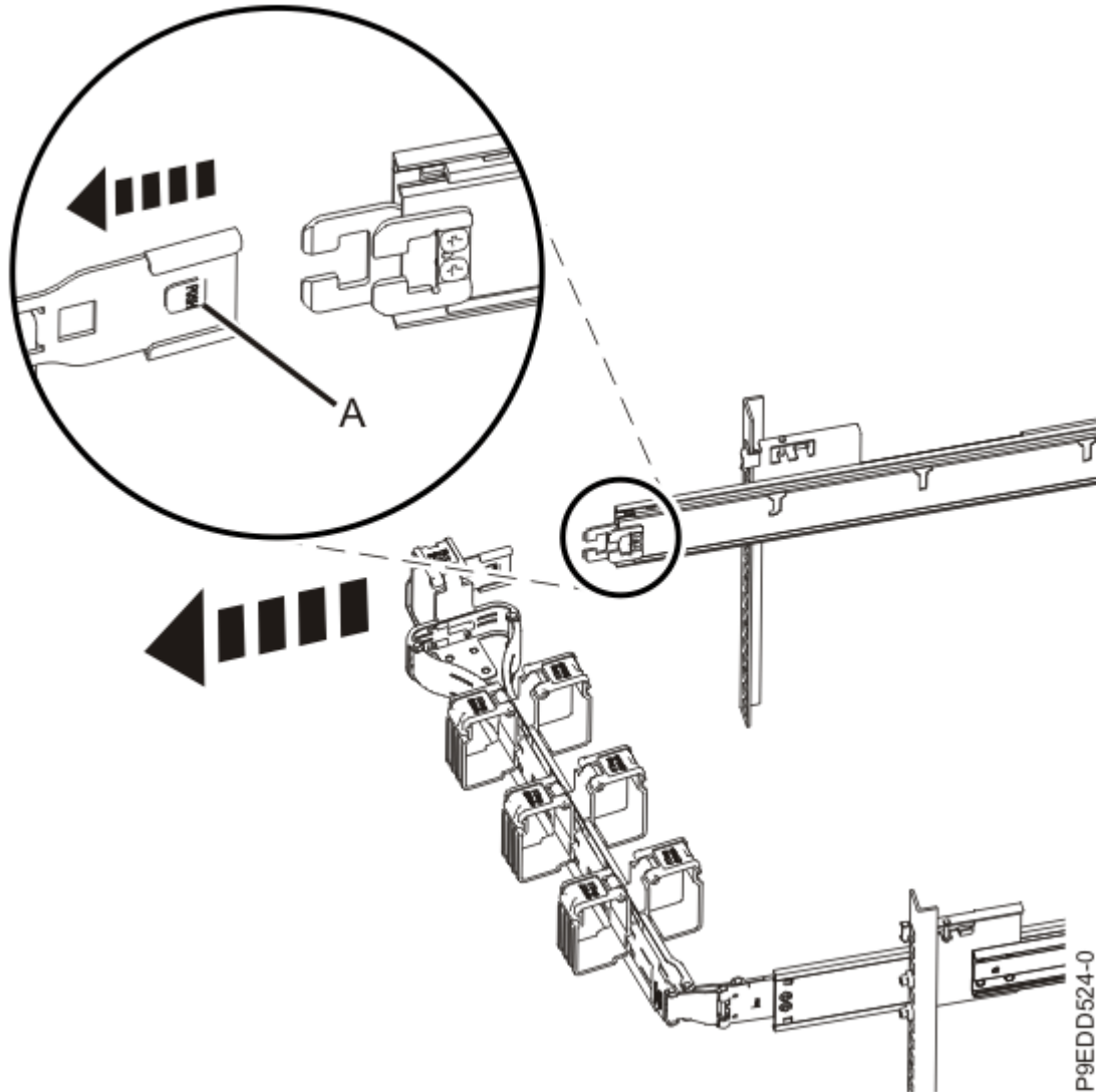
그림 5. 장착 브래킷 해제
