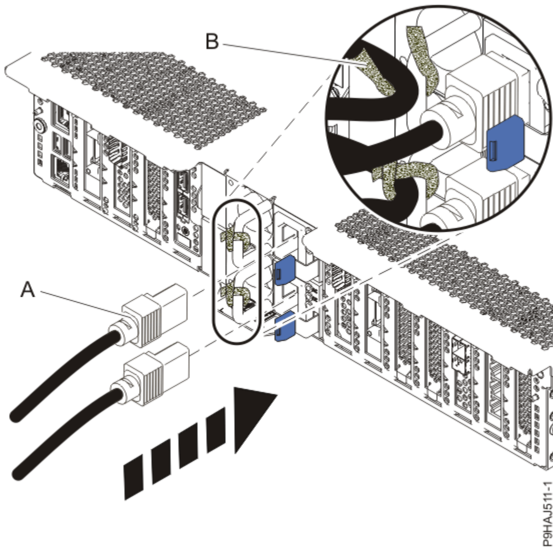
그림 43. 전원 코드 연결
