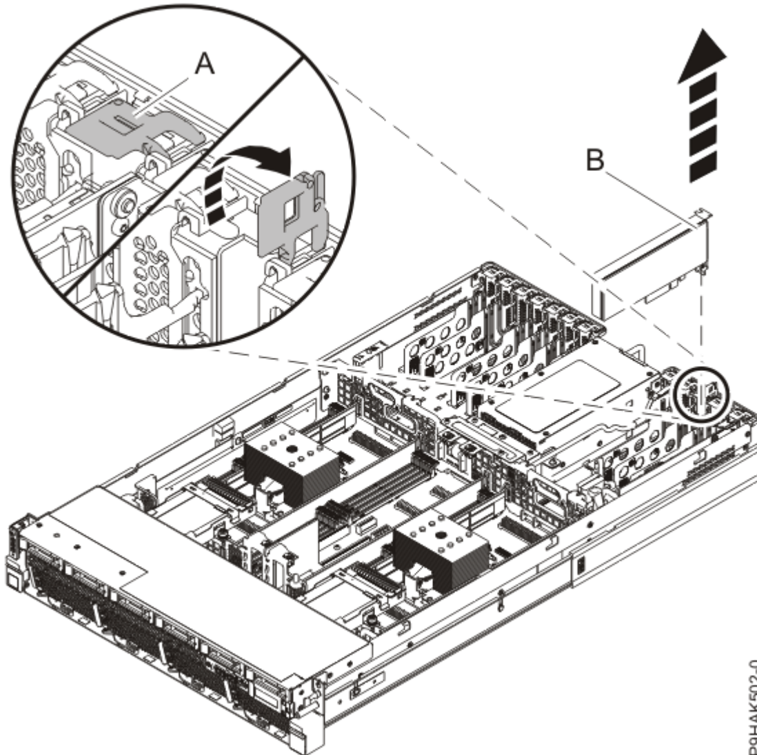
그림 25. 5105-22E, 9008-22L, 9009-22A, 9009-22G, 9223-22H, 또는 9223-22S 시스템에서 어댑터 제거
