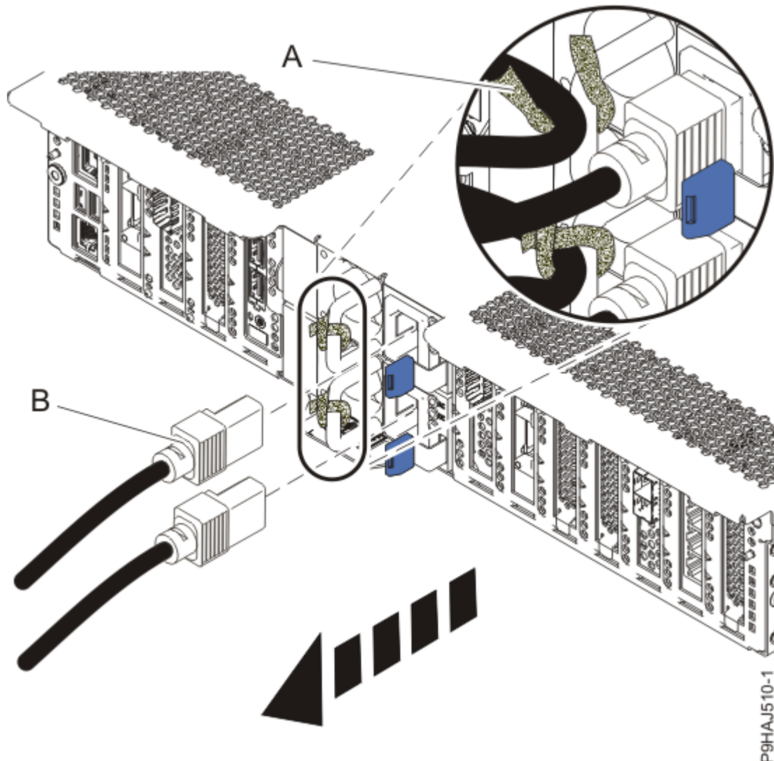
그림 18. 전원 코드 제거
