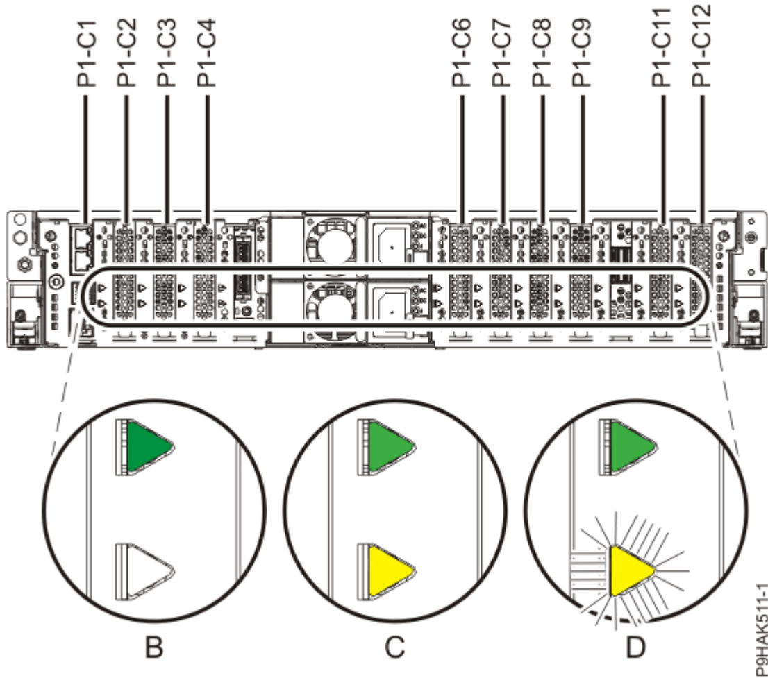
그림 32. 5105-22E, 9008-22L, 9009-22A, 9009-22G, 9223-22H, 또는 9223-22S 시스템에서 어댑터 슬롯 위치 및 LED 위치
