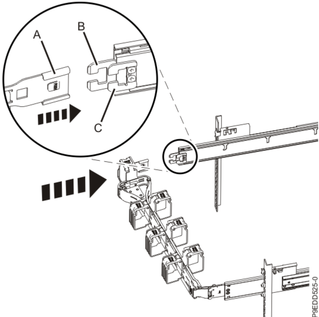
그림 22. 케이블 관리 암(arm) 닫기
