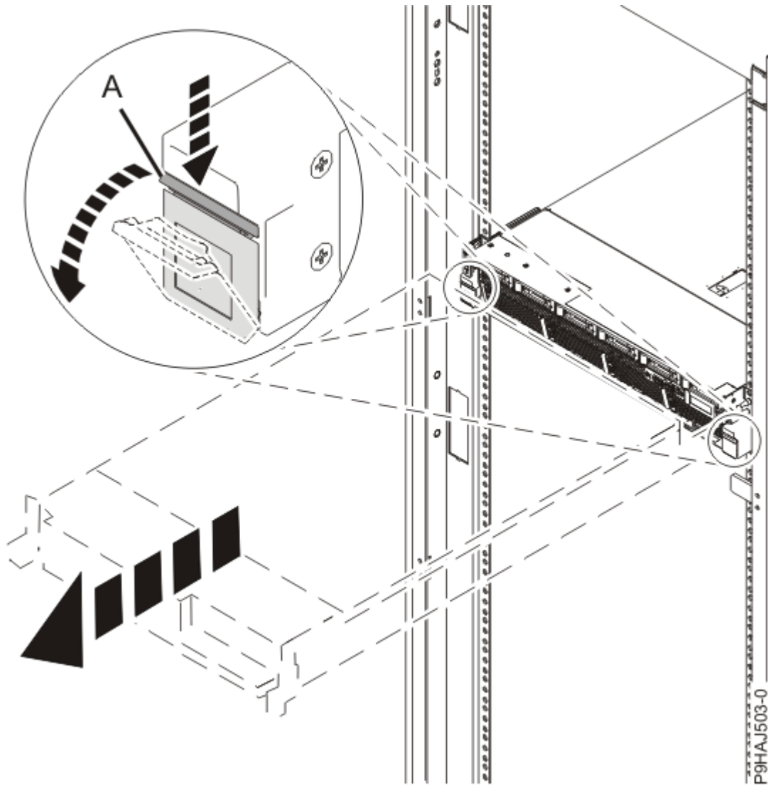
그림 9. 측면 걸쇠 해제
