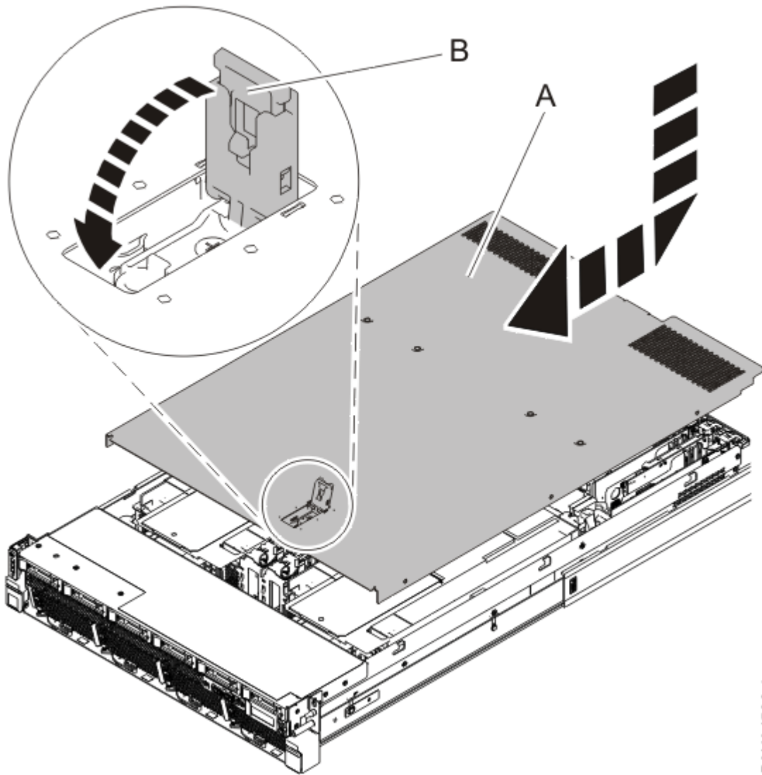
그림 27. 서비스 액세스 커버 설치
