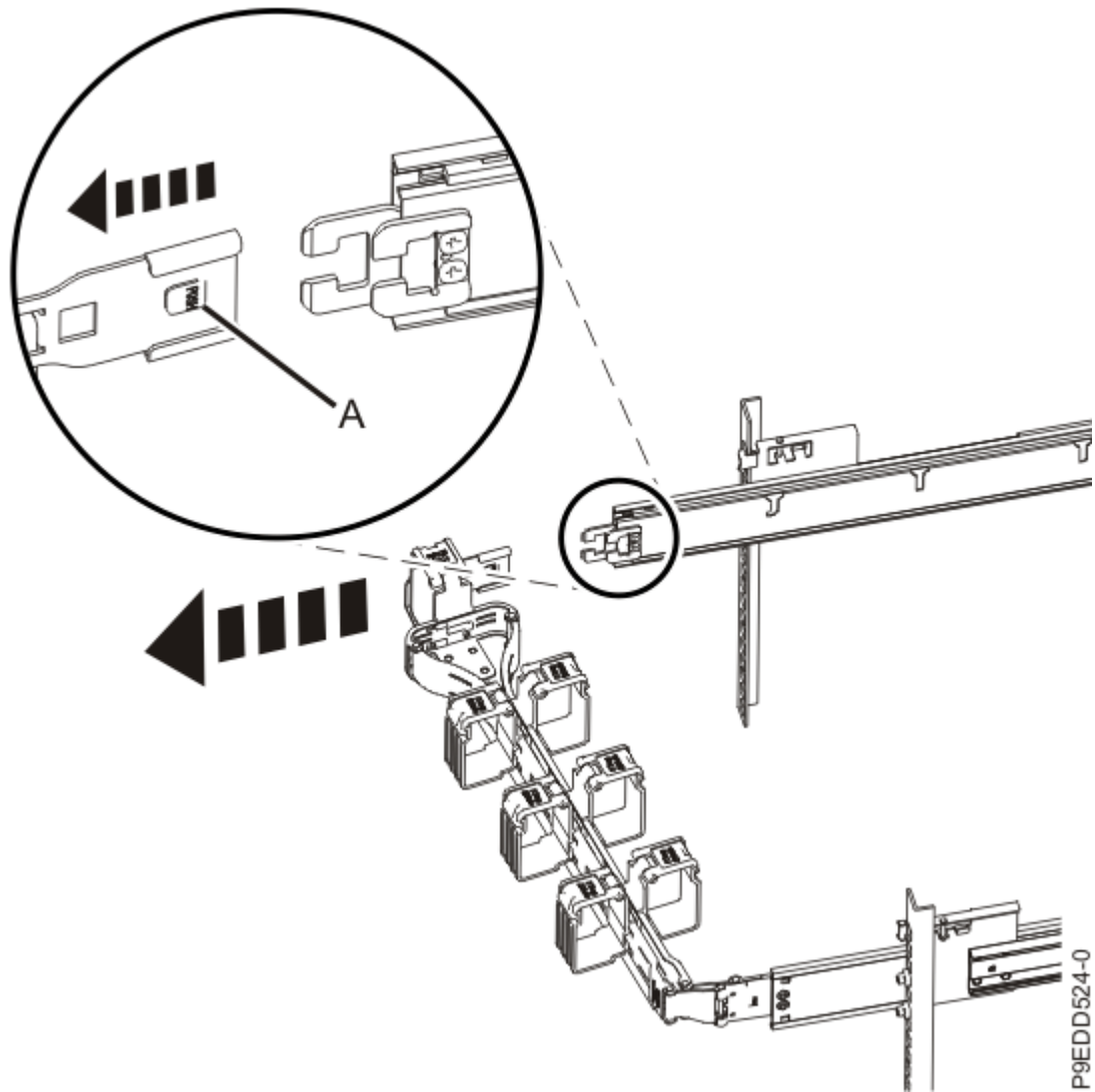
그림 42. 케이블 관리 암( arm ) 해제
