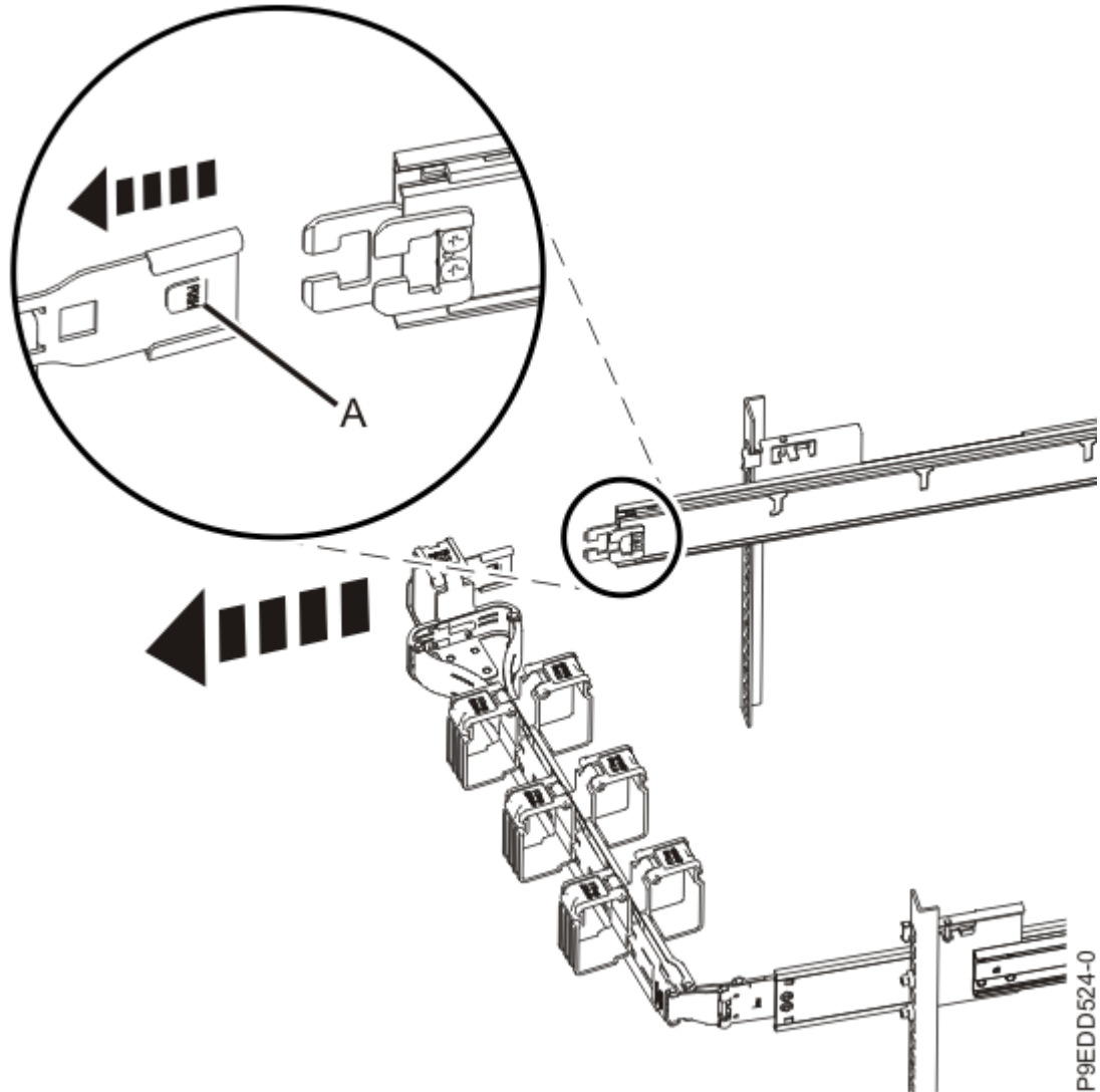
그림 13. 케이블 관리 암(arm) 해제
