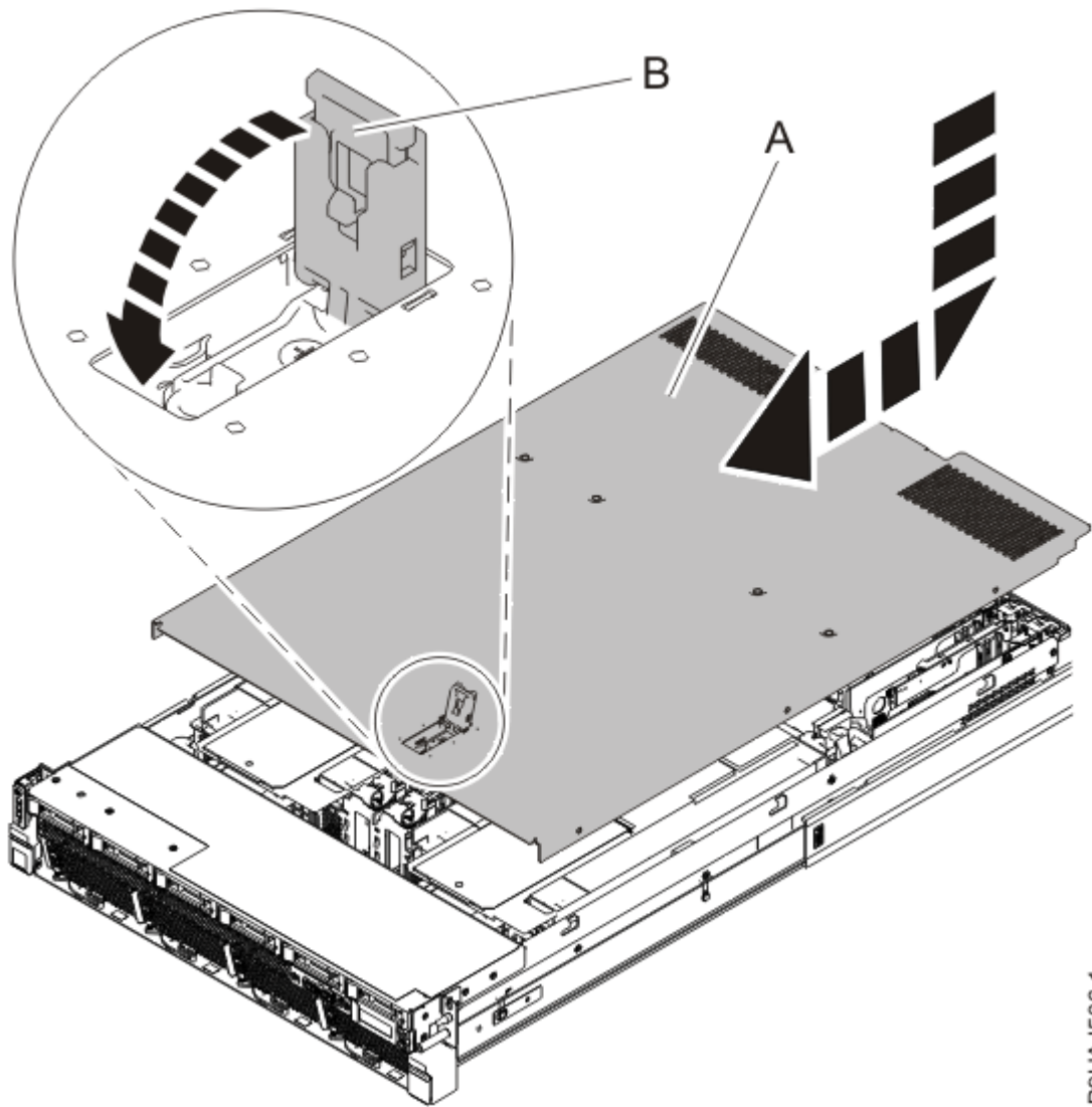
그림 40. 서비스 액세스 커버 설치
