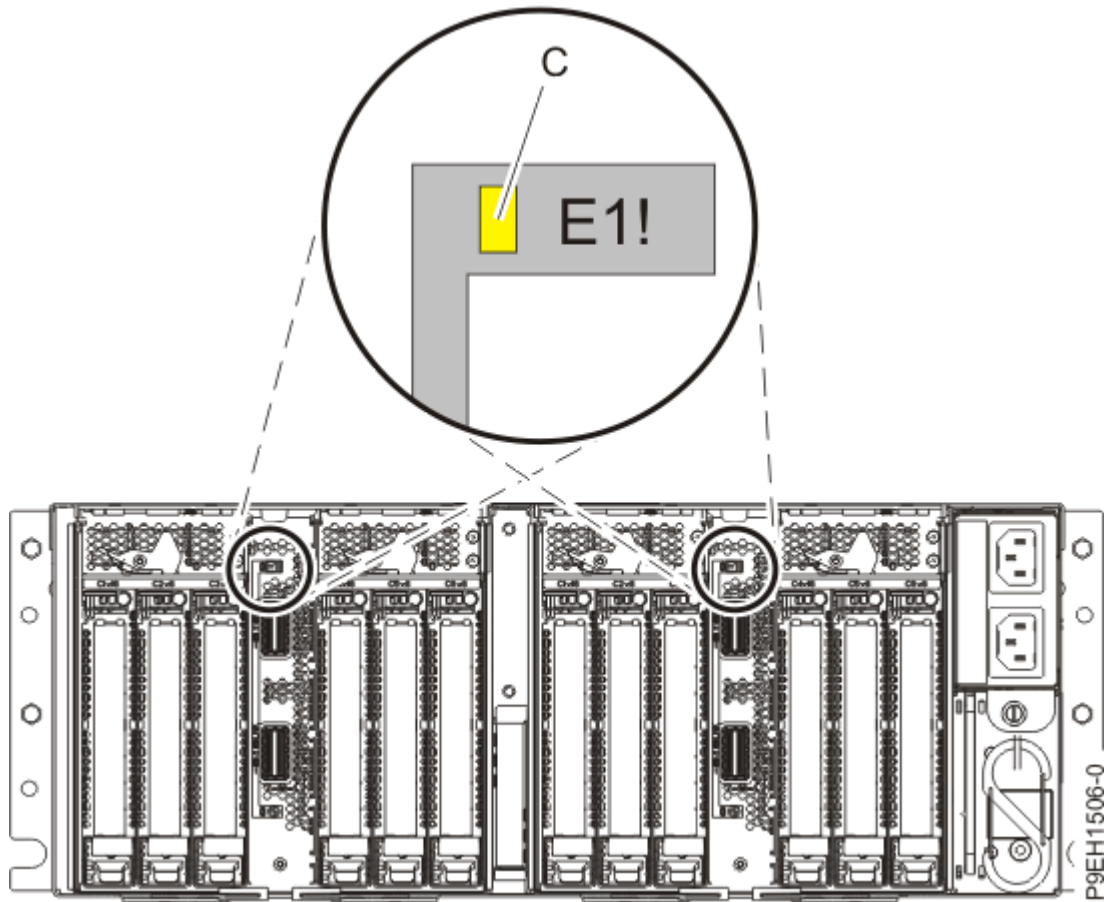
그림 3. 전압 조정 모듈(VRM) LED
