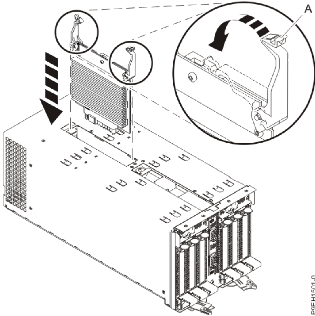
그림 6. 전압 조정 모듈(VRM) 교체
