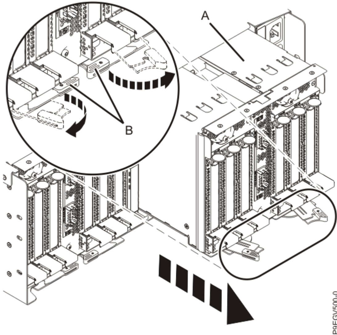
그림 4. 해제 걸쇠 열기
