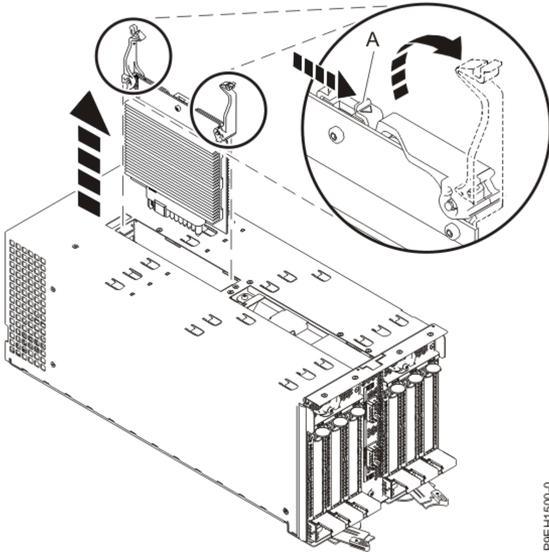
그림 5. 전압 조정 모듈(VRM) 제거
