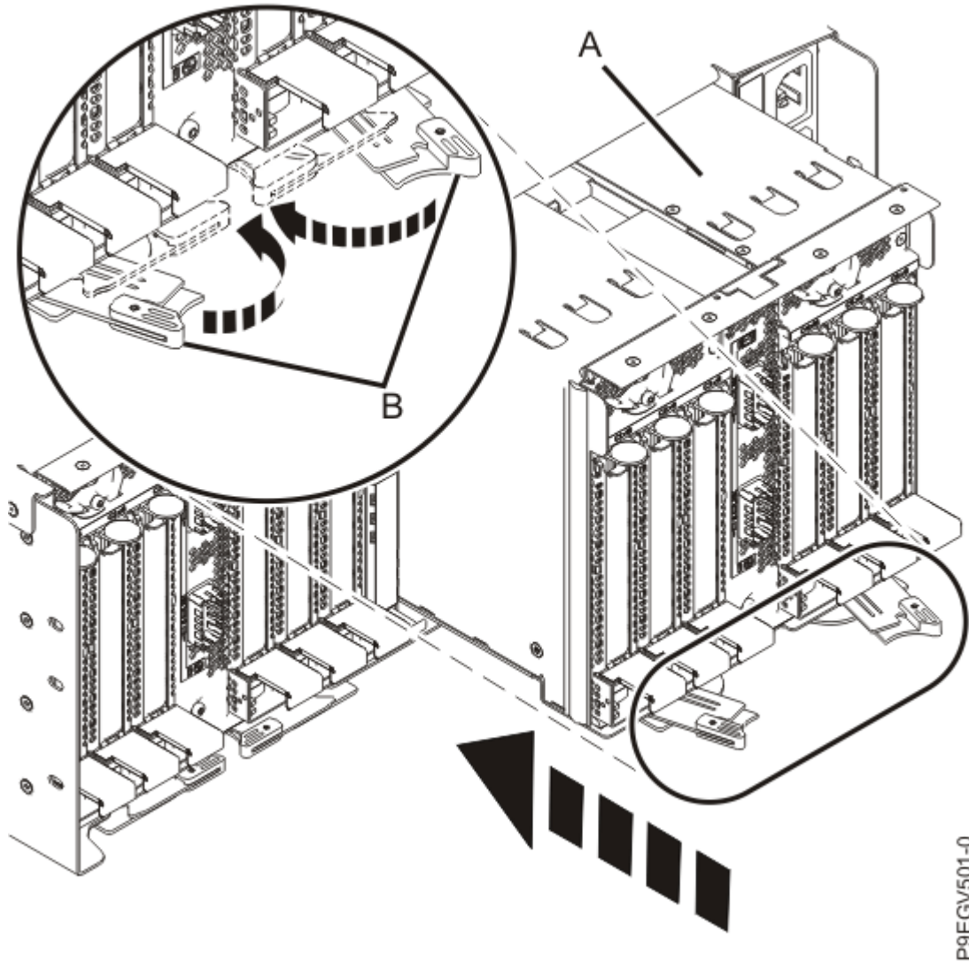
그림 7. 해제 걸쇠 닫기
