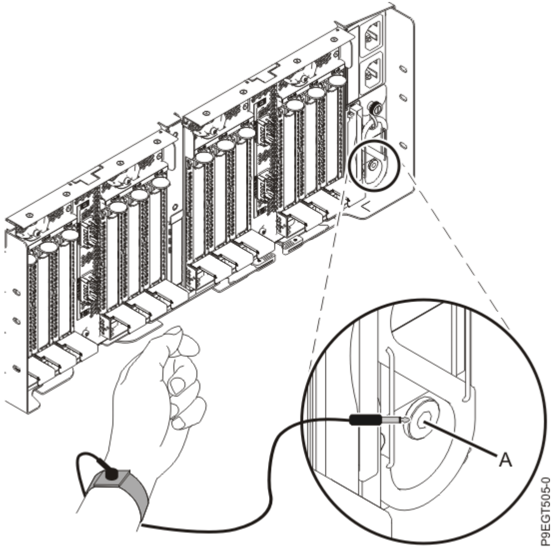
그림 1. EMX0 PCIe3 확장 드로어 뒷면의 ESD 잭 위치
