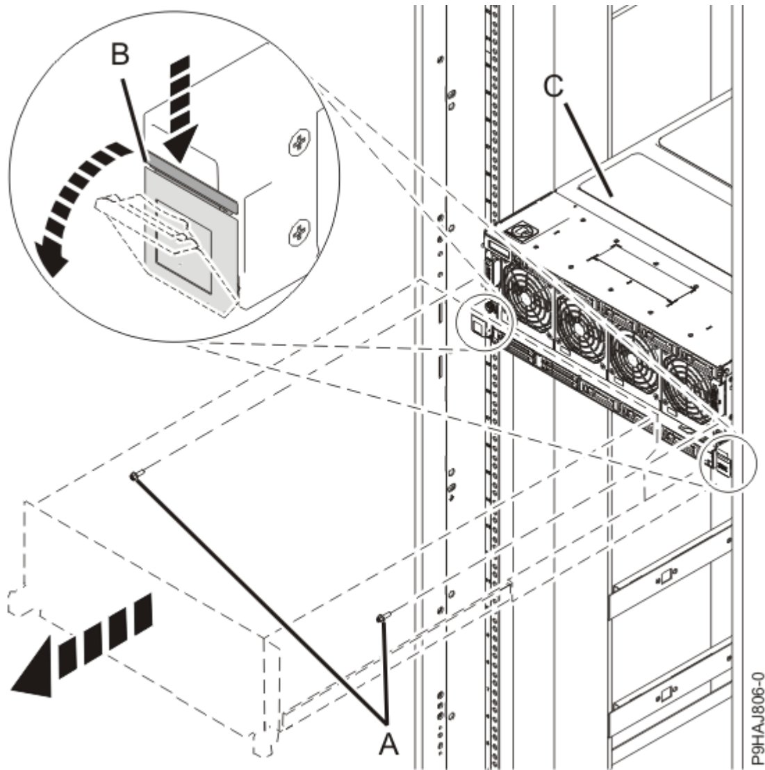
그림 3. 시스템을 서비스 위치에 배치
