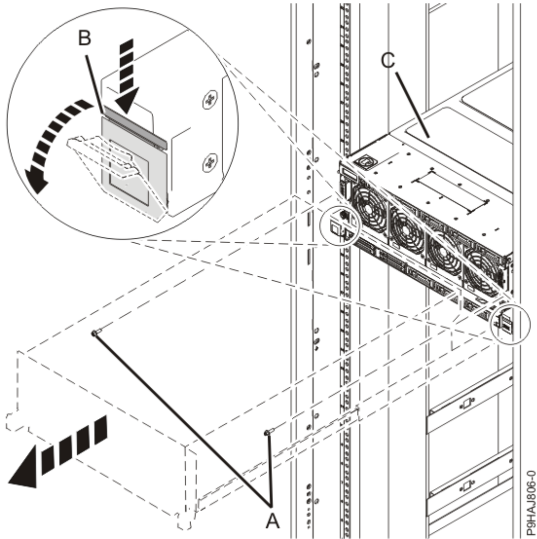
그림 10. 시스템을 서비스 위치에 배치
