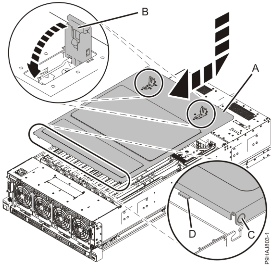
그림 13. 서비스 액세스 커버 설치
