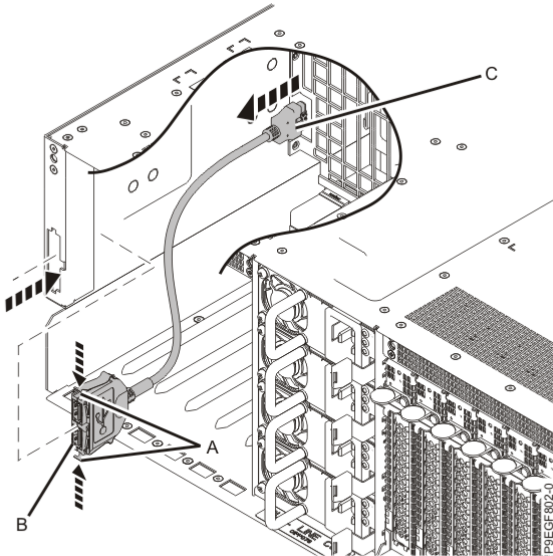
그림 8. 뒷면 USB 포트 커넥터 제거
