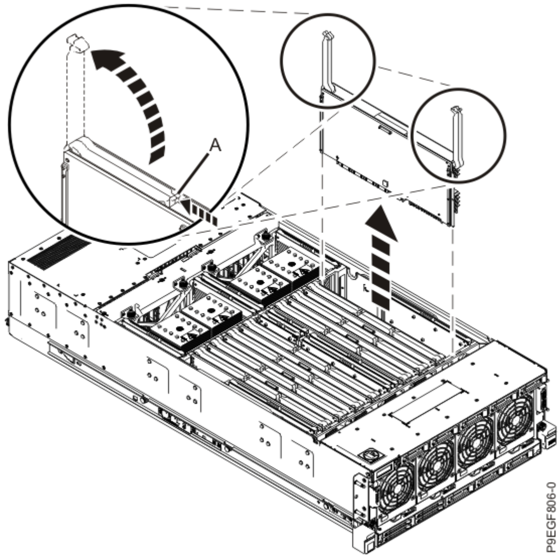
그림 5. 메모리 라이저 제거
