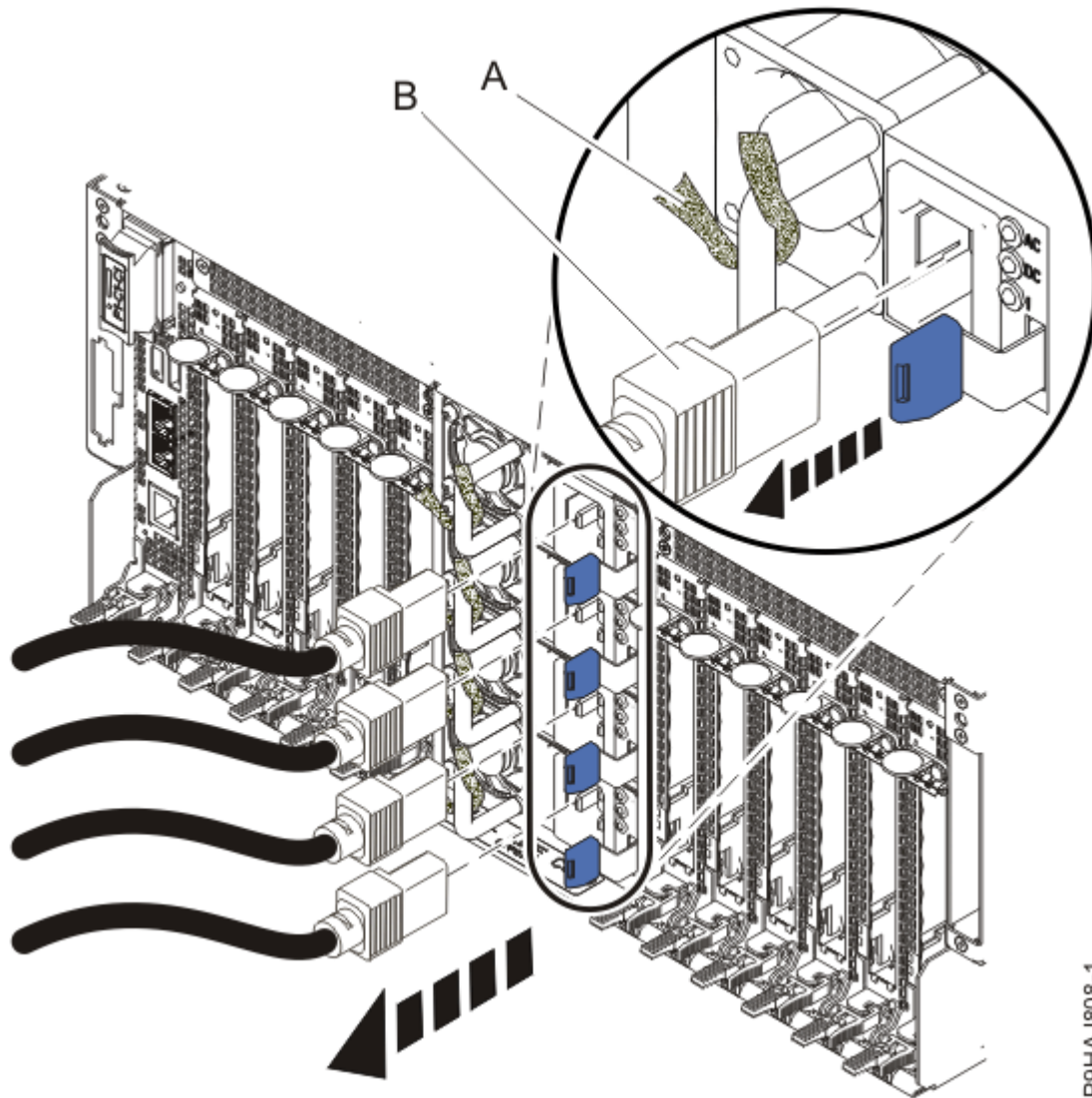
그림 1. 전원 코드 제거
