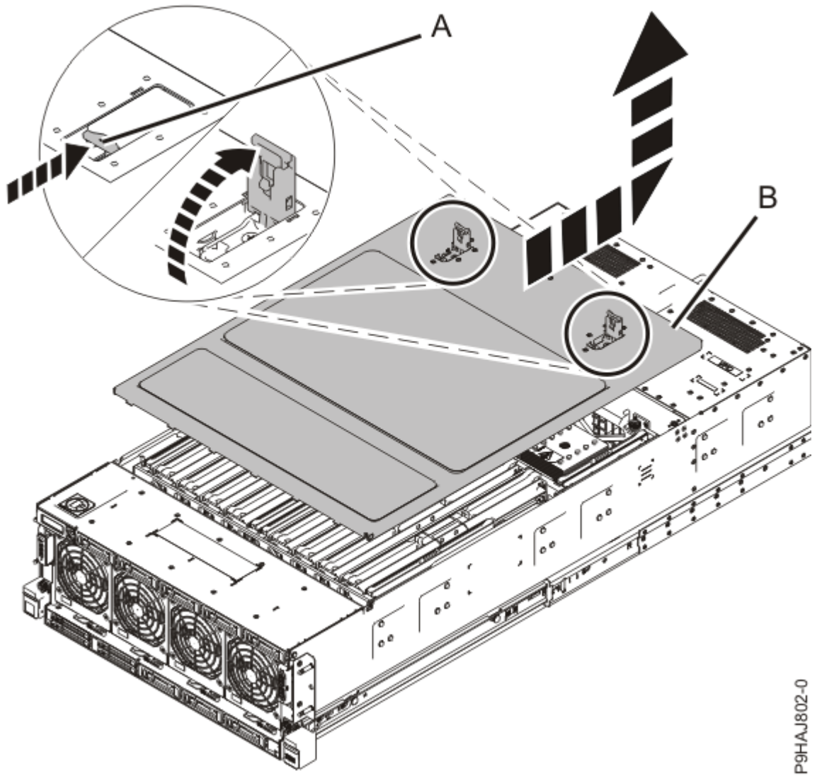
그림 4. 서비스 액세스 커버 제거
