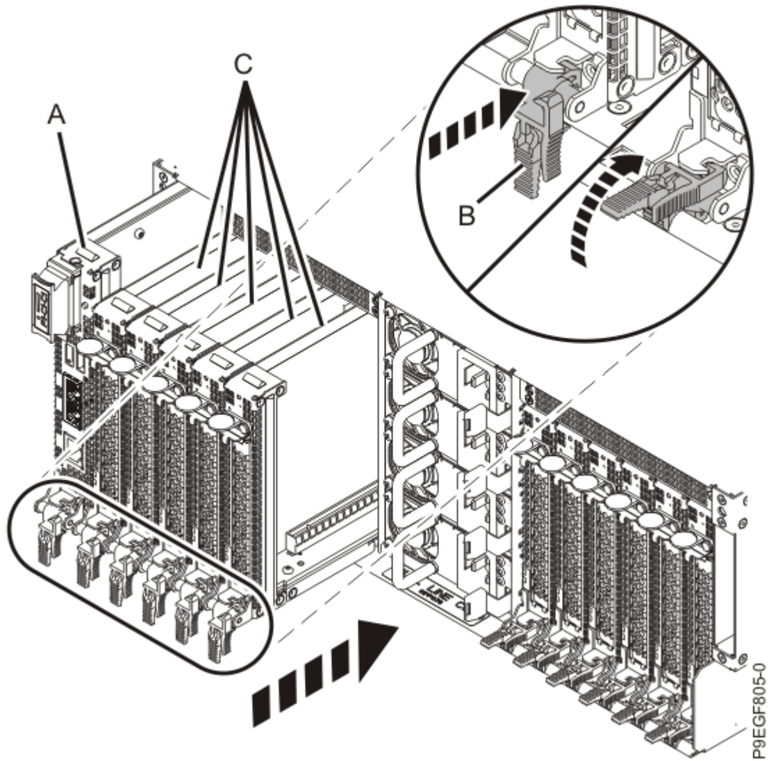
그림 15. 서비스 프로세서 카드 및 PCIe 카세트 교체
