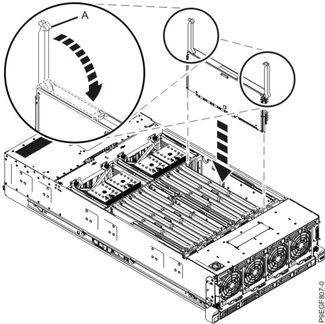
그림 12. 메모리 라이저에 설치
