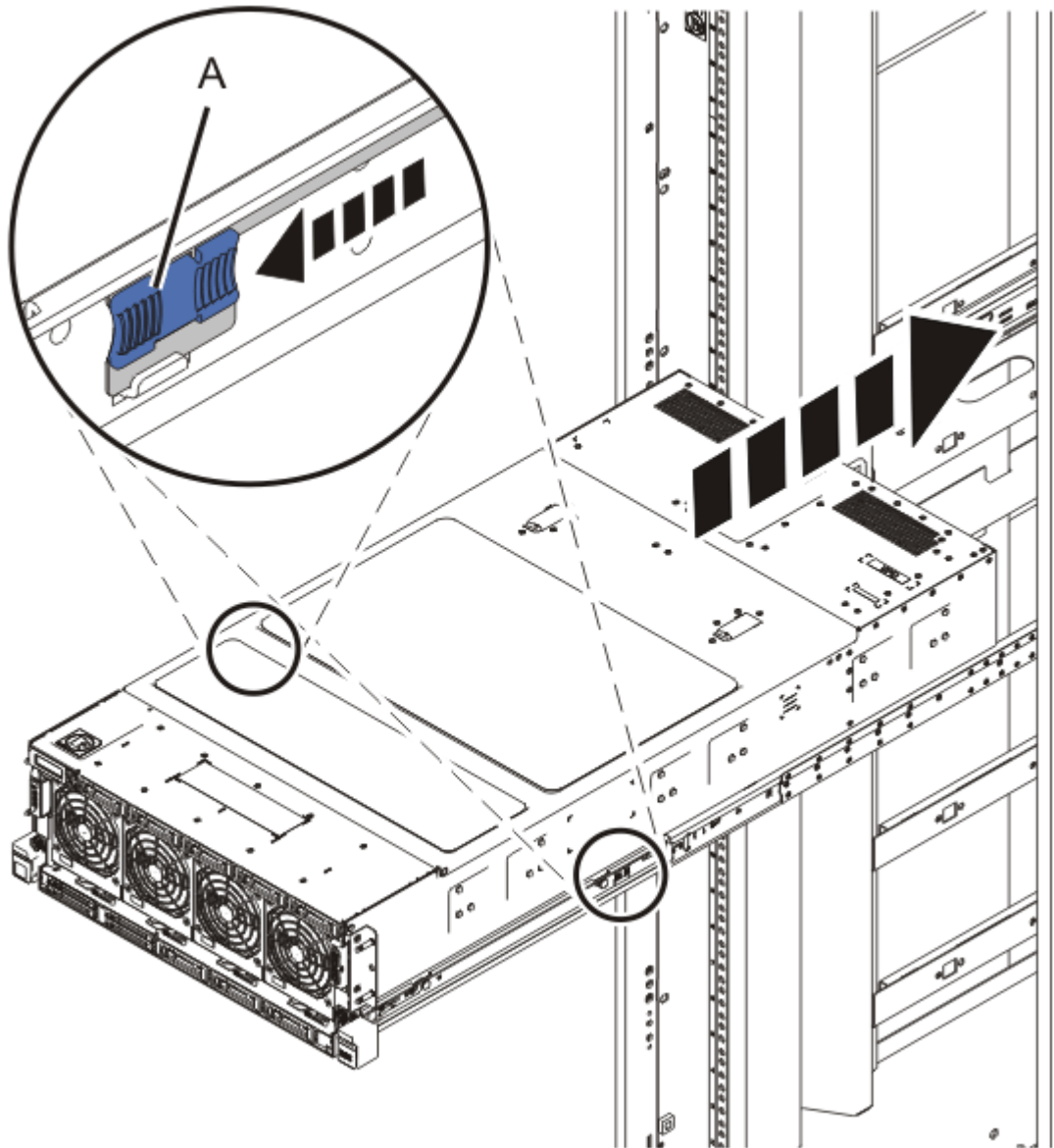
그림 7. 시스템을 작동 위치에 배치
