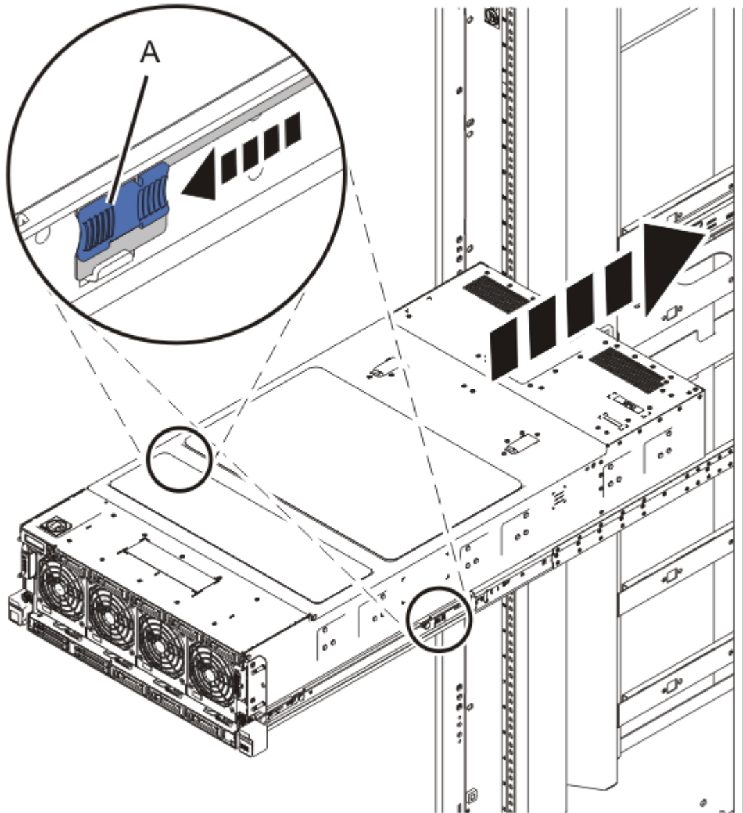
그림 14. 시스템을 작동 위치에 배치
