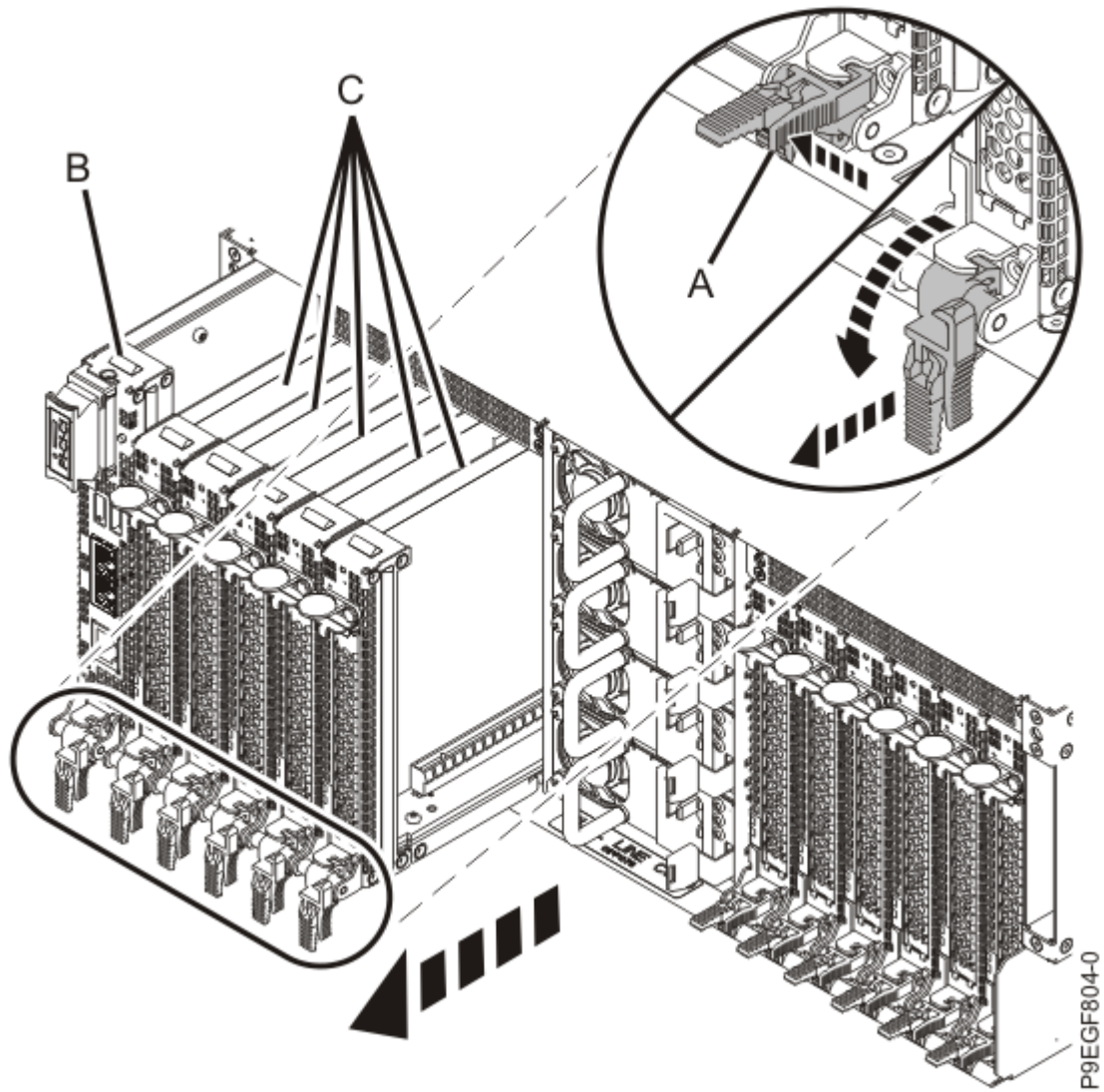
그림 2. 서비스 프로세서 카드 및 PCIe 카세트 제거
