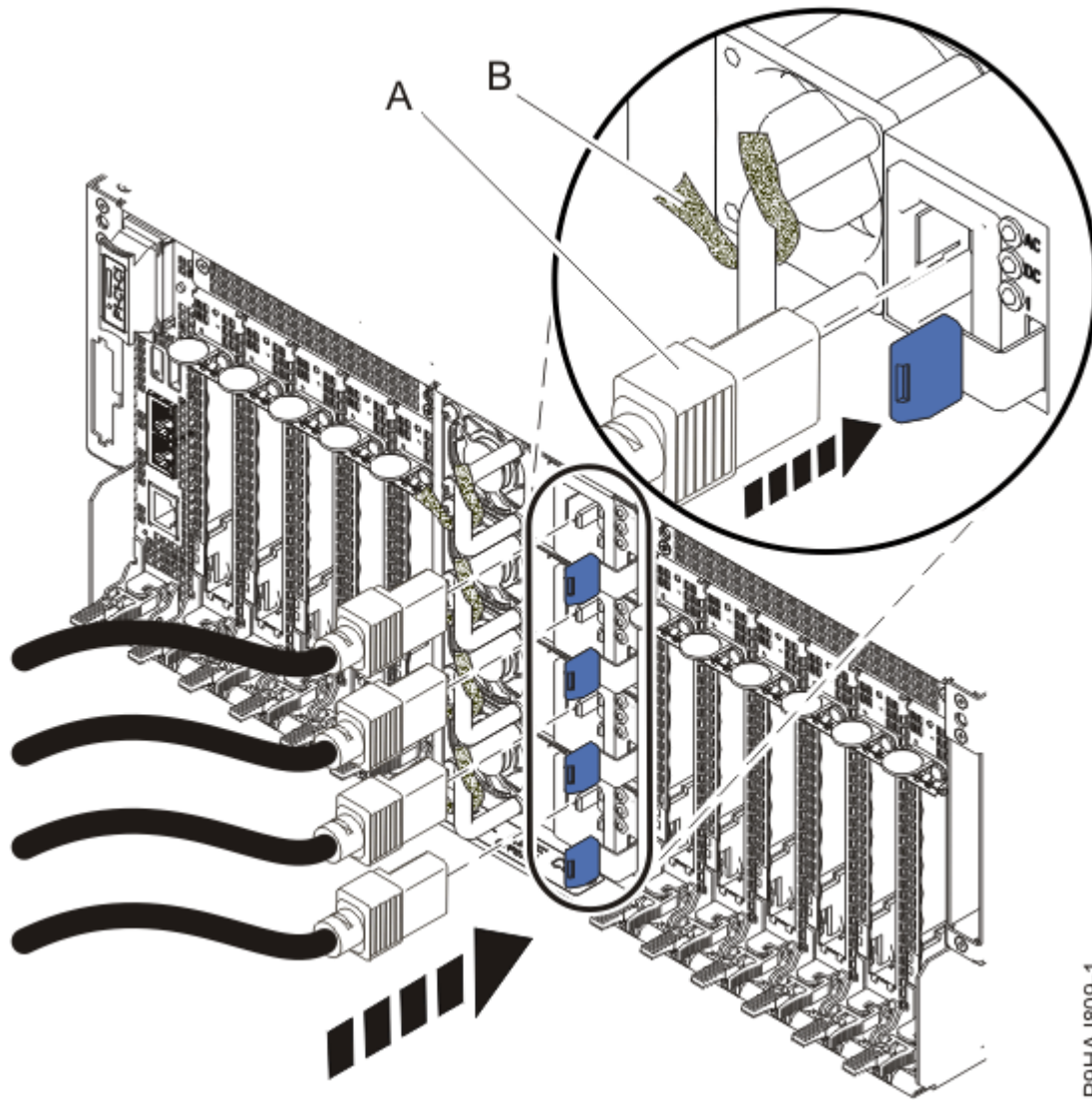
그림 16. 전원 코드 연결
