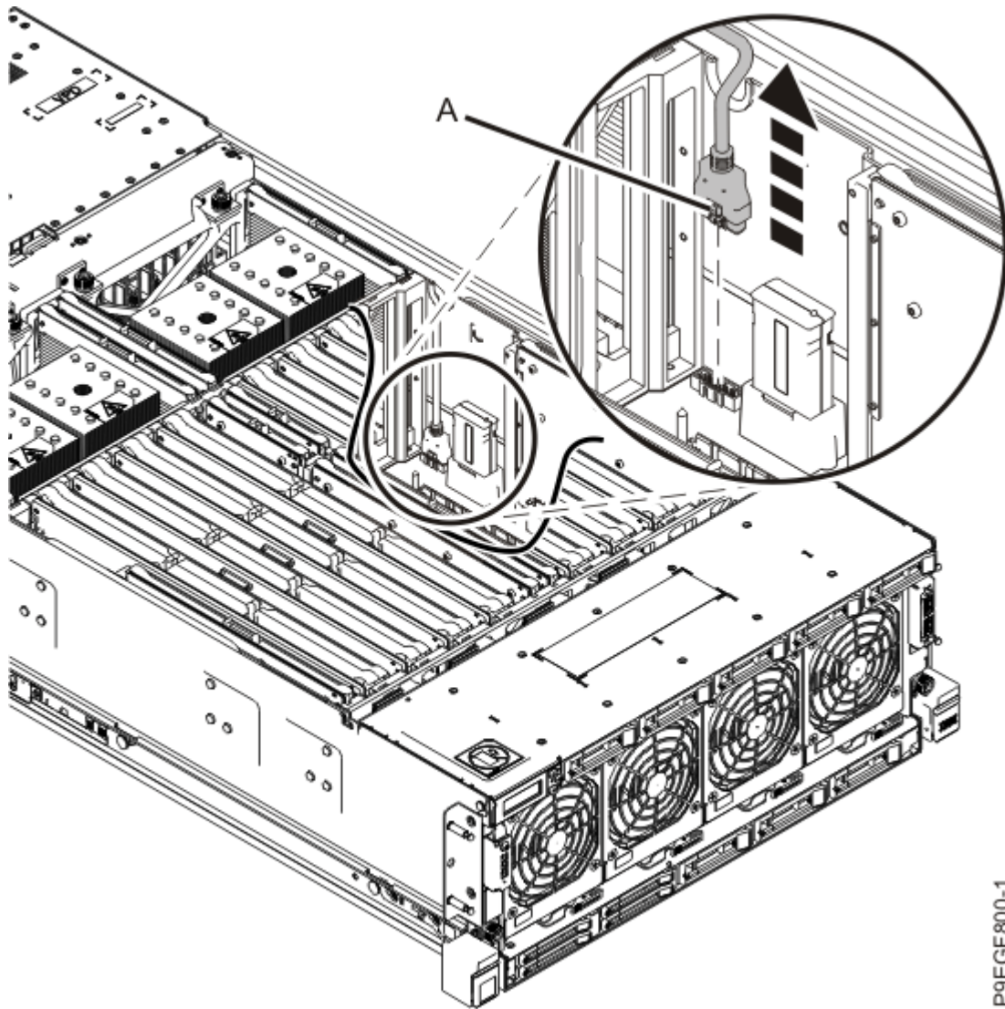
그림 6. 시스템 백플레인에서 뒷면 USB 케이블 제거
