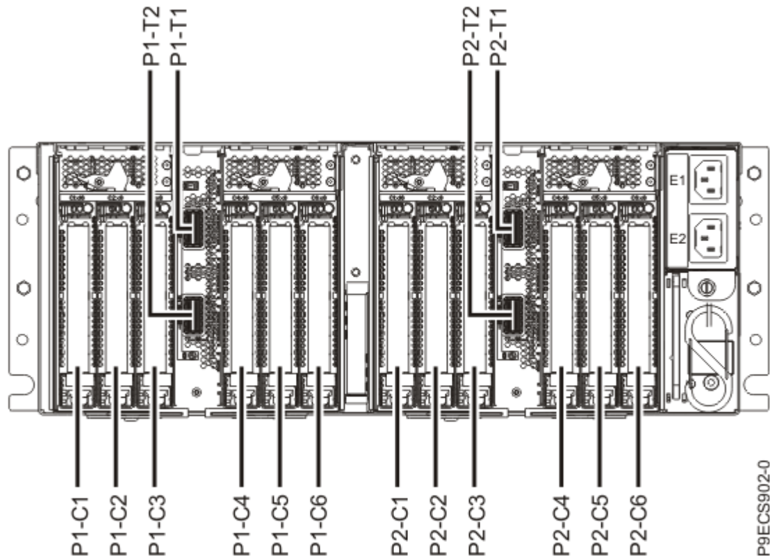
그림 2. PCIe 슬롯 위치 코드를 갖는 EMX0 PCIe3 확장 드로어의 뒷면 모습
