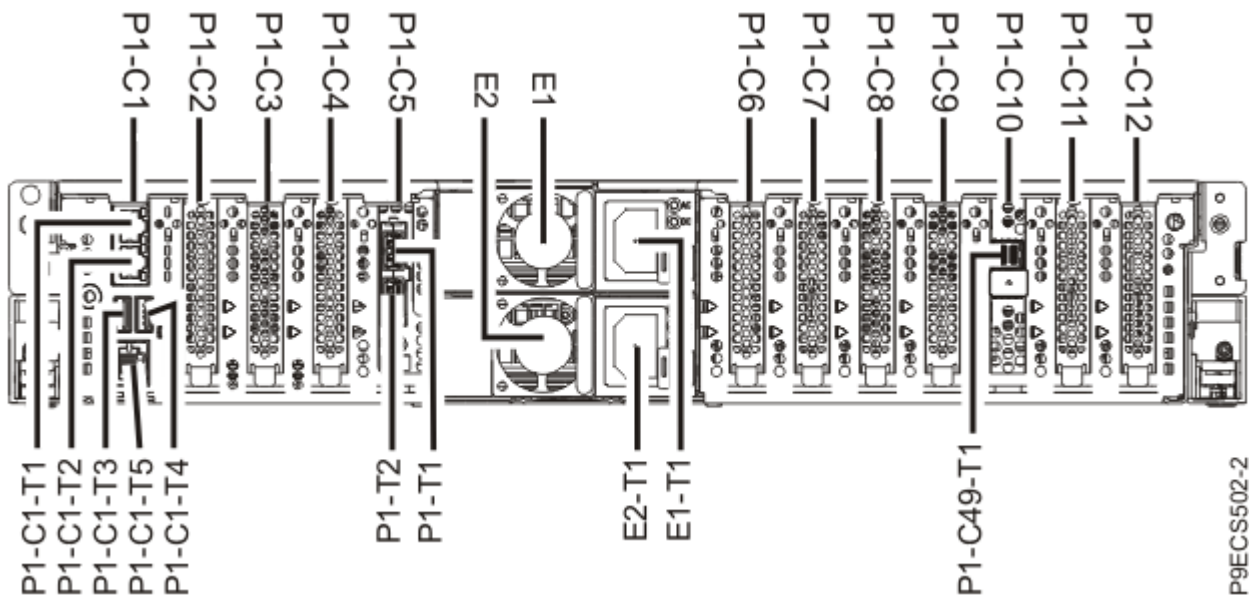
그림 2. PCIe 슬롯 위치 코드가 있는 랙 장착형 9008-22L, 9009-22A 또는 9223-22H 시스템의 뒷면 보기
