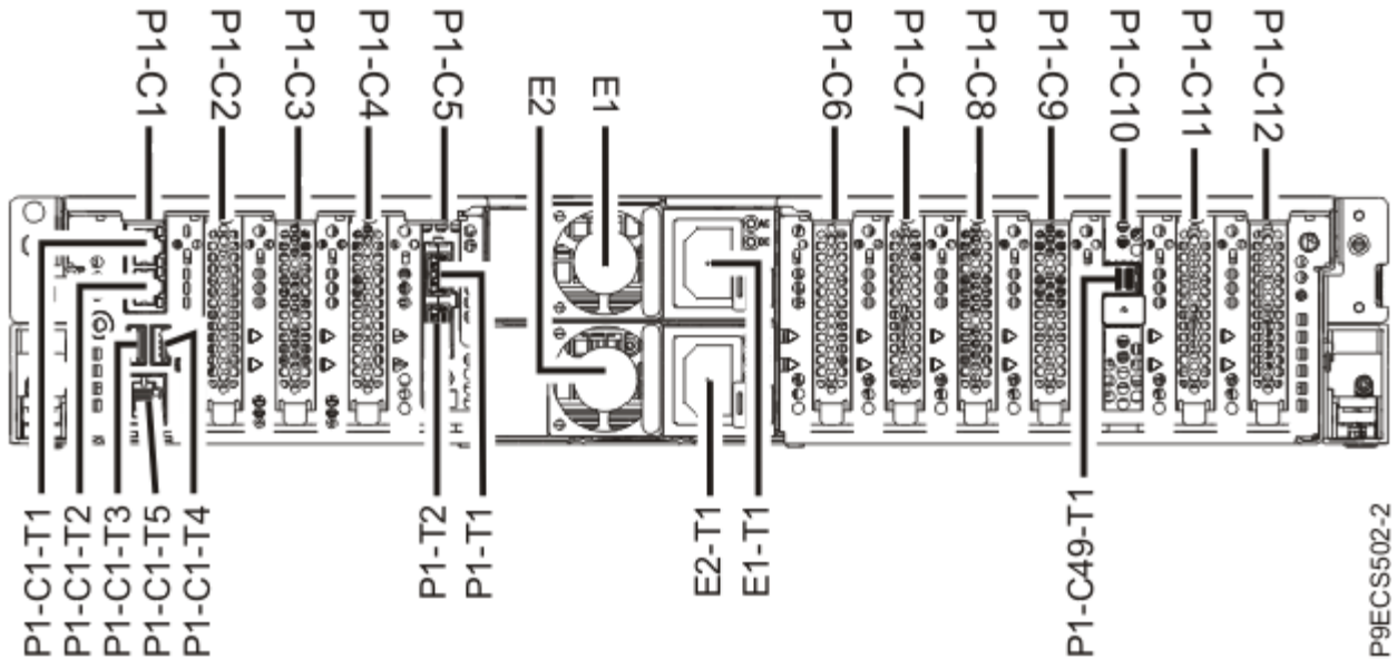
그림 1. PCIe4 슬롯 위치 코드가 있는 랙 장착형 5105-22E, 9009-22G 또는 9223-22S 시스템의 뒷면 보기
