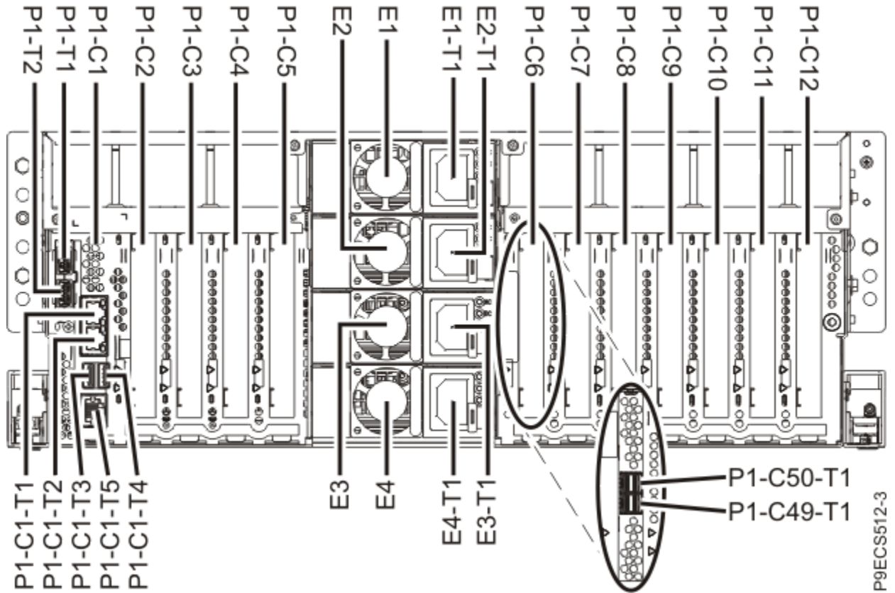
그림 2. PCIe 슬롯 위치 코드가 있는 랙 장착형 9009-41A, 9009-42A 및 9223-42H 시스템의 뒷면 보기
