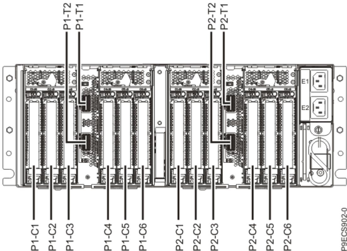
그림 3. PCIe 슬롯 위치 코드를 갖는 EMX0 PCIe3 확장 드로어의 뒷면 모습
