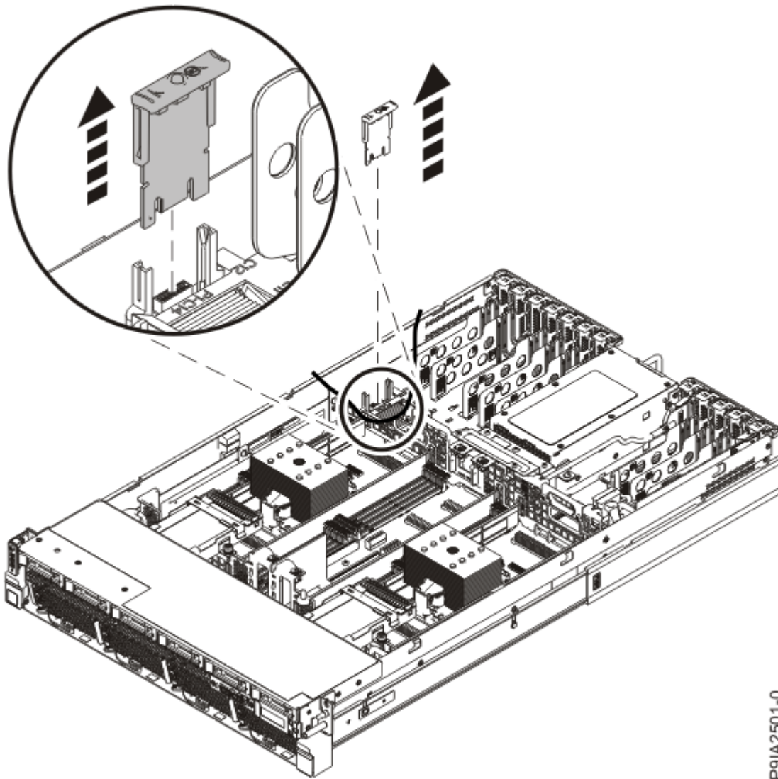
図 6. TPM カードの取り外し
