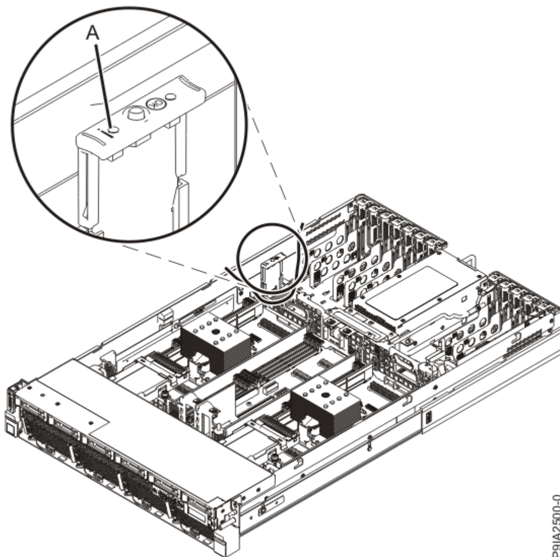
図 5. サービス・インジケータ LED
