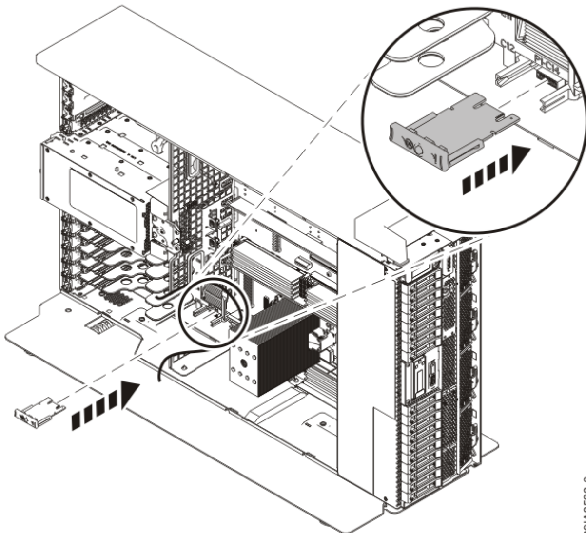
図 12. スタンドアロン・システムの TPM カードの再取り付け
