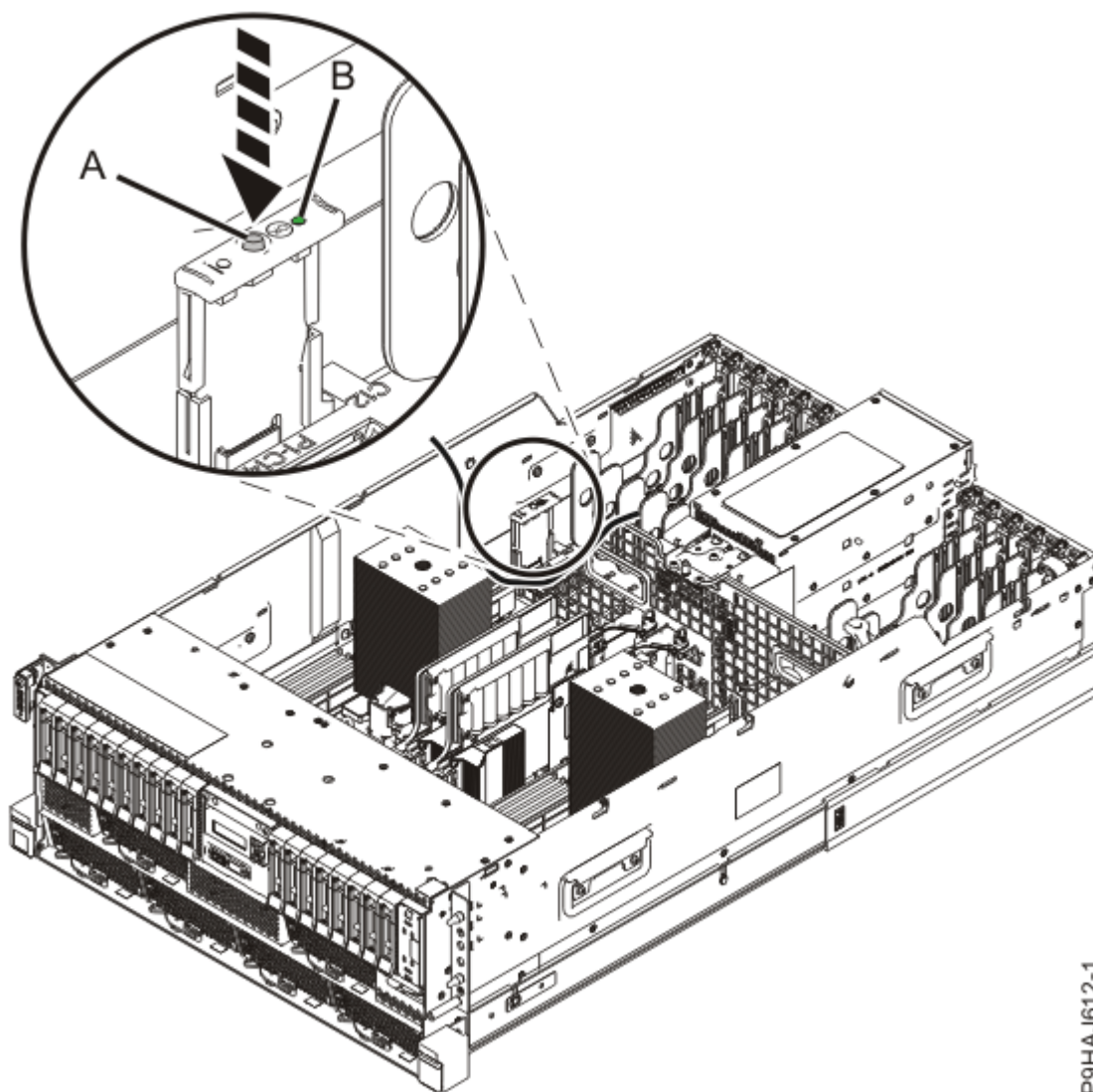
図 6. 識別 LED の活動化
