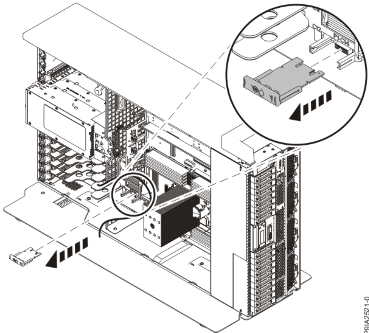
図 10. スタンドアロン・システムからの TPM カードの取り外し
