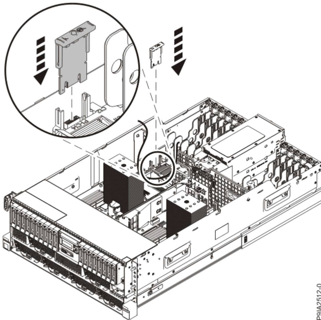
図 11. ラック・マウント型システムへの TPM カードの再取り付け
