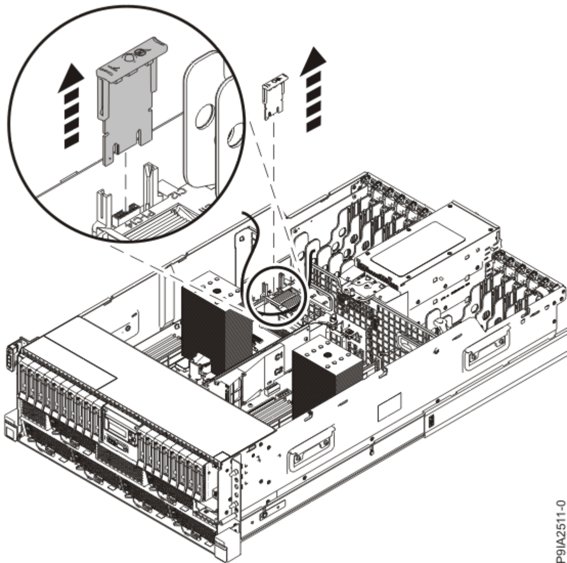
図 9. ラック・マウント型システムからの TPM カードの取り外し
