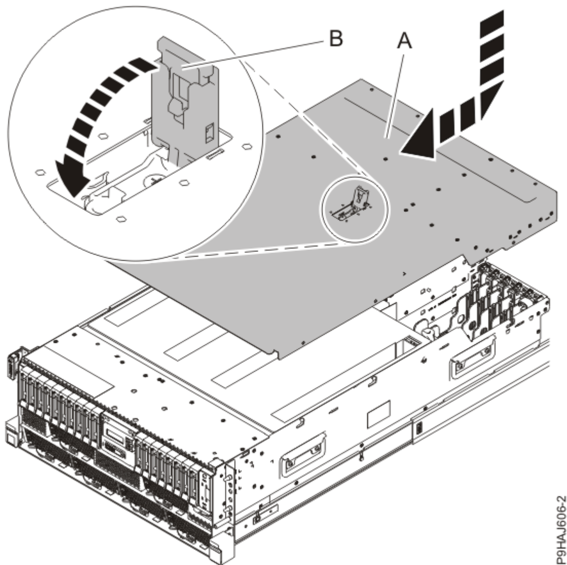
図 13. 保守アクセス・カバーの取り付け
