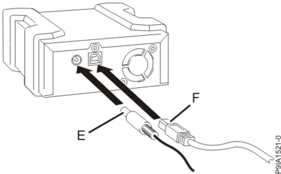
図 3. 外付け RDX ドッキング・ステーションの背面図とそのケーブル
