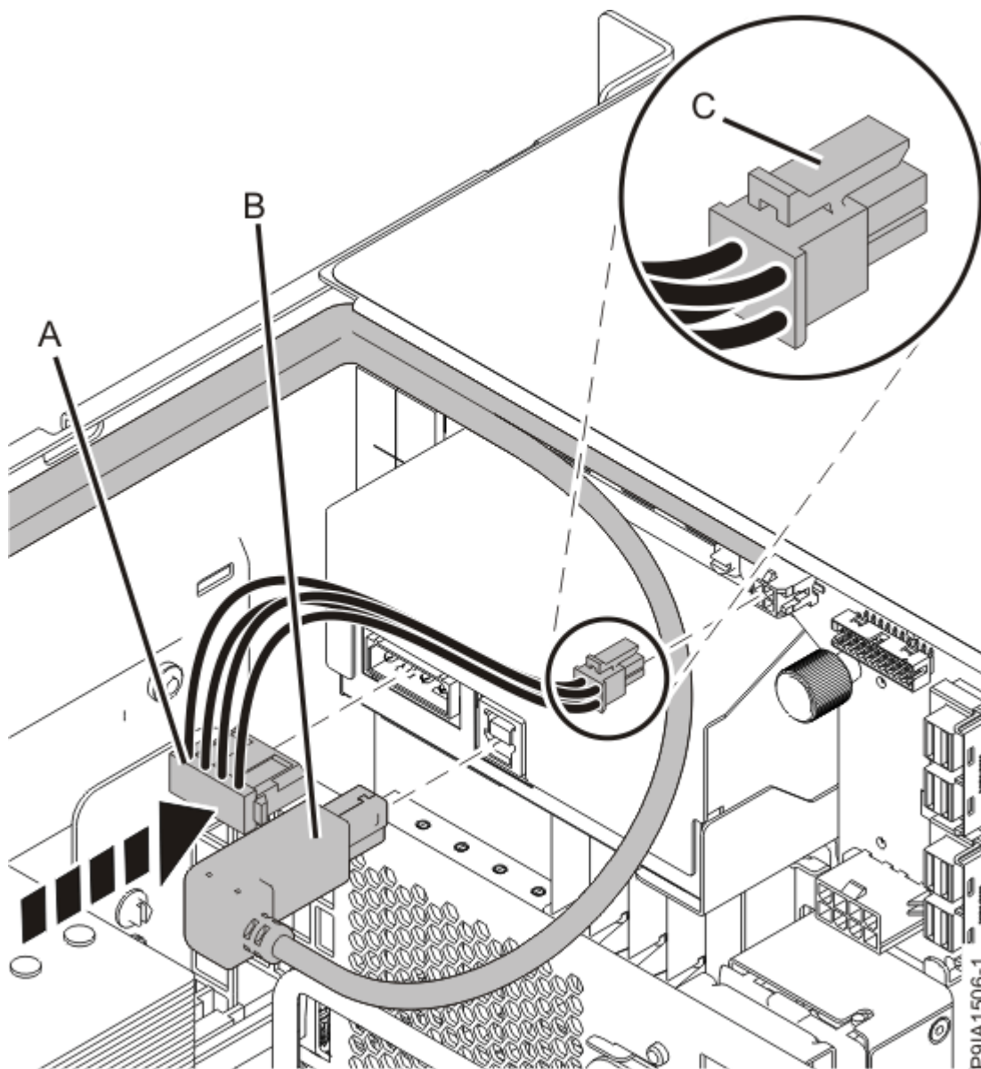
図 38. 内蔵 RDX ドッキング・ステーションの電源および USB ケーブルの接続
