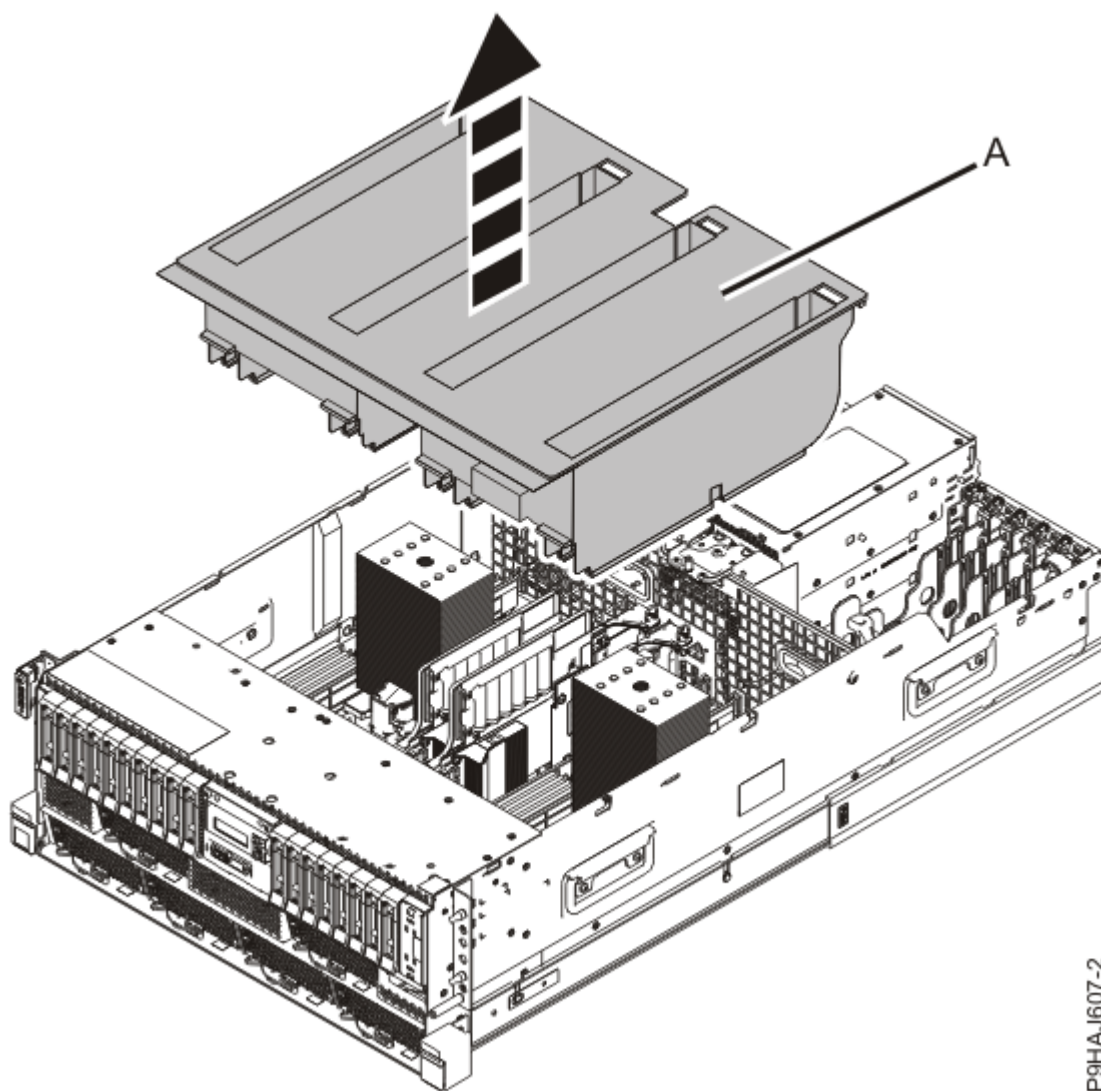
図 8. ラック・マウント型システムからのエア・バッフルの取り外し
