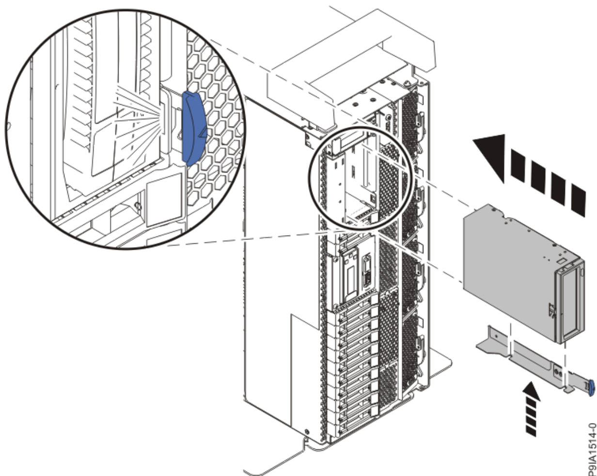
図 37. スタンドアロン・システムへの内蔵 RDX ドッキング・ステーションの再取り付け
