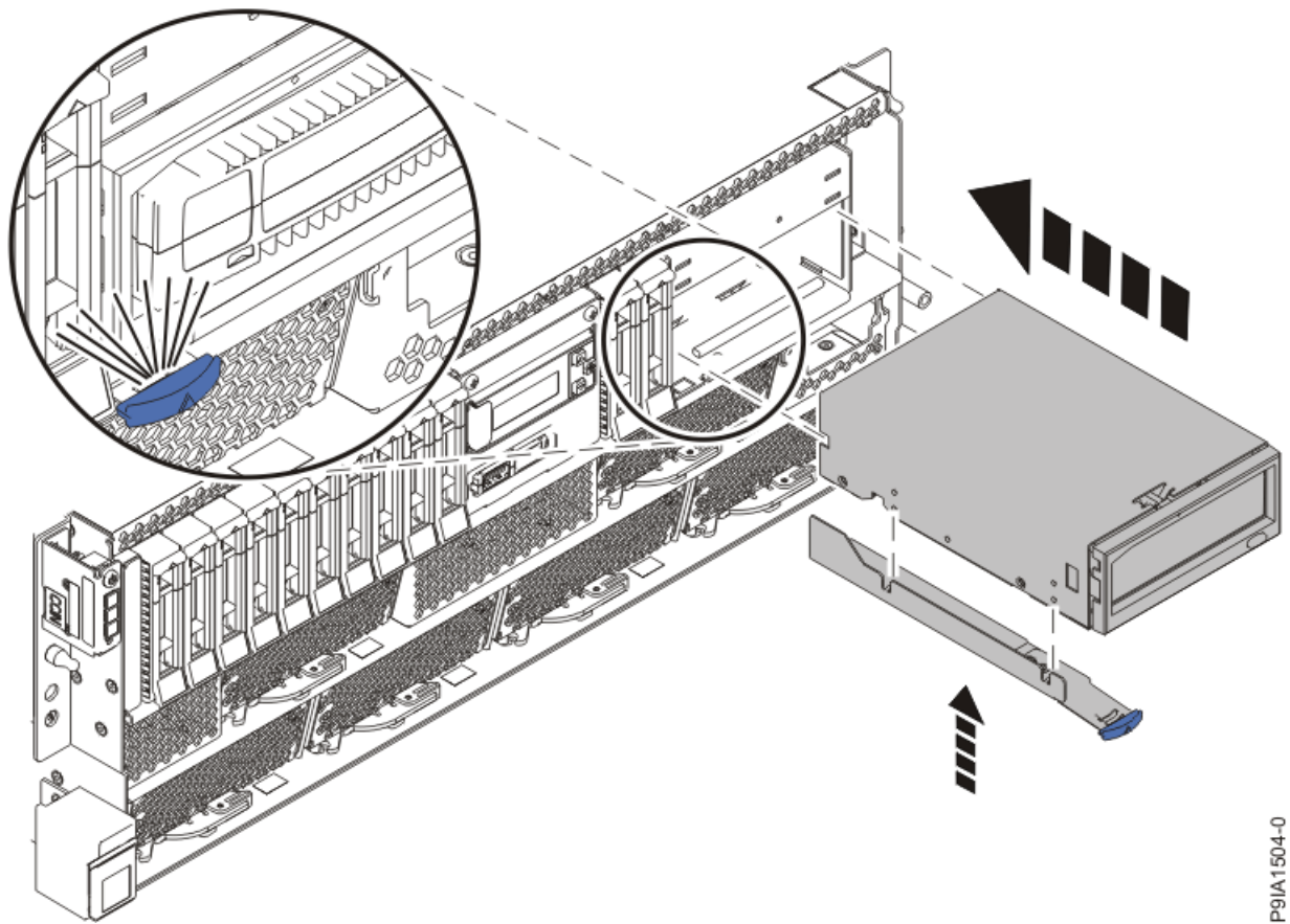
図 36. ラック・マウント型システムへの内蔵 RDX ドッキング・ステーションの再取り付け
