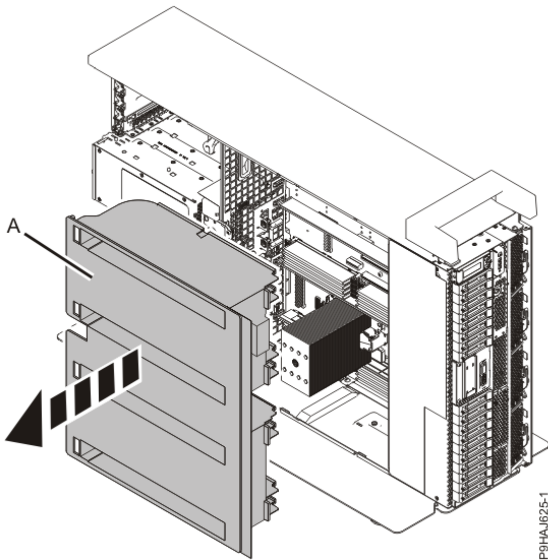
図 9. スタンドアロン・システムからのエア・バッフルの取り外し 4. 背面フィルターを取り外します (14 ページの図 10 を参照)。
