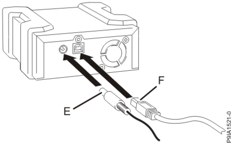
図 1. 外部 USB ケーブルおよび電源機構ケーブルの接続
