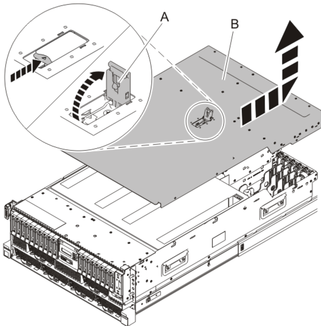
図 28. ラック・マウント型システムからの保守アクセス・カバーの取り外し
