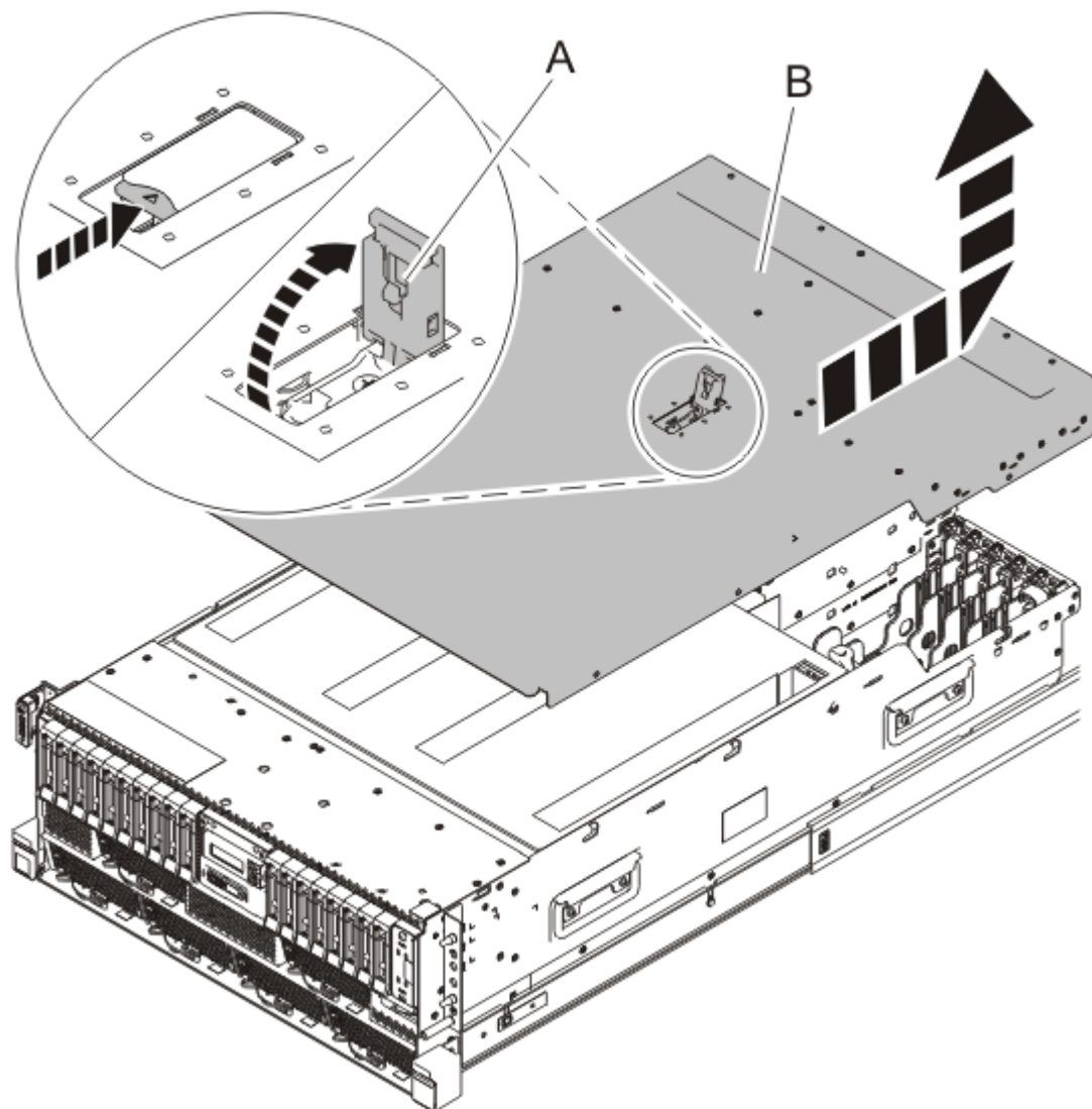
図 50. ラック・マウント型システムからの保守アクセス・カバーの取り外し
