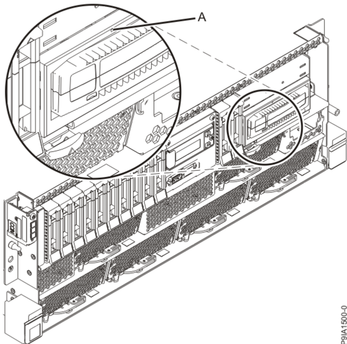
図 66. 内蔵 RDX ドッキング・ステーションおよび取り外し可能ディスク・ドライブの正面図
