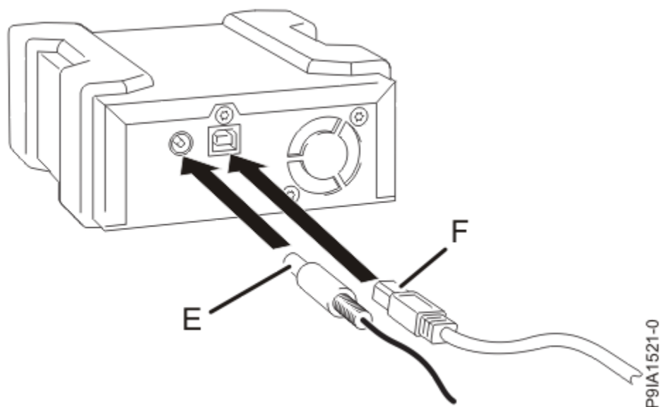
図 68. 外付け RDX ドッキング・ステーションの背面図とそのケーブル
