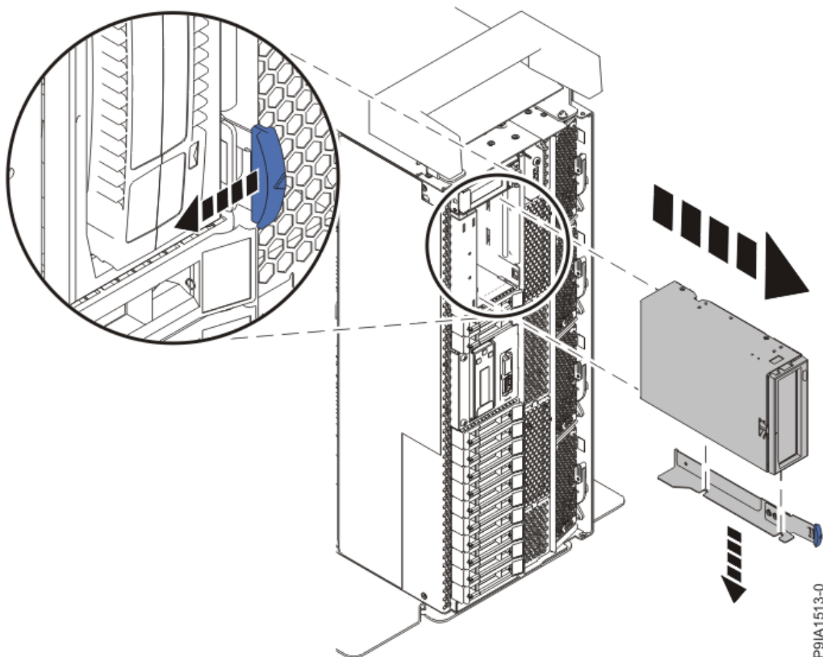
図 35. スタンドアロン・システムからの内蔵 RDX ドッキング・ステーションの取り外し
