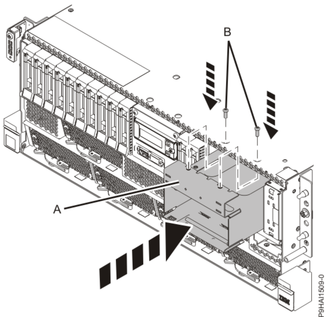
図 12. ラック・マウント型システムへの内蔵 RDX ドッキング・ステーション・スリーブの取り付け
