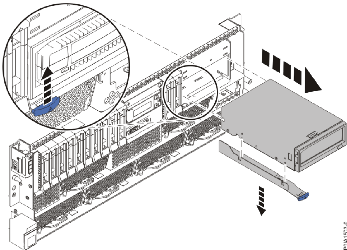
図 34. ラック・マウント型システムからの内蔵 RDX ドッキング・ステーションの再取り外し
