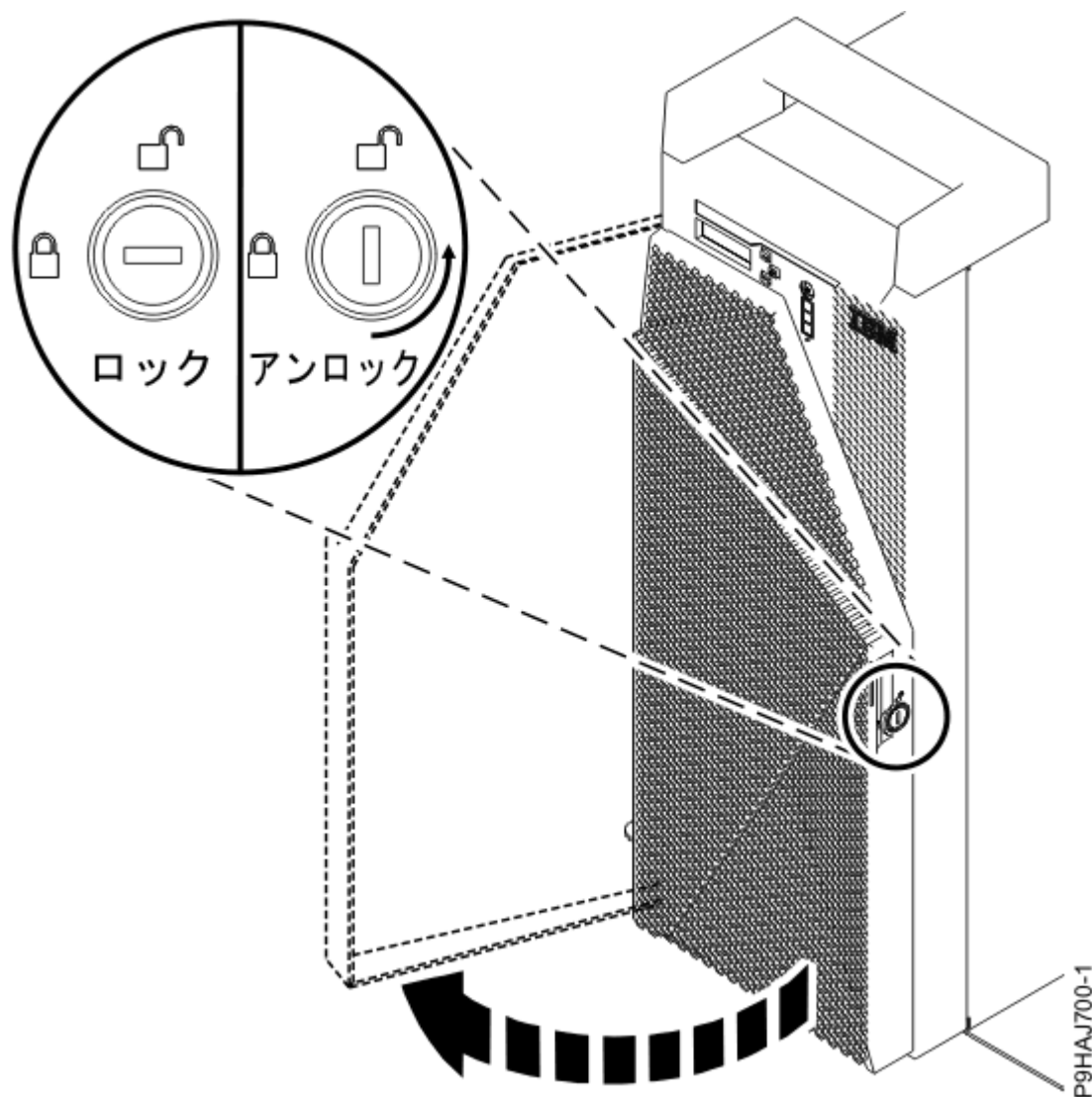
図 32. 前面ドアのアンロック
