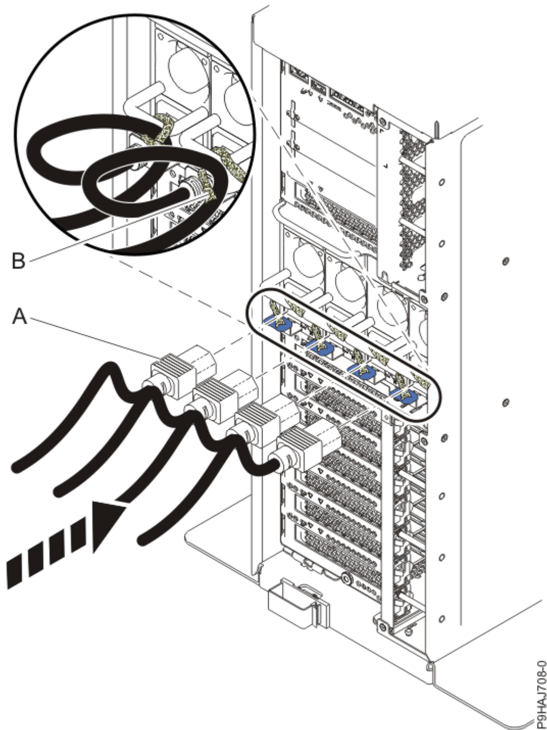
図 24. スタンドアロン・システムへの電源コードの接続
