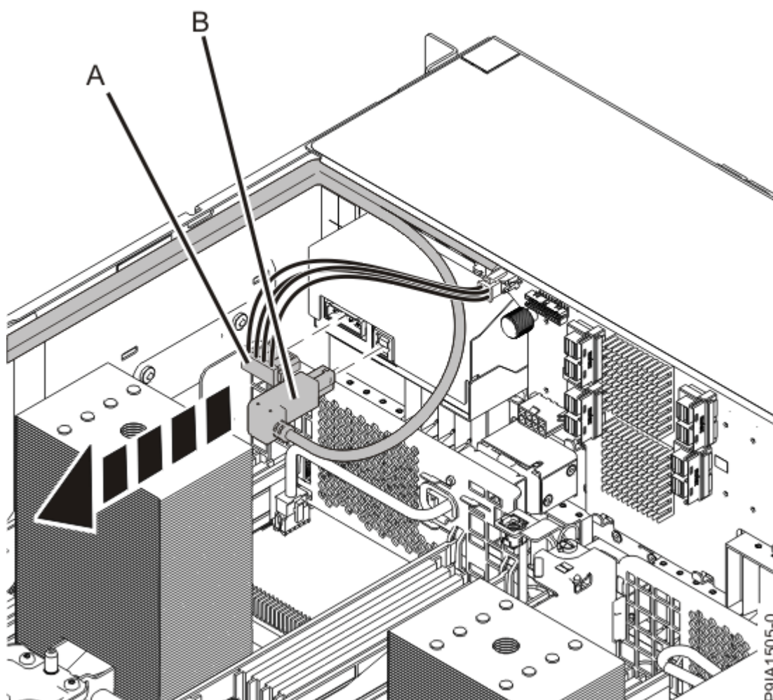
図 33. 内蔵 RDX ドッキング・ステーションの電源および USB ケーブルの切り離し
