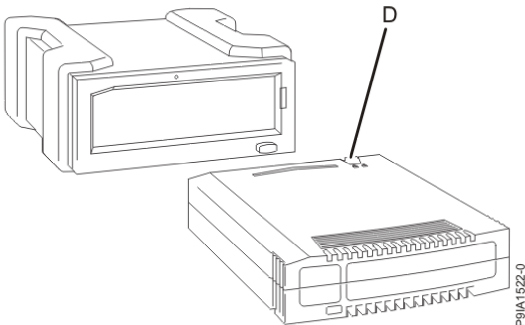
図 67. 外付け USB ドッキング・ステーションおよび取り外し可能ディスク・ドライブ・カートリッジの正面図
