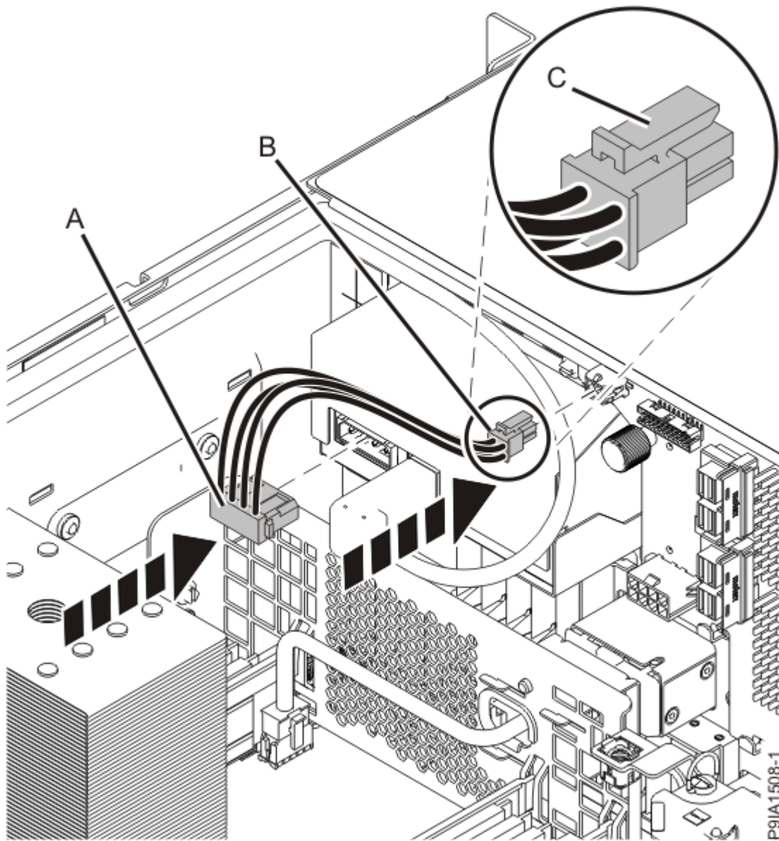
図 55. 内蔵 RDX 電源ケーブルの接続
