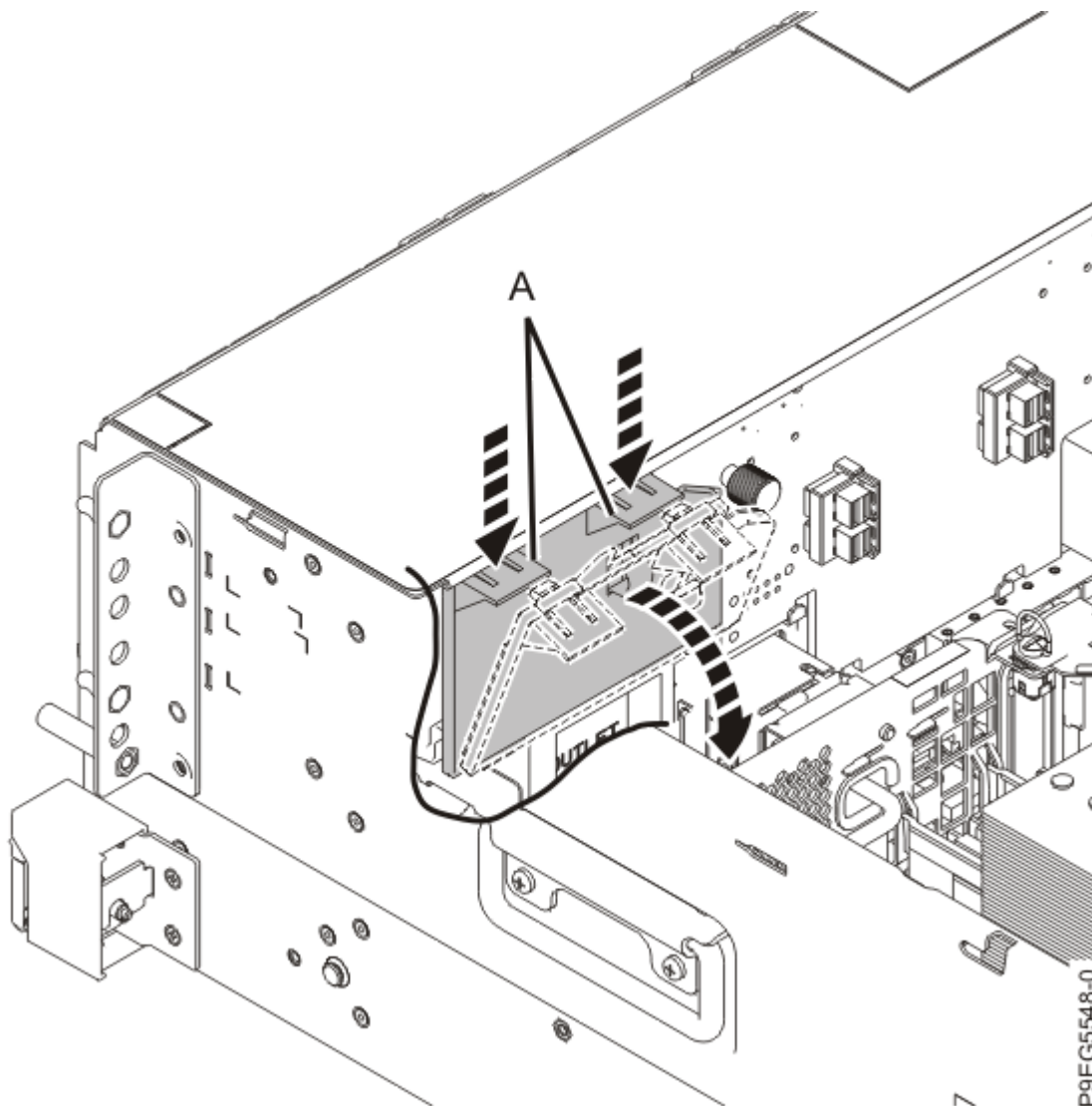
図 10. 内蔵 RDX ドッキング・ステーション背面フィラーの取り外し 5. 直接アクセス・ストレージ・デバイス (DASD) フィラーを取り外します (15 ページの図 11 を参照)。
