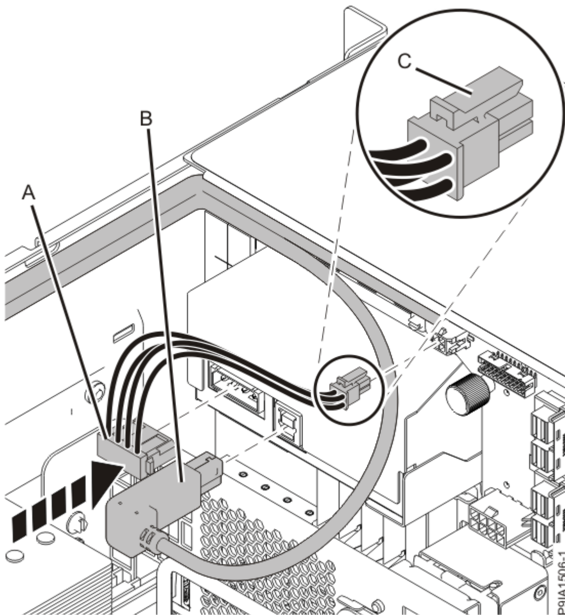
図 16. 内蔵 RDX ドッキング・ステーションの電源および USB ケーブルの接続
