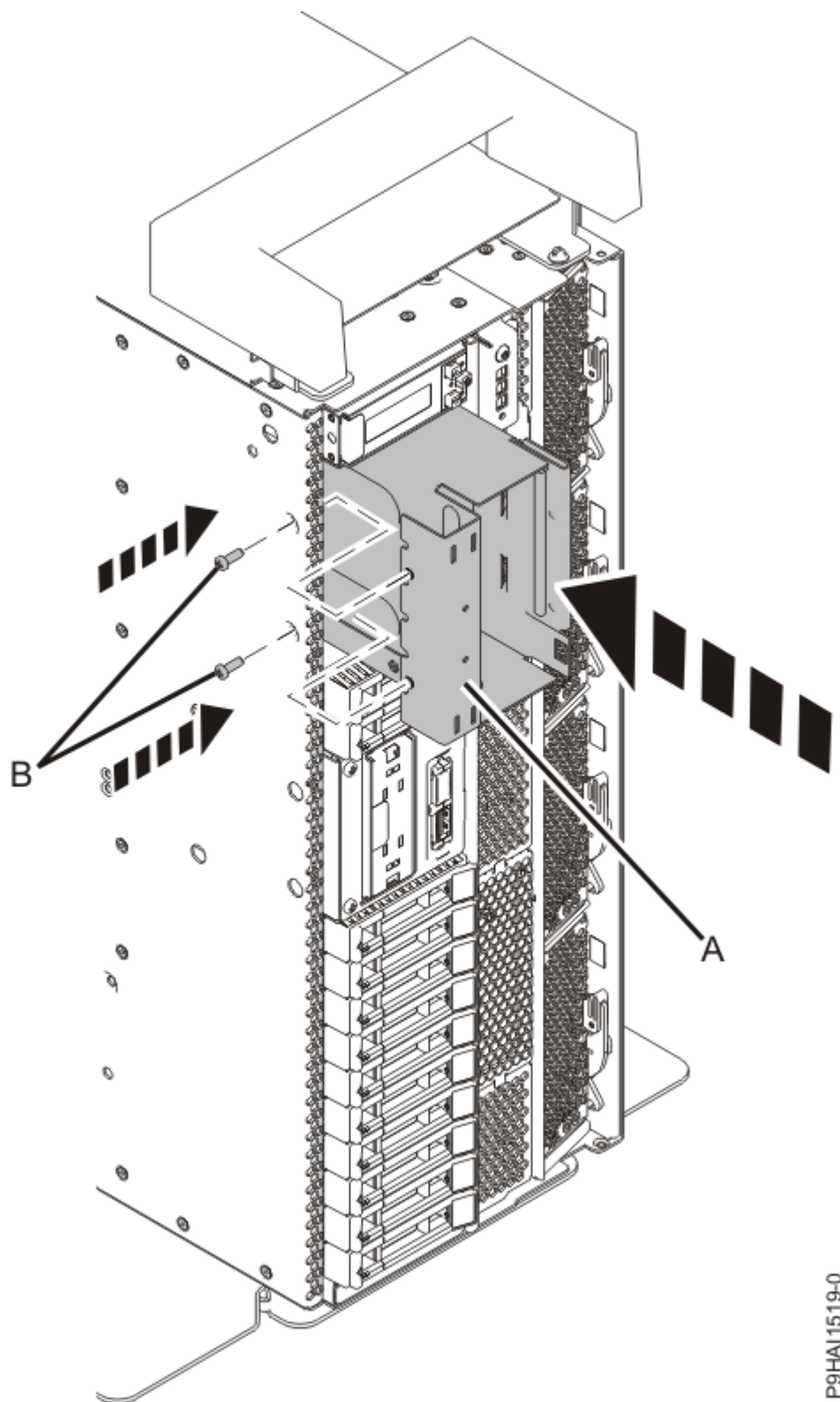
図 13. スタンドアロン・システムへの内蔵 RDX ドッキング・ステーション・スリーブの取り付け
