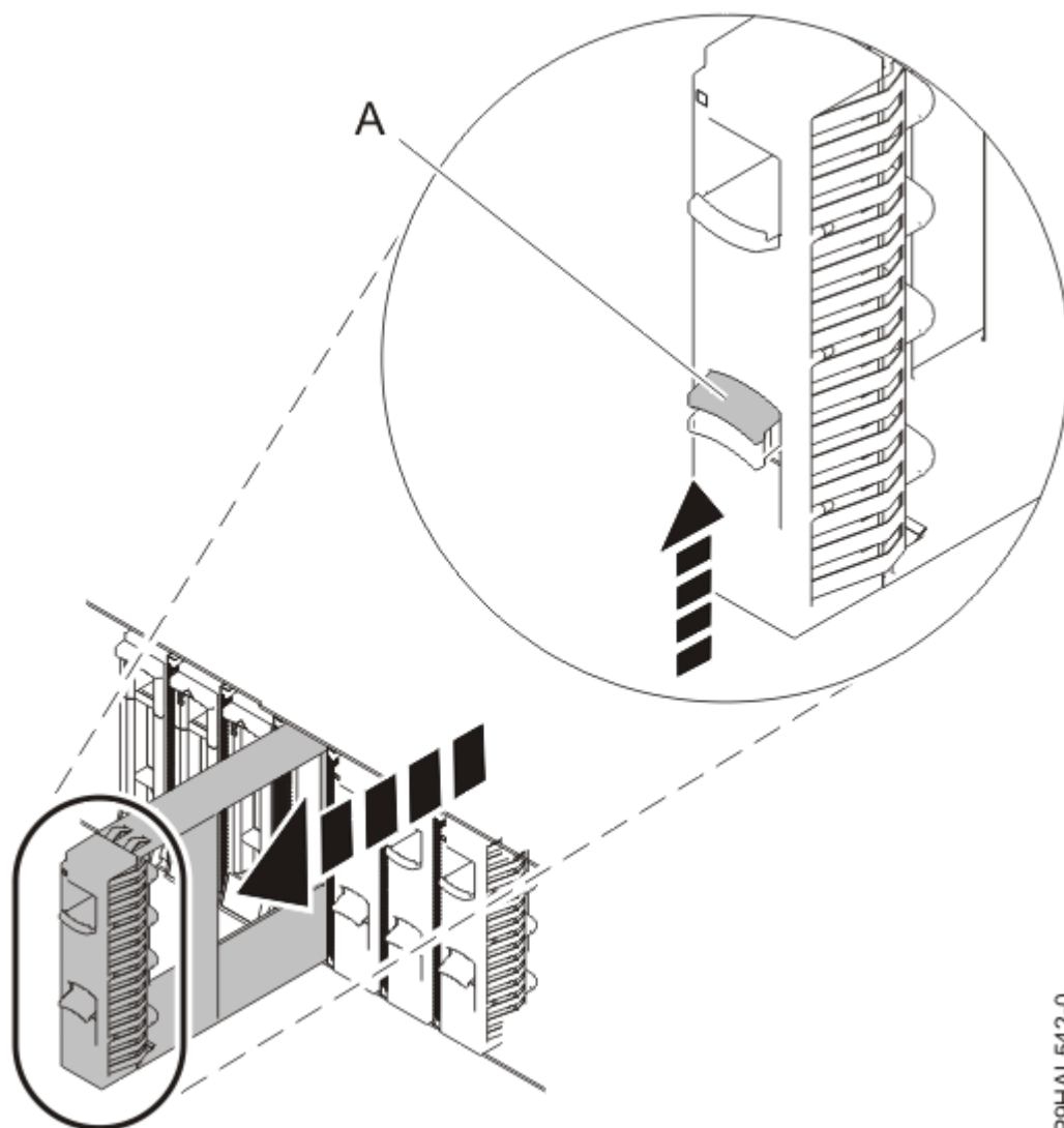
図 11. DASD フィラーの取り外し
