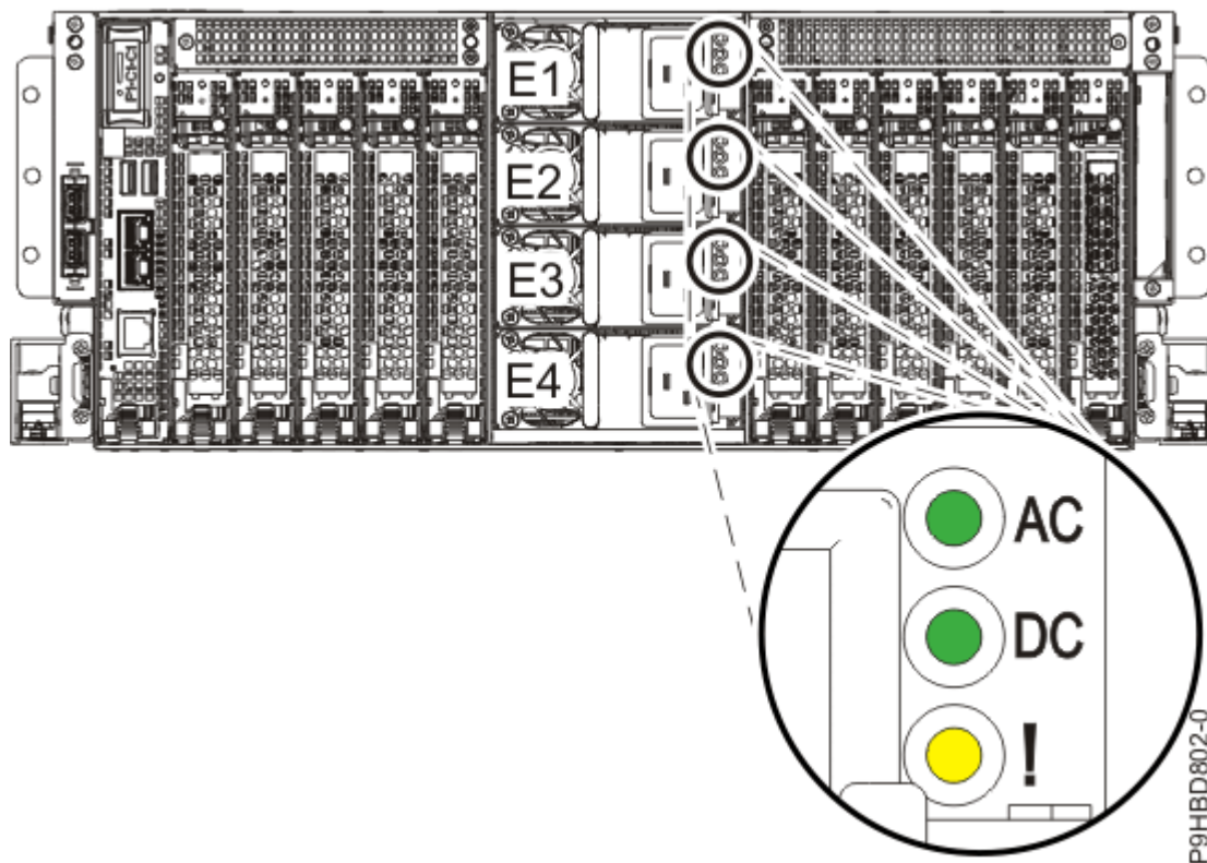
図 1. 電源装置と LED の位置
