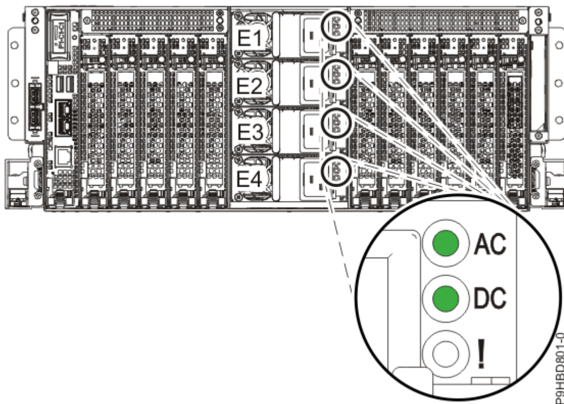
図 6. 動作中の電源装置の LED
