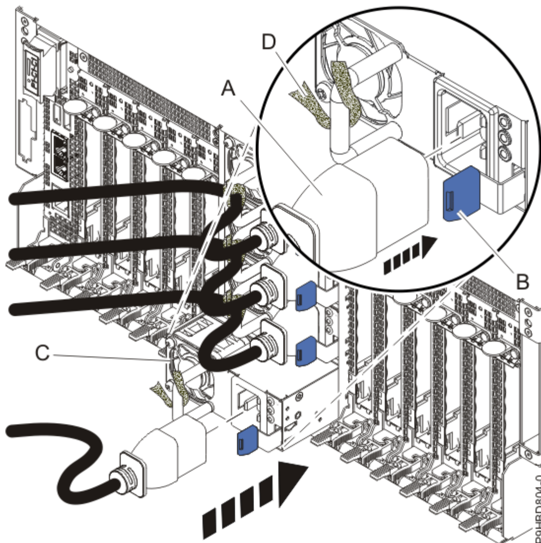
図 5. 電源装置の再取り付け
