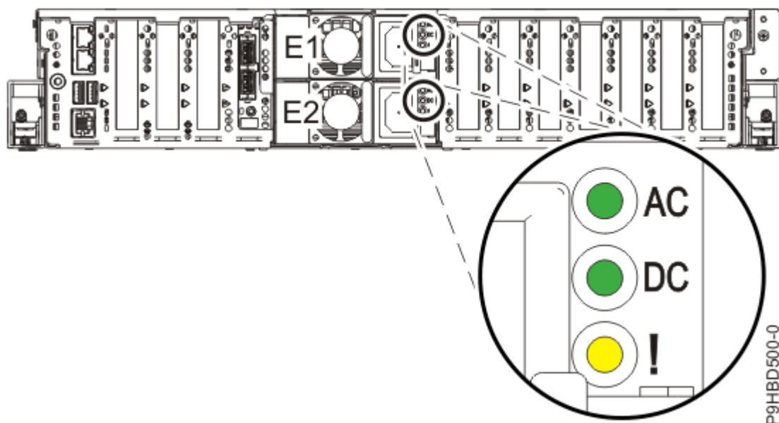
図 1. システムの電源装置と LED の位置
