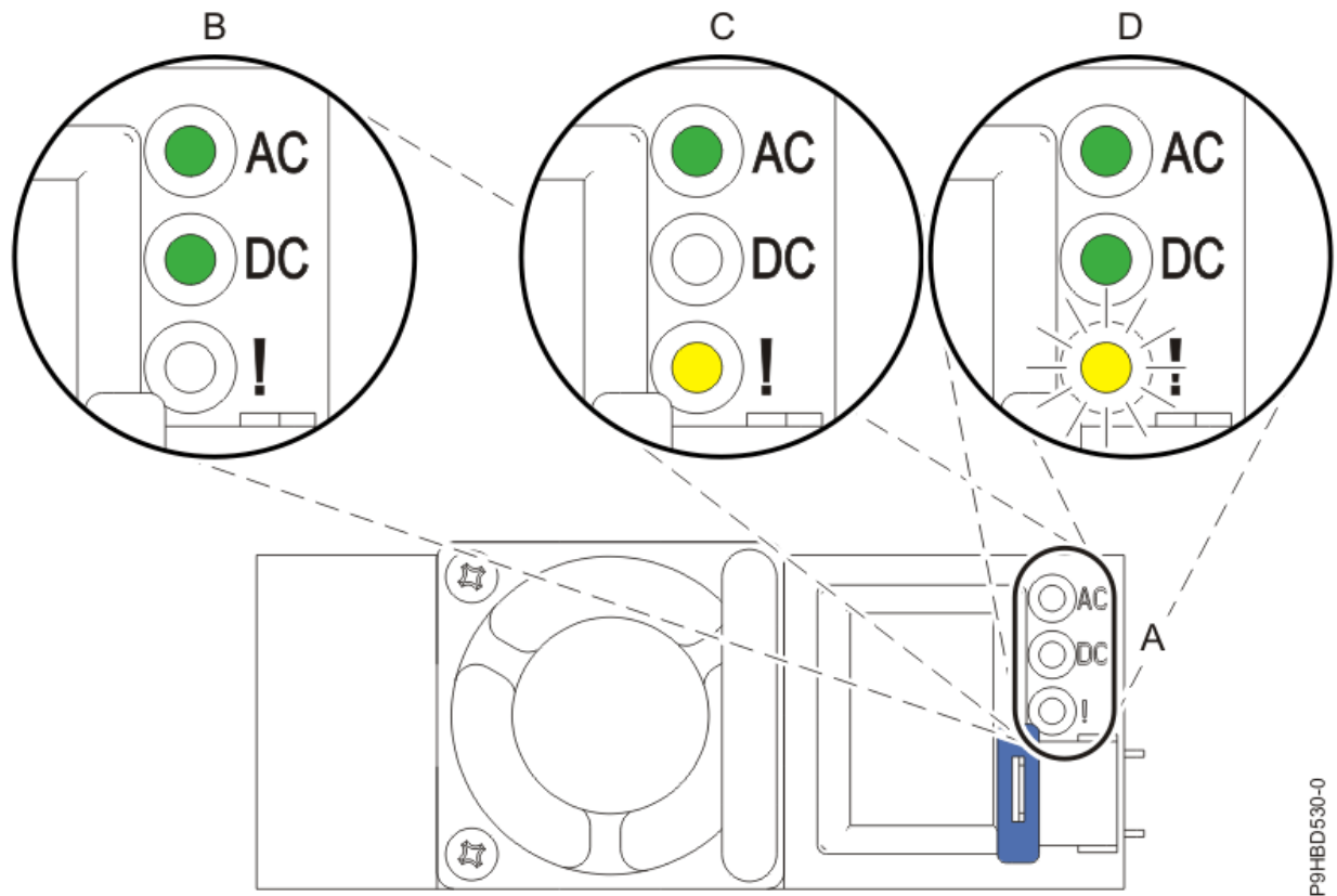
図 2. 動作中 (B) 電源装置および障害が発生した (C、D) 電源装置の LED
