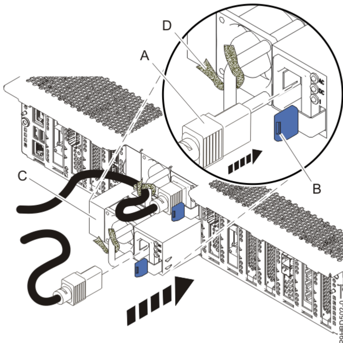
図 6. 電源装置の再取り付け
