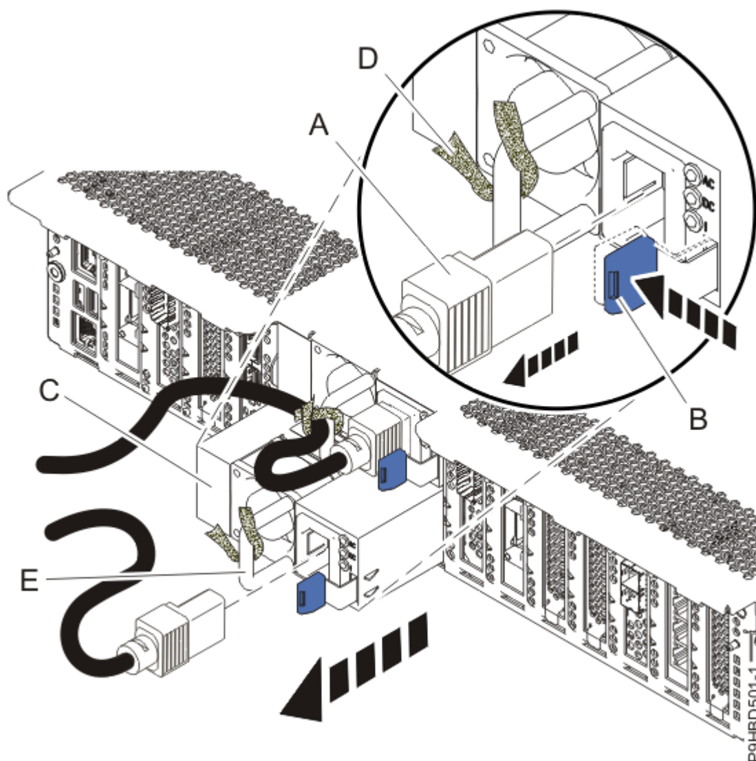
図 5. 電源装置の取り外し
