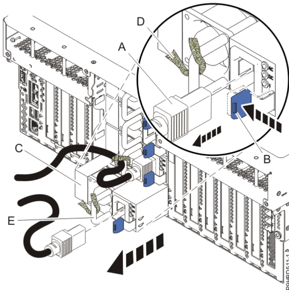
図 8. 電源装置の取り外し
