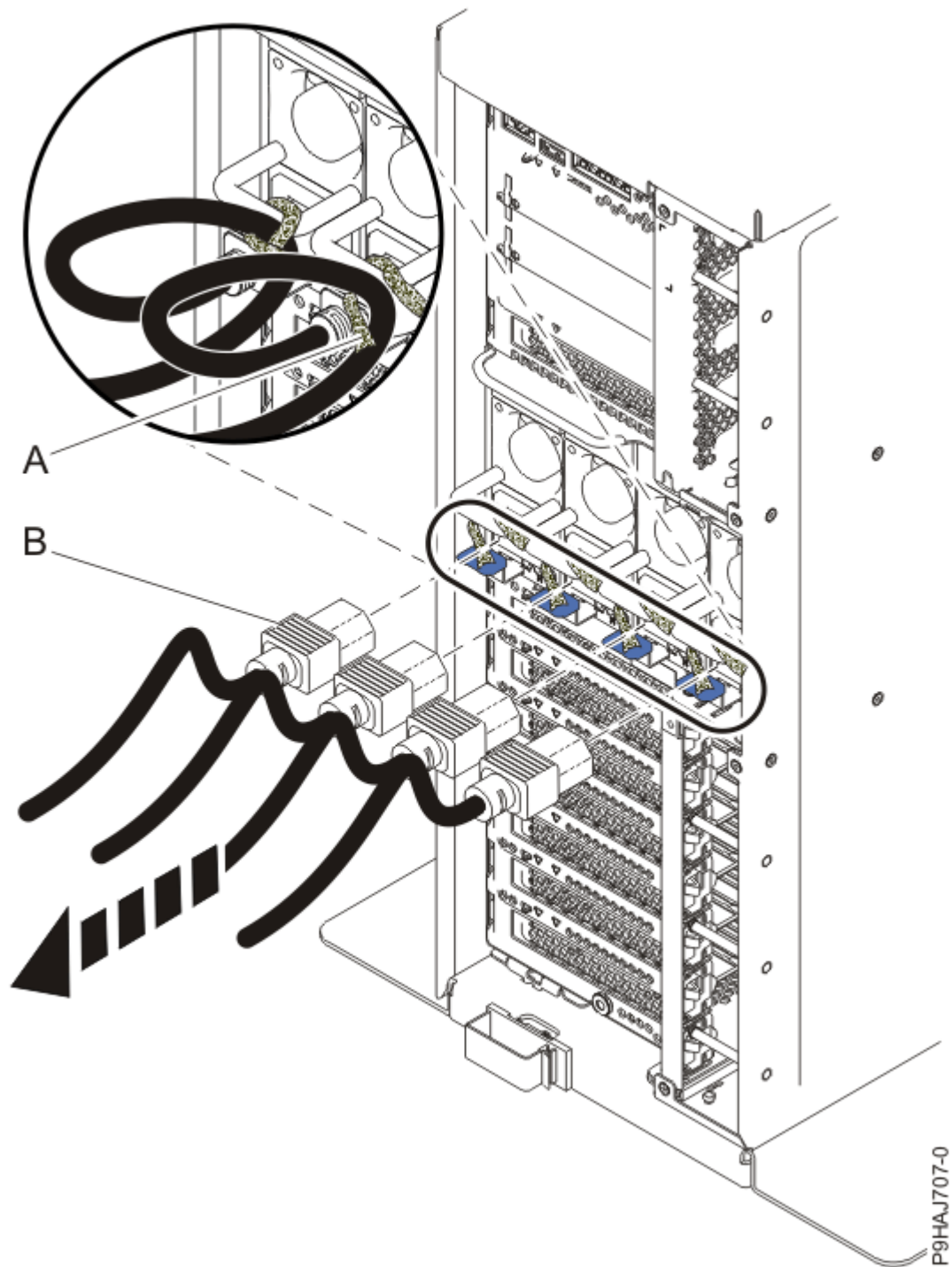
図 6. スタンドアロン型サーバーからの電源コードの取り外し
