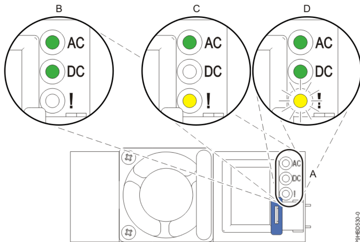
図 3. ラック・マウント型システムの動作中 (B) 電源装置および障害が発生した (C、D) 電源装置の LED
