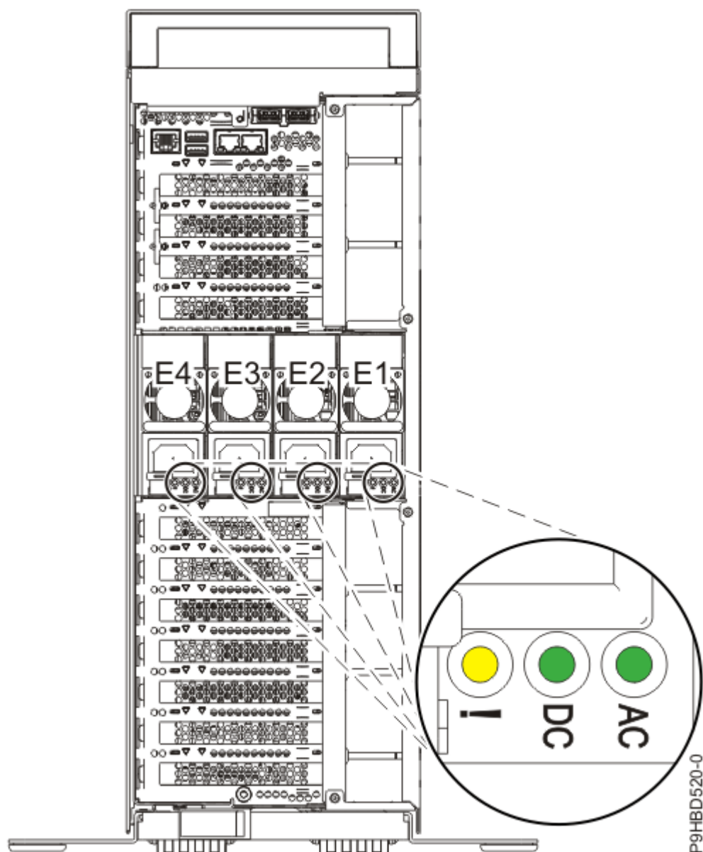
図 2. スタンドアロン・システムの電源装置と LED の位置
