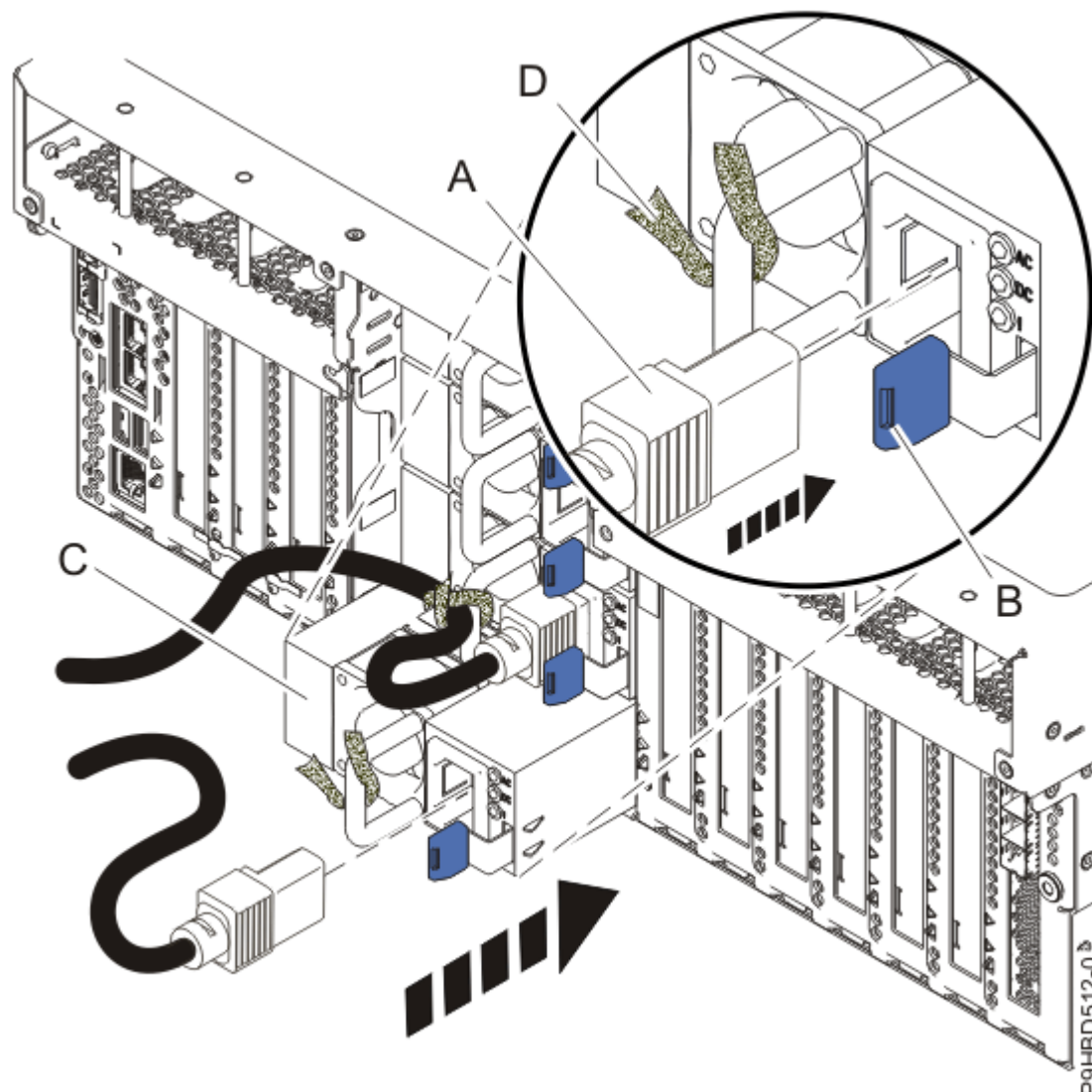
図 9. 電源装置の再取り付け
