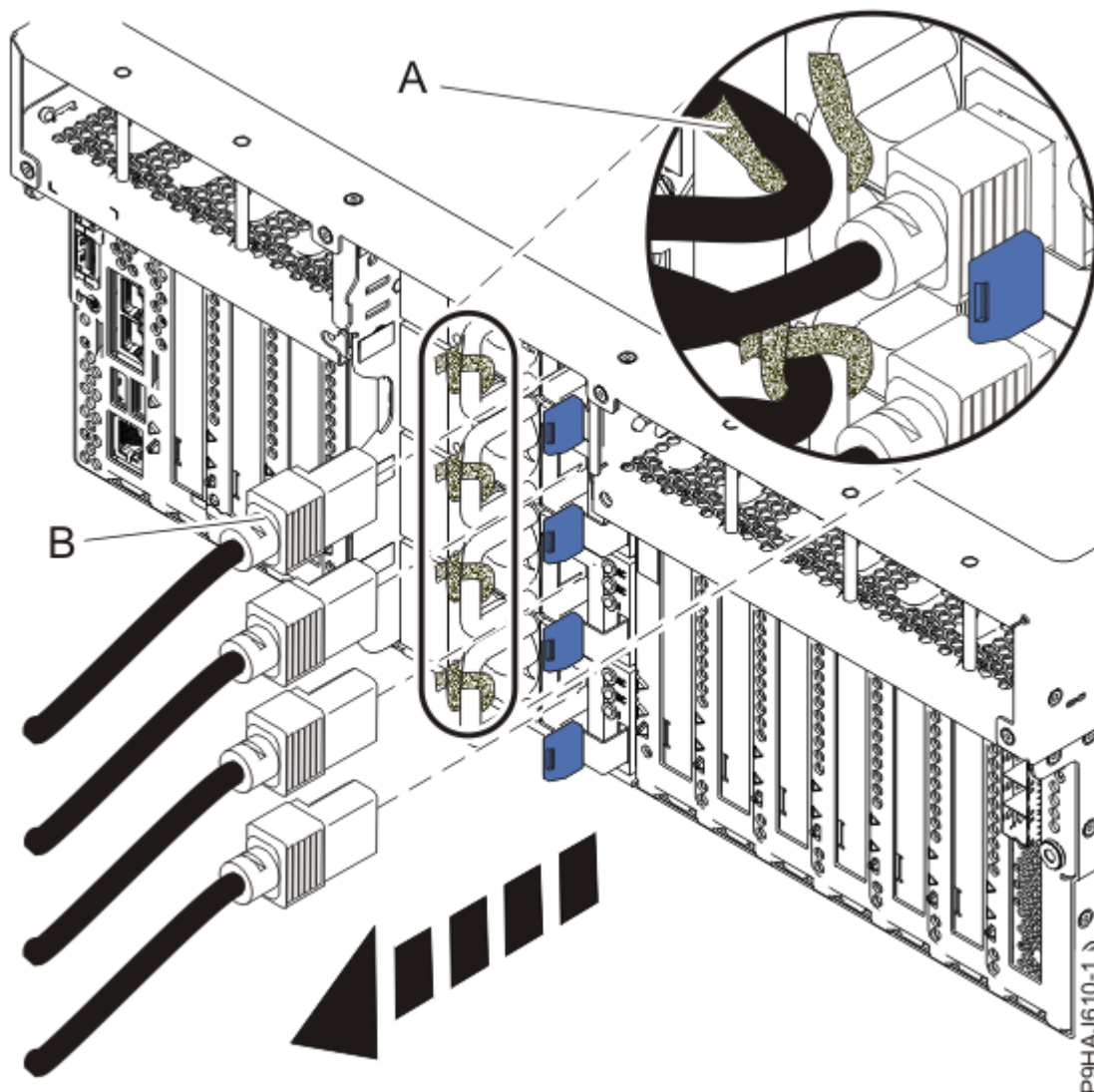
図 5. ラック・マウント型サーバーからの電源コードの取り外し
