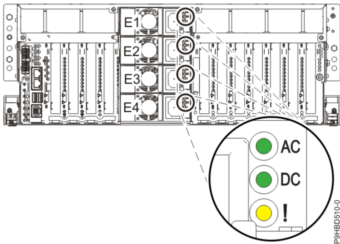
図 1. ラック・マウント型システムの電源装置と LED の位置
