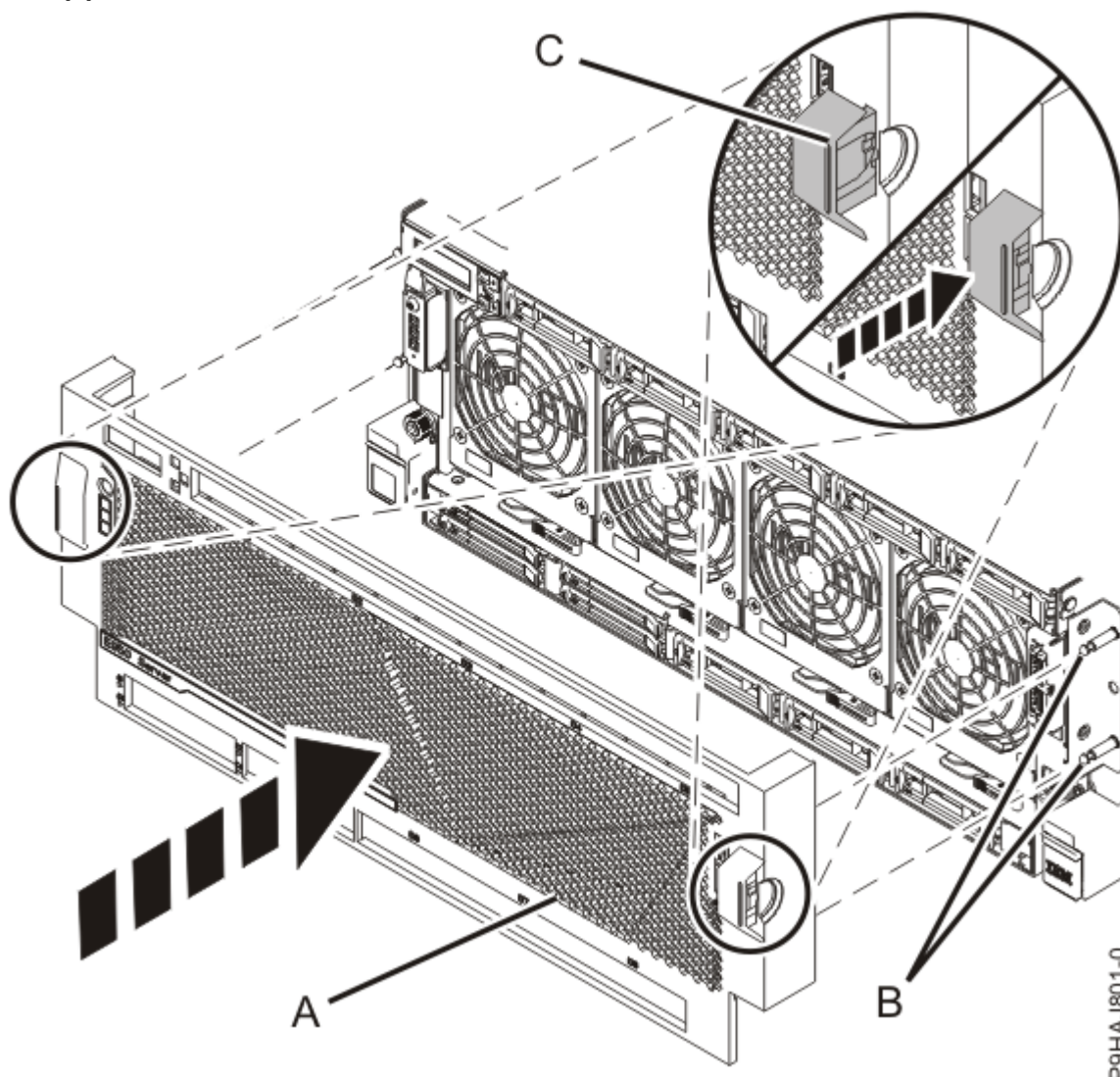
図 5. 前面カバーの取り付け
