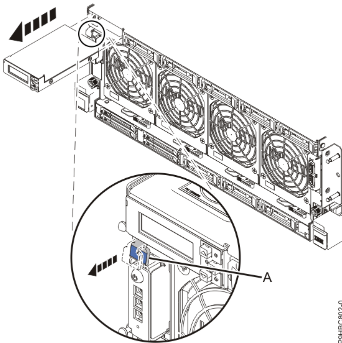
図 8. コントロール・パネル・ディスプレイの取り外し
