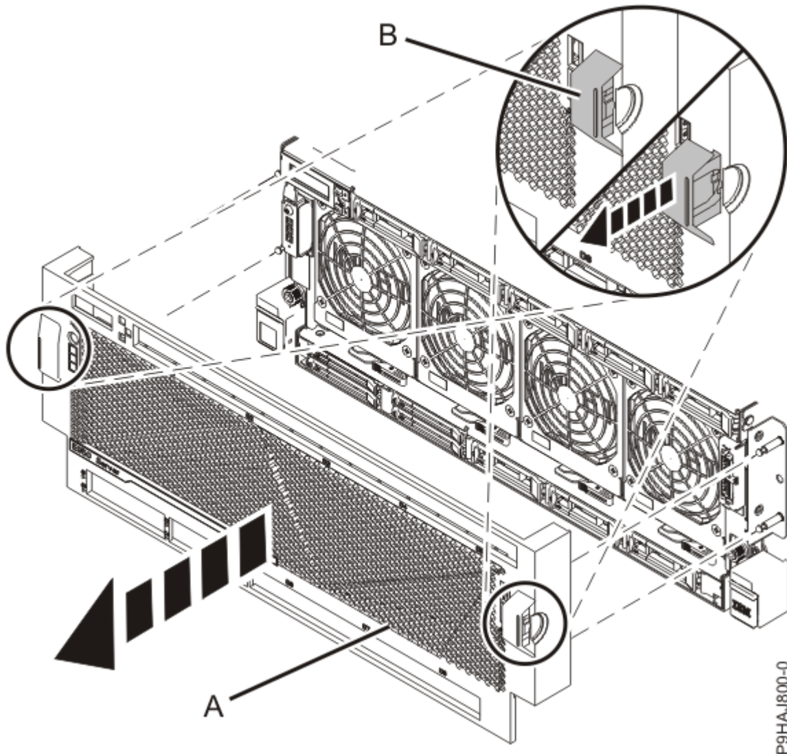
図 7. 前面カバーの取り外し
