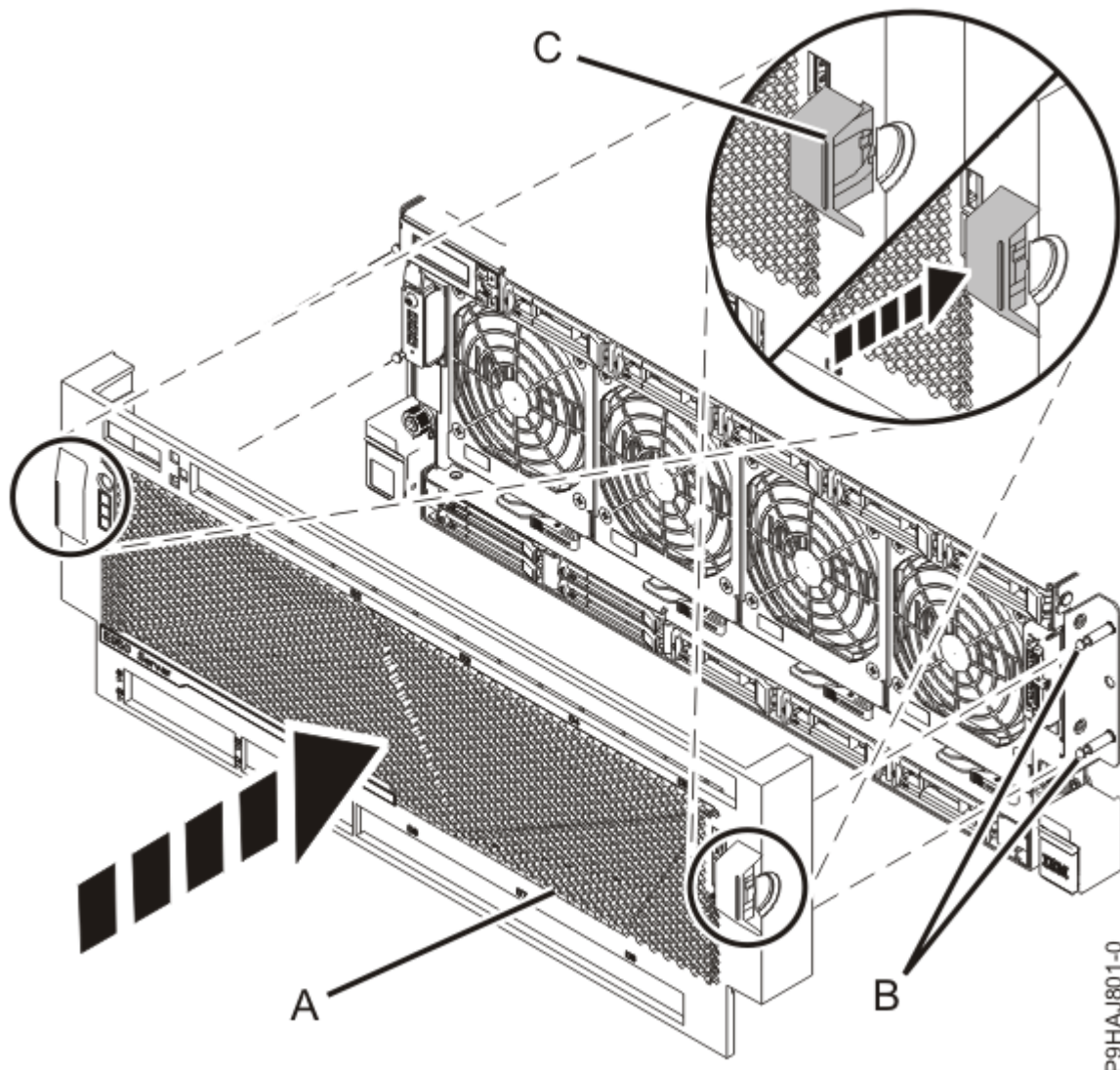
図 10. 前面カバーの取り付け
