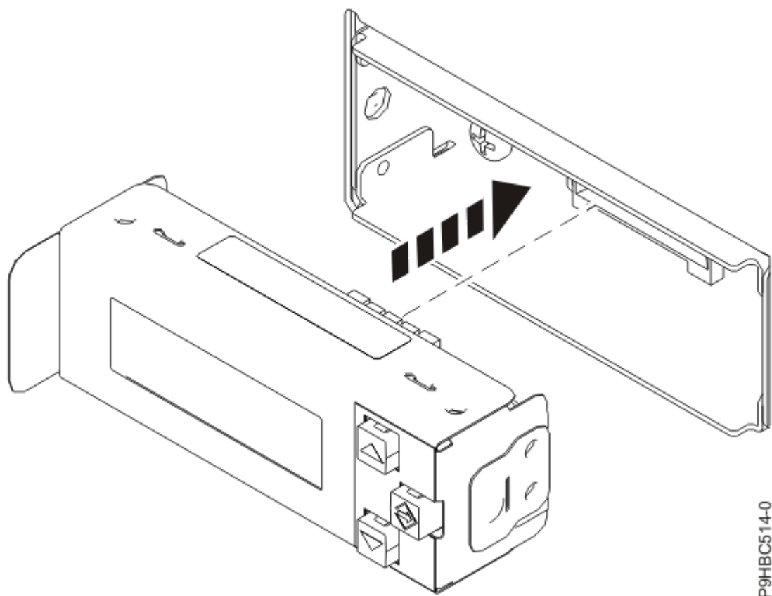
図 127. コントロール・パネル・ディスプレイの挿入
