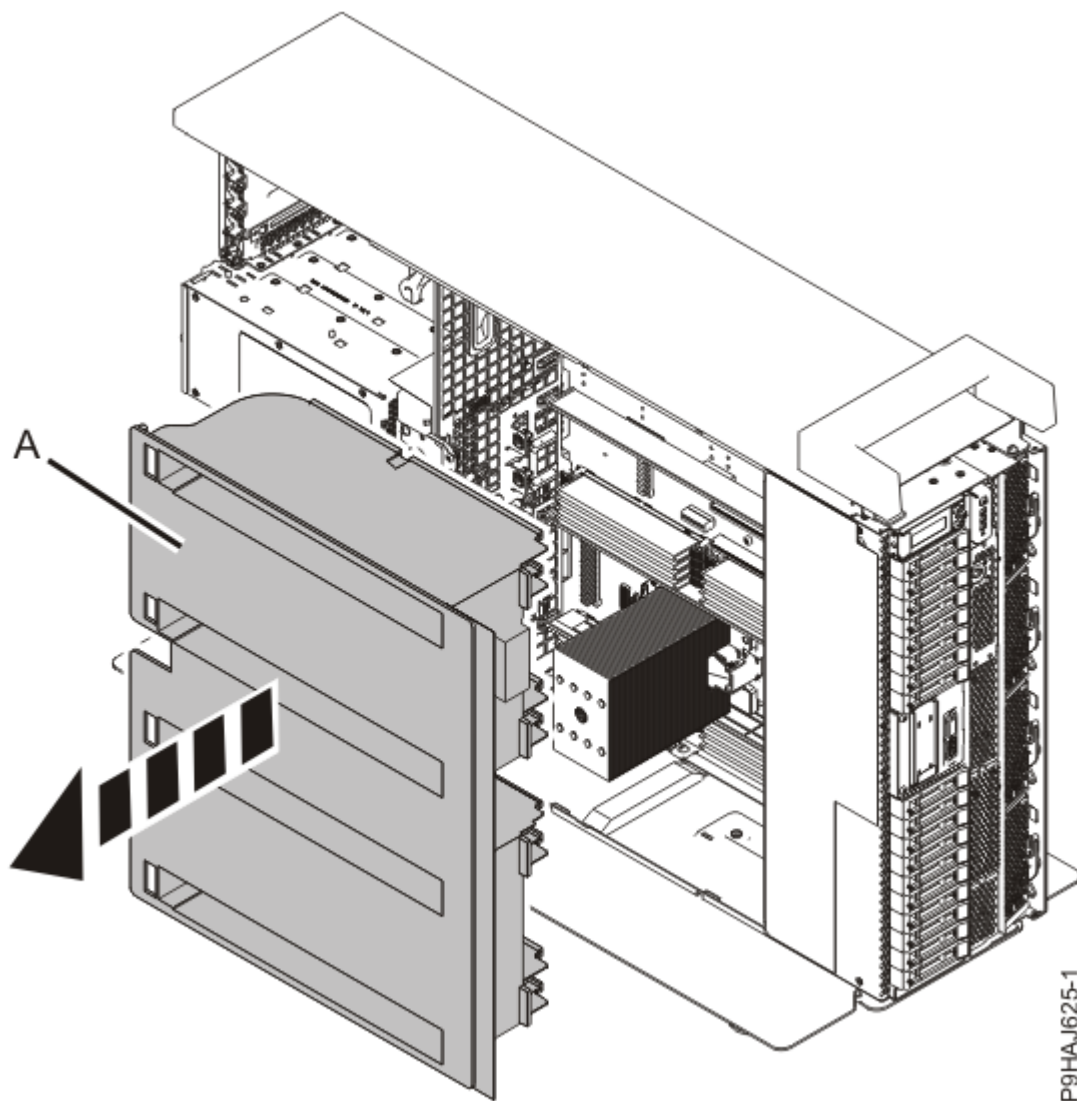
図 60. スタンドアロン・システムからのエア・バッフルの取り外し
