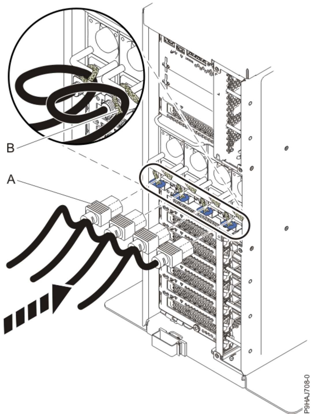
図 93. スタンドアロン・システムへの電源コードの接続
