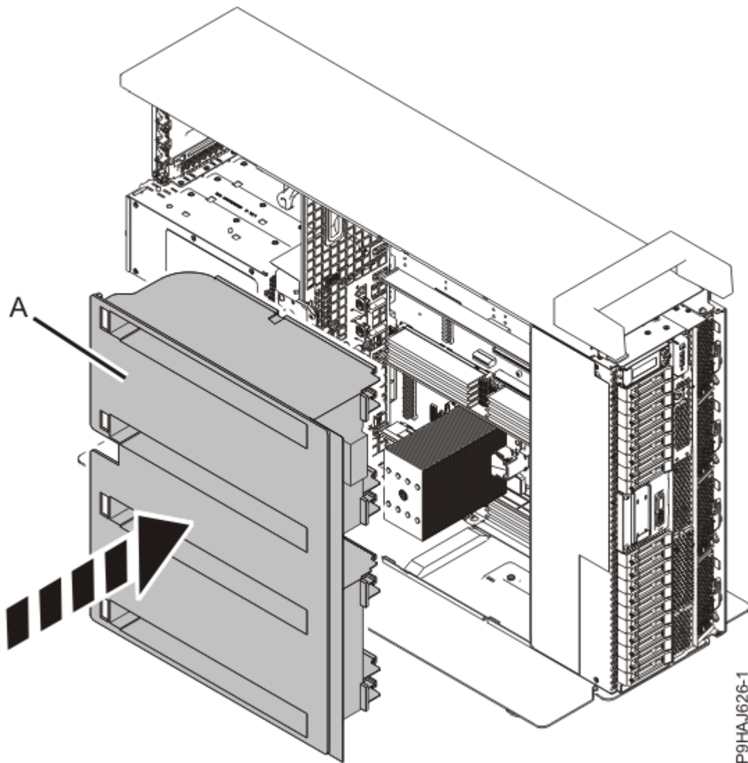
図 129. スタンドアロン・システムのエア・バッフルの再取り付け
