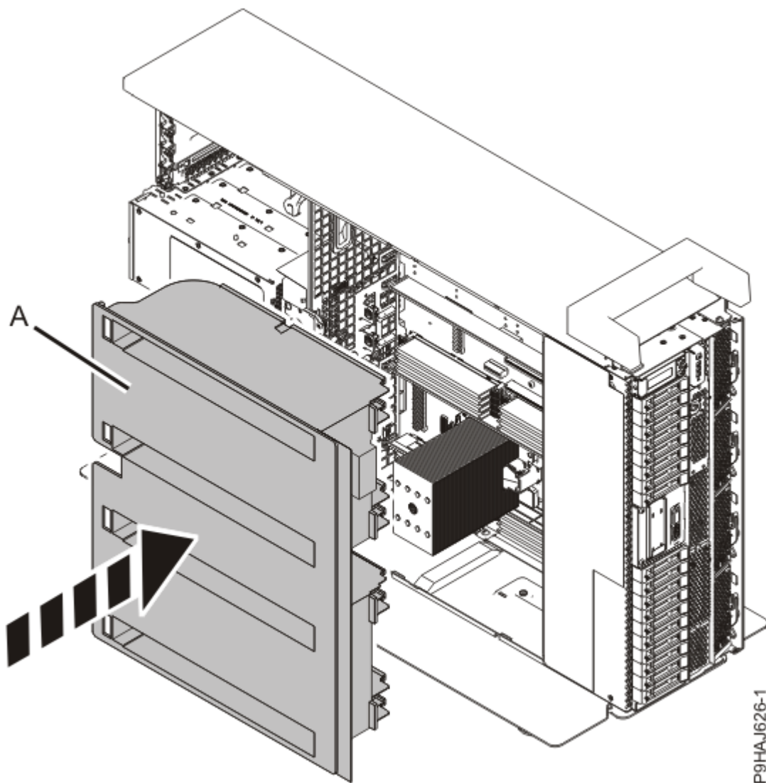
図 84. スタンドアロン・システムのエア・バッフルの再取り付け
