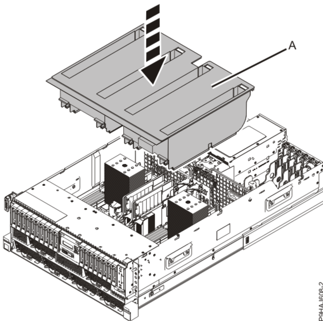
図 128. ラック・マウント型システムのエア・バッフルの再取り付け
