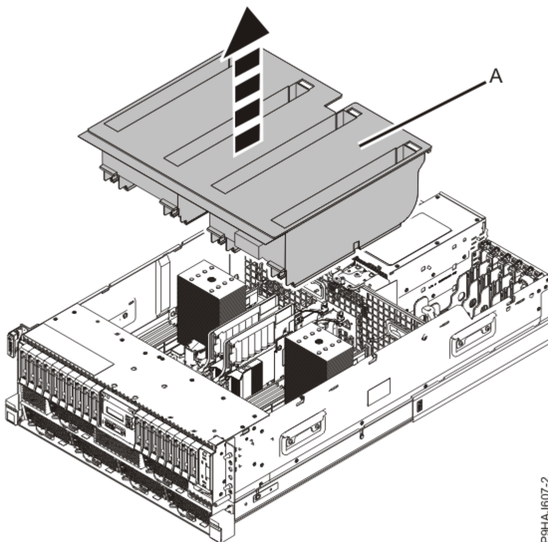
図 105. ラック・マウント型システムからのエア・バッフルの取り外し
