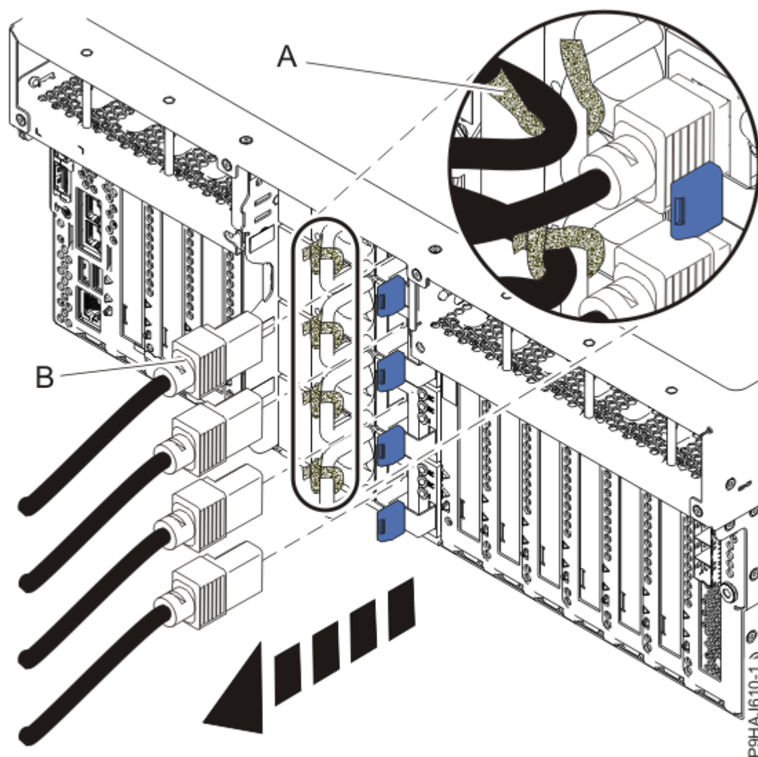
図 95. ラック・マウント型サーバーからの電源コードの取り外し
