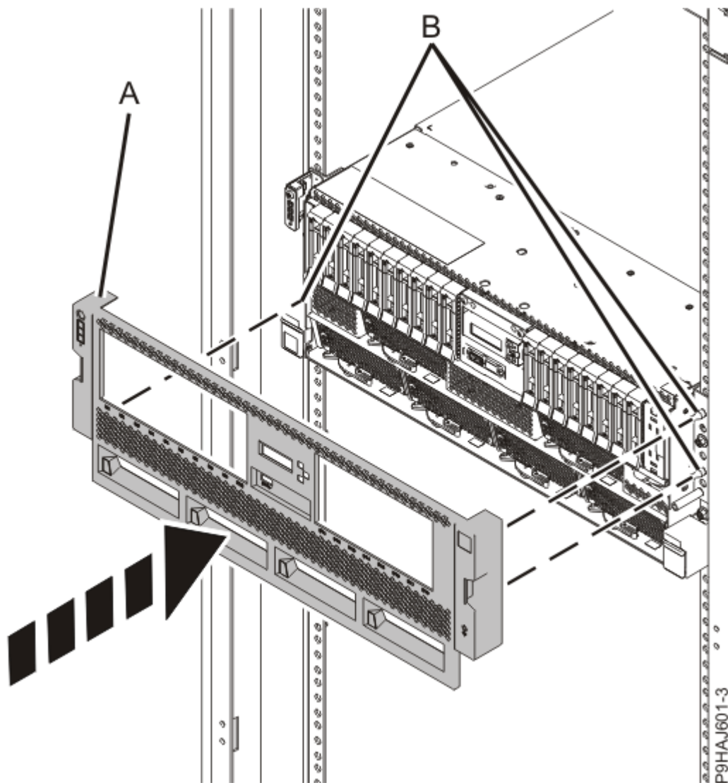
図 45. 前面カバーの取り付け
