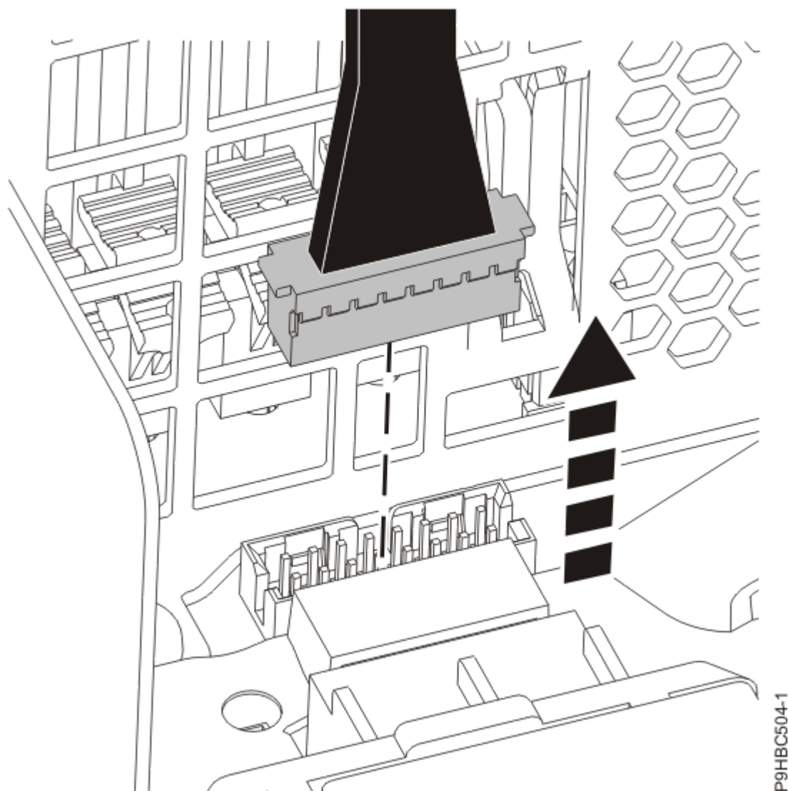
図 61. ラック・マウント型システムのシステム・バックプレーンからのコントロール・パネル・ケーブルの切り離し
