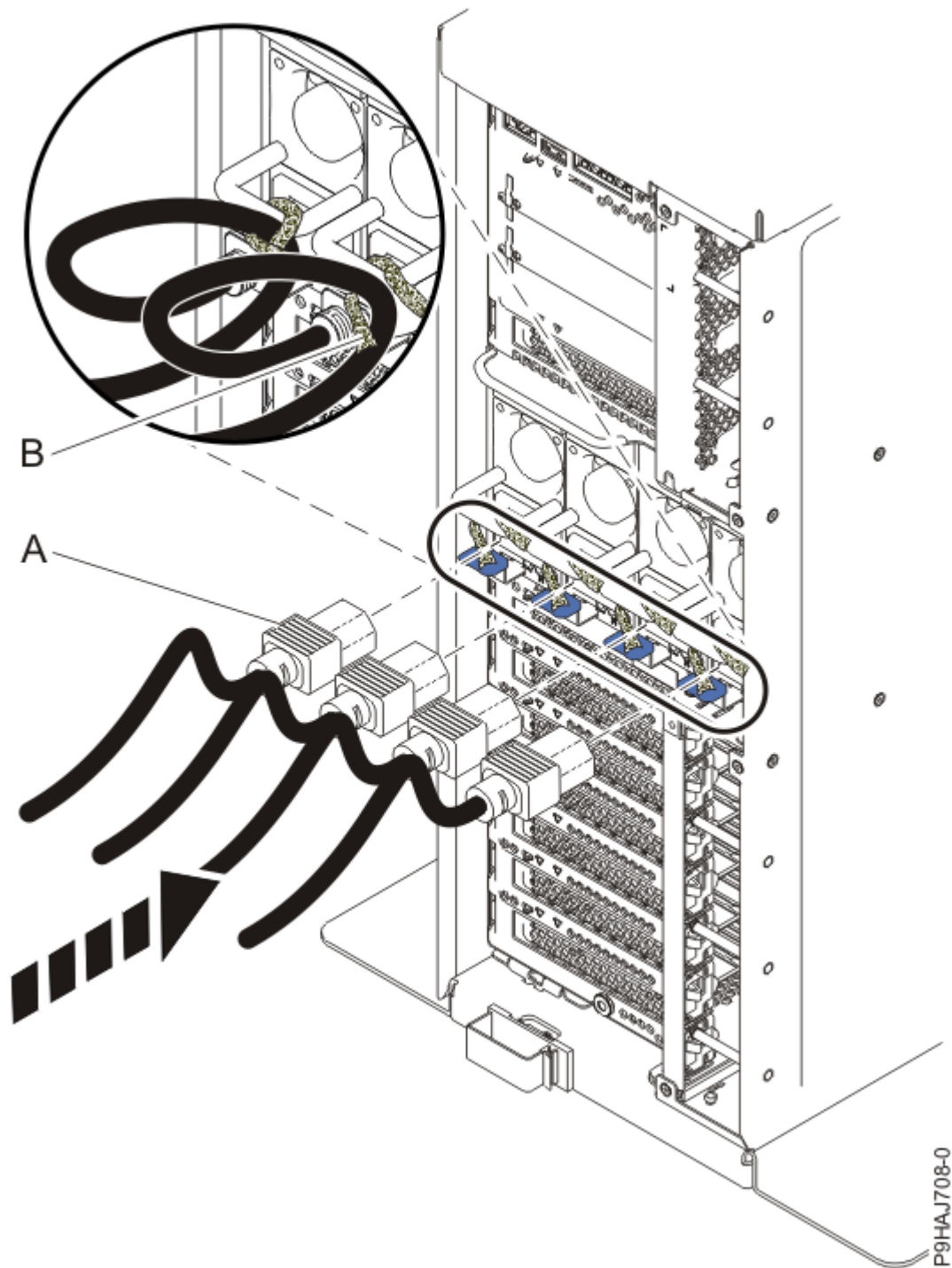
図 34. スタンドアロン・システムへの電源コードの接続 8. 次の図に示すように、電源 LED (A) が明滅していることを確認します。
