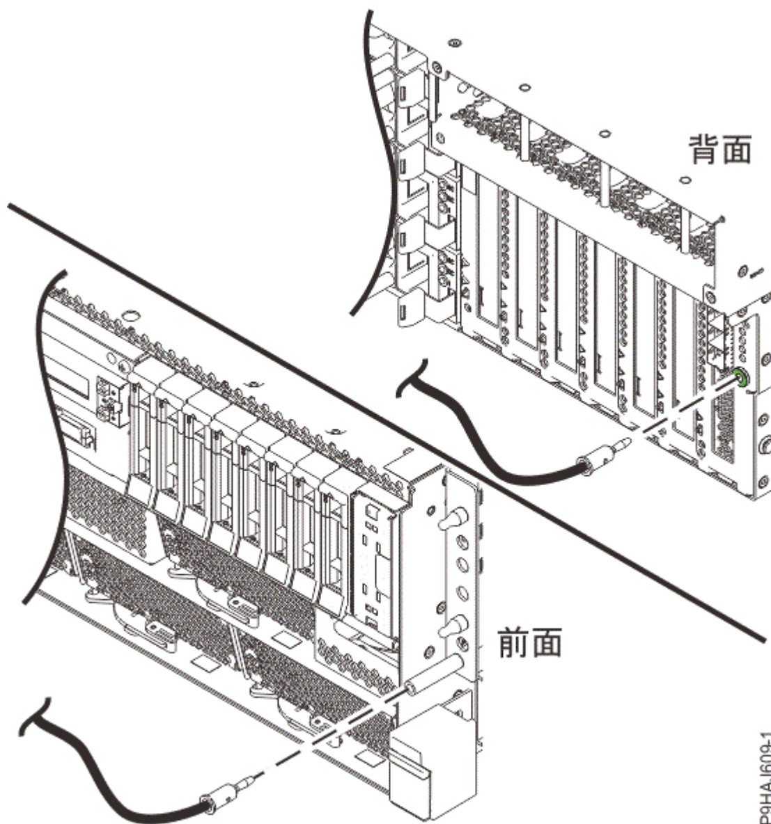
図 56. ESD プラグの位置
