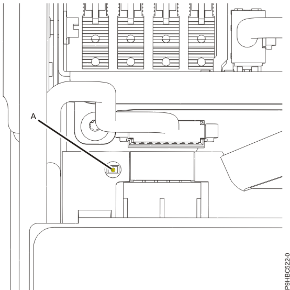
図 14. ラック・マウント型システムのコントロール・パネル LED の位置
