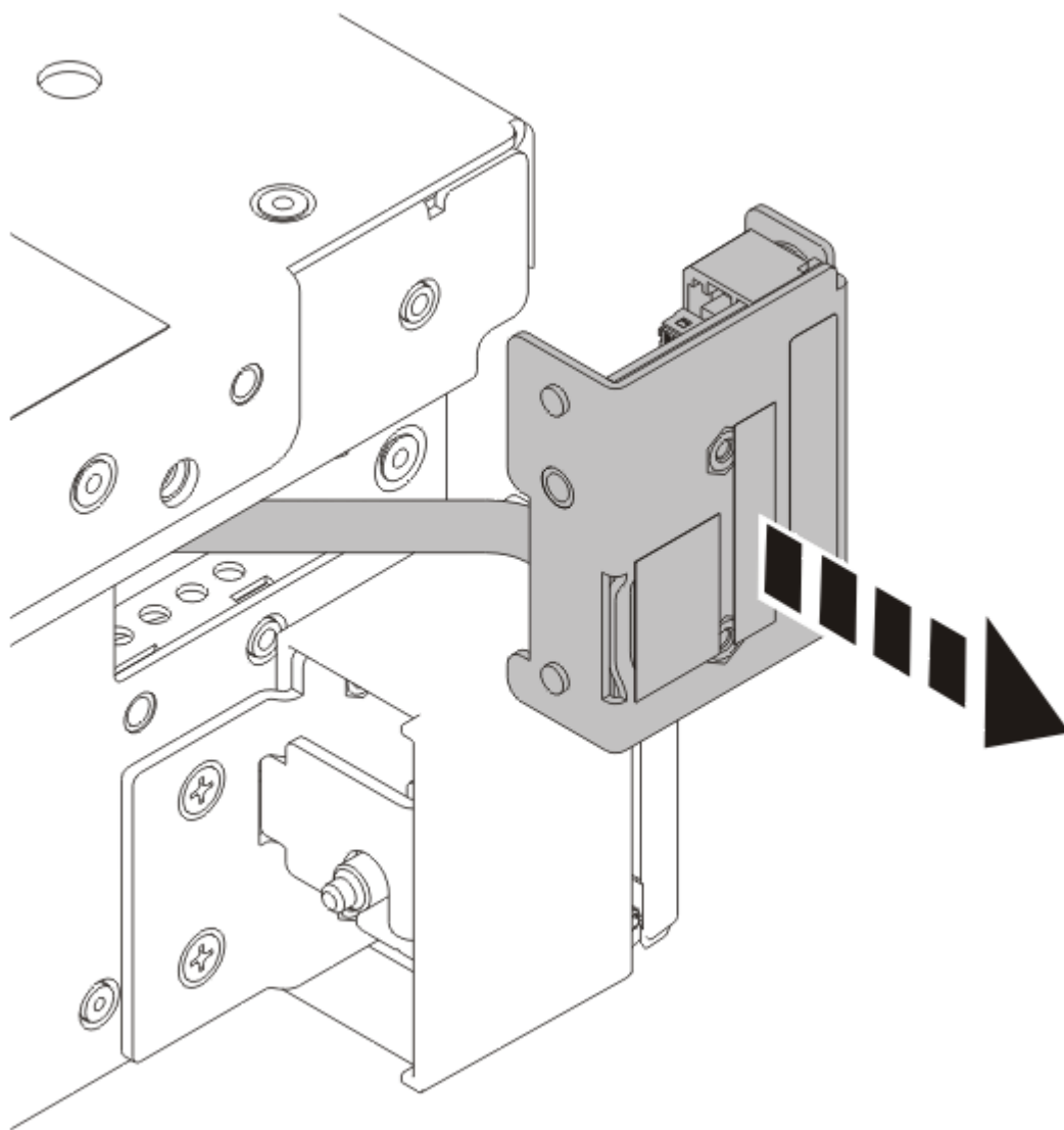
図 67. ラック・マウント型システムからのコントロール・パネルおよびケーブルの取り外し
