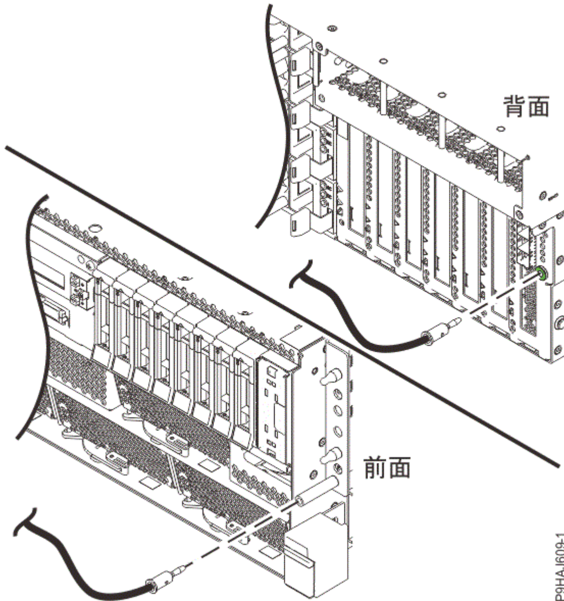
図 10. ESD プラグの位置
