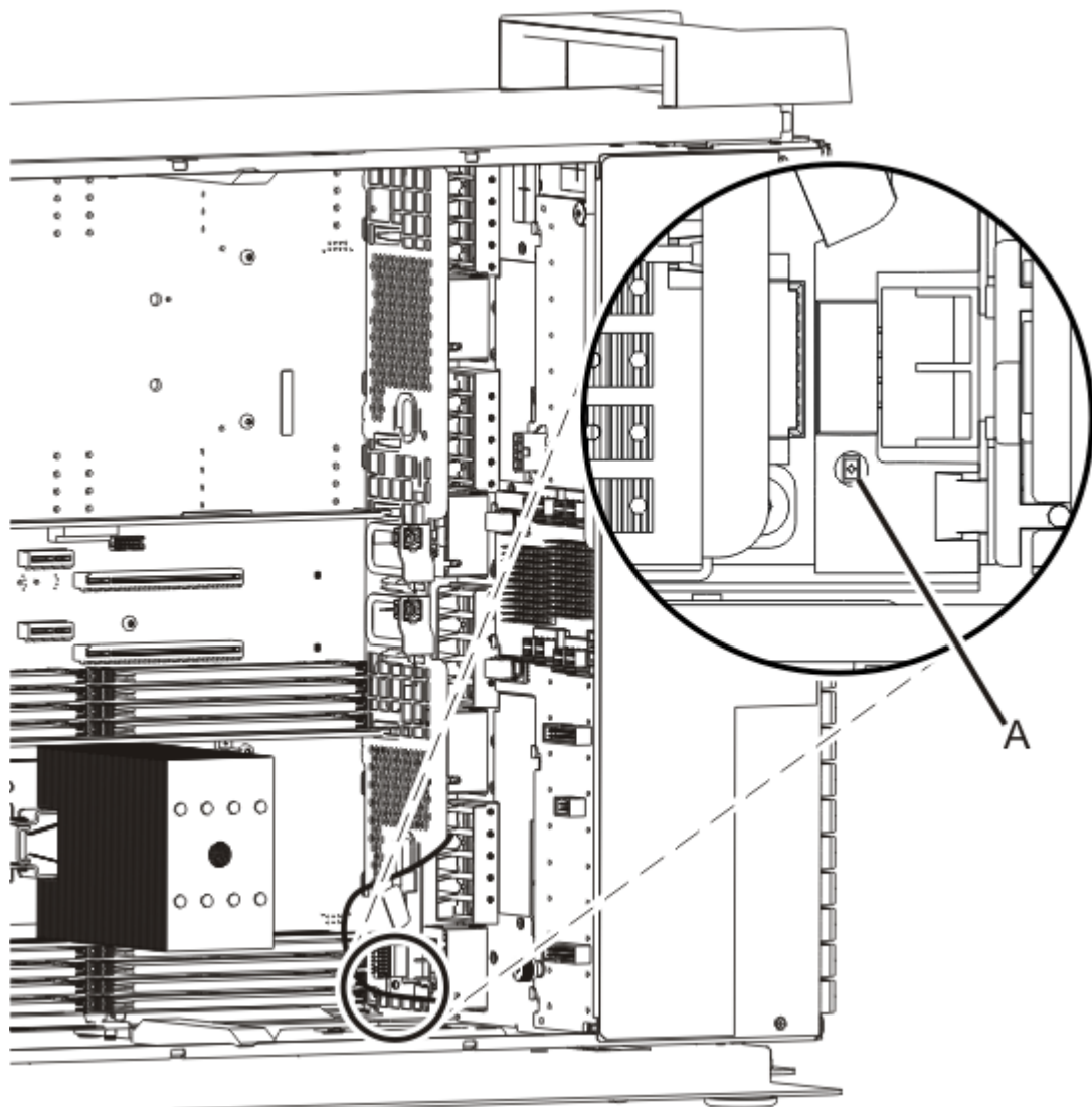
図 15. スタンドアロン・システムのコントロール・パネル LED の位置
