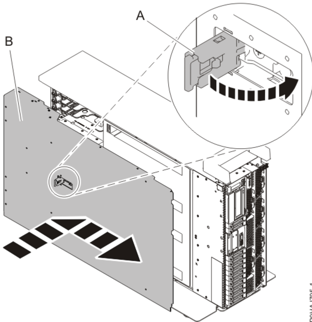
図 27. 保守アクセス・カバーの取り付け
