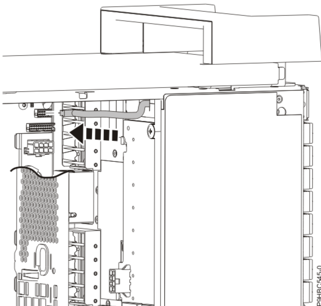
図 124. スタンドアロン・システムのシステム・バックプレーンへのコントロール・パネル・ディスプレイ・ケーブルの接続
