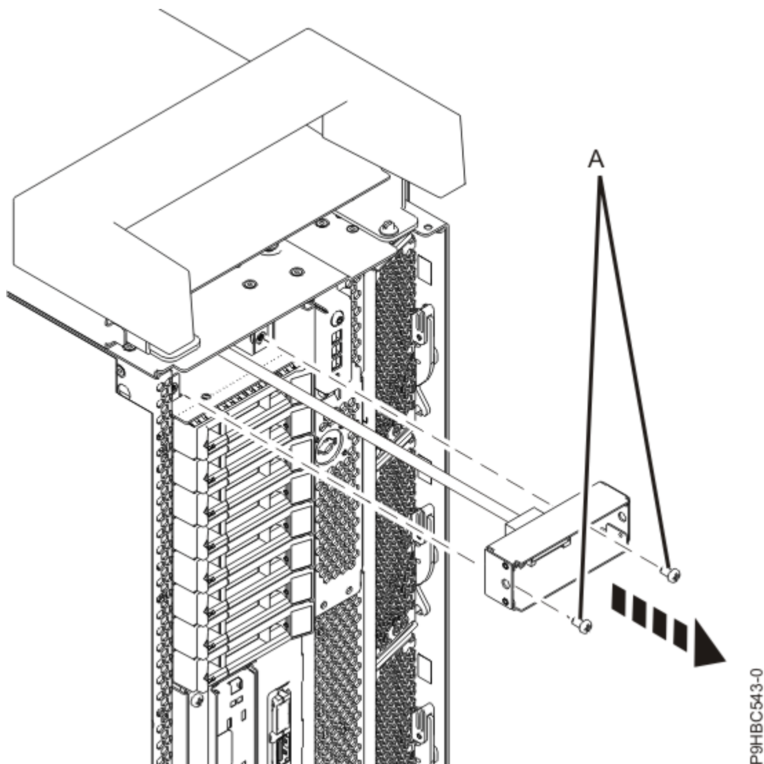
図 112. ラック・マウント型システムのブラケットからのコントロール・パネル・ディスプレイ・ホルダーの取り外し
