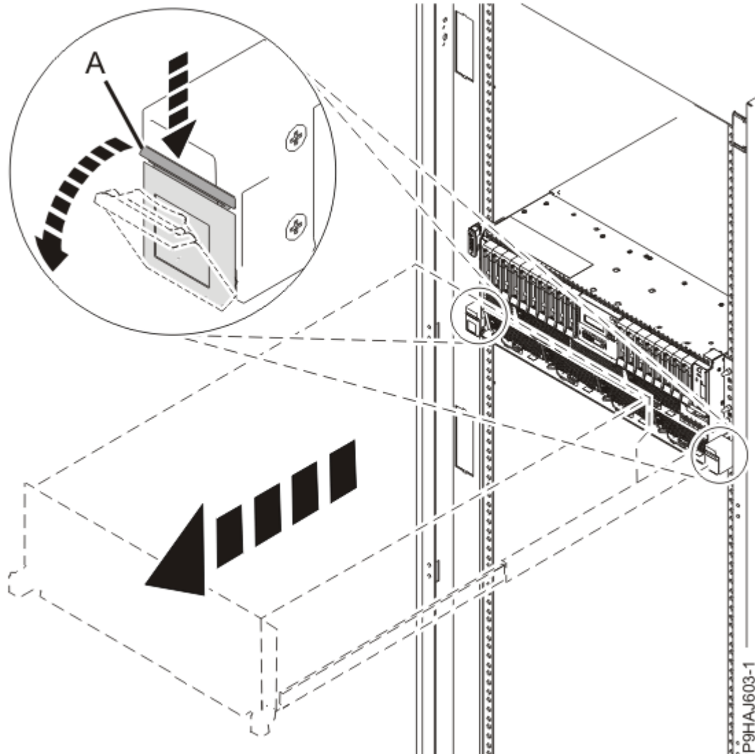
図 55. サイド・ラッチのリリース
