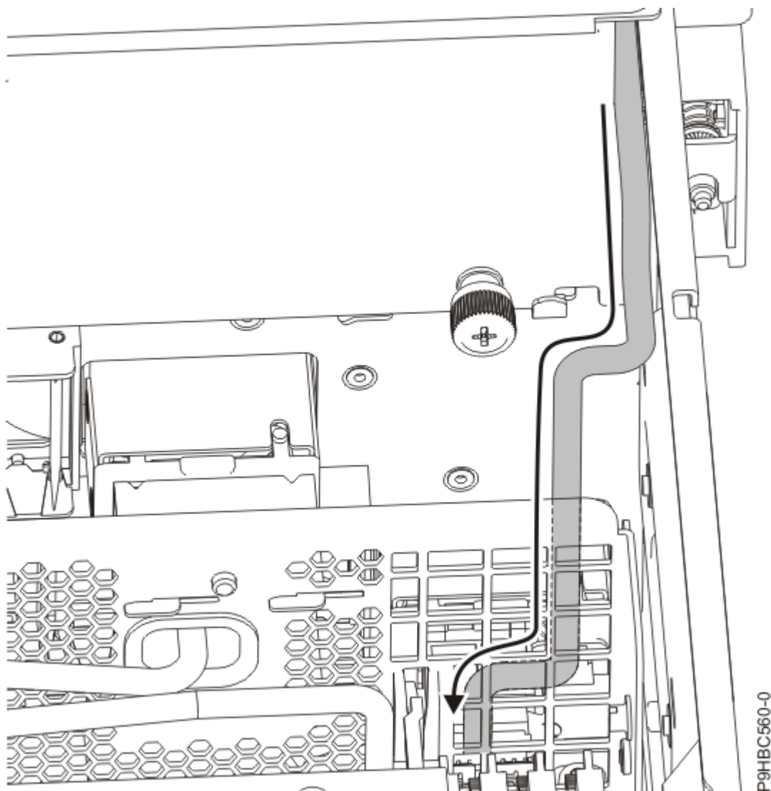
図 74. ラック・マウント型システムのコントロール・パネル・ケーブルの進路
