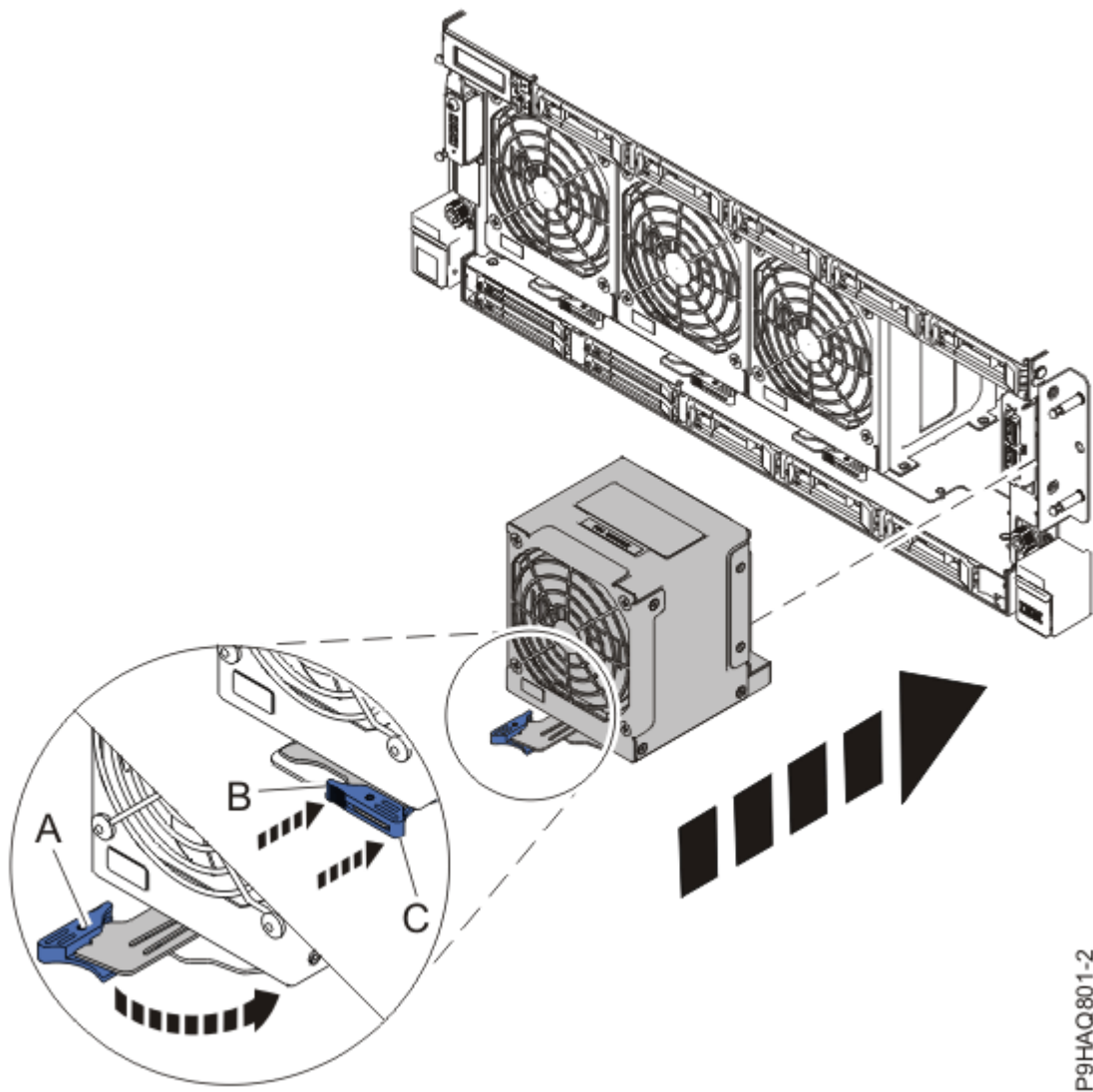
図 5. システムでのファンの再取り付け
