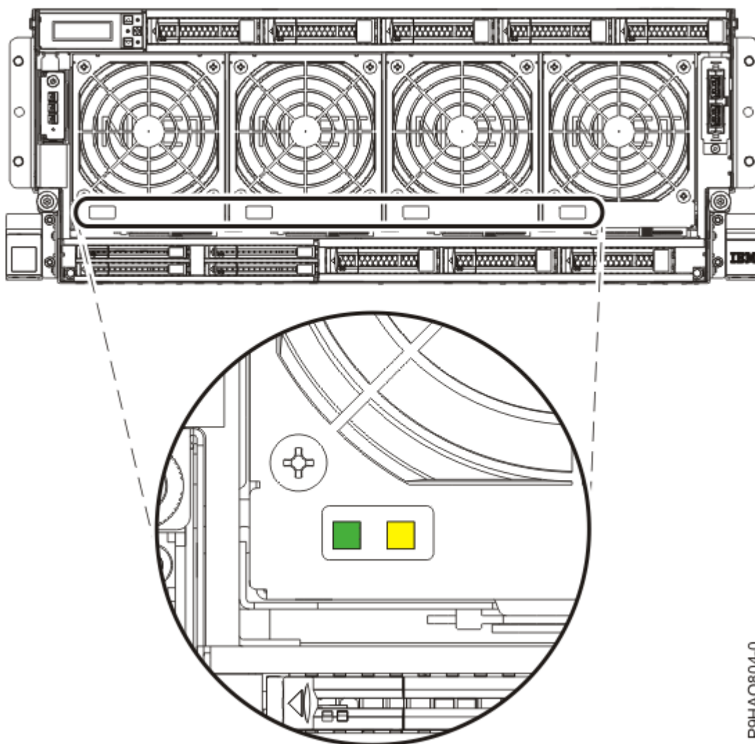
図 2. システムのファン LED
