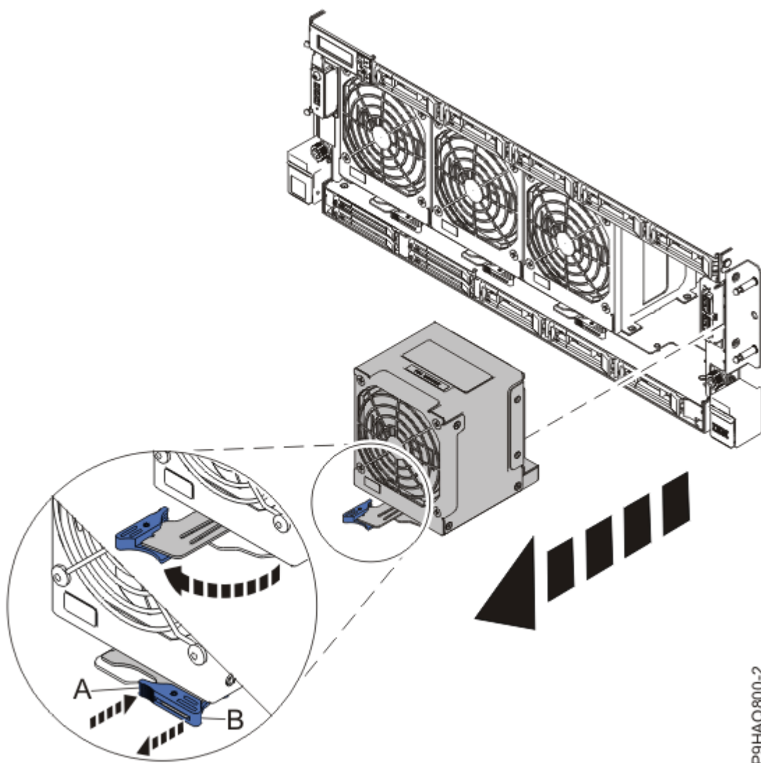
図 4. システムからのファンの取り外し
