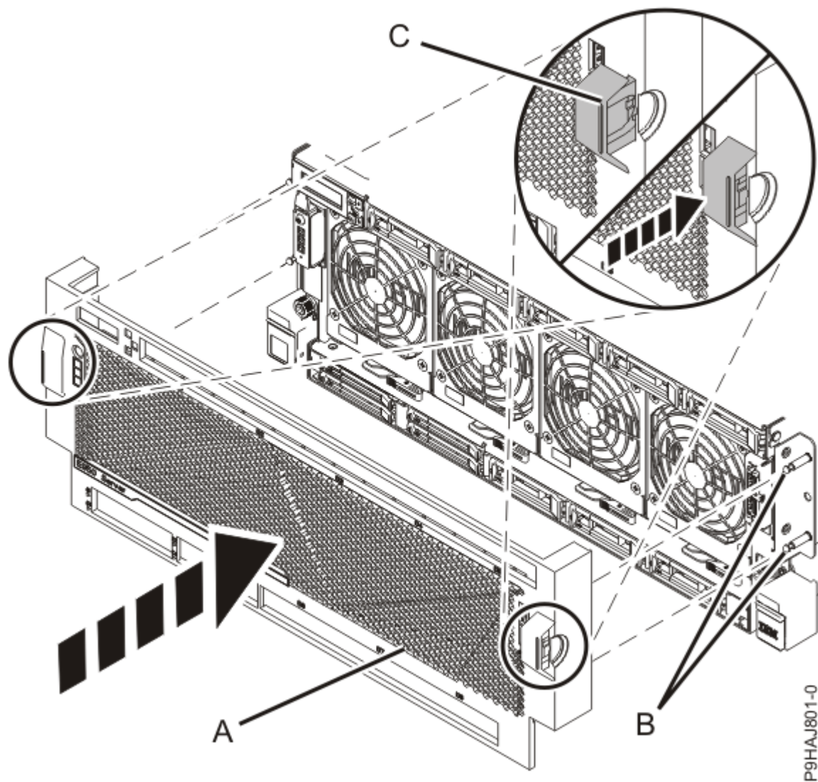
図 6. 前面カバーの取り付け 7. 該当する場合は、ラックの前面ドアを閉じます。
