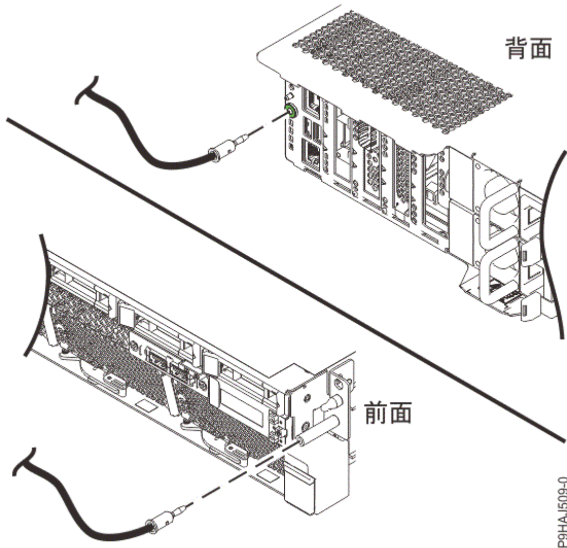
図 4. ESD プラグの位置
