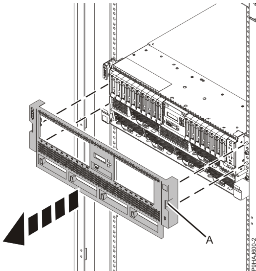
図 1. 前面カバーの取り外し
