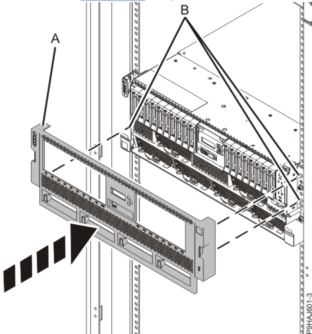
図 12. 前面カバーの取り付け
