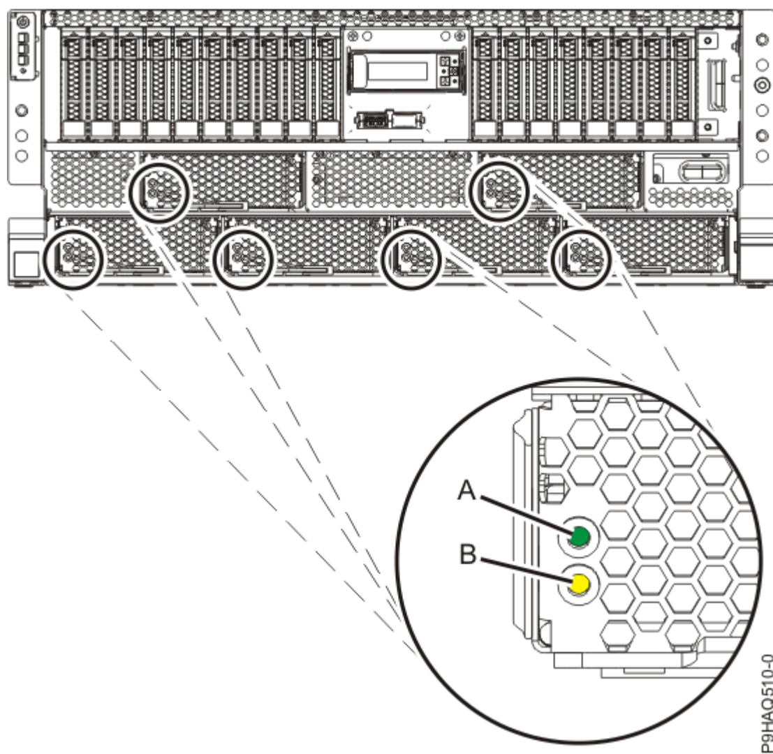
図 5. ラック・マウント型システムのファン LED
