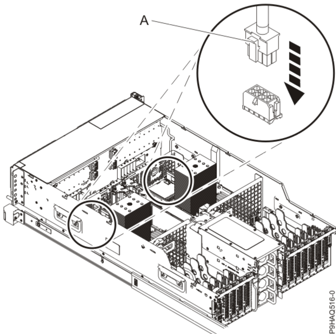
図 32. システム・バックプレーンへのファン・ケーブルの再取り付け
