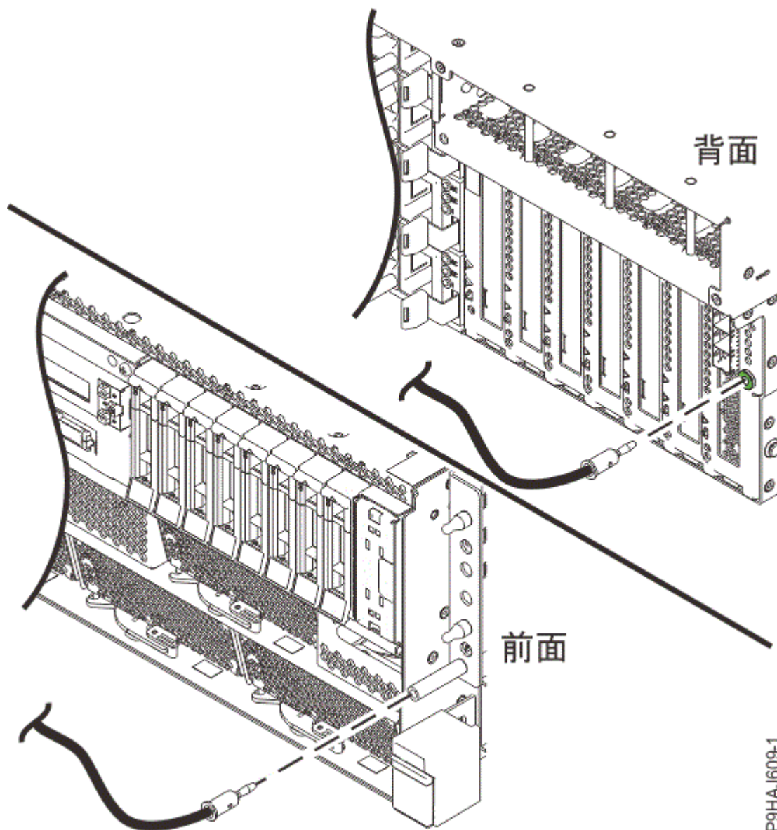
図 9. ESD プラグの位置
