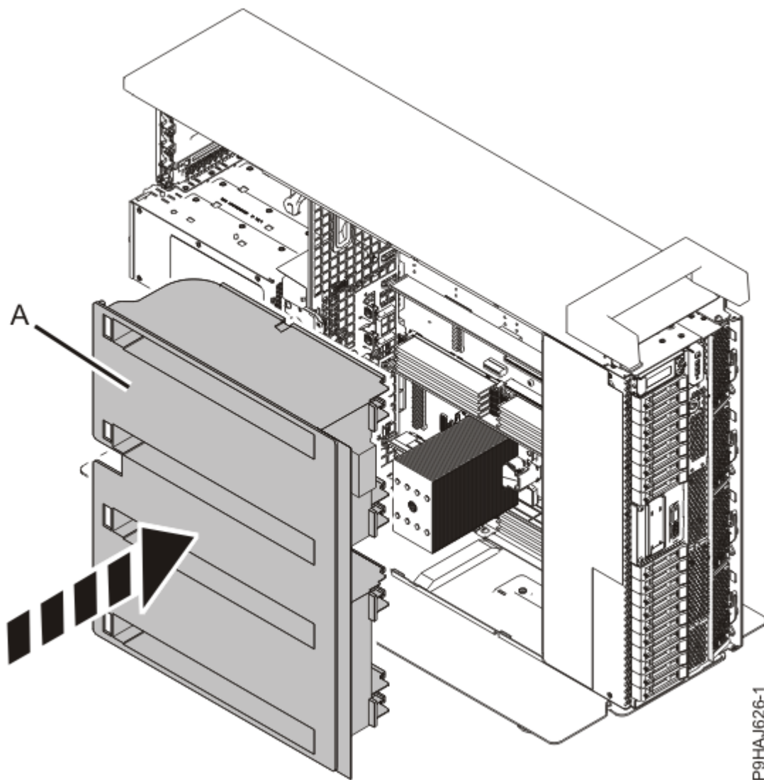
図 34. スタンドアロン・システムのエア・バッフルの再取り付け
