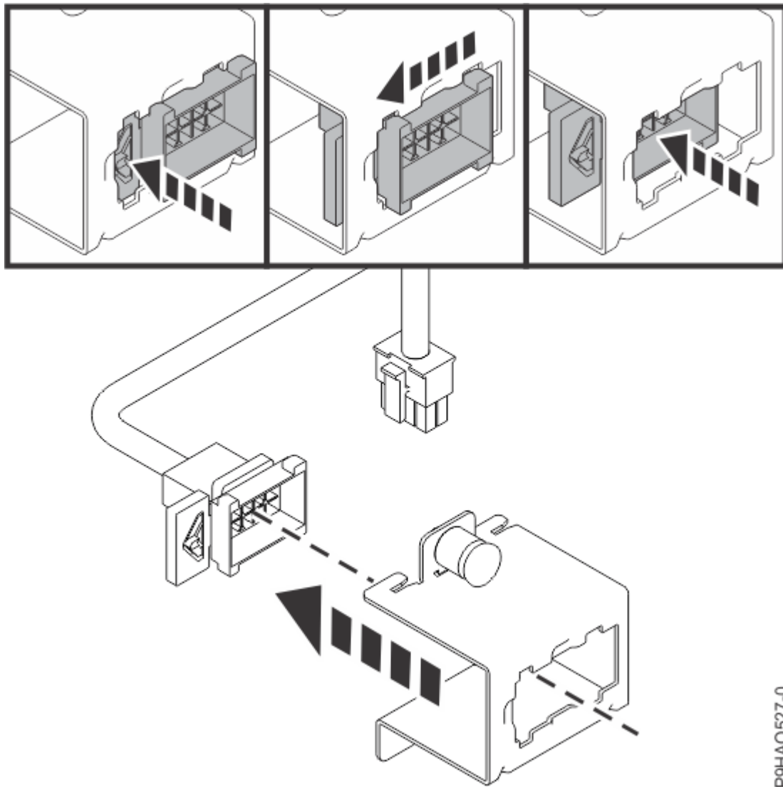
図 28. ファン・ケーブル・ブラケットからのファン・ケーブルの取り外し
