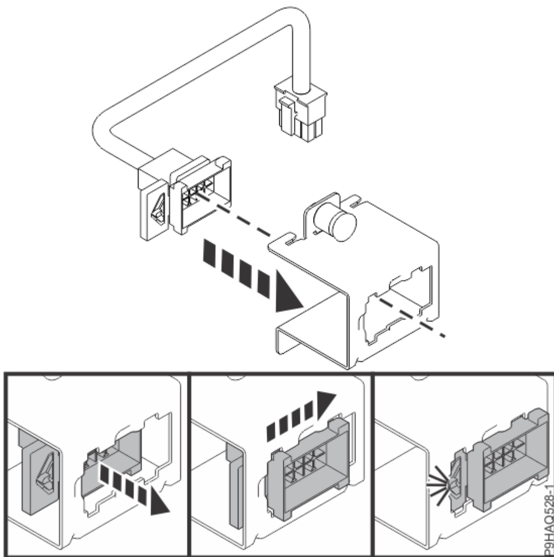
図 29. ファン・ケーブル・ブラケットへのファン・ケーブルの再取り付け
