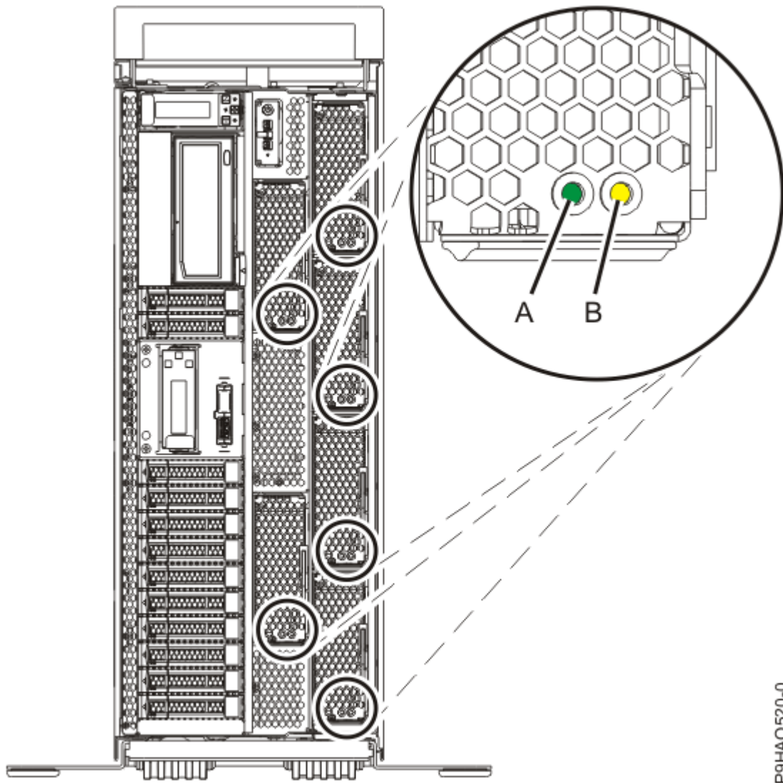
図 6. スタンドアロン・システムのファン LED
