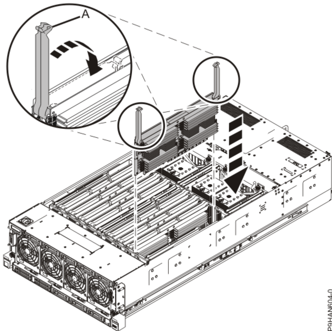
図 19. メモリー・ライザーの挿入
