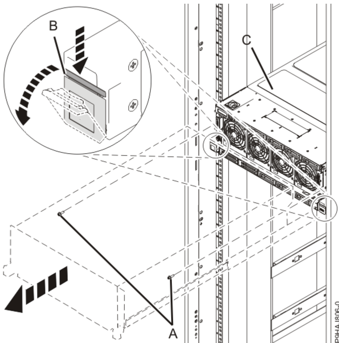
図 41. システムの保守位置への設置
