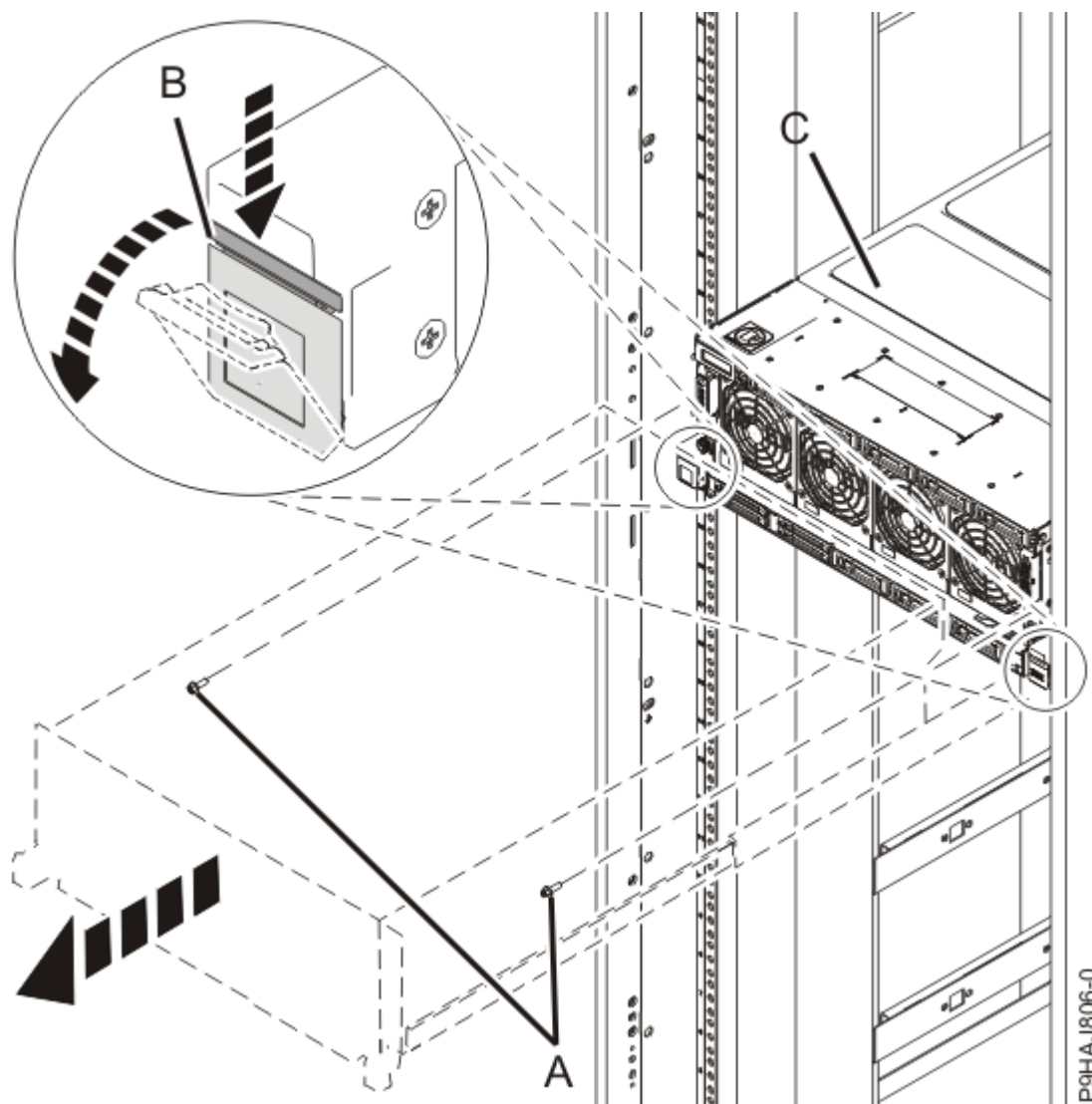
図 33. システムの保守位置への設置
