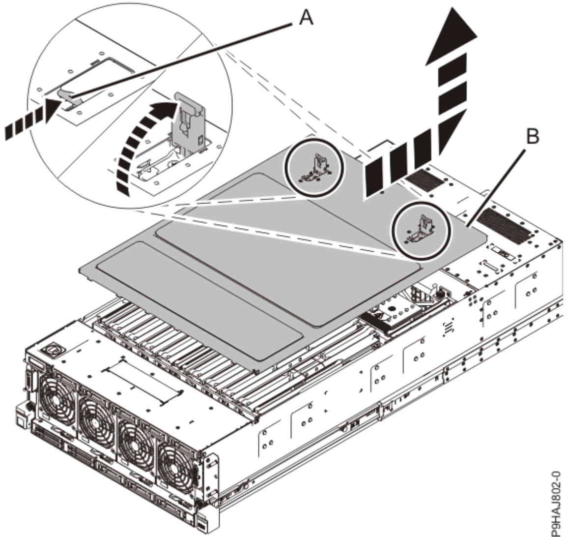
図 12. 保守アクセス・カバーの取り外し
