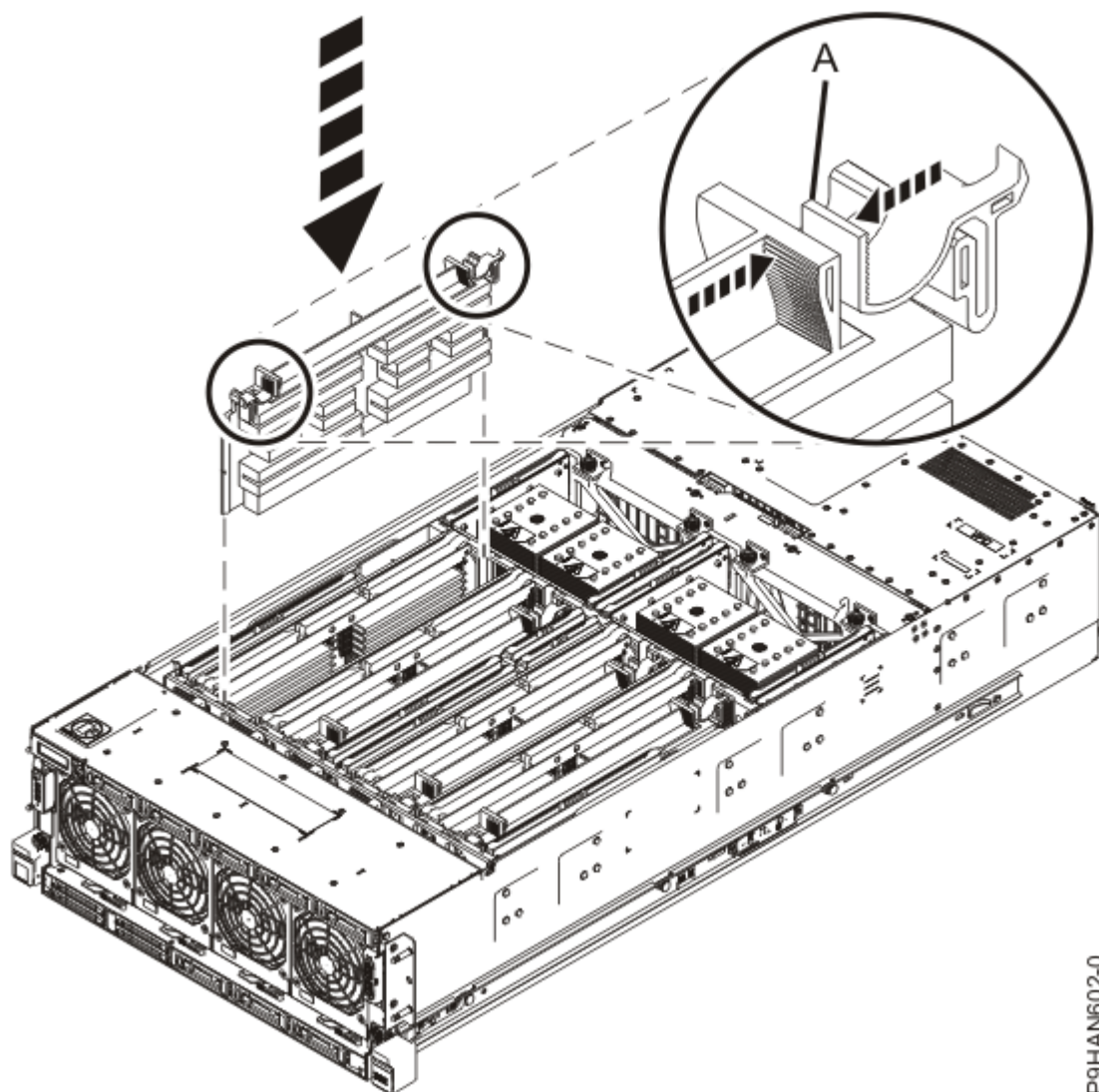
図 56. メモリー・ライザー・フィラーの挿入
