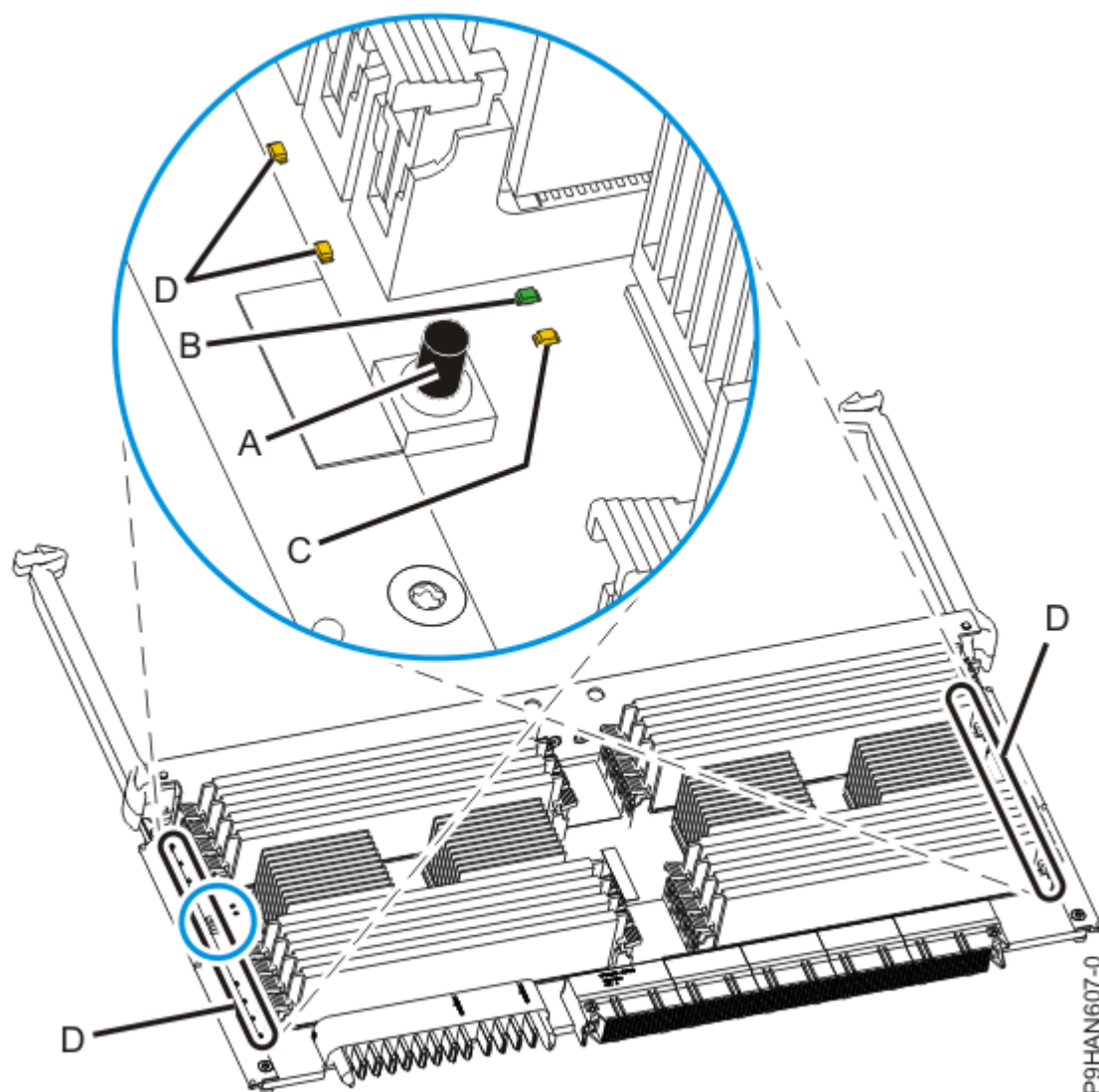
図 16. メモリー・モジュールの識別
