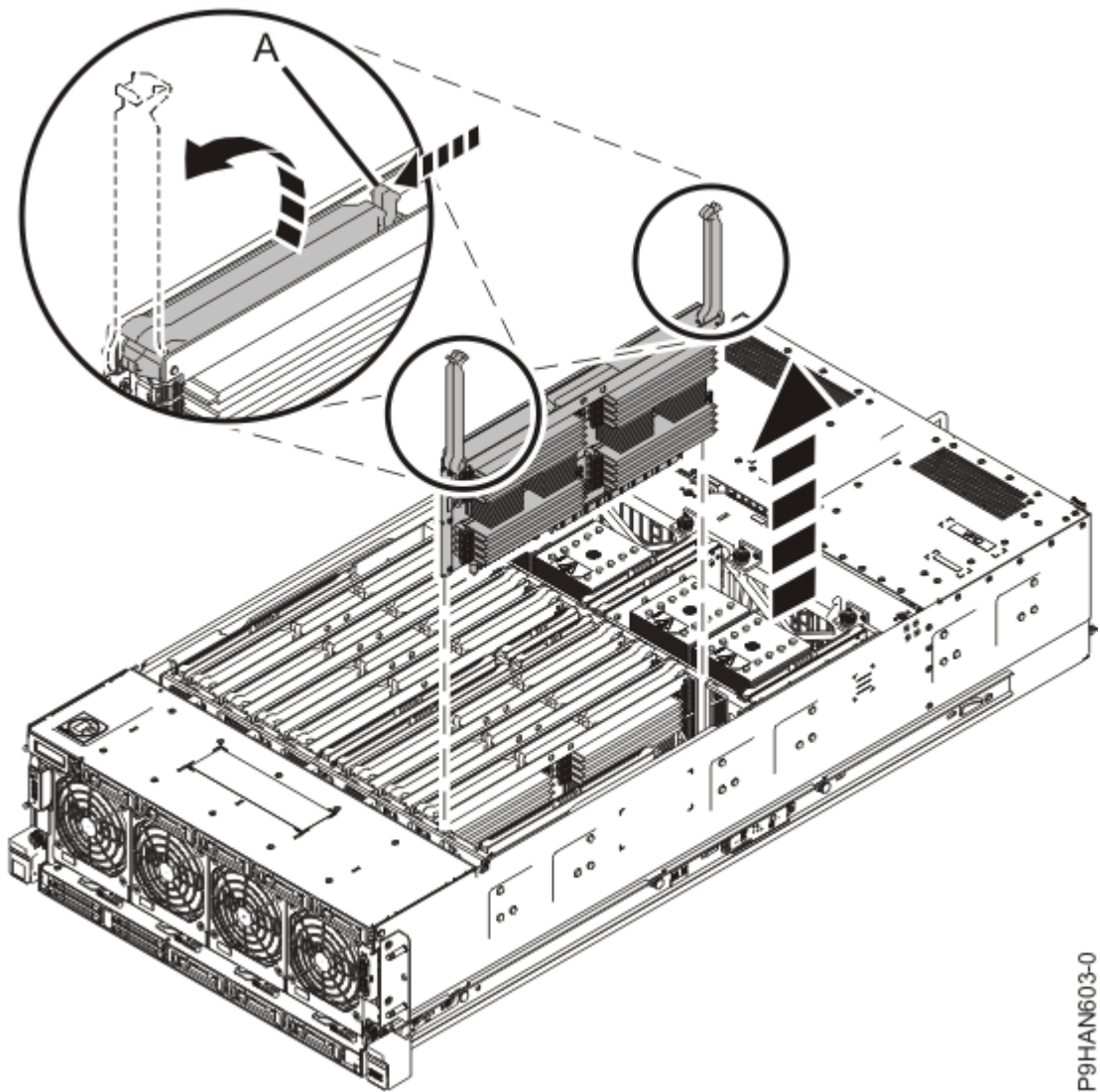
図 4. メモリー・ライザーの取り外し
