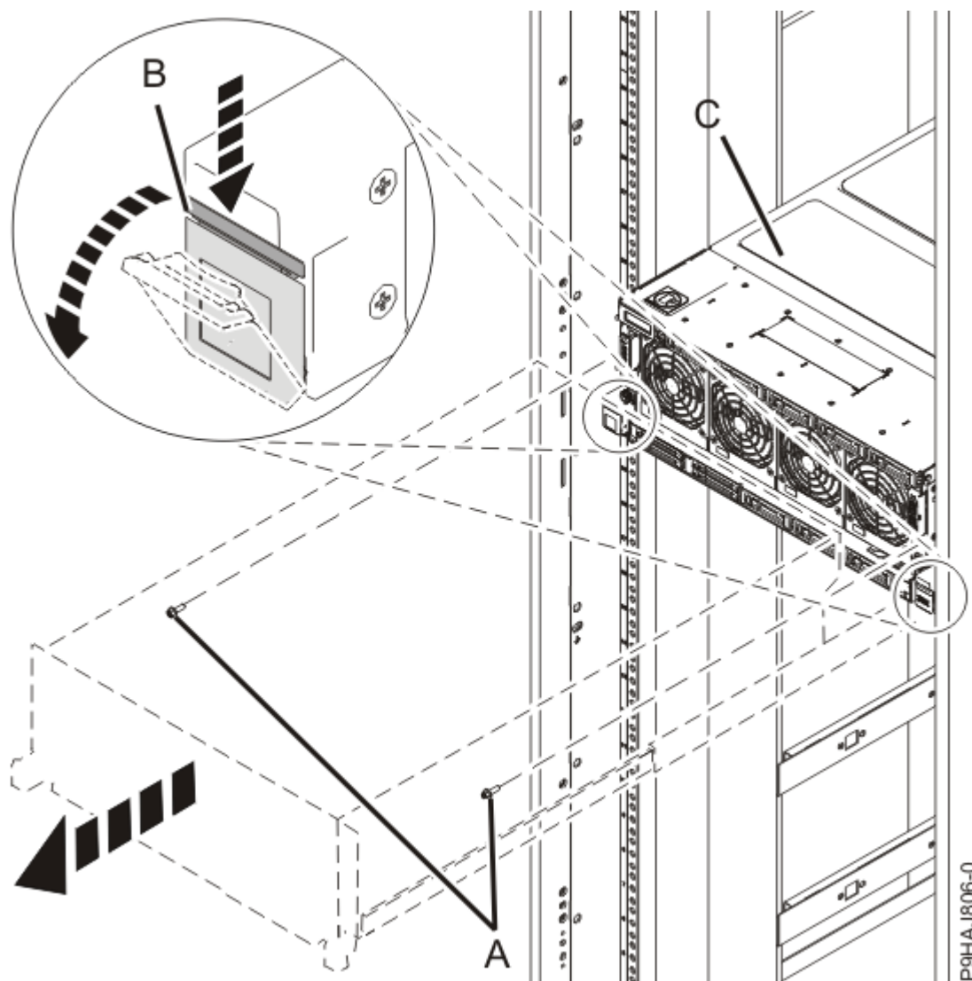
図 24. システムの保守位置への設置
