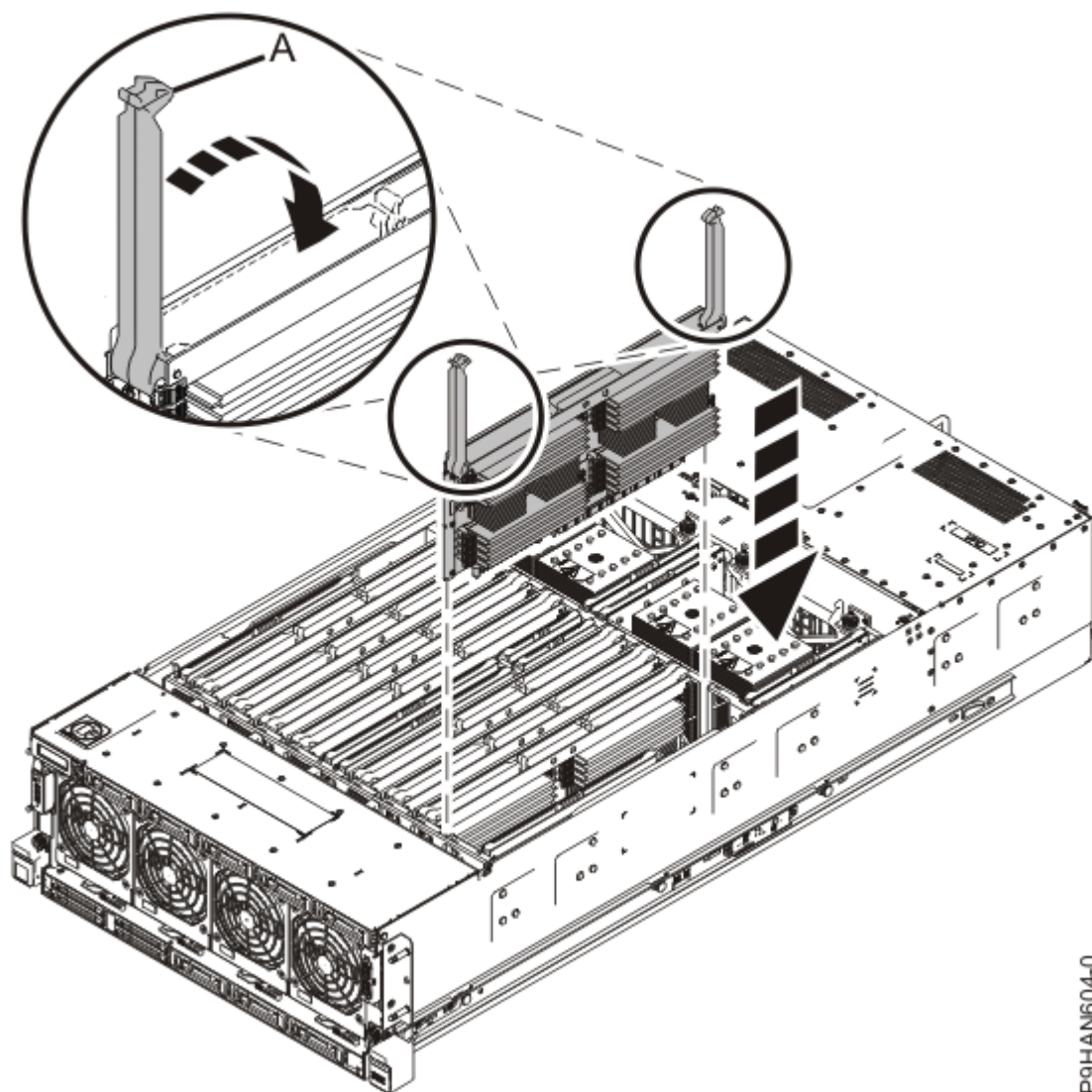
図 28. メモリー・ライザーの挿入
