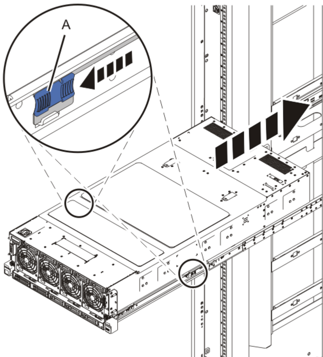
図 50. システムの操作位置への設置
