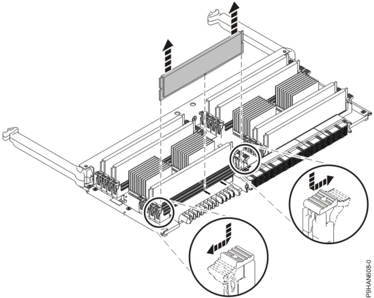
図 46. メモリー・モジュールの取り外し
