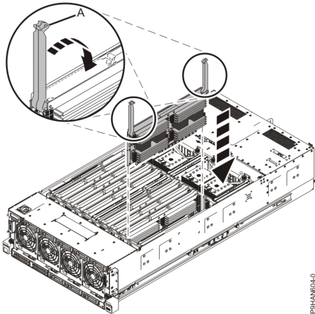
図 36. メモリー・ライザーの挿入
