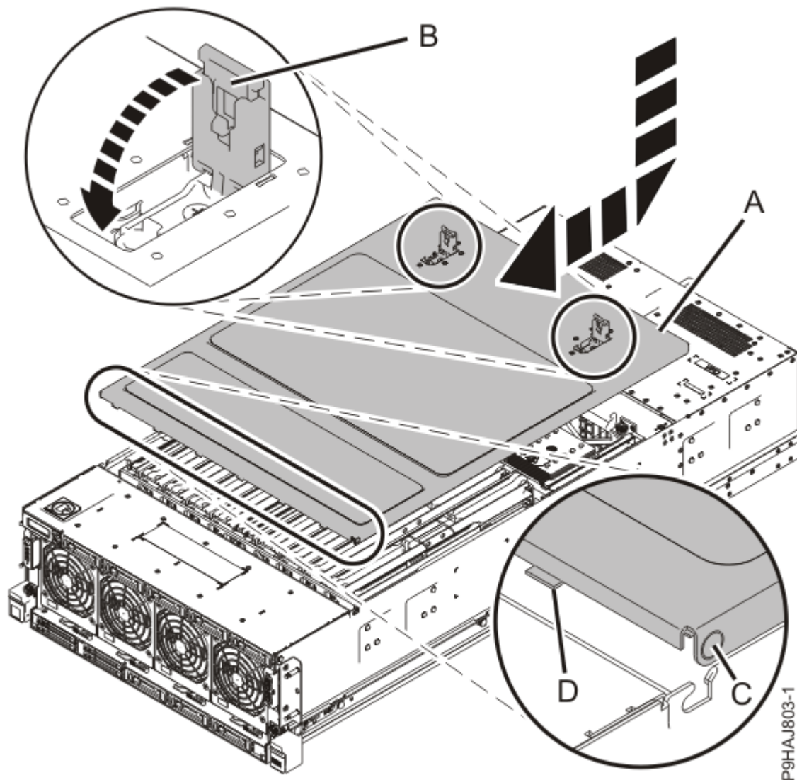
図 57. 保守アクセス・カバーの取り付け
