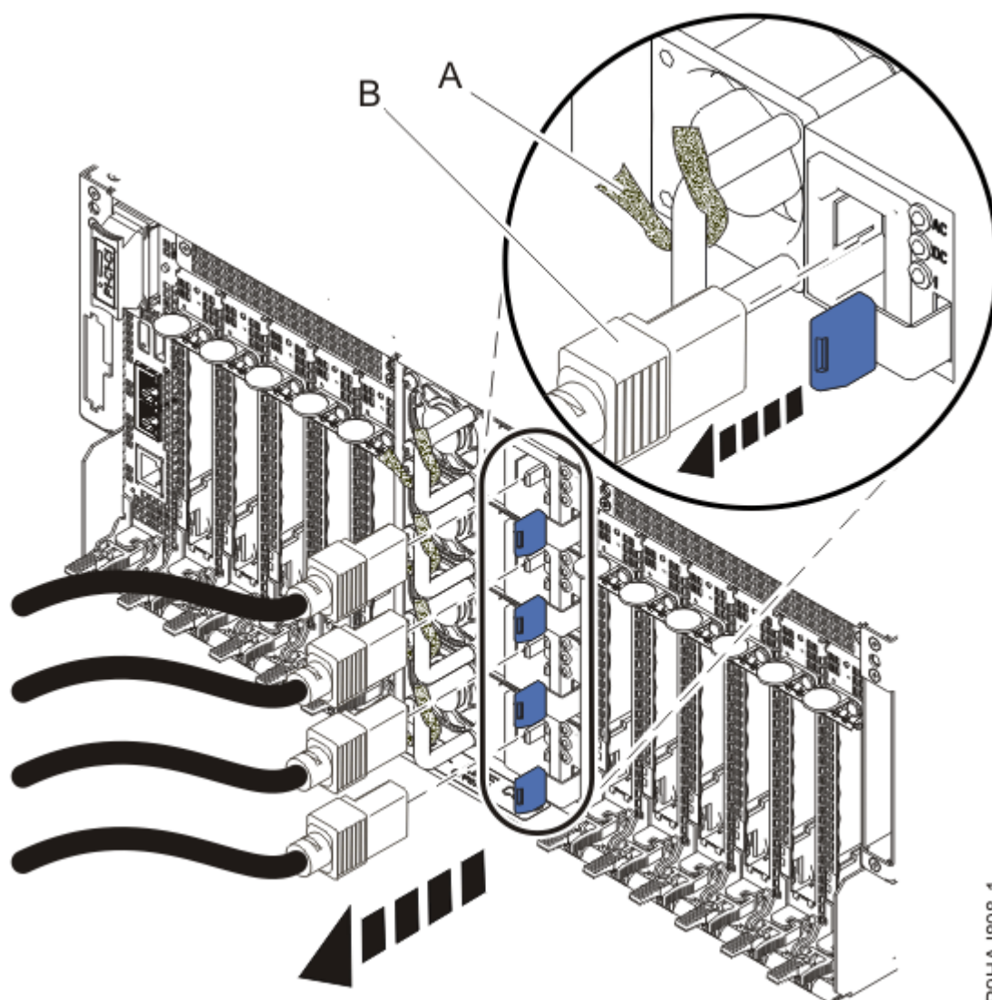
図 23. 電源コードの取り外し
