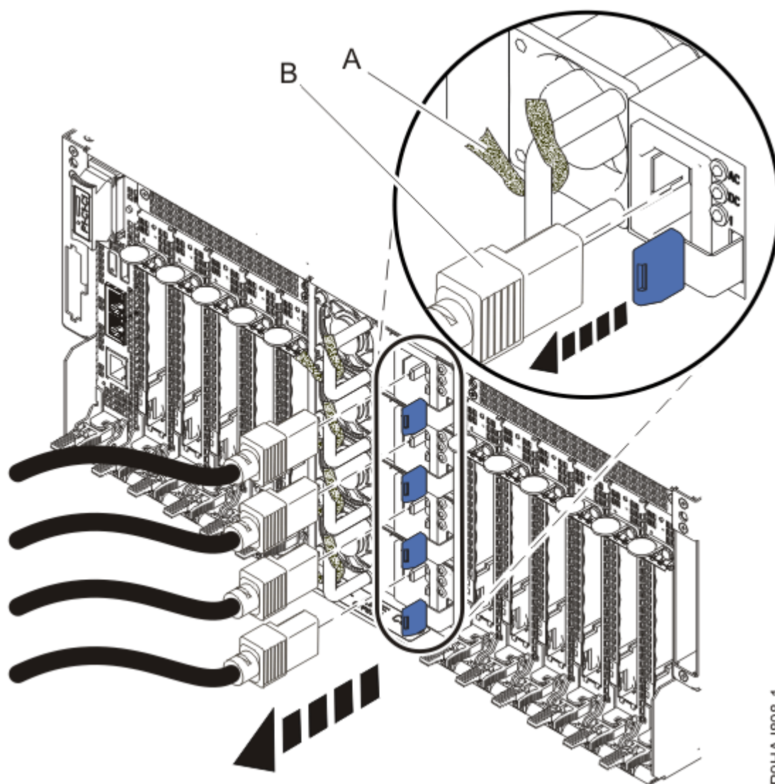
図 52. 電源コードの取り外し
