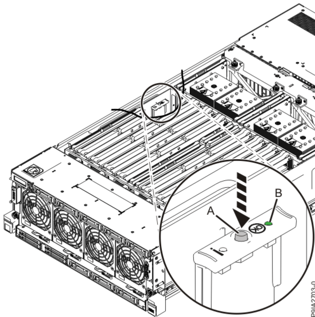
図 13. 識別 LED の活動化
