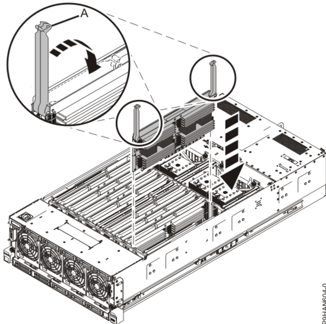
図 6. メモリー・ライザーの挿入
