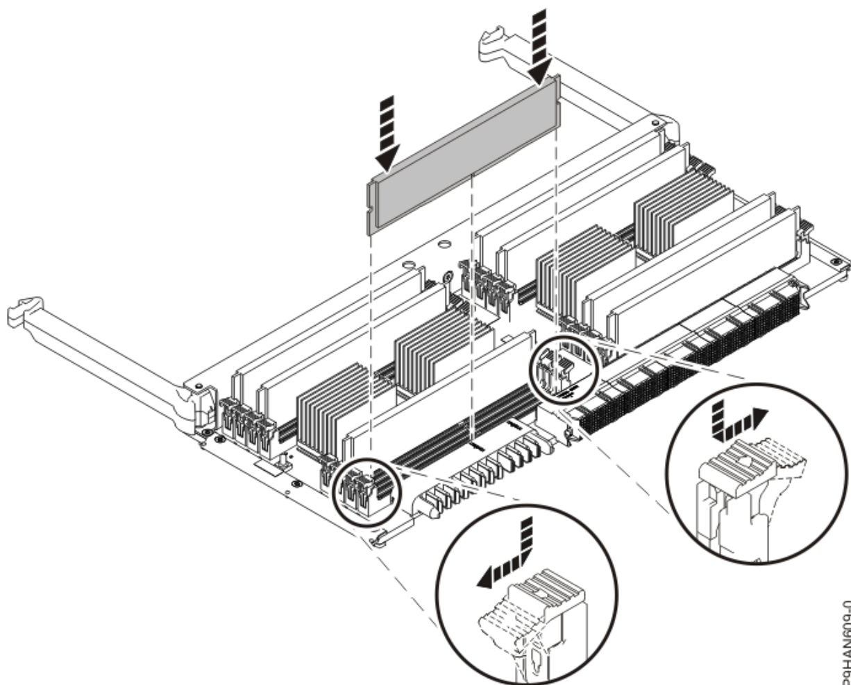
図 5. メモリー・ライザーへのメモリー・モジュールの取り付け
