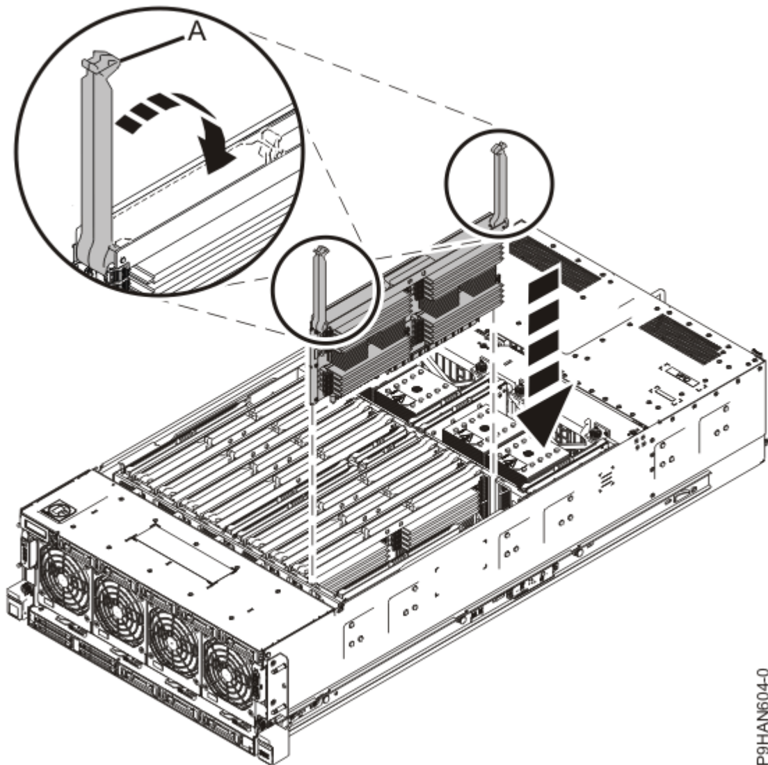
図 48. メモリー・ライザーの挿入
