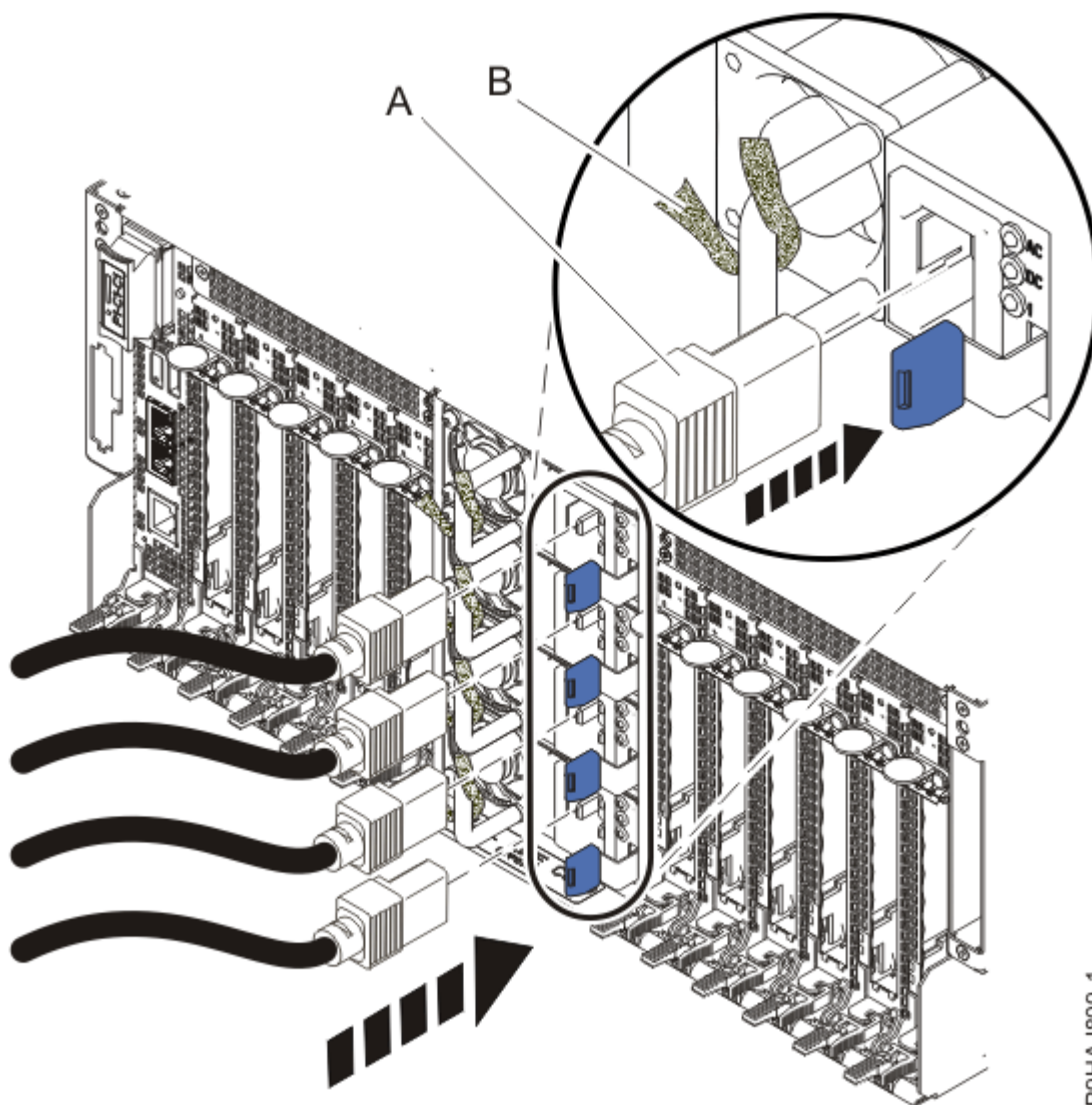
図 9. 電源コードの接続
