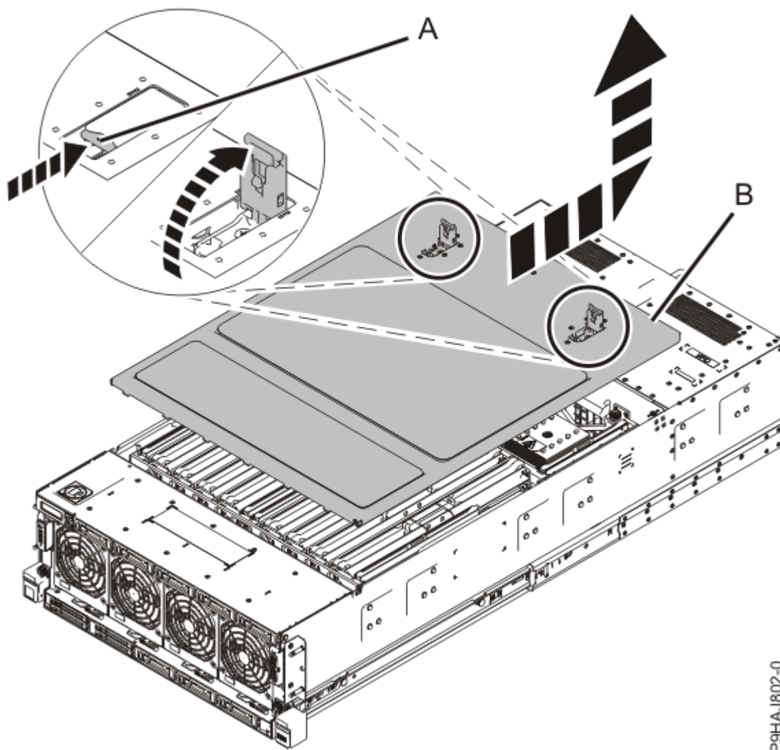
図 54. 保守アクセス・カバーの取り外し
