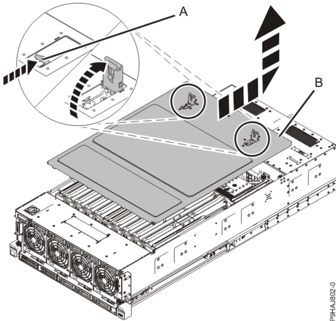
図 42. 保守アクセス・カバーの取り外し
