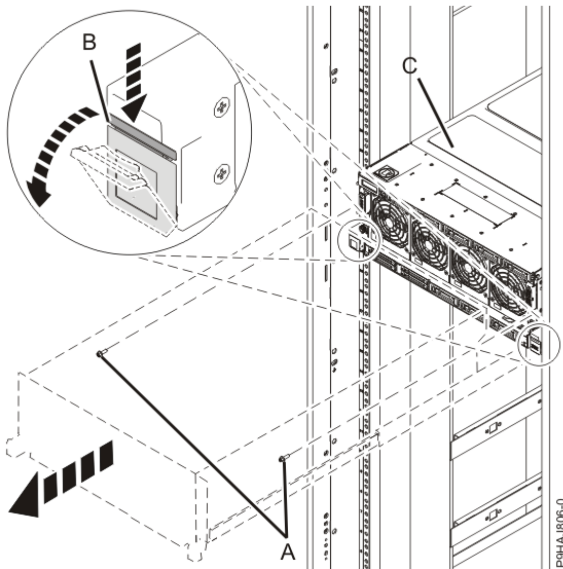
図 53. システムの保守位置への設置
