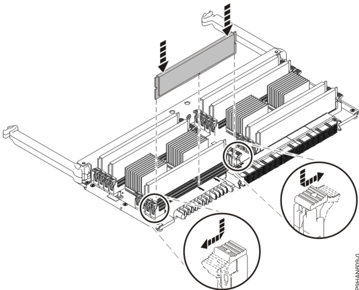
図 47. メモリー・モジュールの取り替え
