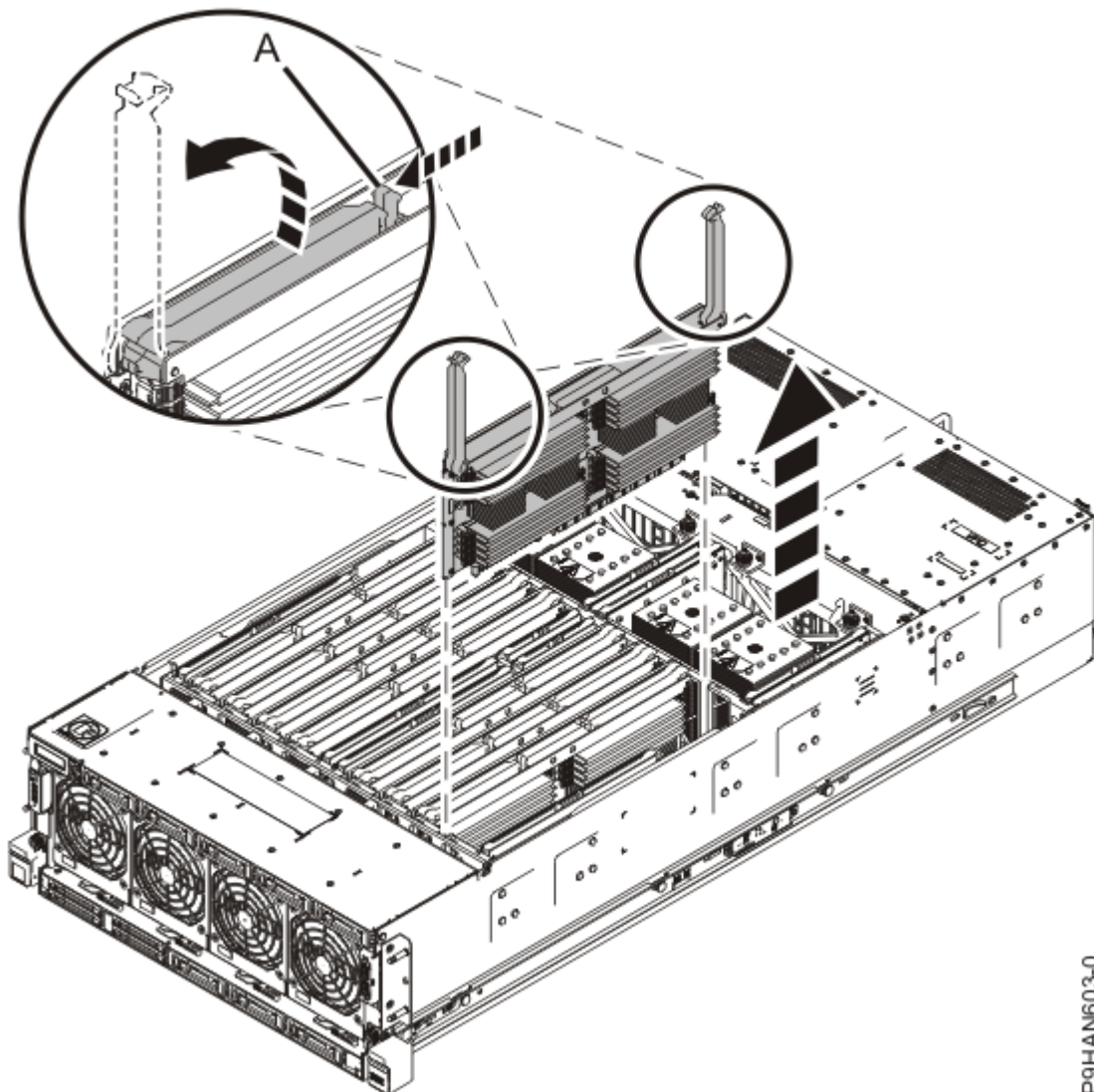
図 45. メモリー・ライザーの取り外し
