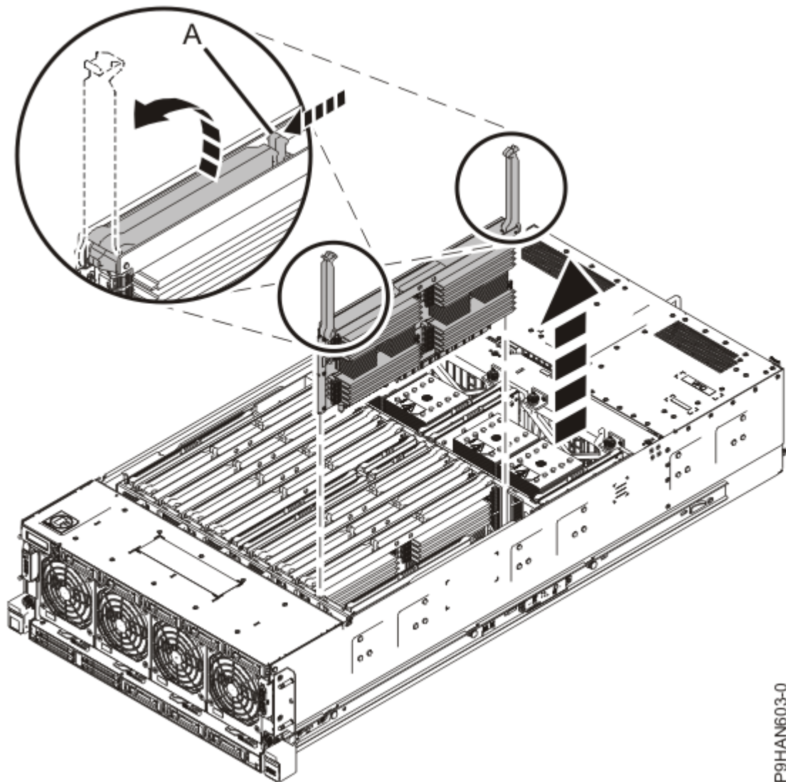
図 15. メモリー・ライザーの取り外し
