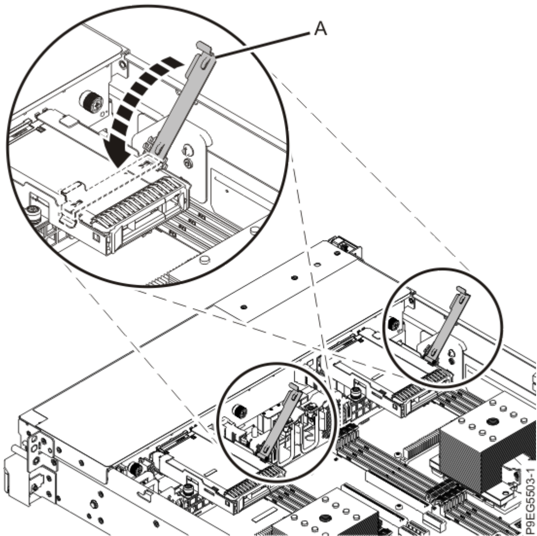
図 22. BPM ホルダー・レバーを閉じる
