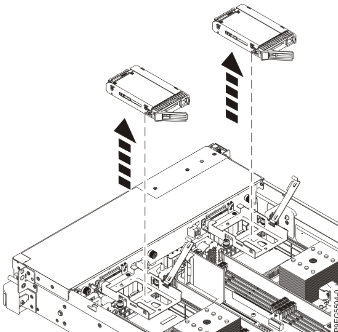
図 15. BPM の取り外し
