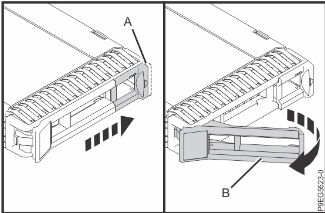
図 11. BPM ハンドルのロック解除
