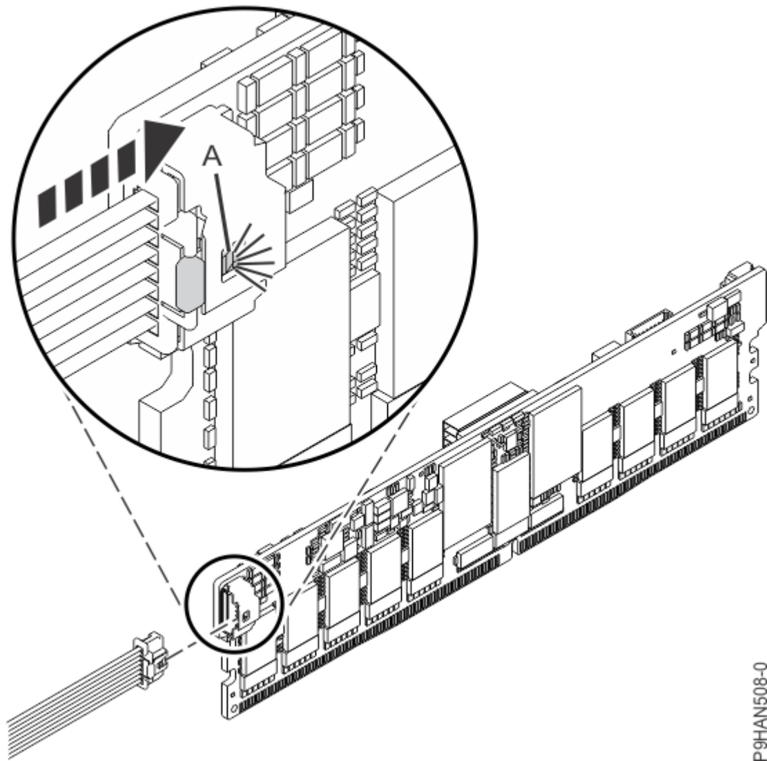
図 25. NVDIMM への BPM ケーブルの接続
