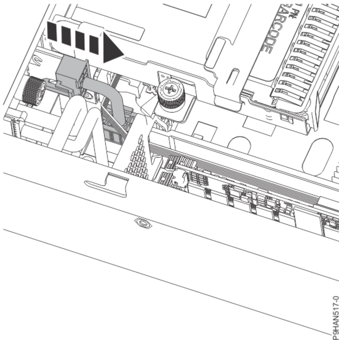
図 9. ドライブ・バックプレーン電源ケーブルの取り外し
