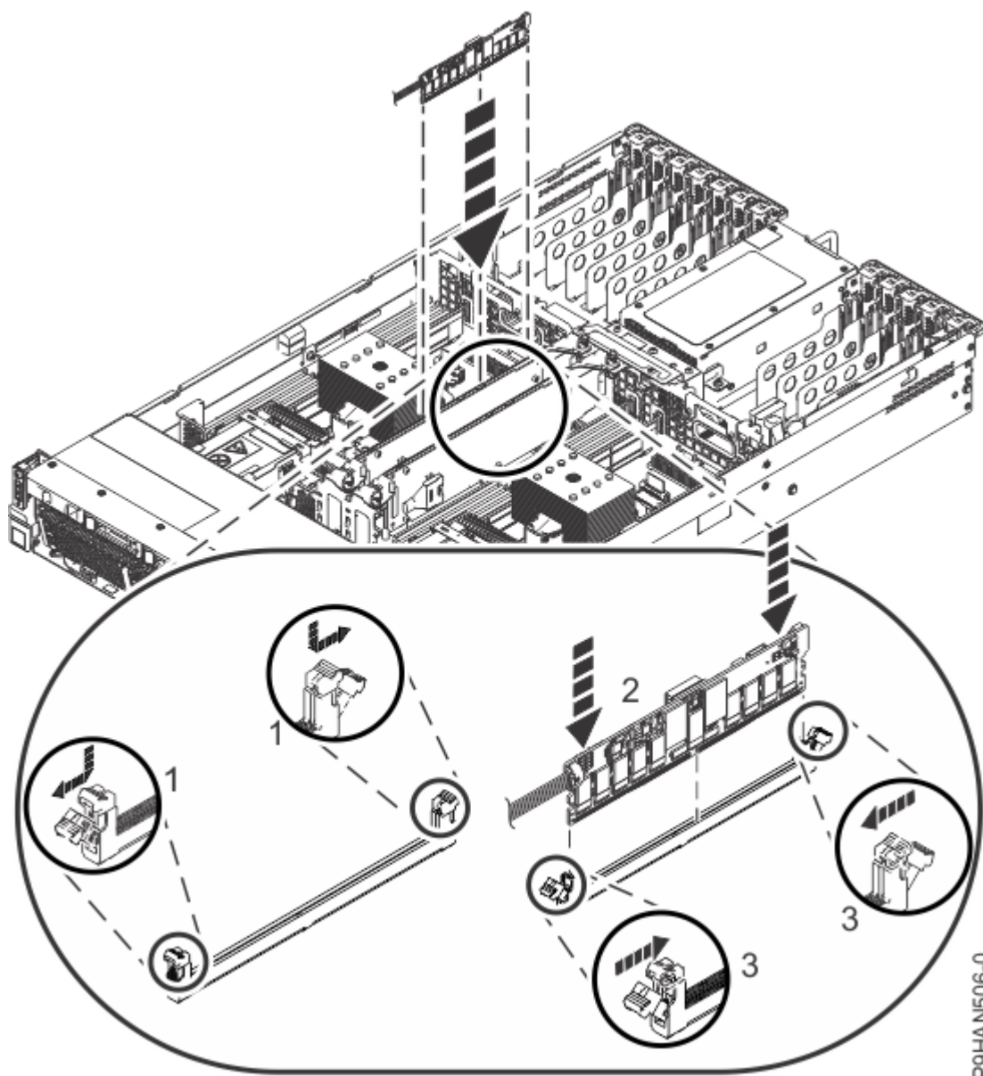
図 26. NVDIMM の再取り付け
