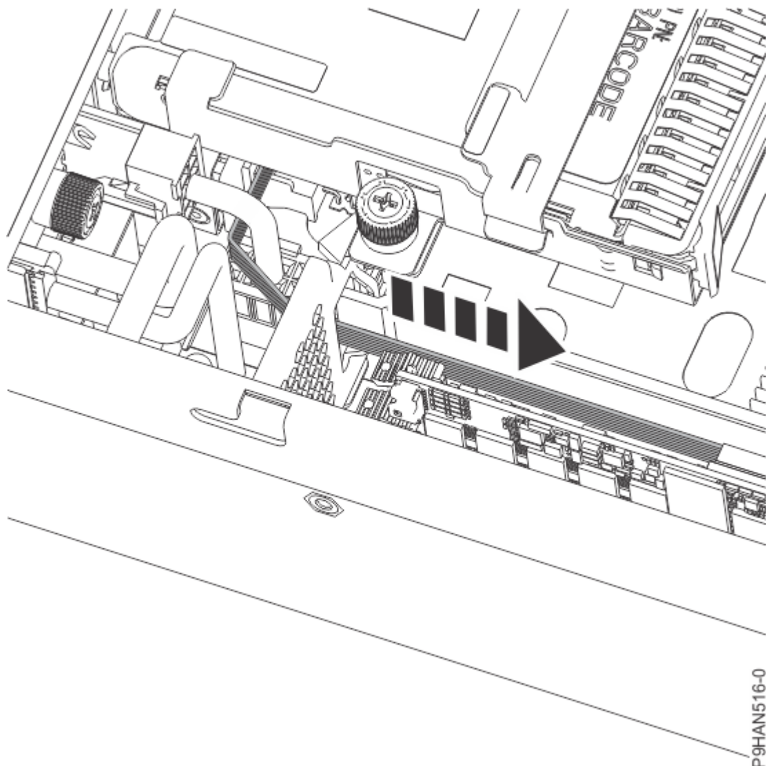
図 24. BPM を引いてケーブルの遊びを取り除く
