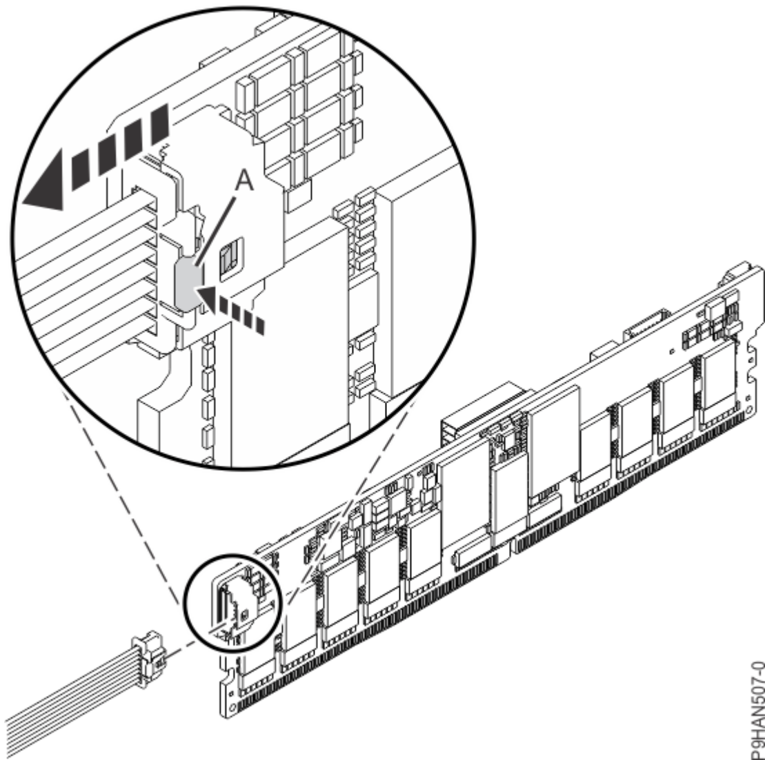
図 7. NVDIMM からの BPM ケーブルの取り外し
