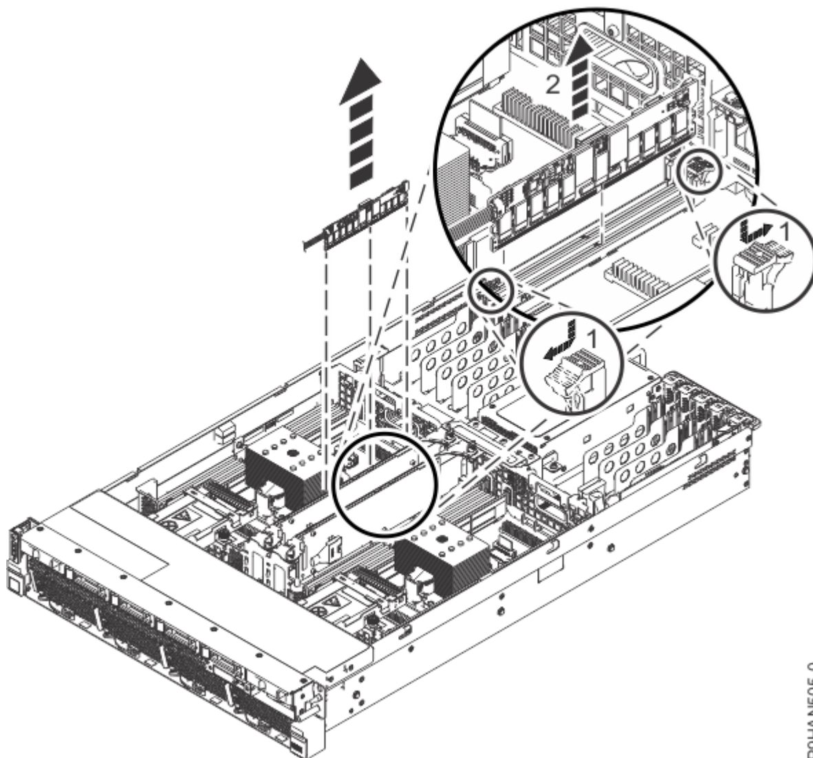
図 6. NVDIMM の取り外し
