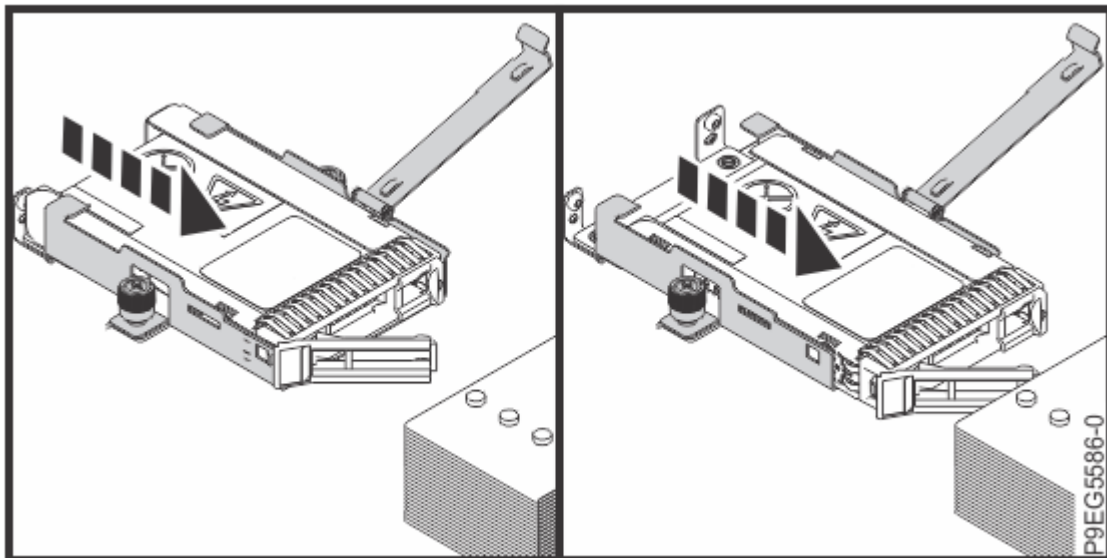
図 12. 前方への BPM のスライド
