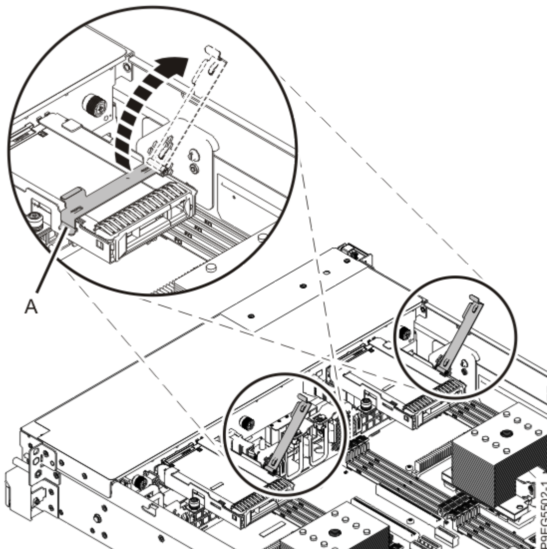
図 10. BPM ホルダー・レバーを開く
