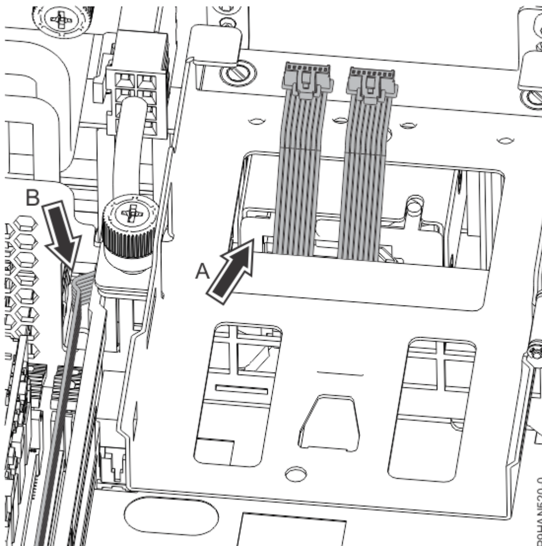
図 16. シートメタル・カットアウトからの BPM ケーブルの取り外し
