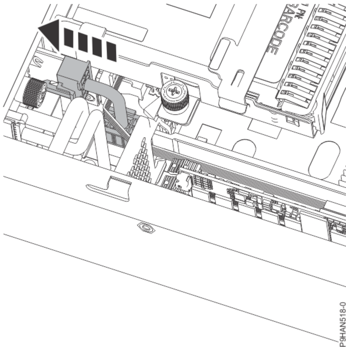
図 23. ドライブ・バックプレーン電源ケーブルの再接続
