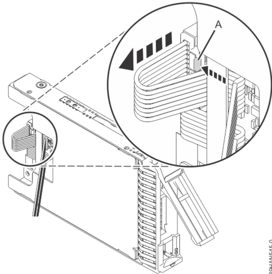
図 14. BPM ケーブルの取り外し f) BPM を取り外します。次の図を参照してください。
