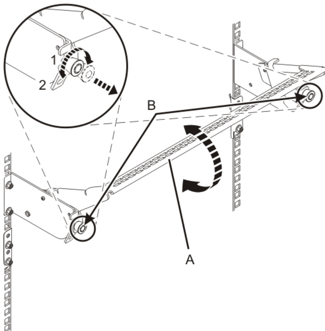
図 25. 下げた操作位置へのケーブル管理ブラケットの設置
