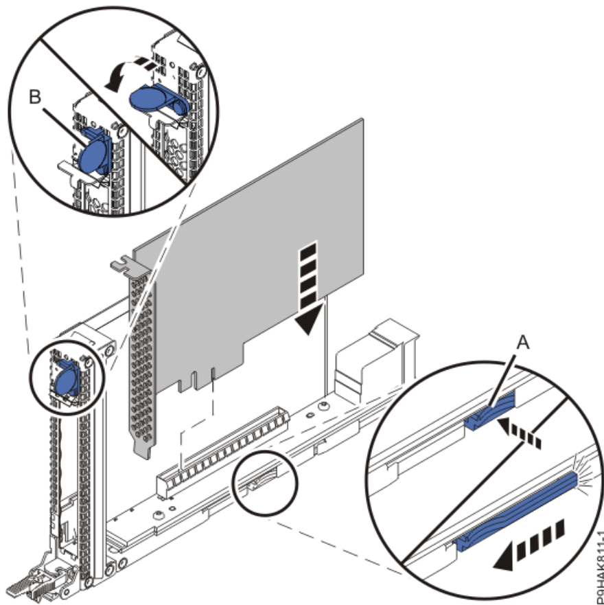
図 23. 9040-MR9 システムのカセットへのアダプターの取り付け
