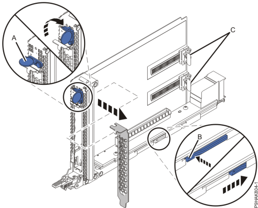
図 5. 9040-MR9 システムのカセットからのテール・ストック・フィラーの取り外し
