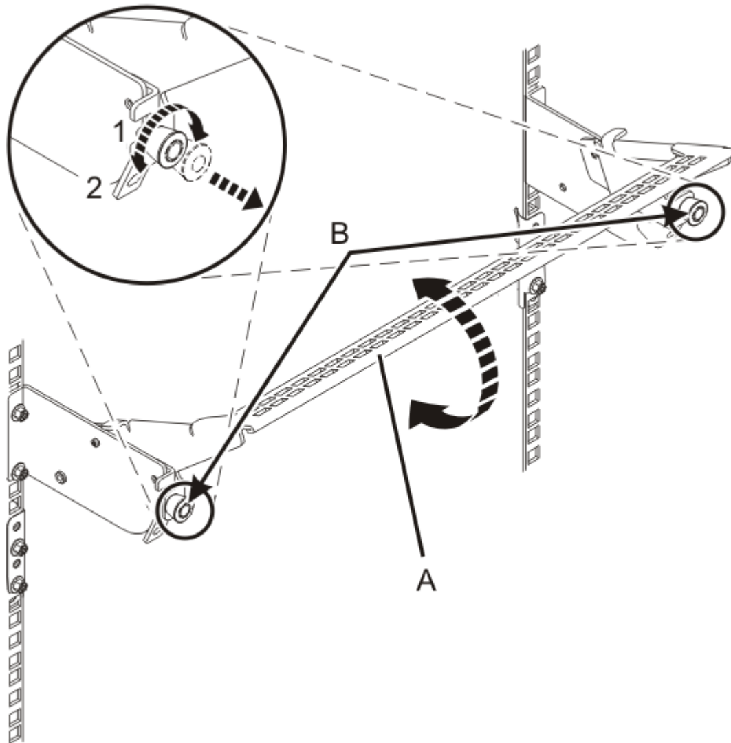
図 28. 上げた保守位置へのケーブル管理ブラケットの設置
