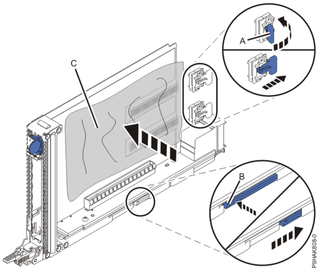
図 6. 9040-MR9 カセットのストリップを ESD 安全シートでカバー
