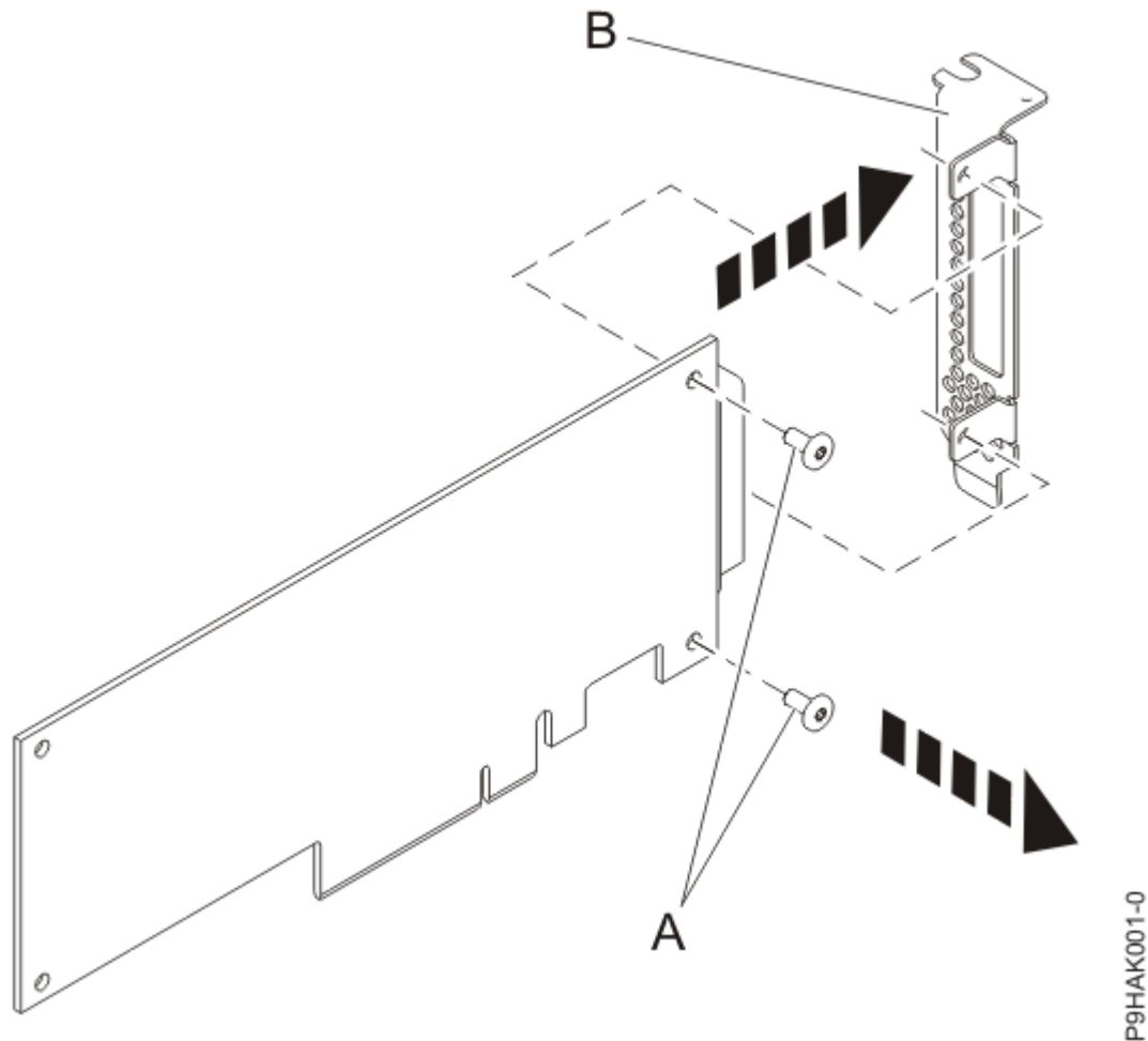
図 36. アダプターからのロープロファイル・テール・ストックの取り外し
