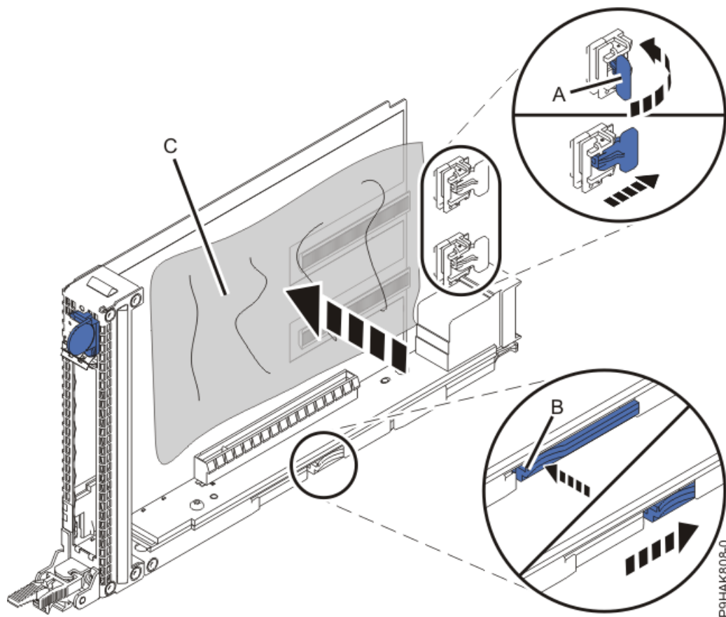
図 20. 9040-MR9 カセットのストリップを ESD 安全シートでカバー
