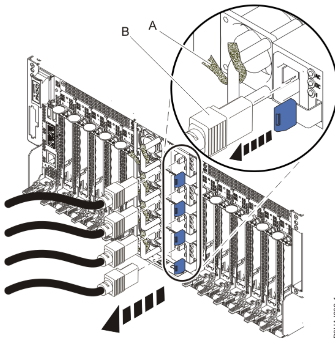
図 2. 電源コードの取り外し
