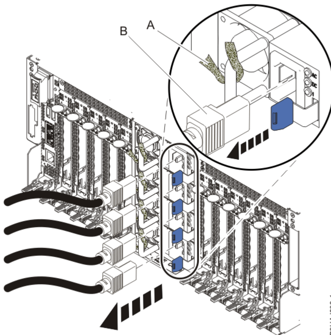
図 27. 電源コードの取り外し
