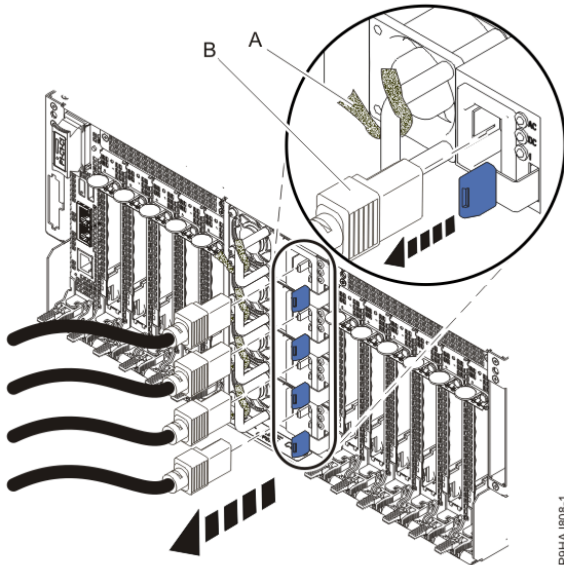
図 14. 電源コードの取り外し
