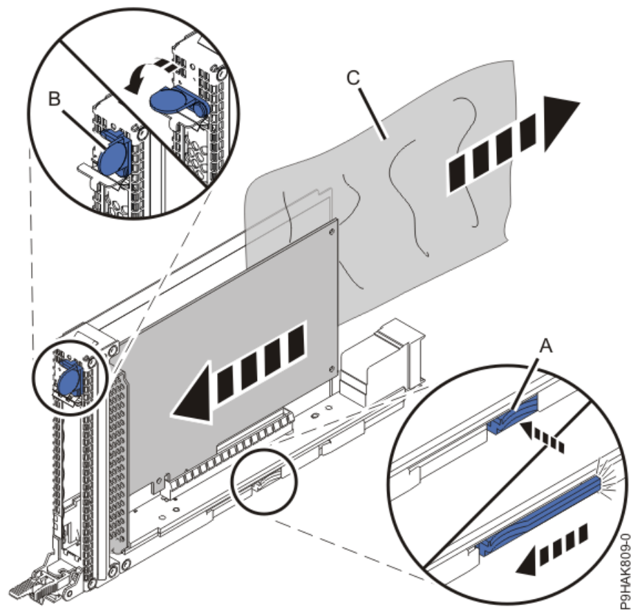
図 21. 9040-MR9 システムのカセットへのアダプターの取り付け
