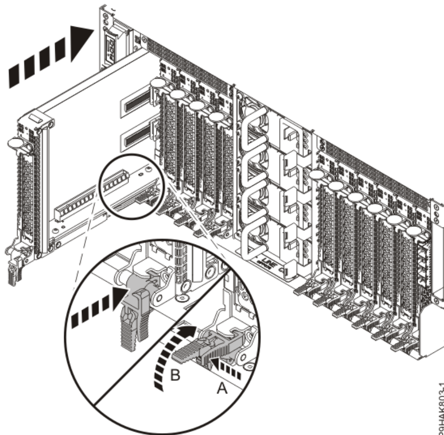
図 24. 9040-MR9 システムでのカセットの取り付け
