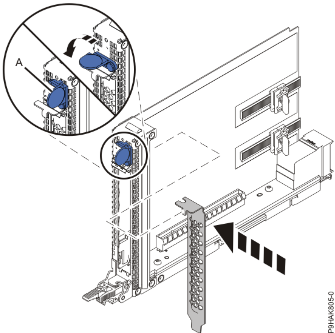
図 32. 9040-MR9 システムのカセットへのアダプターの再取り付け 8. 以下のステップを実行して、カセットをスライドさせてスロットに収めます。
