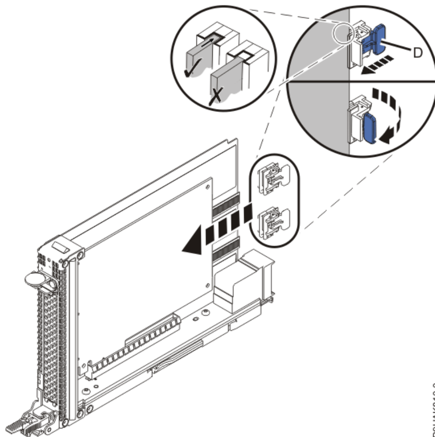
図 22. 9040-MR9 システムのアダプター保持器具を使用したアダプターの固定
