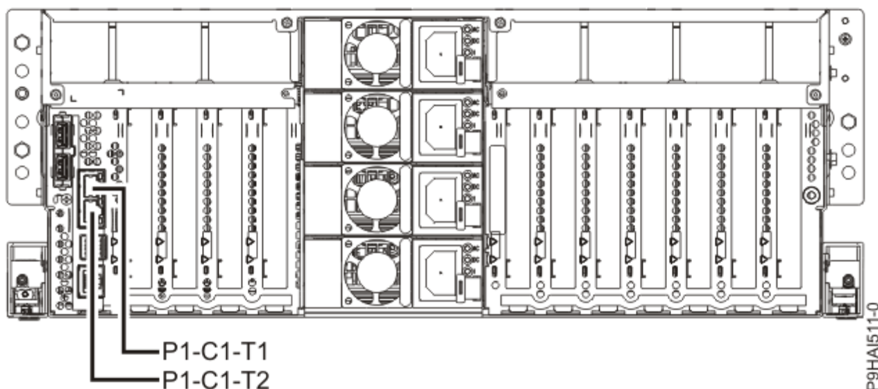
図 27. 9009-41A、9009-41G、9009-42A、9009-42G、9223-42H、および 9223-42S HMC ポートの位置
