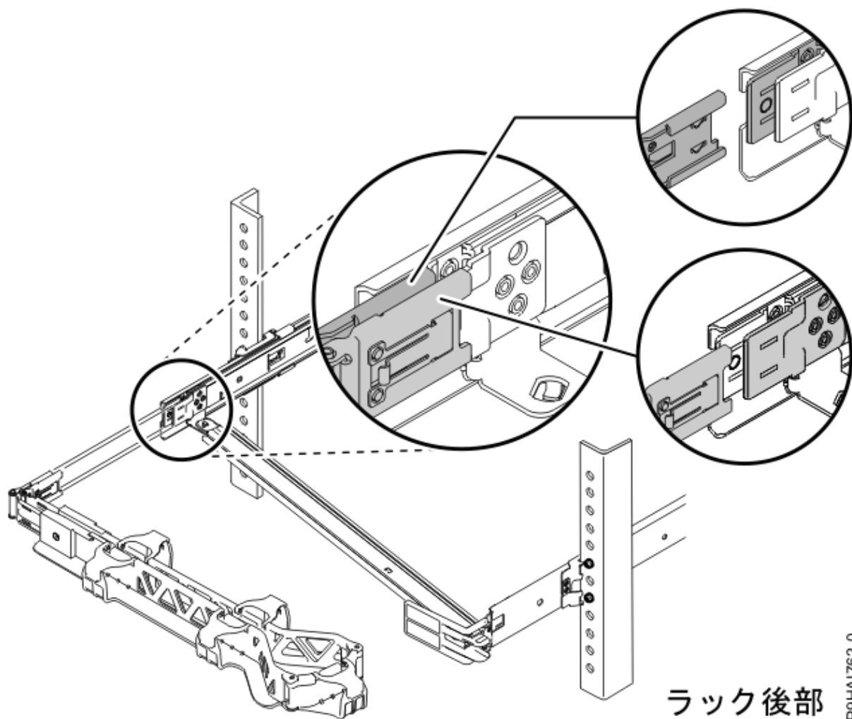
図 20. ケーブル・マネージメント・アームの接続
