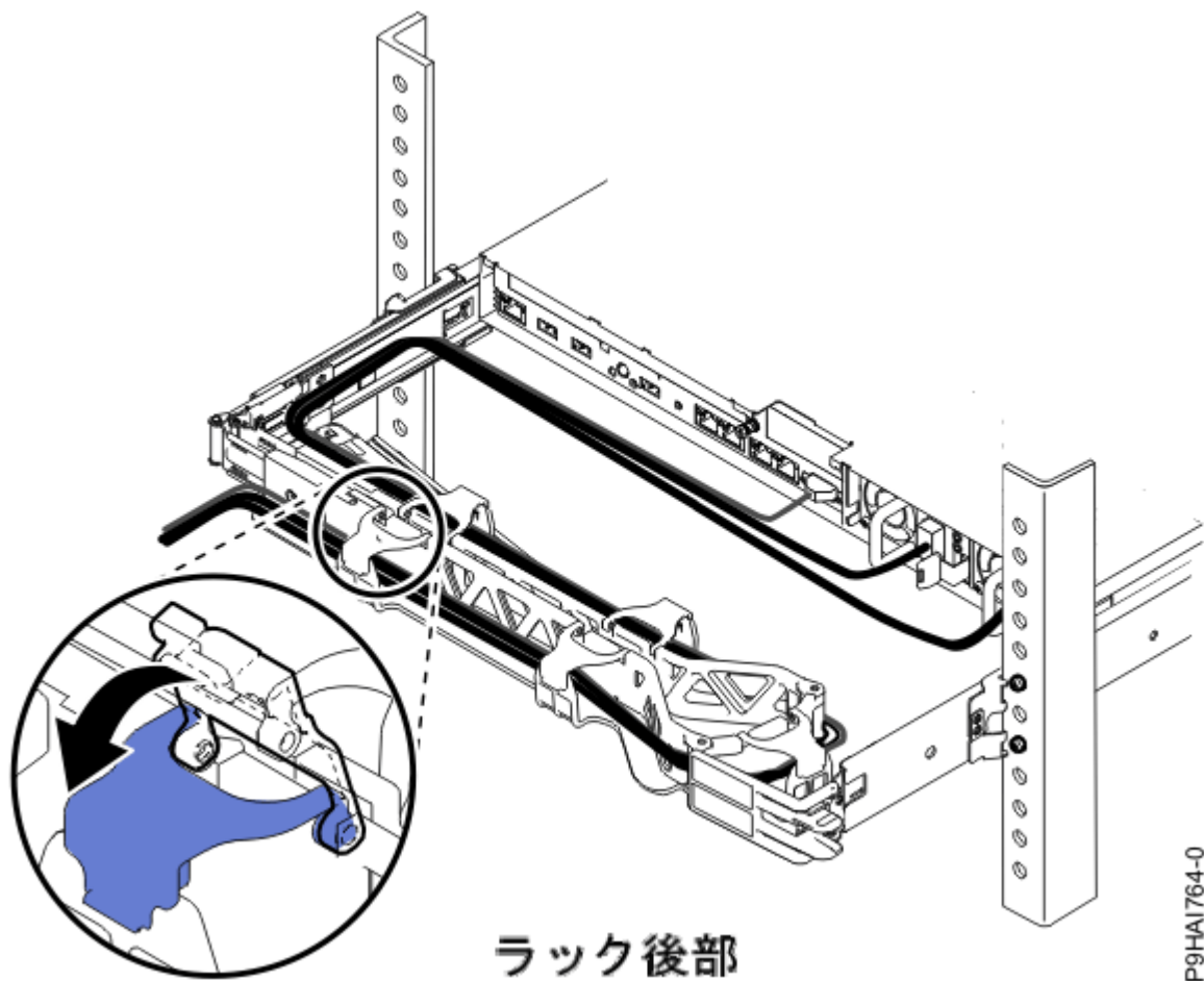
図 22. 電源コードの取り付けとケーブルの配線
