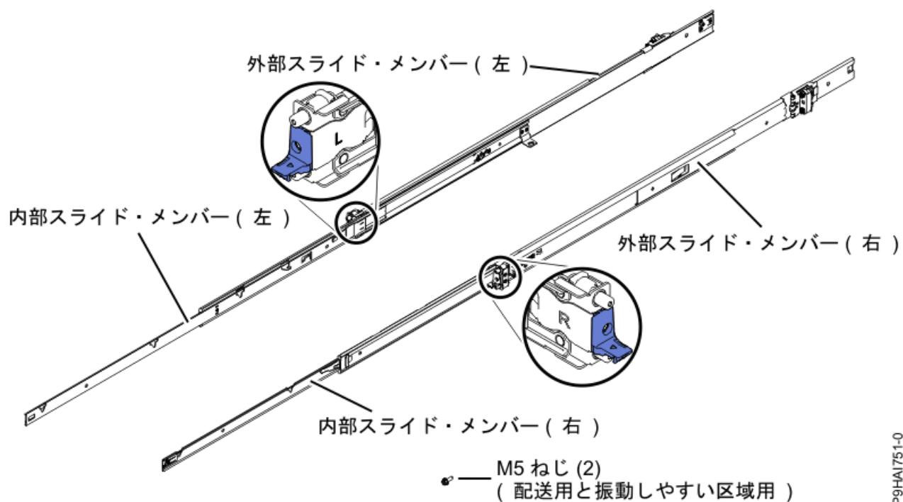
図 10. レール・ボックスの内容
