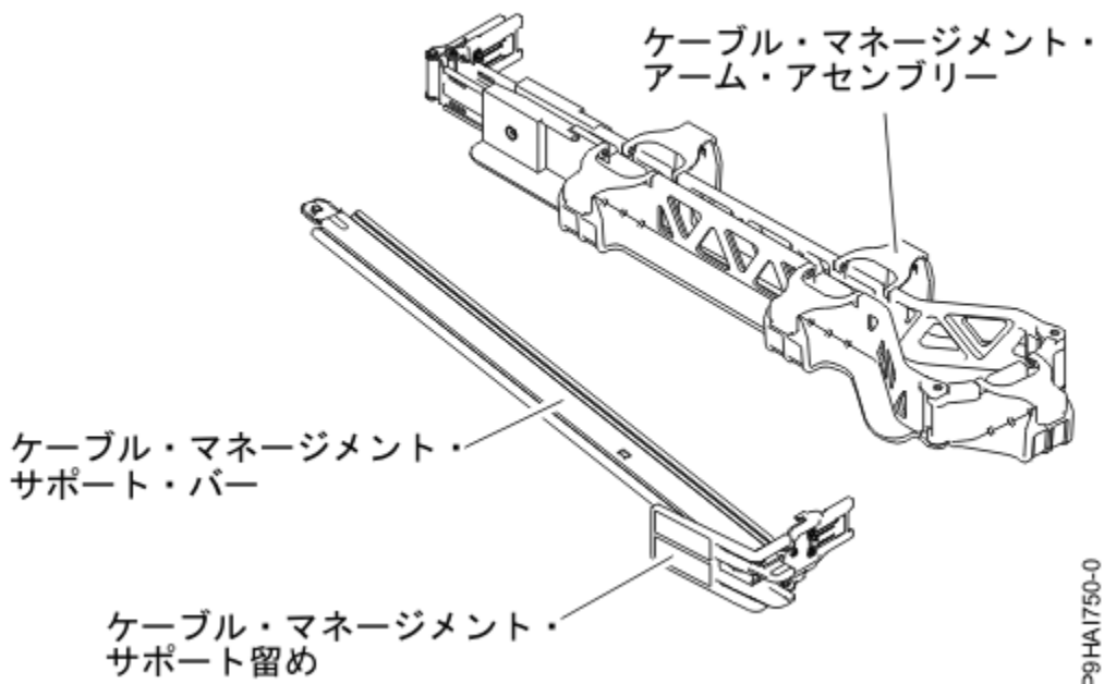
図 9. ケーブル・マネージメント・アーム・ボックスの内容
