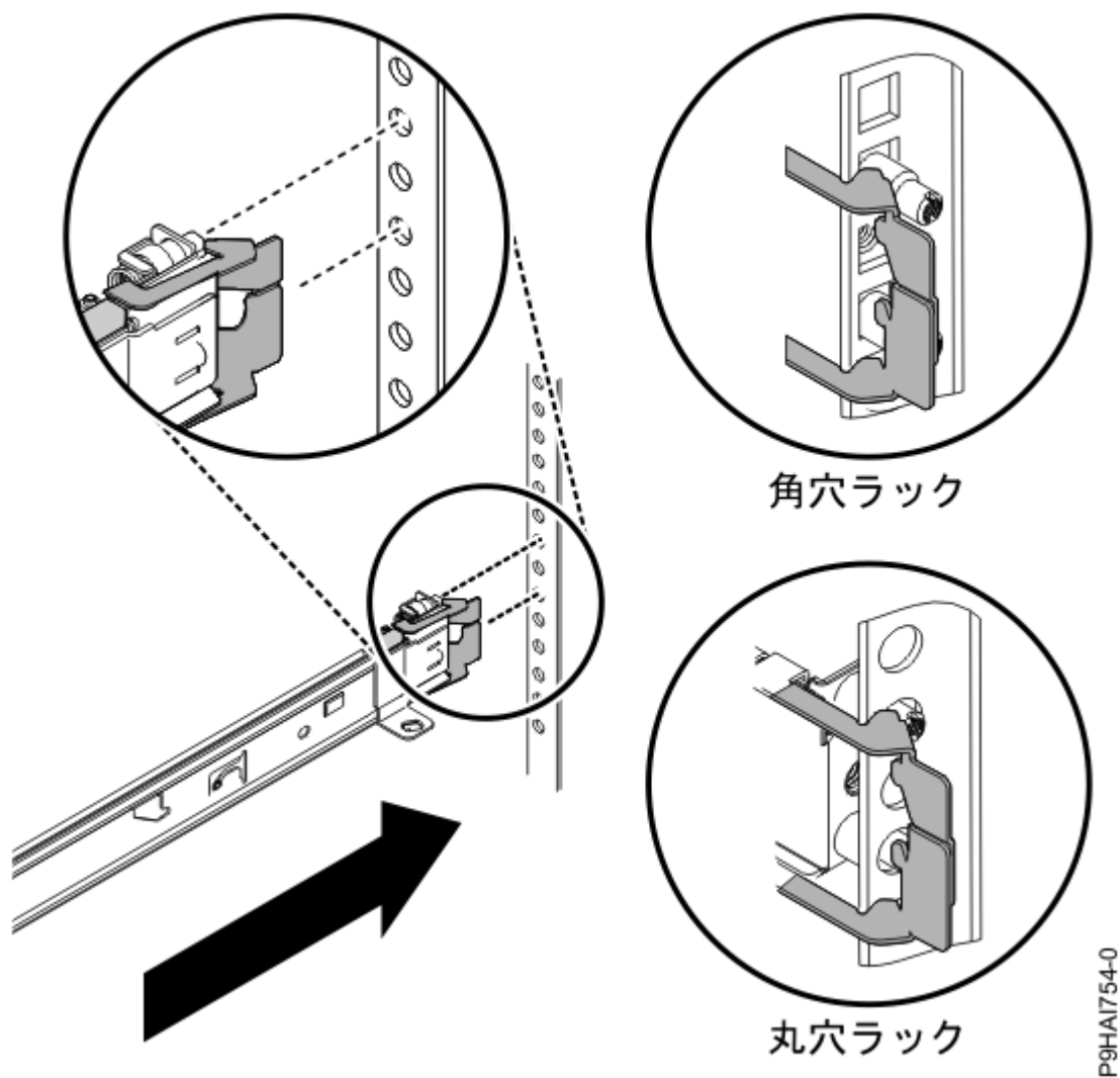
図 13. ピンとラック後部の穴の位置合わせ
