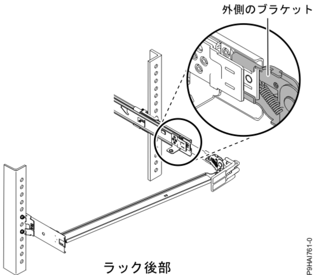
図 19. スライド・レールへの停止ブラケットの接続
