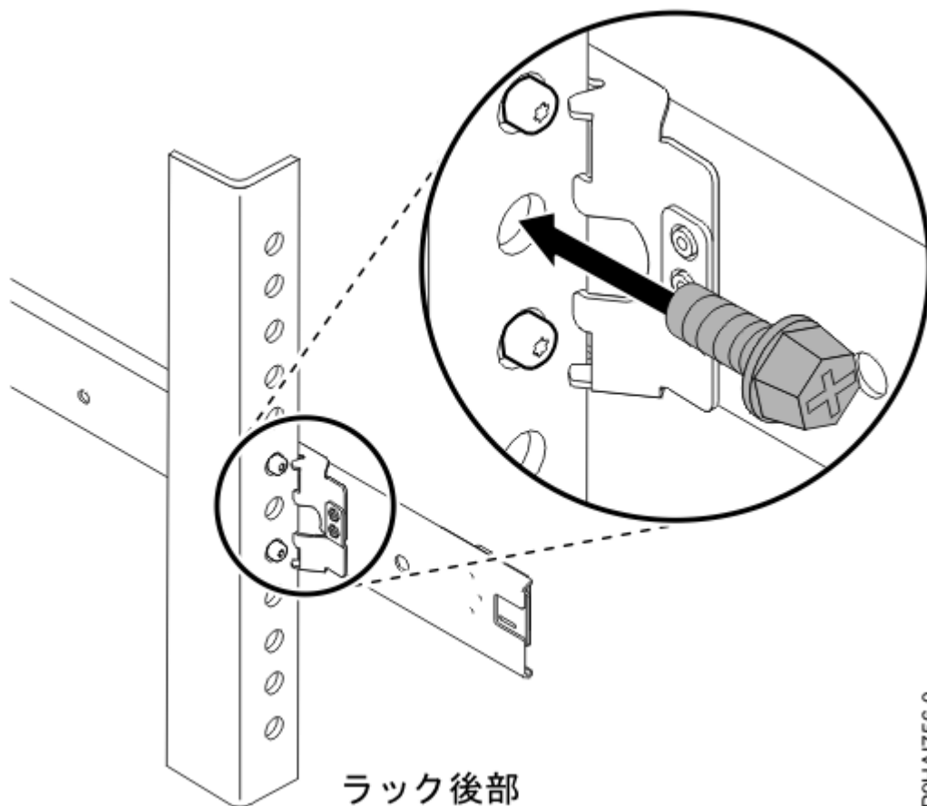
図 24. 配送のためのサーバーの固定
