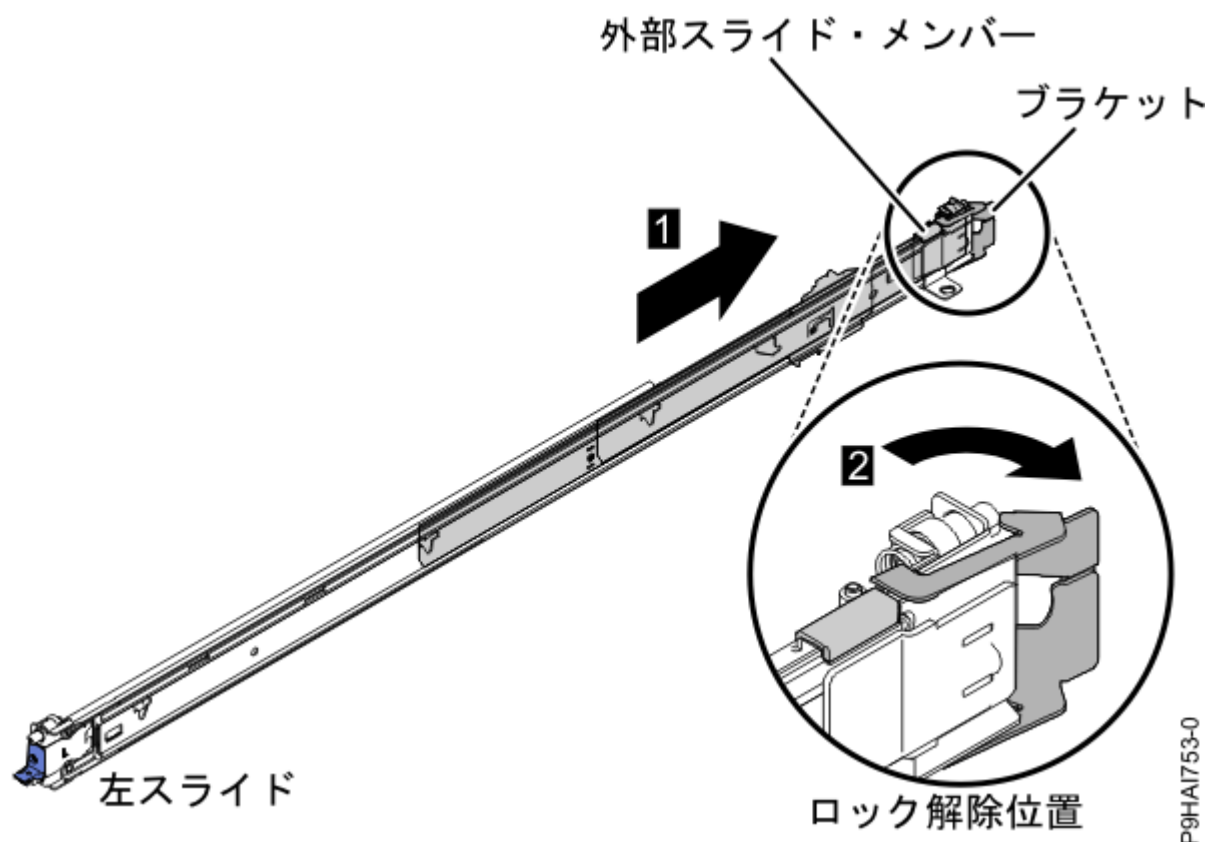
図 12. スライド・レールと外部スライド・メンバー
