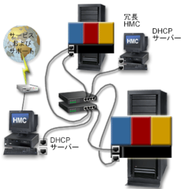
図 25. DHCP サーバーとしての 1 台の HMC を持つプライベート・ネットワーク
