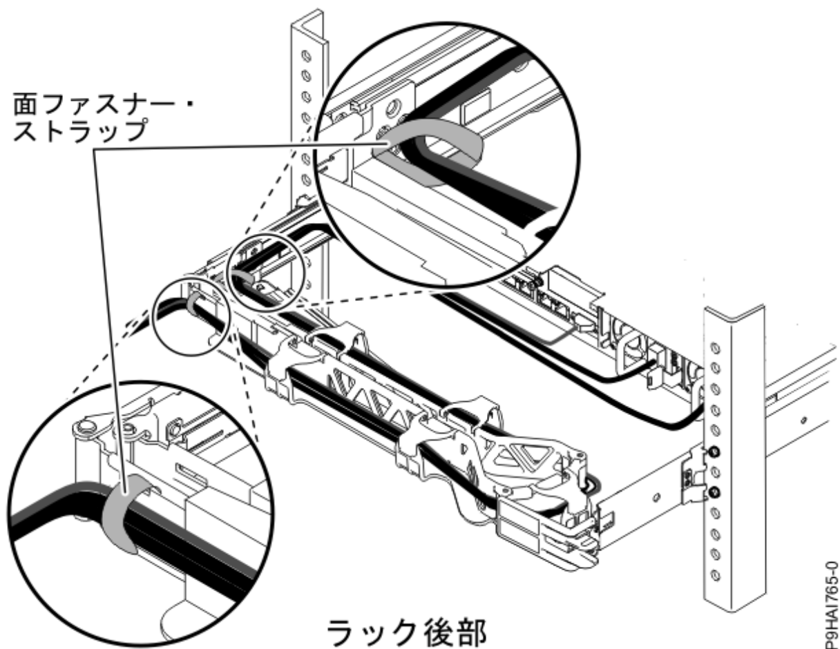
図 23. 面ファスナー
