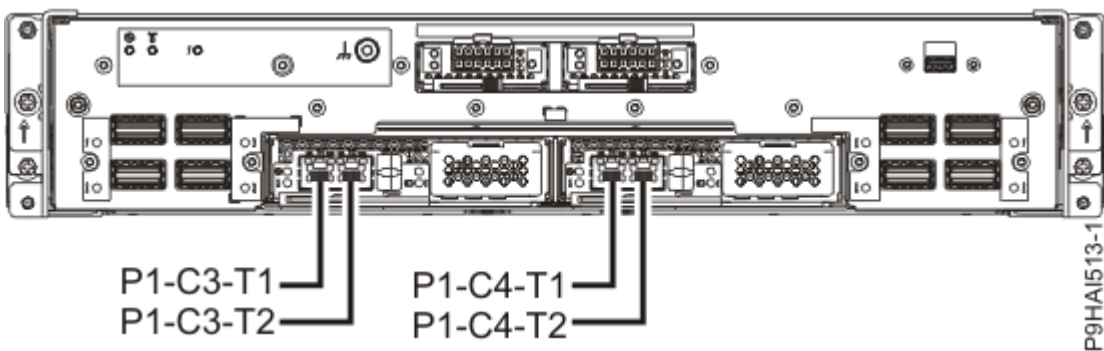
図 29. 9080-M9S の HMC ポート位置
