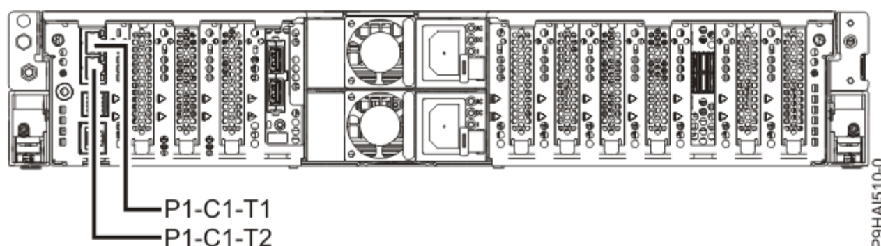
図 26. 5105-22E、9008-22L、9009-22A、9009-22G、9223-22H、および 9223-22S HMC ポートの位置
