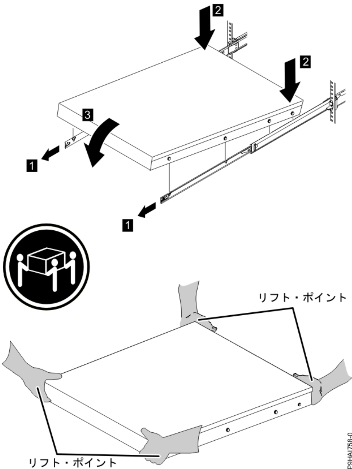
図 16. 引き出したスライド・レール、レールのスロットと位置合わせしたサーバーのくぎの頭、およびリフト・ポイント
