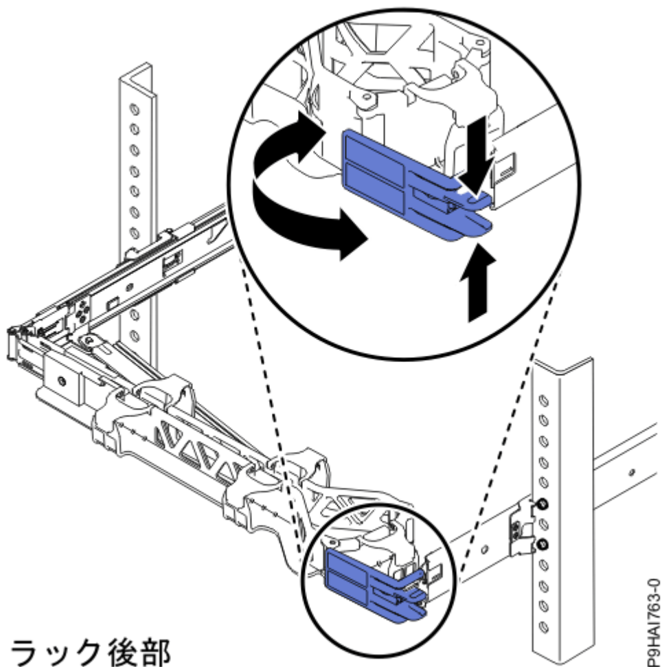
図 21. ケーブル・マネージメント・サポート留めブラケット
