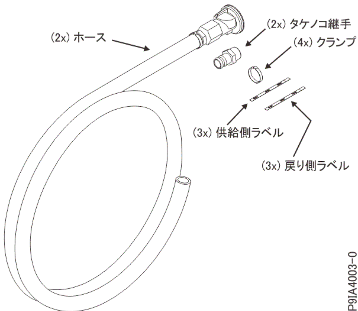
図 26. ホース・キット
