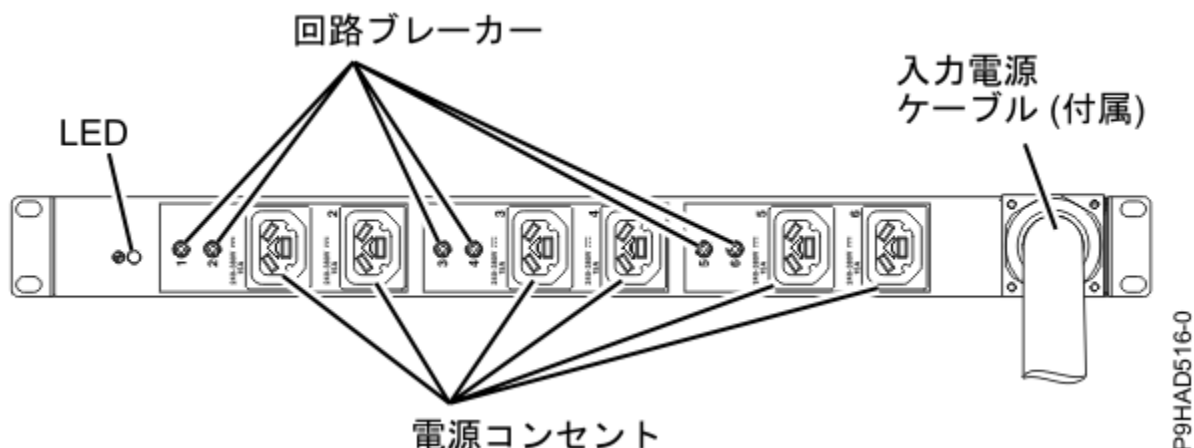
図 42. HVDC PDU
