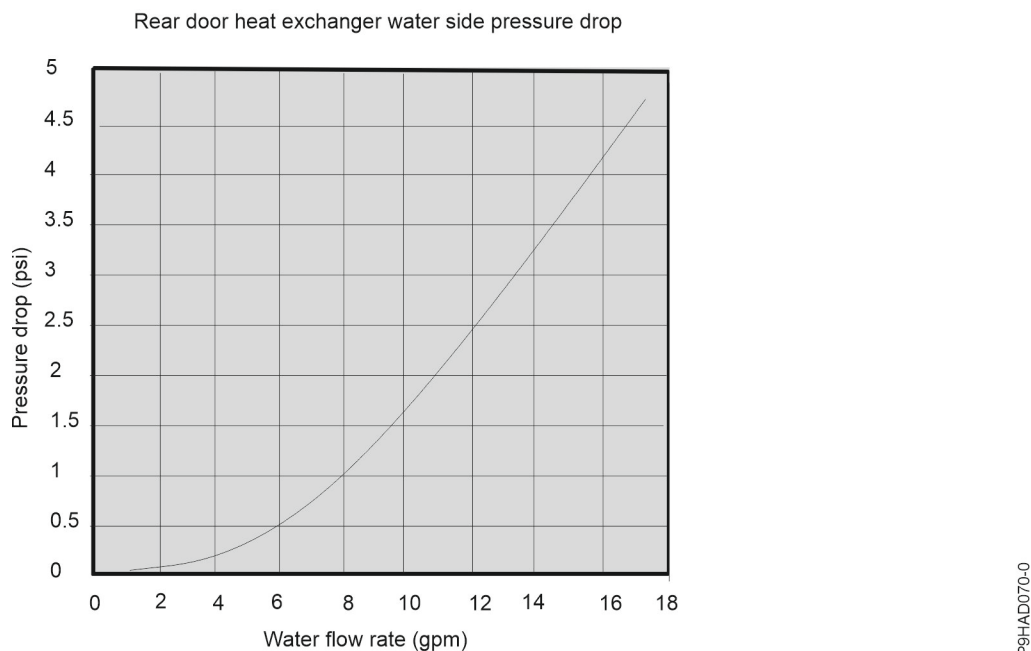
図 24. 圧力低下 (標準法)
