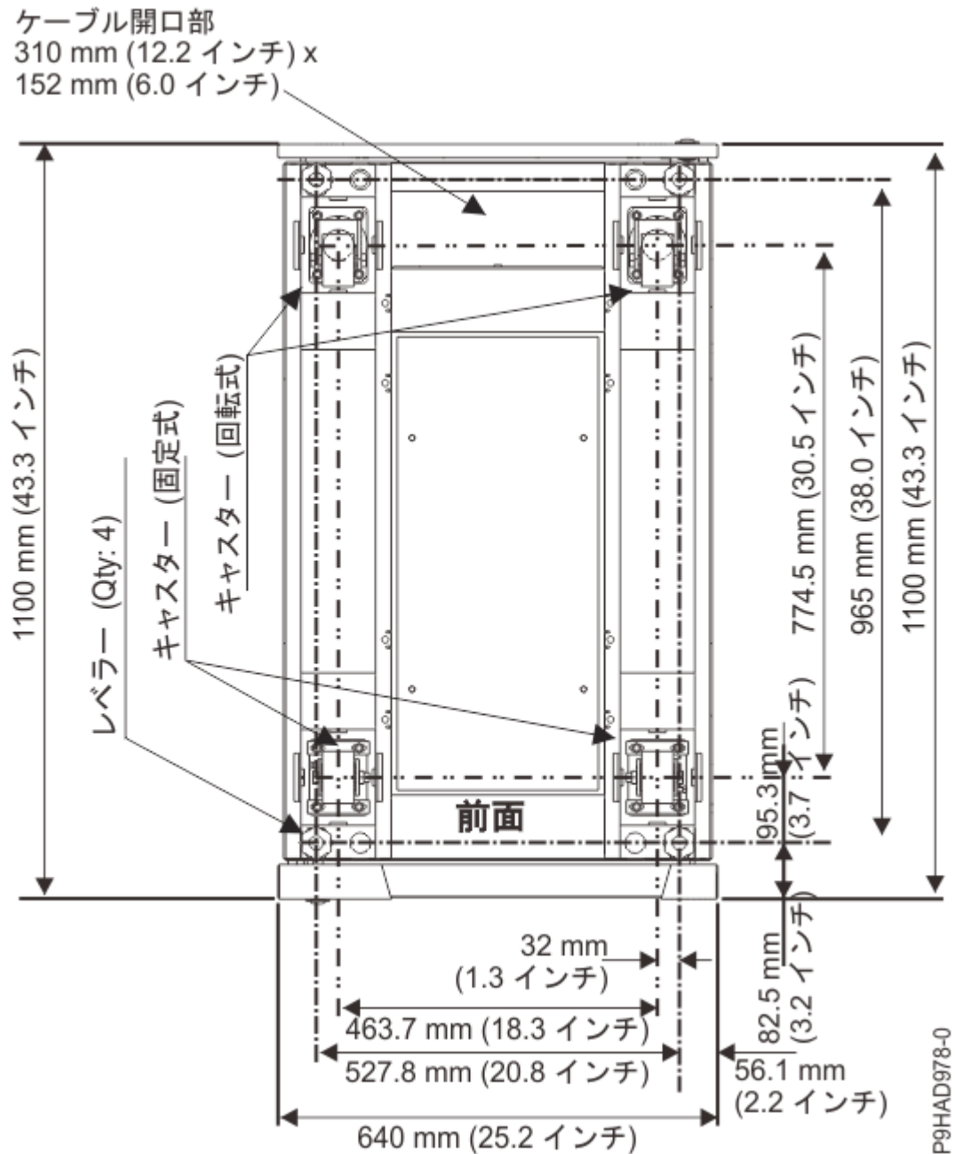
図 4. キャスターおよびレベルの位置
