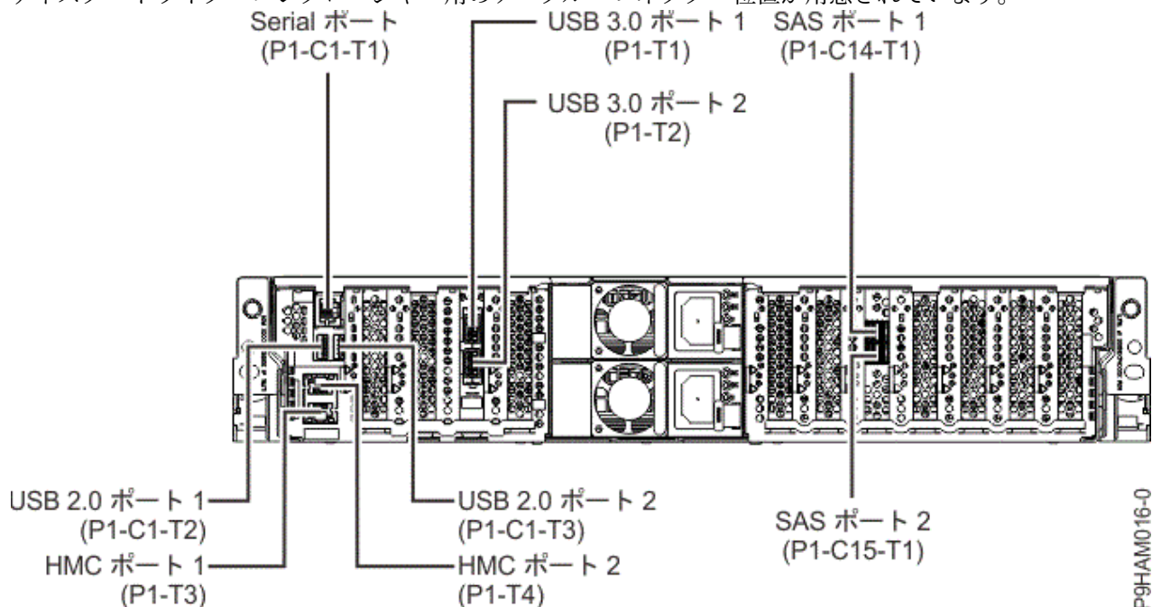
図 35. 拡張機能 8247-21L、8247-22L、8284-21A、および 8284-22A の各システムのコネクター位置
