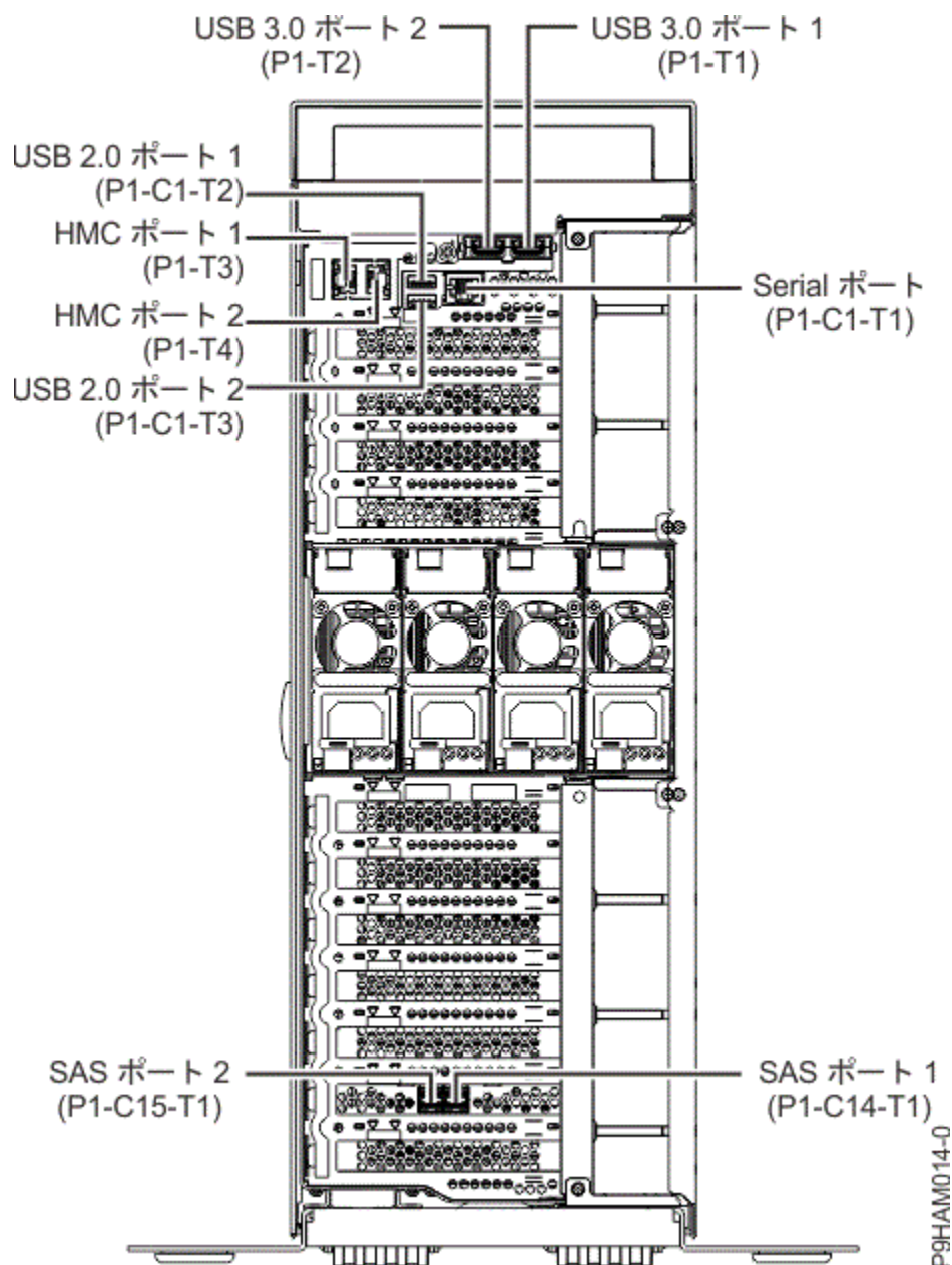
図 37. スタンドアロン 8286-41A (拡張機能) システムのコネクター位置
