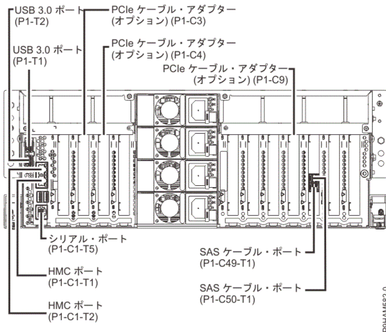
図 32. 9009-41A、9009-41G、9009-42A、9009-42G、および 9223-42H システムのコネクター位置
