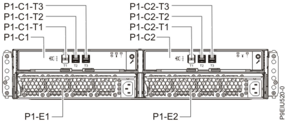
図 30. ESLL ストレージ・エンクロージャーおよび ESLS ストレージ・エンクロージャー のコネクタ位置
