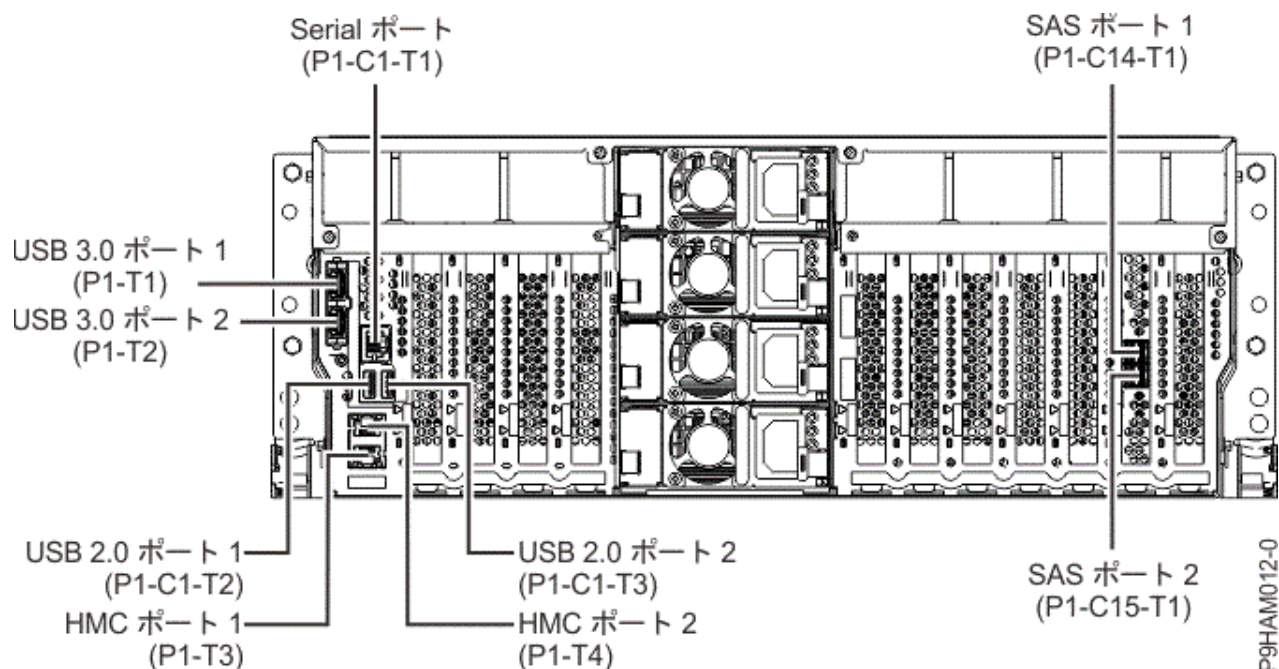
図 38. 8247-42L システムおよび 8286-42A (拡張機能) システムのコネクター位置
