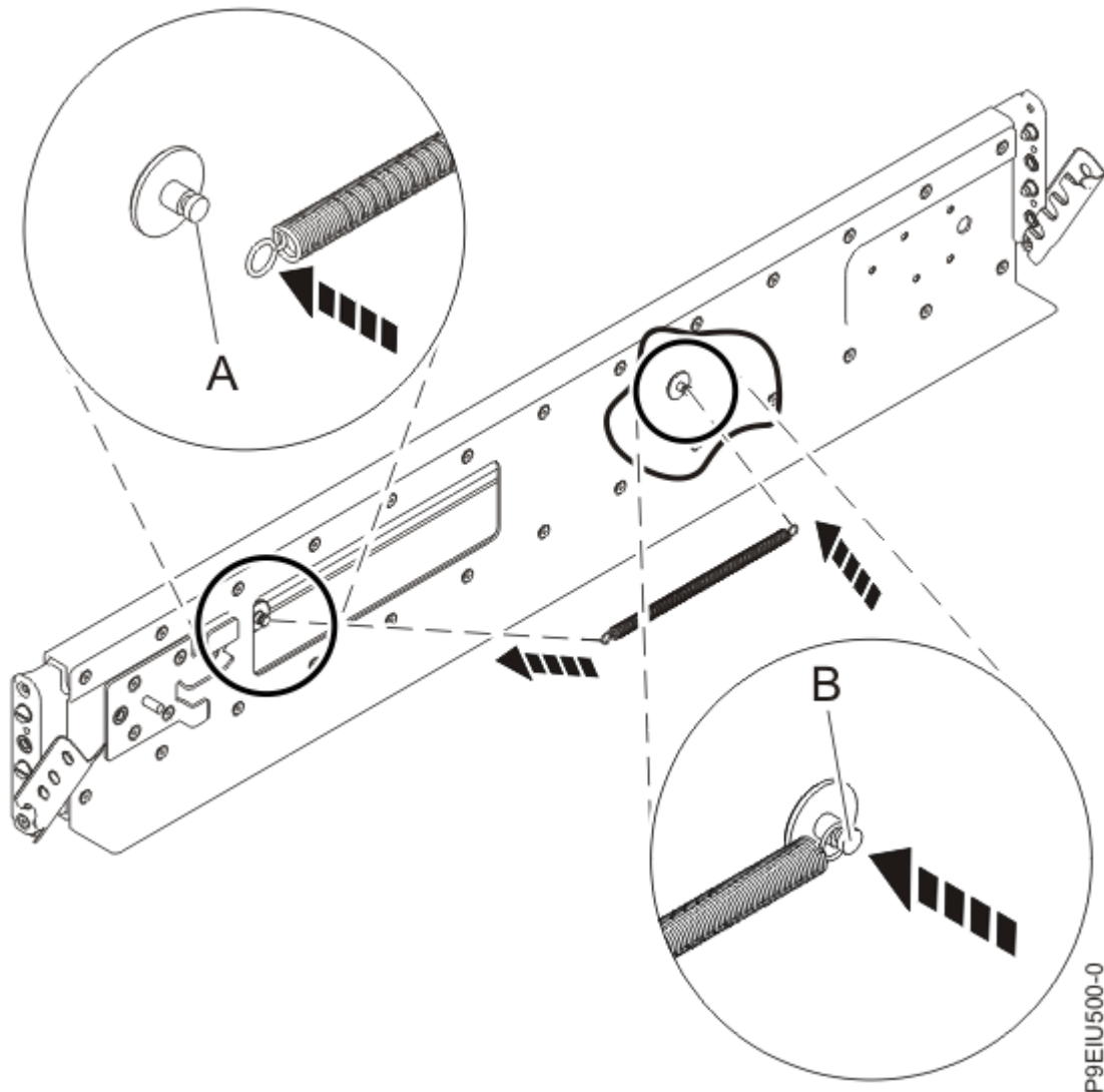
図 3. バネのレールへの取り付け
