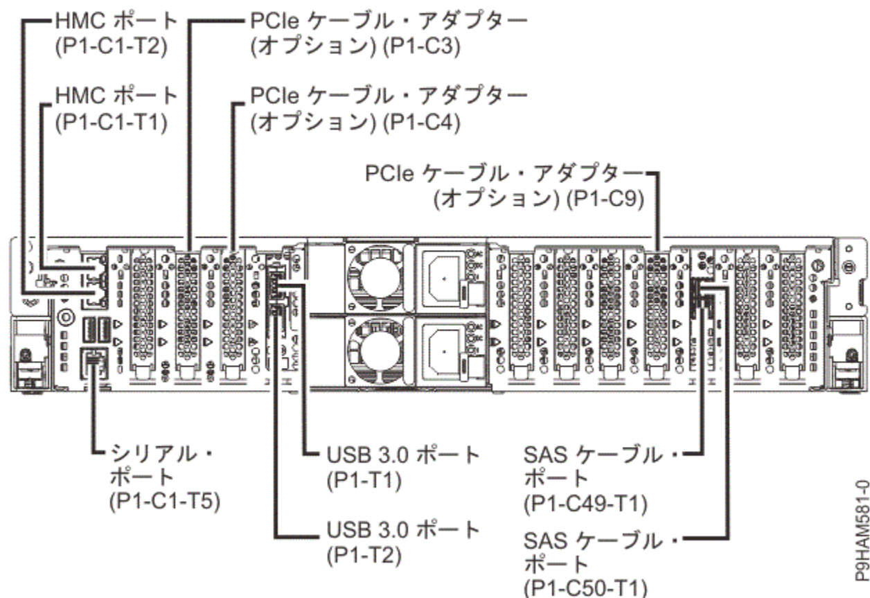
図 31. 5105-22E、9008-22L、9009-22A、9009-22G、および 9223-22H システムのコネクター位置
