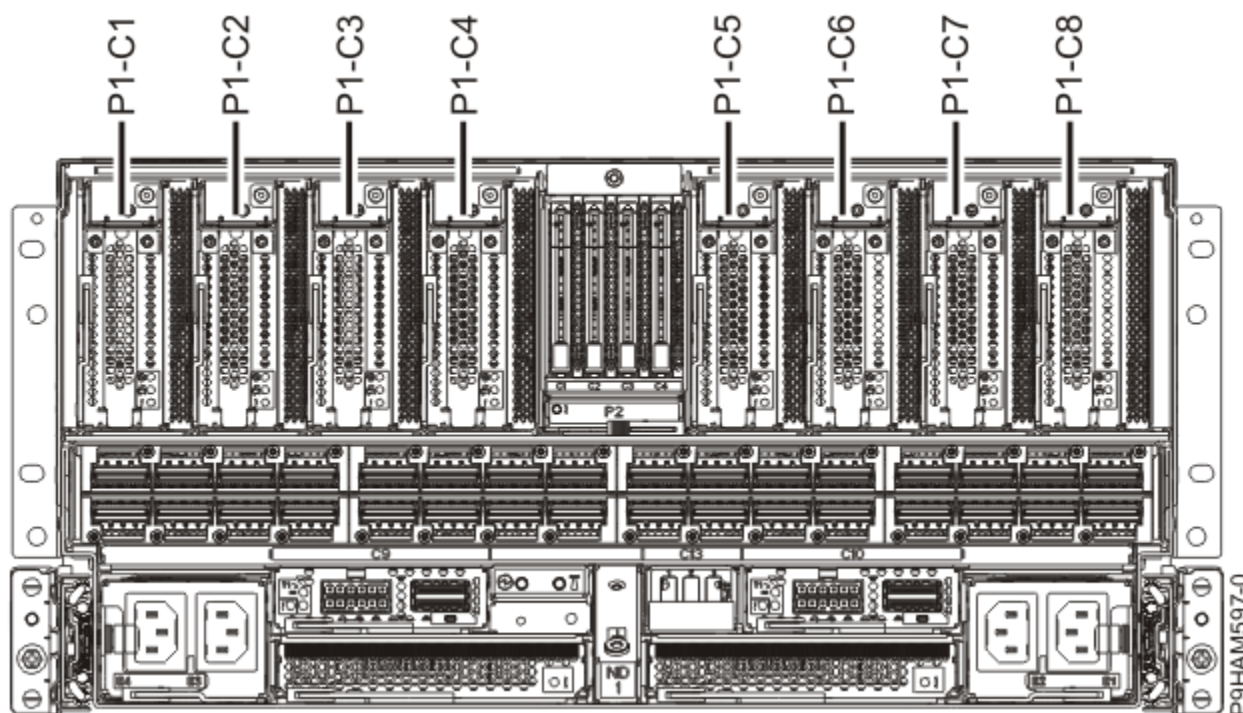
図 34. 9080-M9S システムの背面図
