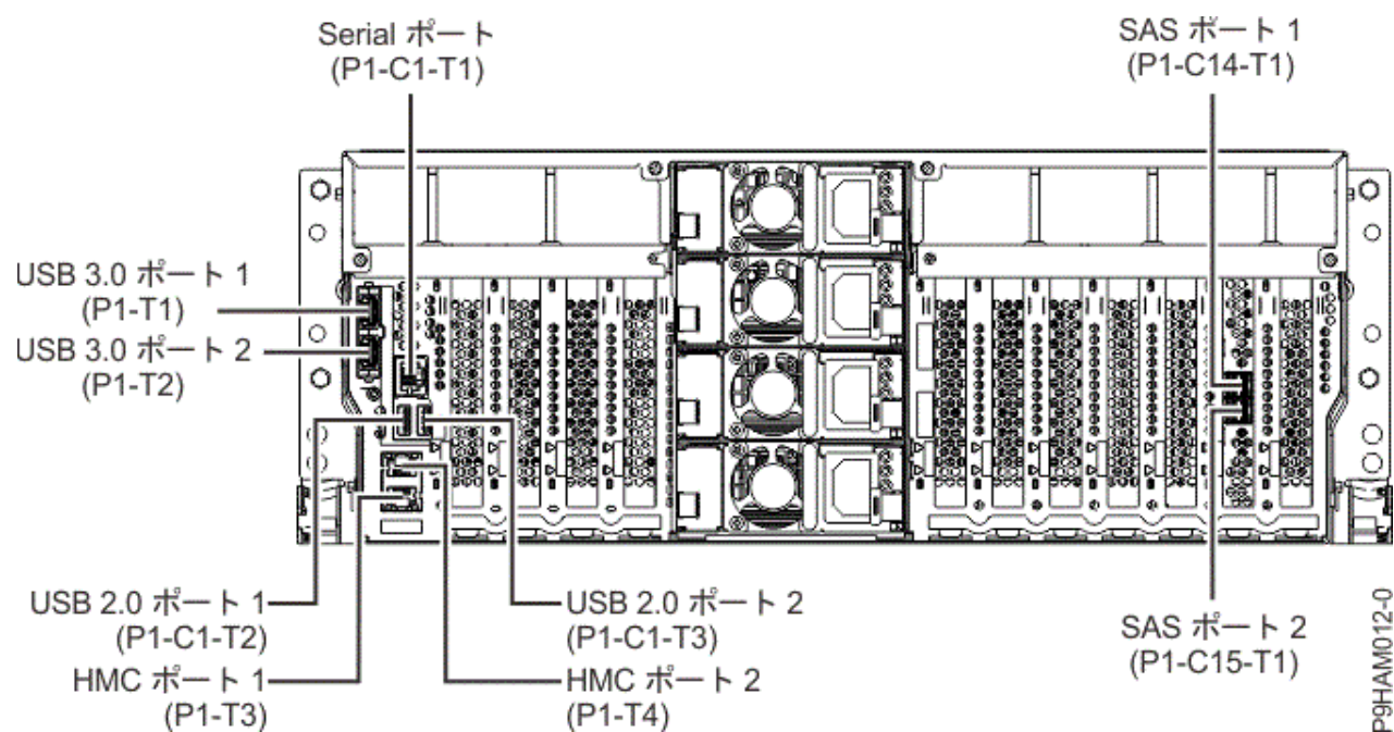
図 36. ラック・マウント型 8286-41A (拡張機能) システムのコネクター位置
