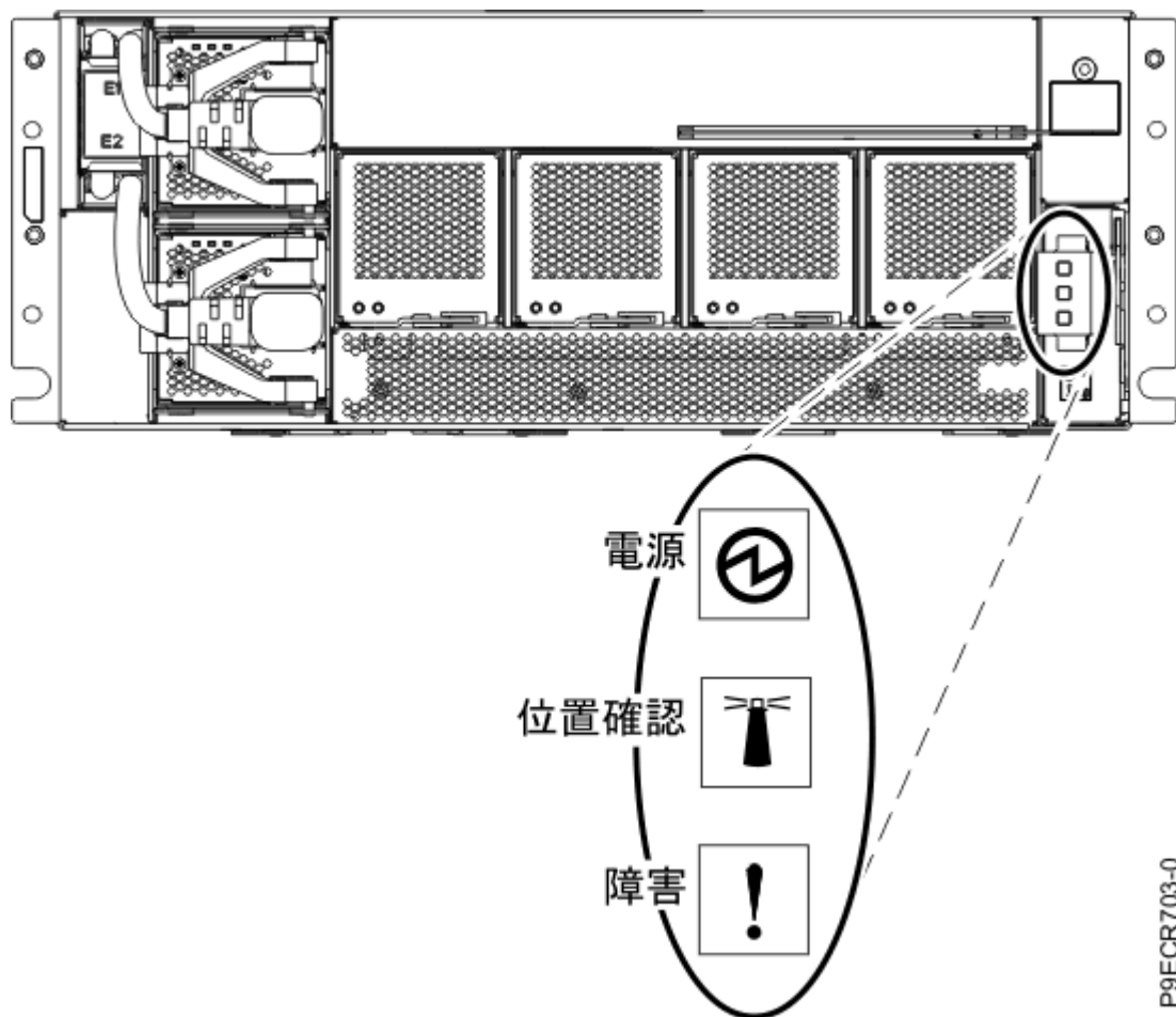
図 7. EMX0 PCIe3 拡張ドロワーの前面電源表示ライト
