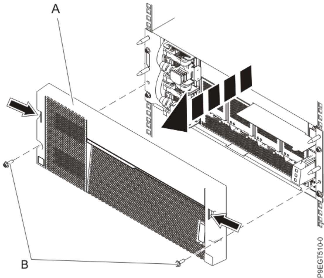
図 1. 前面カバーの取り外し
