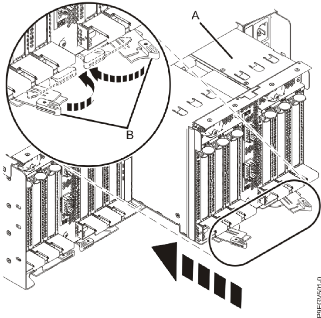
図 7: リリース・ラッチのクローズ
