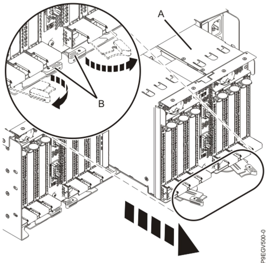
図 4: リリース・ラッチのオープン
