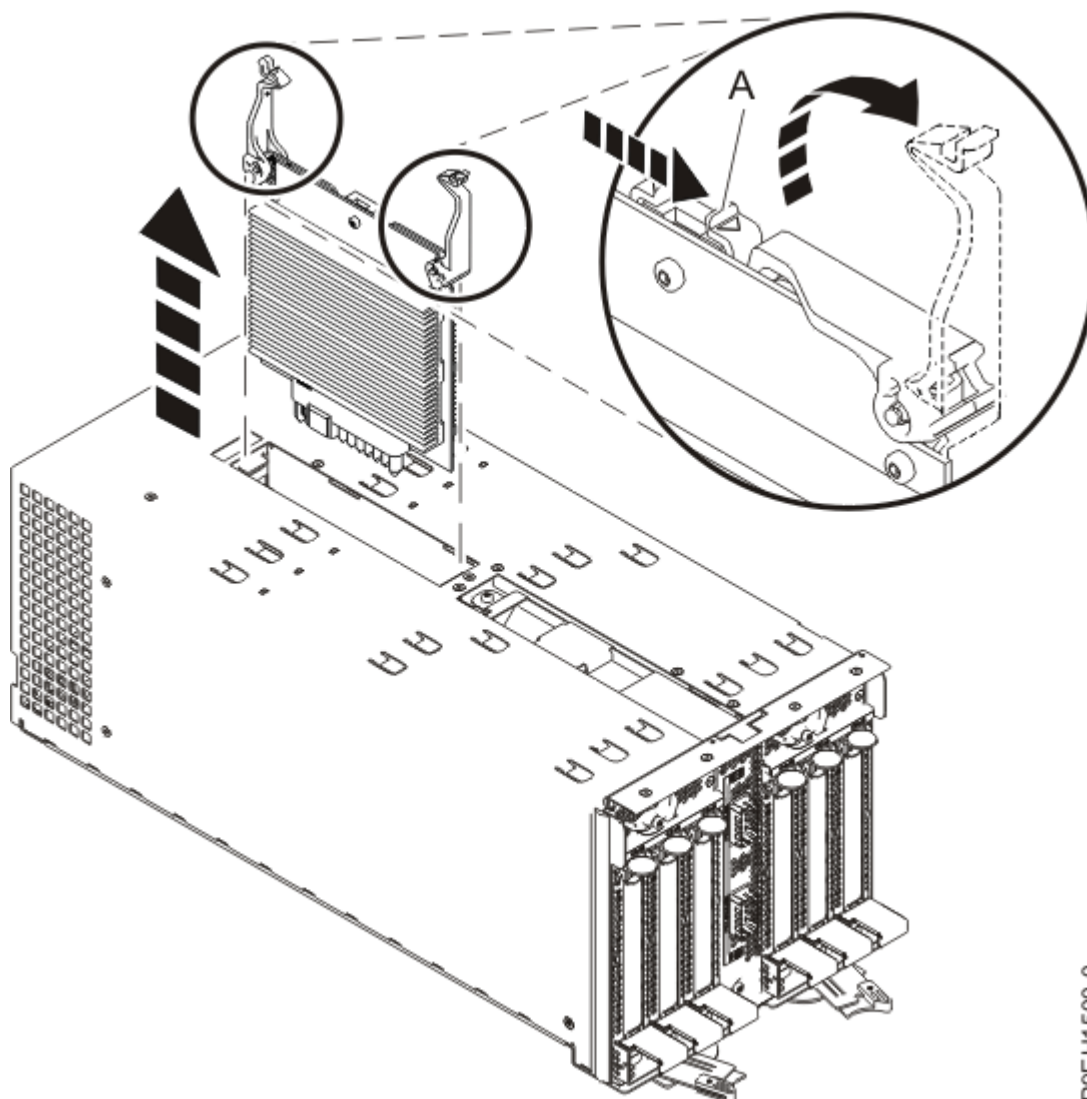
図 5: 電圧調節モジュールの取り外し
