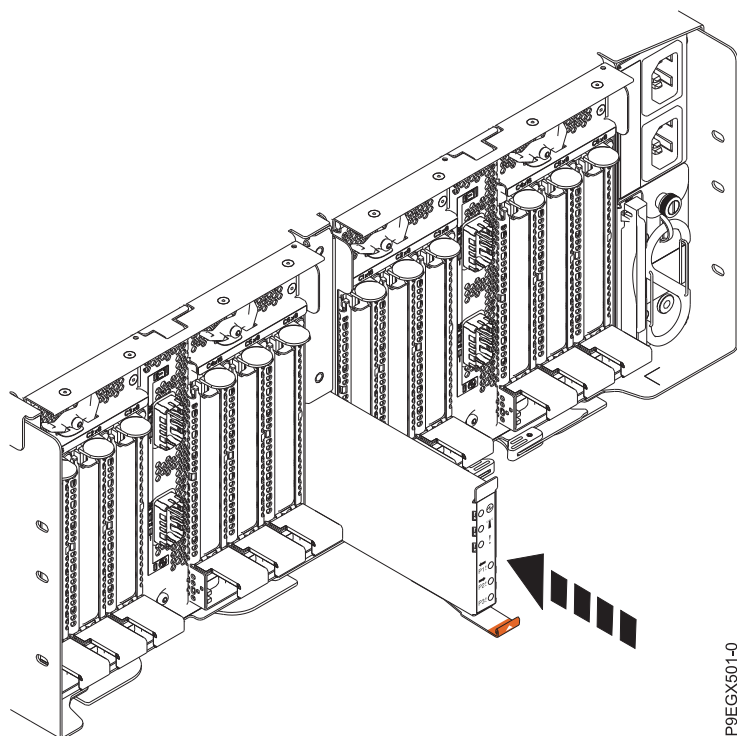
図 4. EMX0 PCIe3 拡張ドロワーでのライト・パイプ・コンジットの再取り付け
