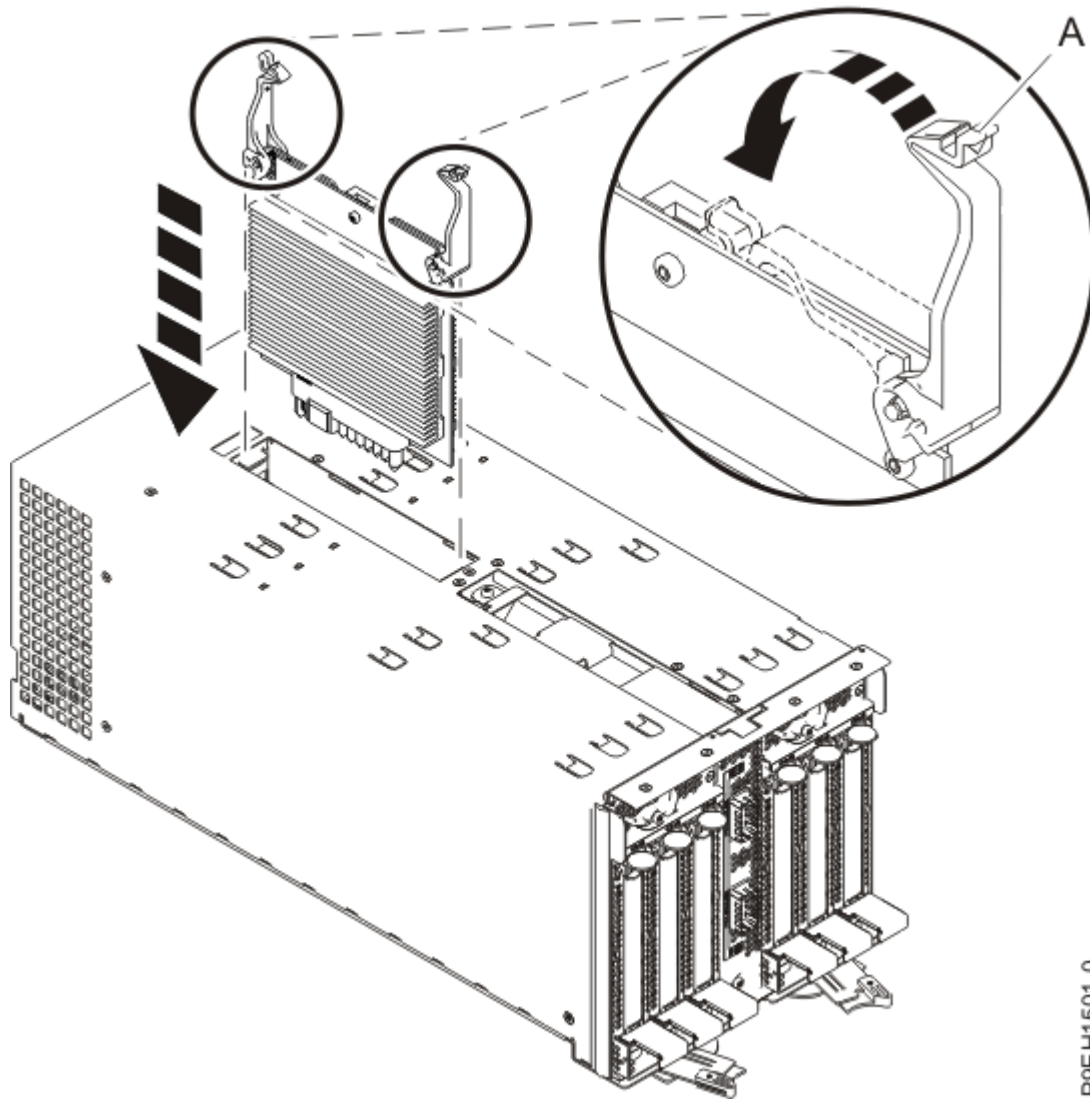
図 14. 電圧調節モジュールの再取り付け
