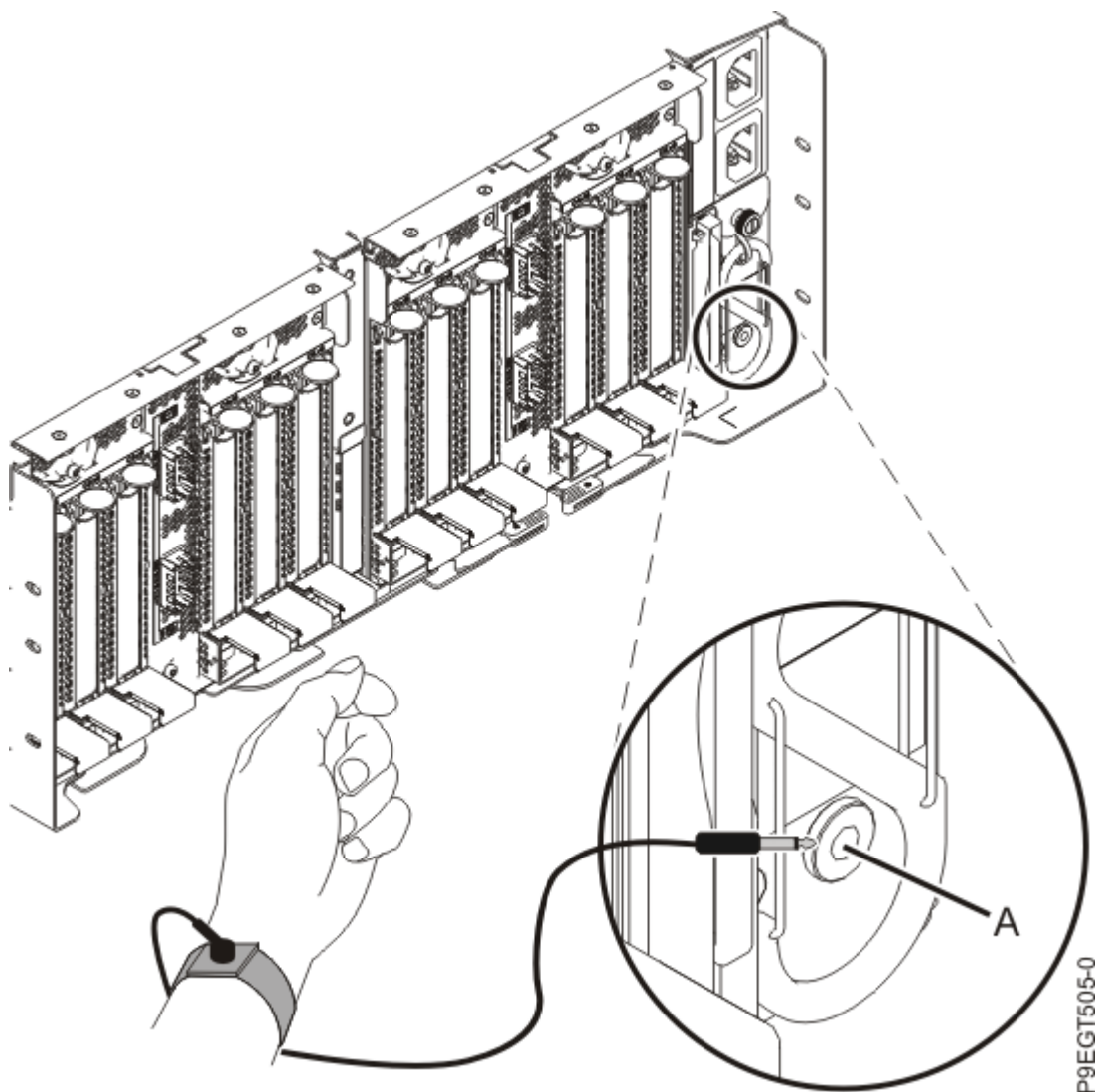
図 8. MX0 PCIe3 拡張ドロワーの背面での ESD ジャックの位置
