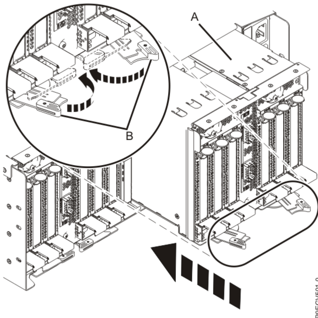
図 4. PCIe3 6 スロット・ファンアウト・モジュールのリリース・ラッチのクローズ
