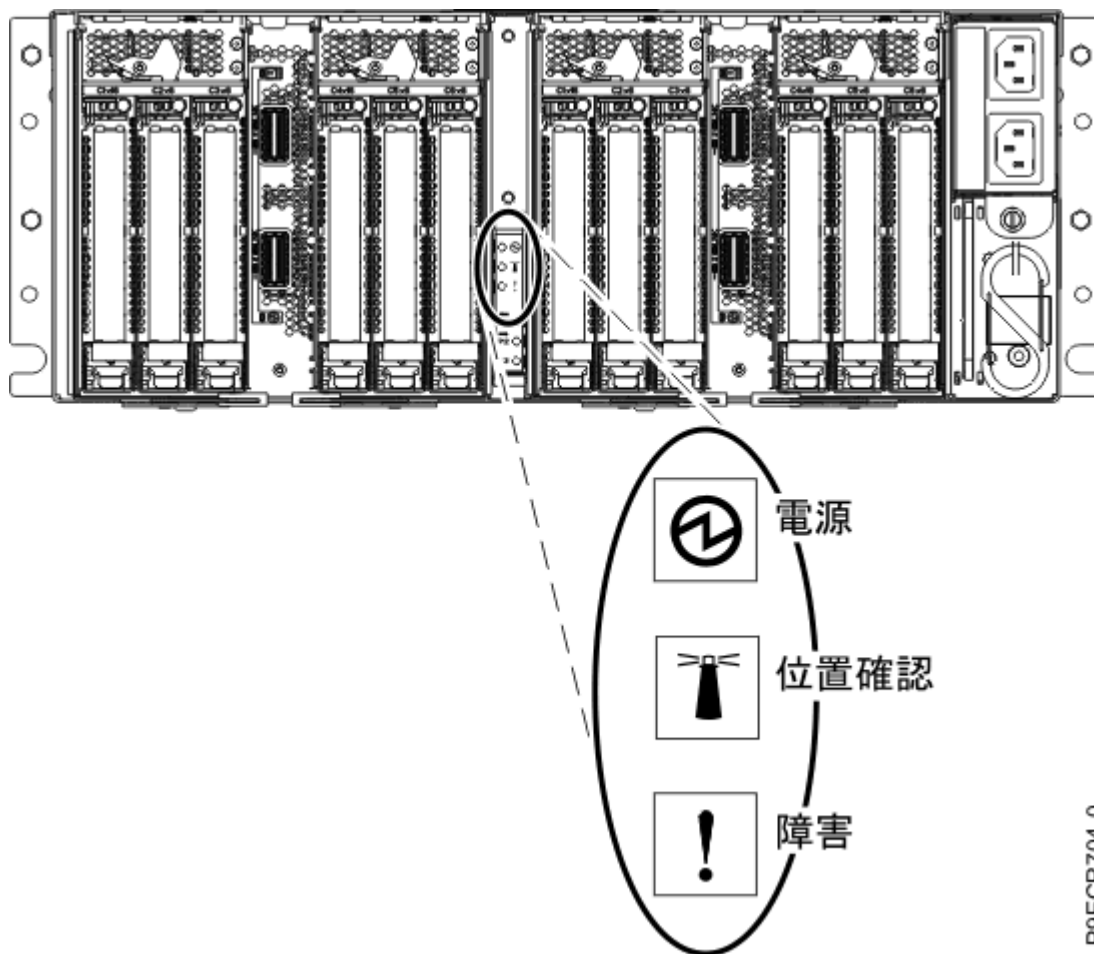
図 24. EMX0 PCIe3 拡張ドロワーの背面電源表示ライト
