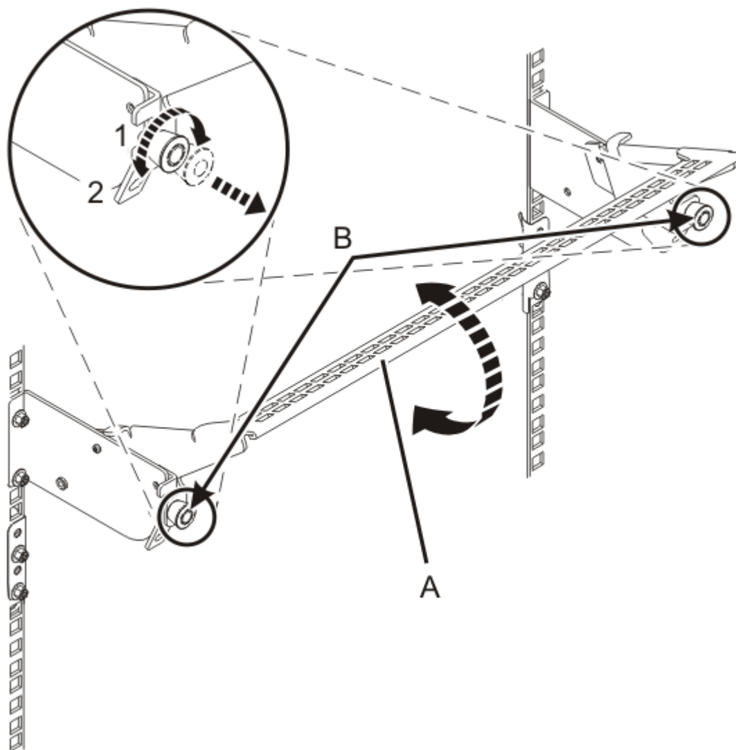
図 6. 下げた操作位置へのケーブル管理ブラケットの設置
