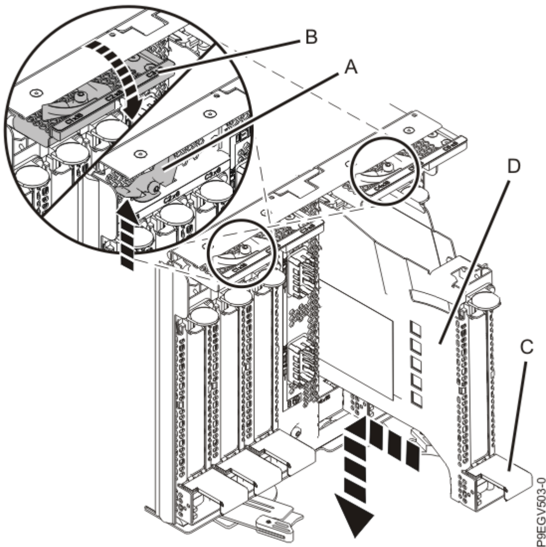
図 13. PCIe アダプター・カセットの取り付け
