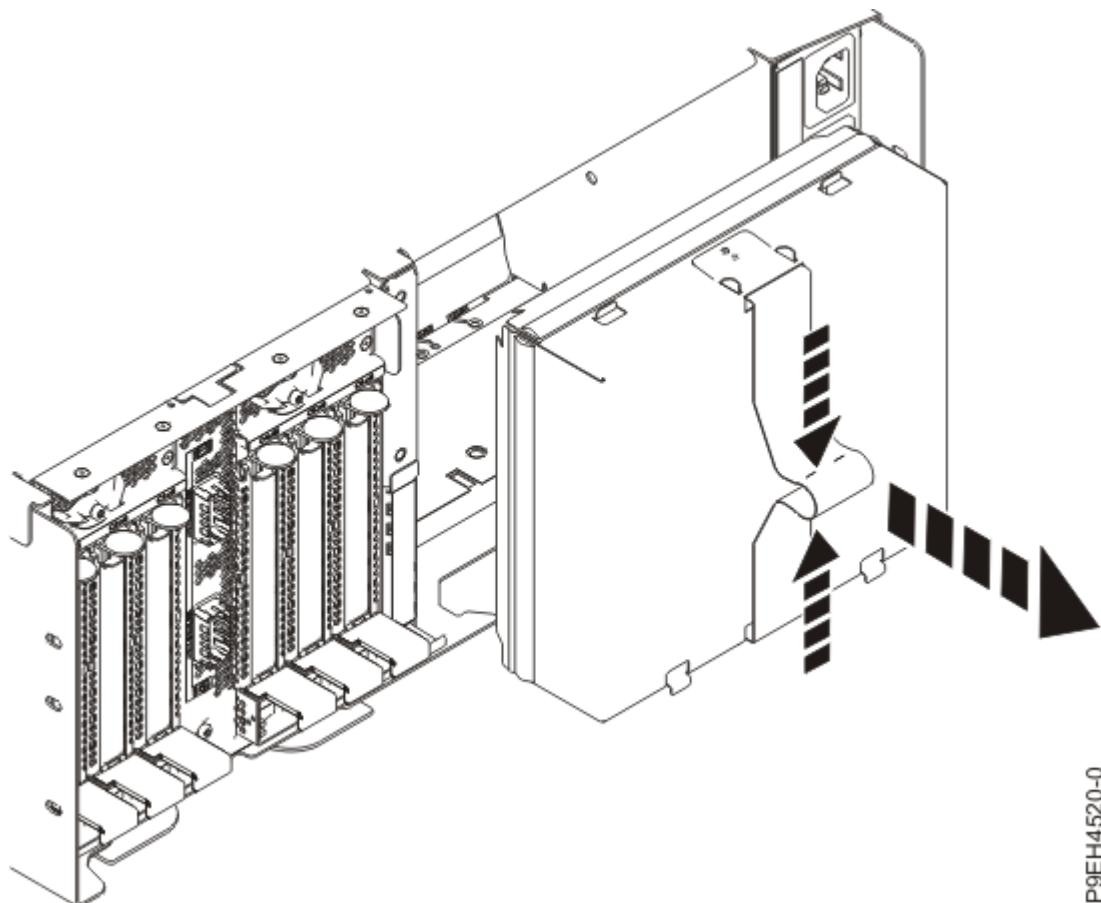
図 3. フィラーの取り外し
