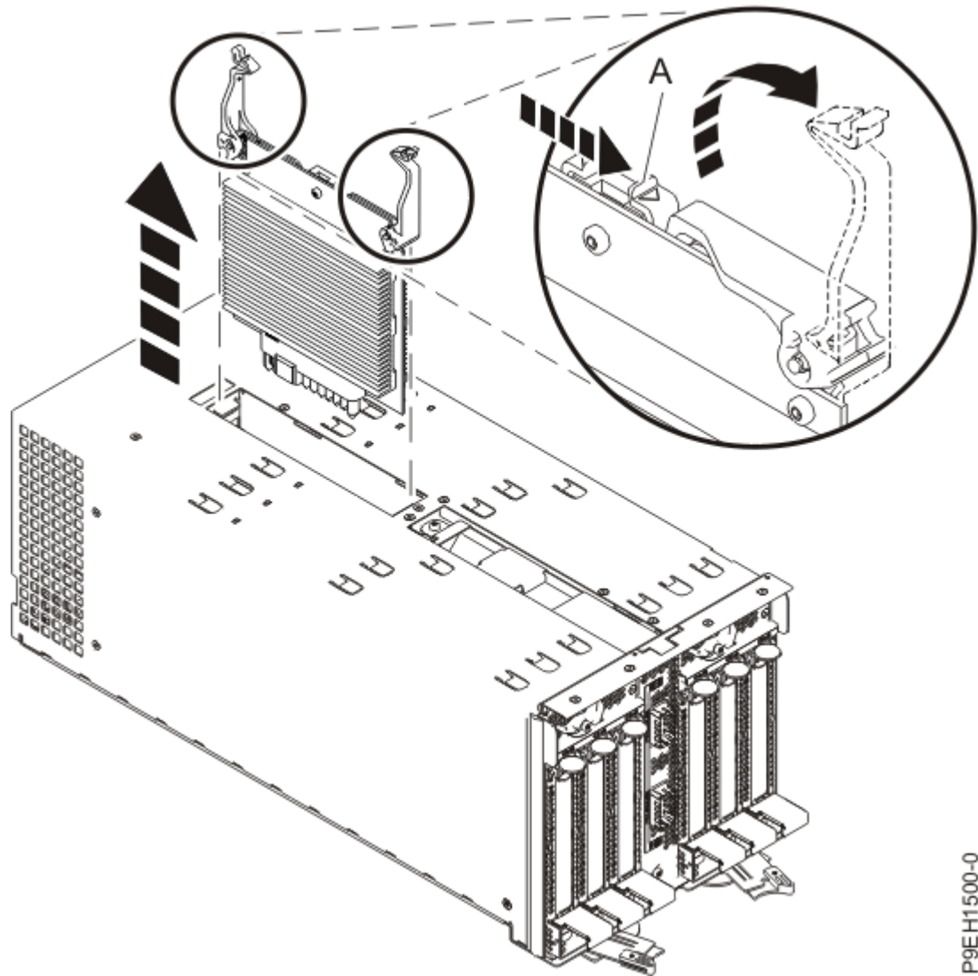
図 11. 電圧調節モジュールの取り外し
