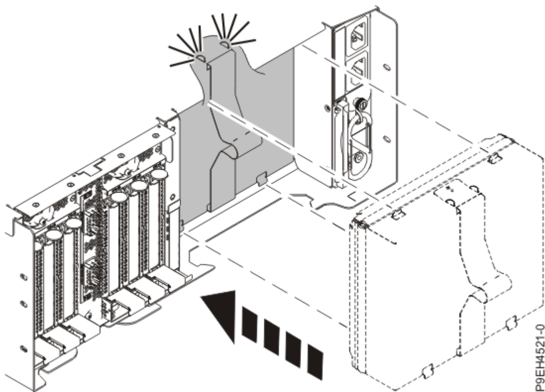
図 21. フィラーの取り付け
