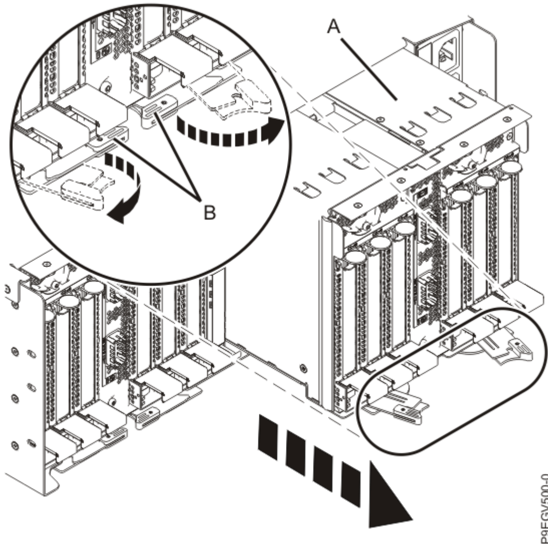
図 10. リリース・ラッチのオープン
