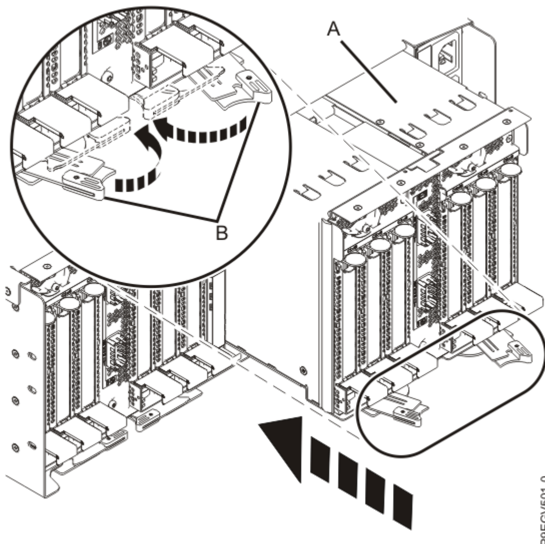
図 15. PCIe3 6 スロット・ファンアウト・モジュールのリリース・ラッチのクローズ
