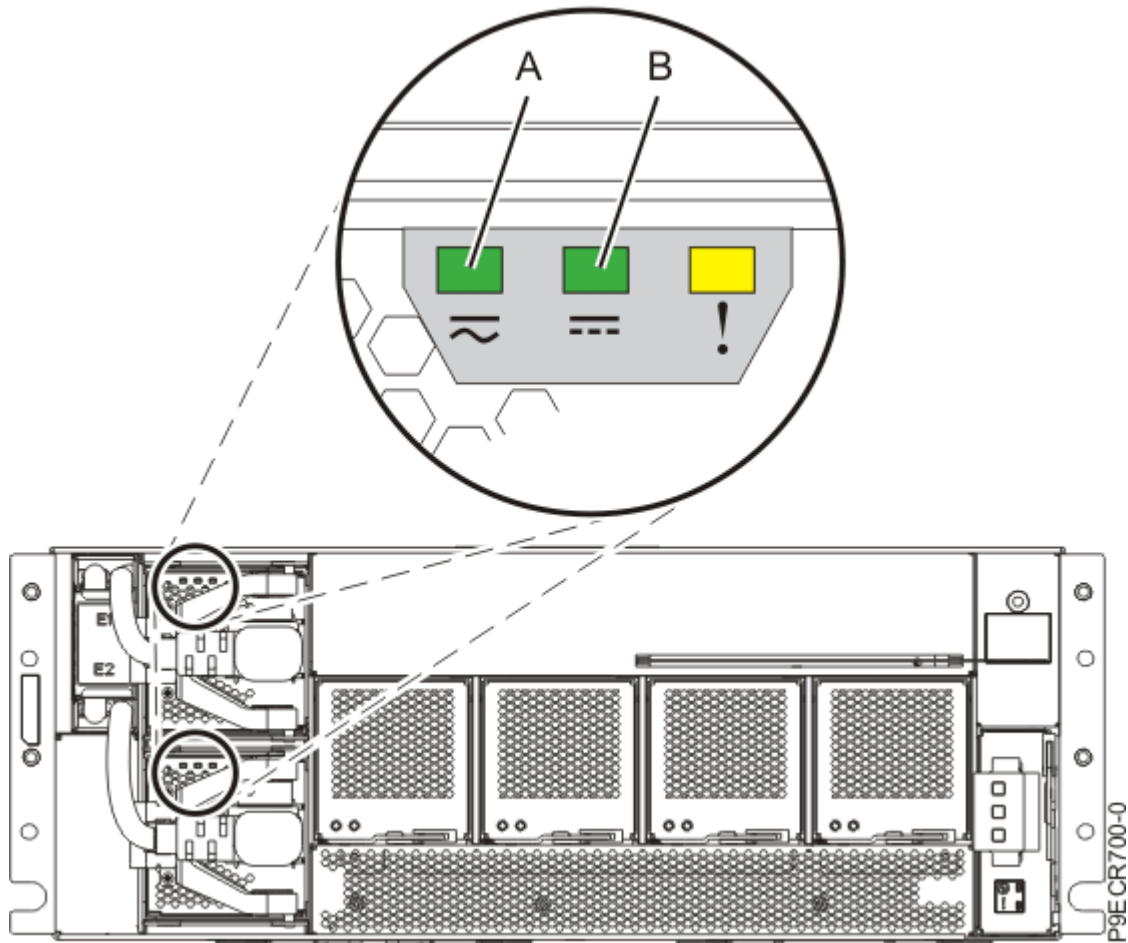
図 7. 電源装置 LED の点灯の確認
