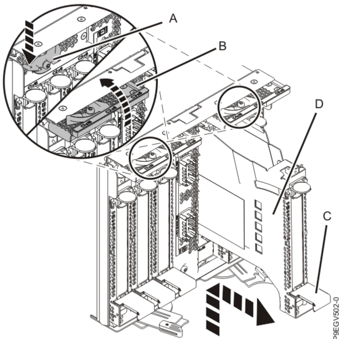
図 12. PCIe アダプター・カセットの取り外し
