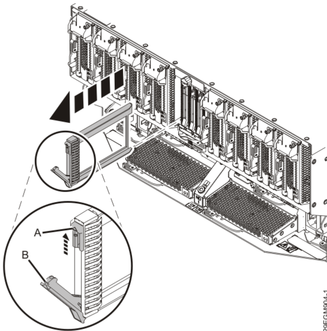
図 6. 9080-M9S システムからの NVMe ドライブ・フィラーの取り外し
