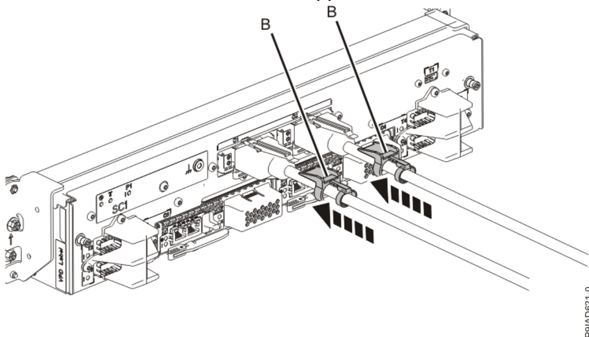
図 10. システム・コントロール・ユニットへの UPIC ケーブルの再取り付け
