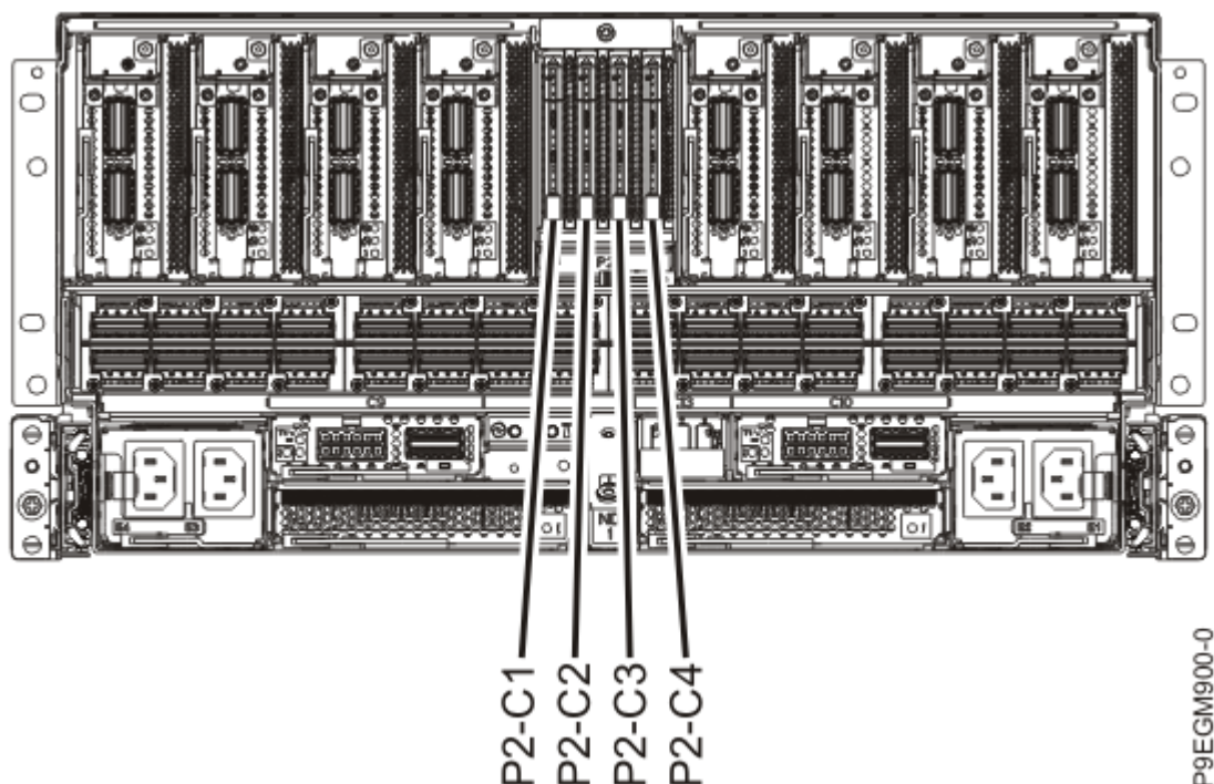
図 1. 9080-M9S システムの NVMe U.2 ドライブの位置
