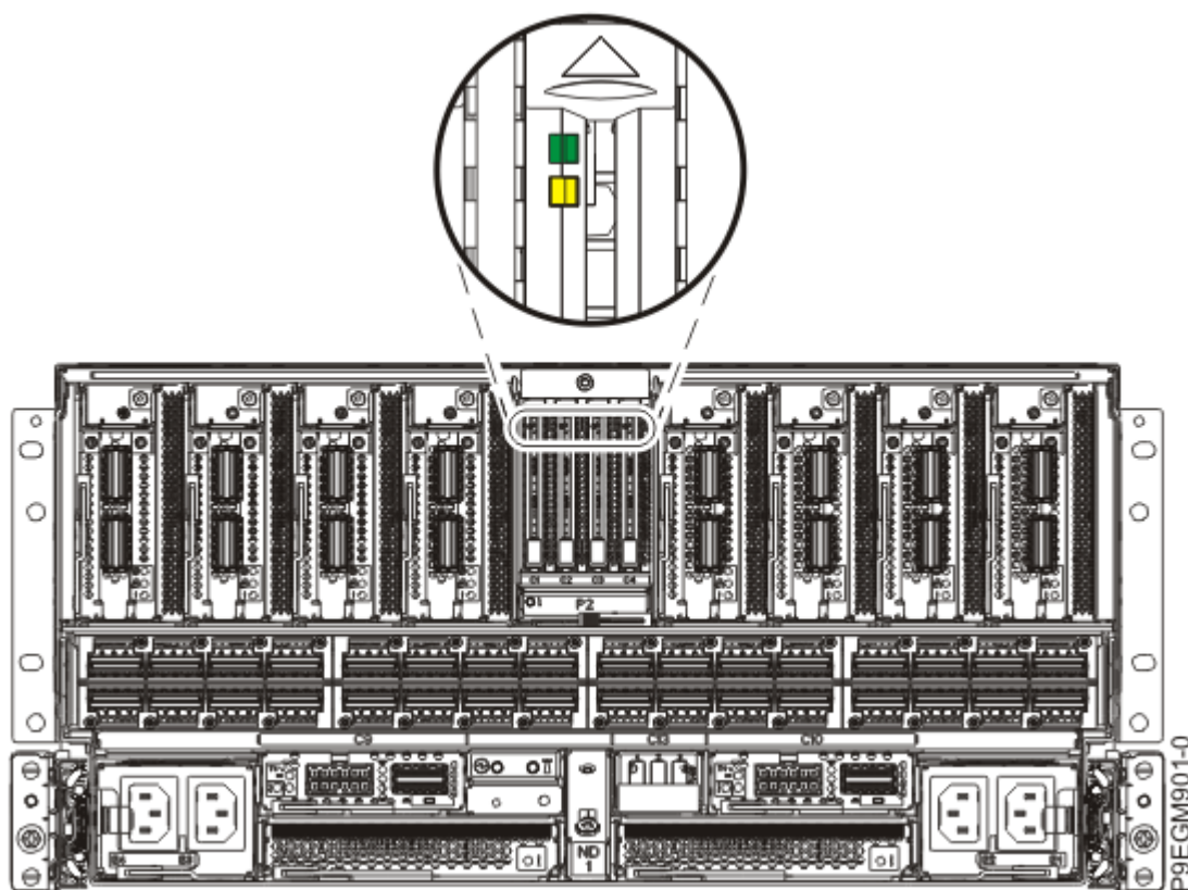
図 2. 9080-M9S システムの NVMe U.2 LED の位置
