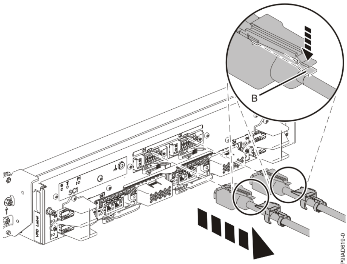
図 4. システム・コントロール・ユニットからの UPIC ケーブルの取り外し
