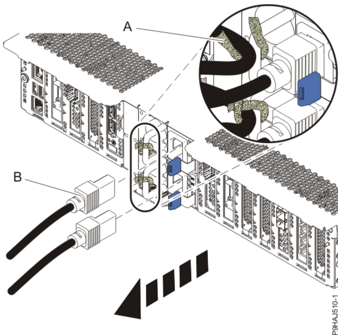
図 10. 電源コードの取り外し
