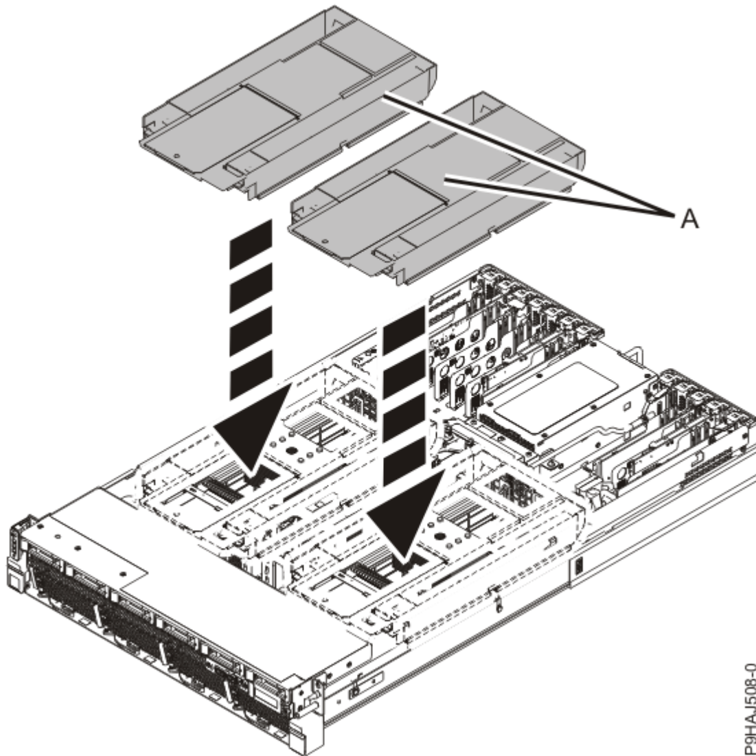
図 24. エア・バッフルの取り替え
