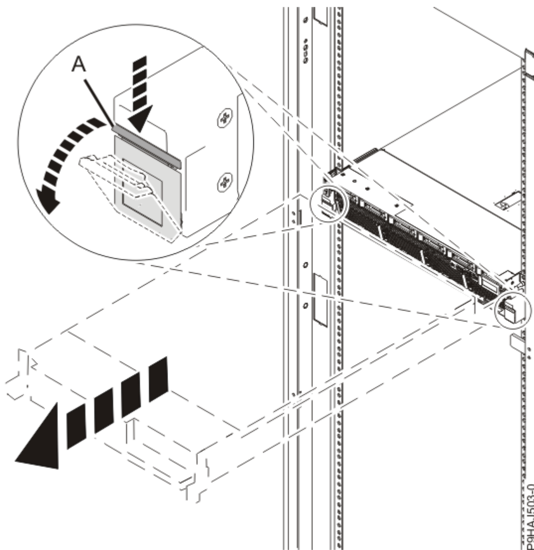
図 17. サイド・ラッチのリリース
