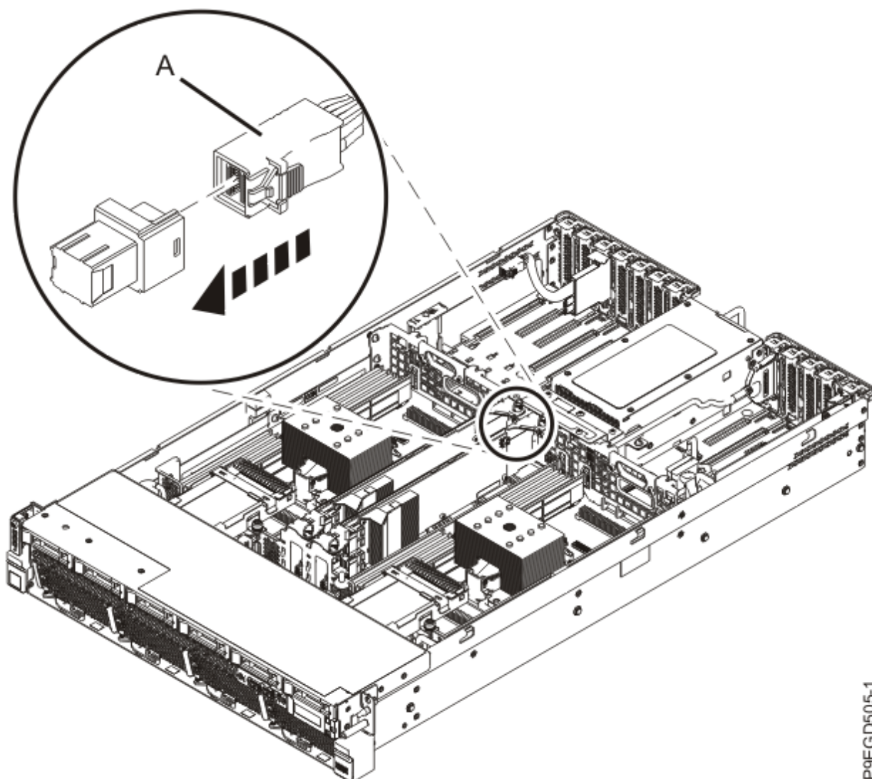
図 9. 背面 SAS ケーブルの再接続
