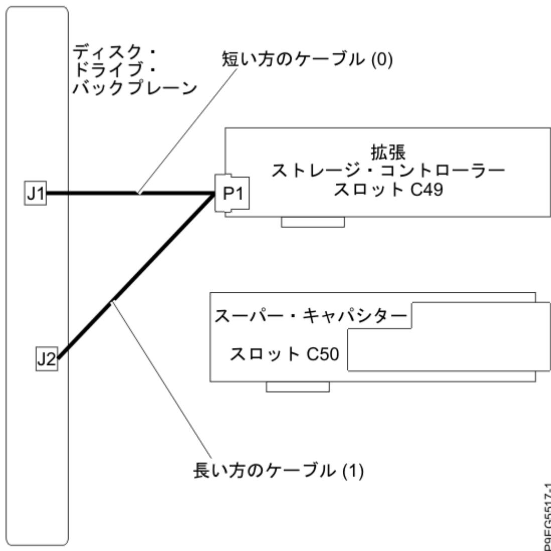
図 7. ハイパフォーマンス・ストレージ・コントローラ構成での「Y」 SAS ケーブルの再接続
