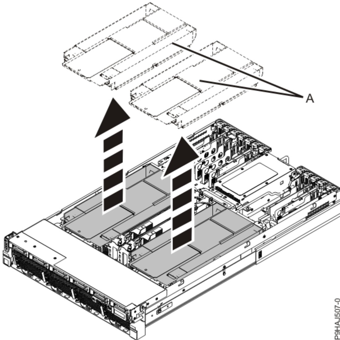
図 19. エア・バッフルの取り外し
