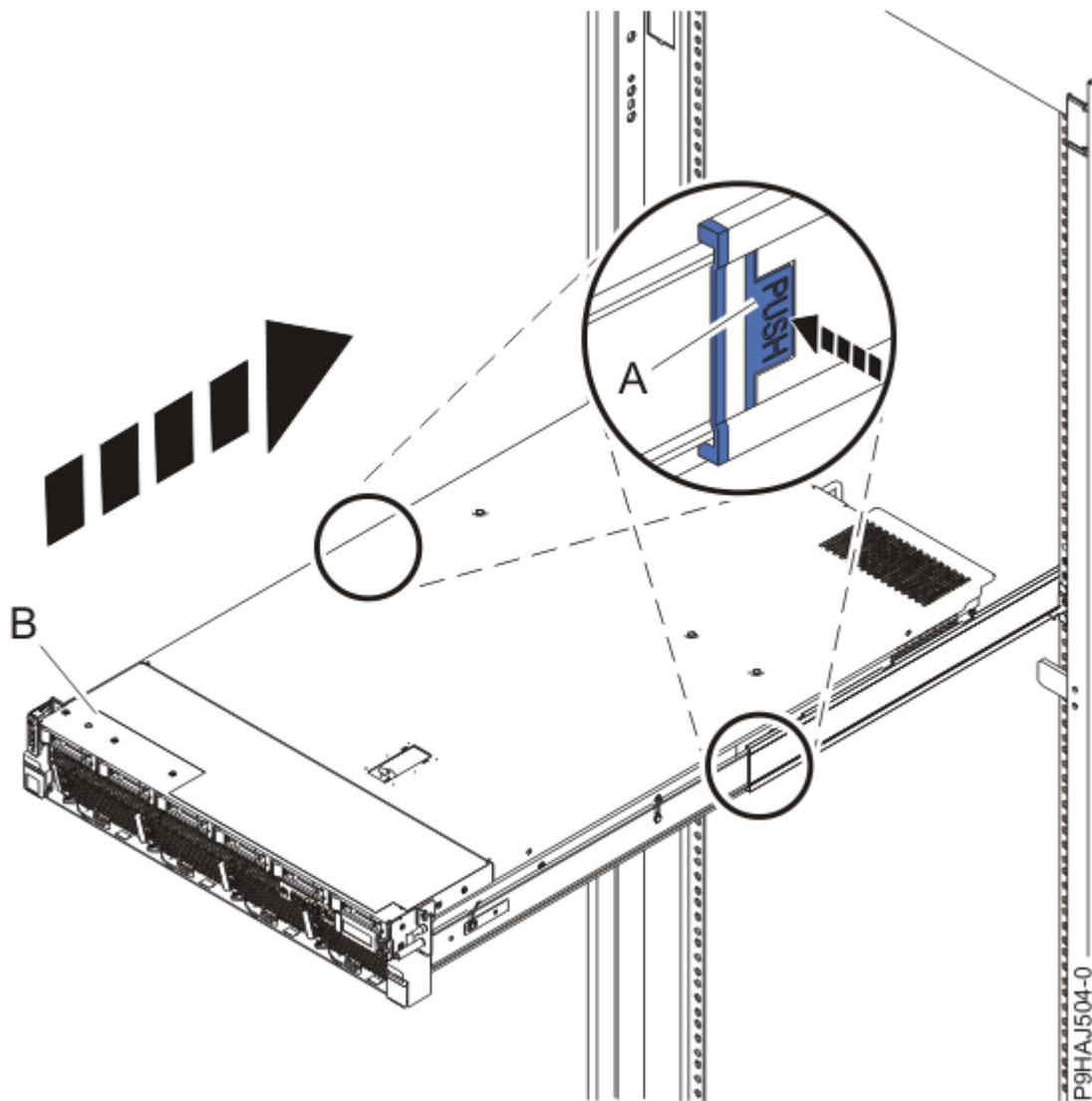
図 32. システムの操作位置への設置
