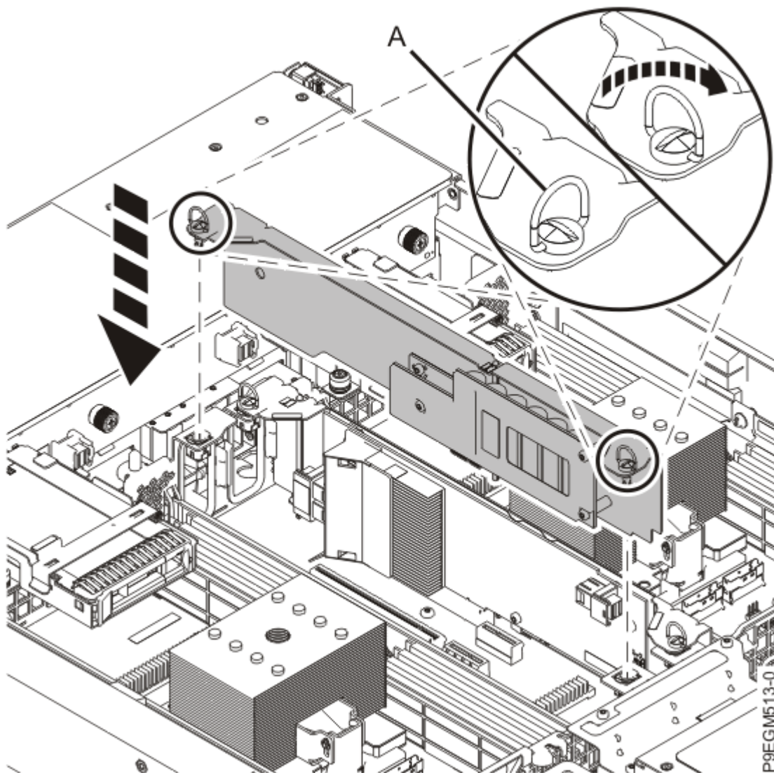
図 29. バックアップ電源モジュールの取り付け
