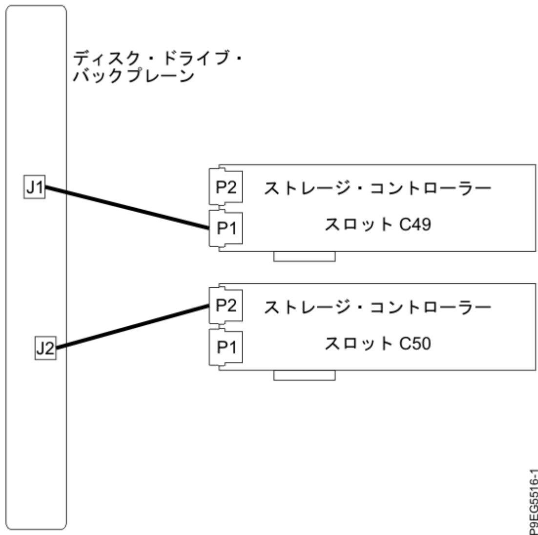
図 6. 分割ディスク構成での SAS ケーブルの再接続
