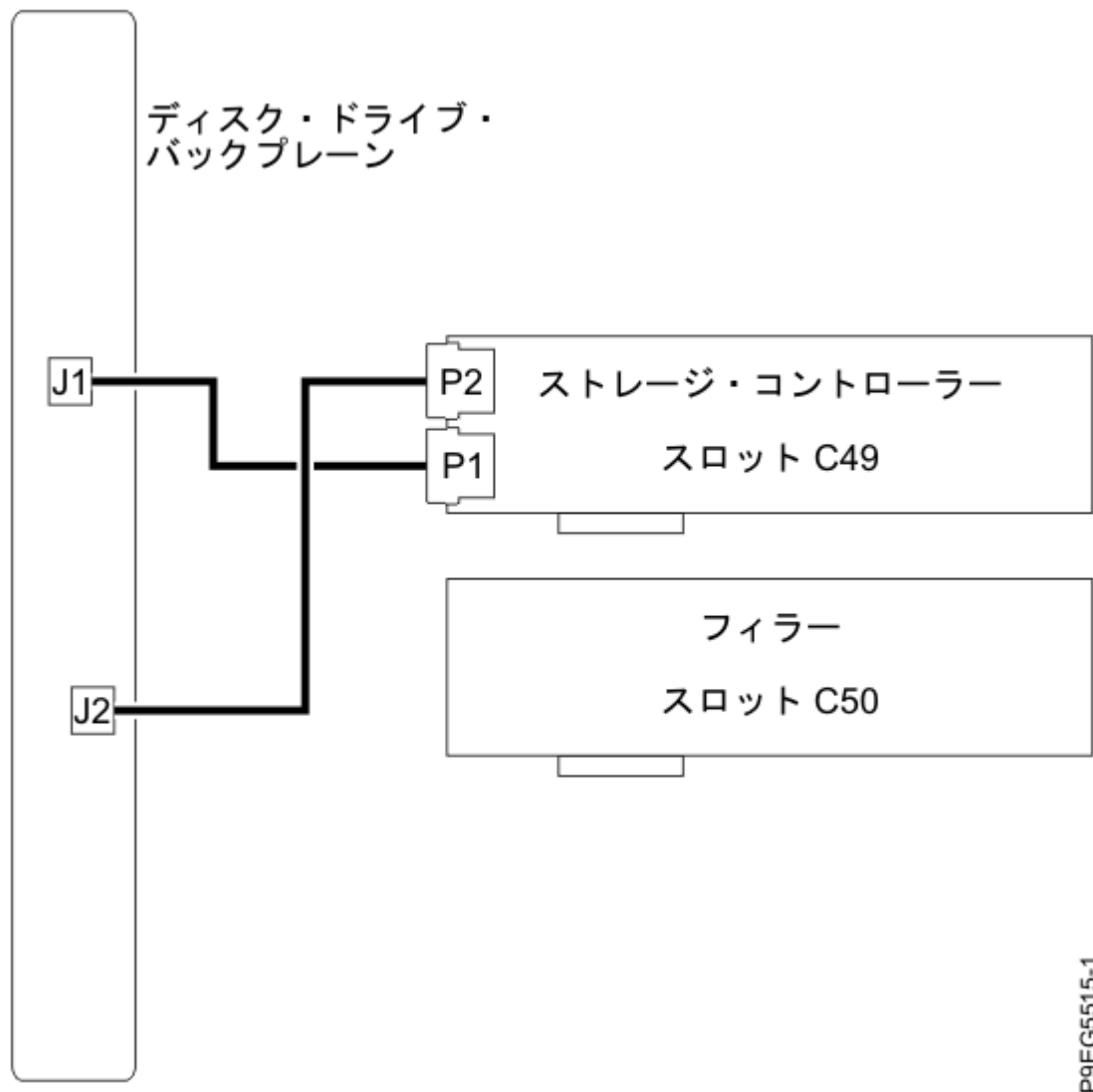
図 5. 基本ストレージ構成での SAS ケーブルの再接続
