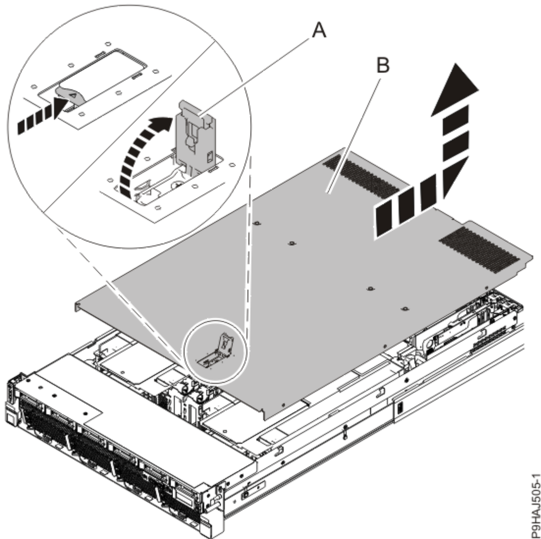
図 18. 保守アクセス・カバーの取り外し
