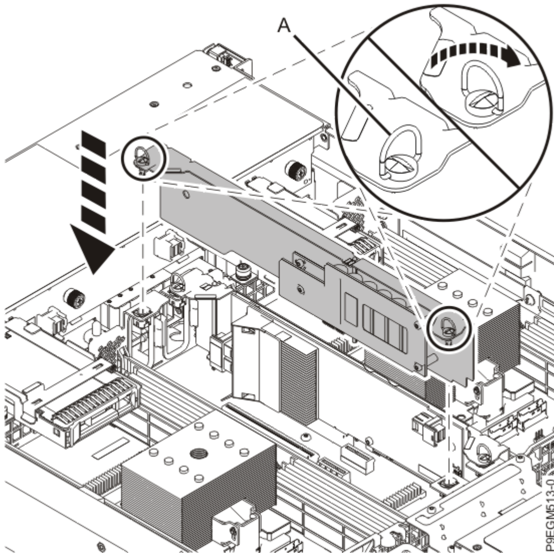
図 11. バックアップ電源モジュールの取り付け
