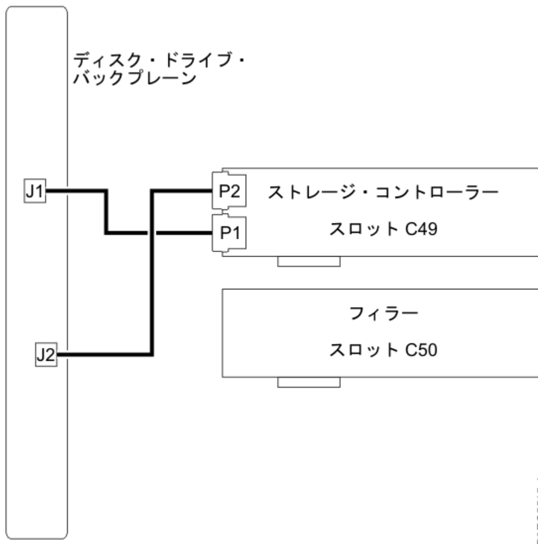
図 24. 基本ストレージ構成での SAS ケーブルの再接続
