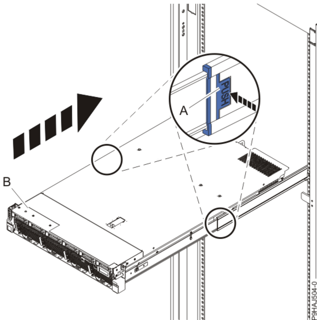
図 14. システムの操作位置への設置
