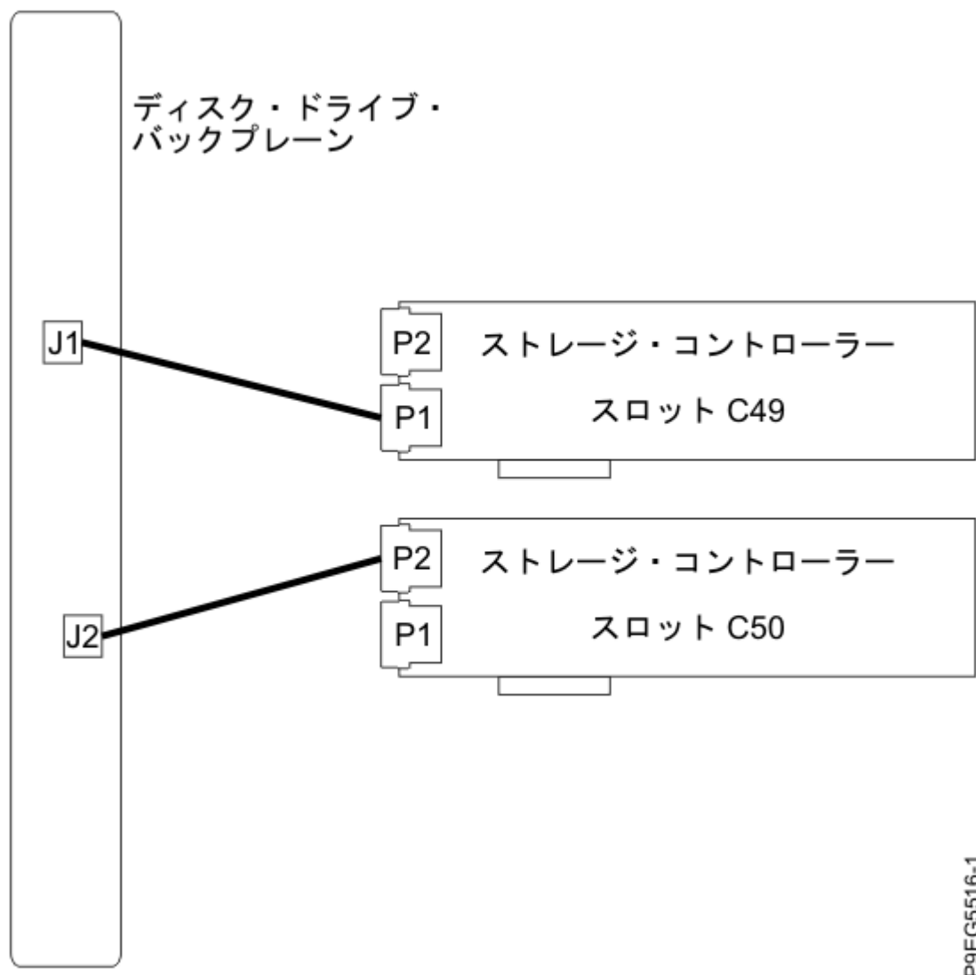
図 25. 分割ディスク構成での SAS ケーブルの再接続
