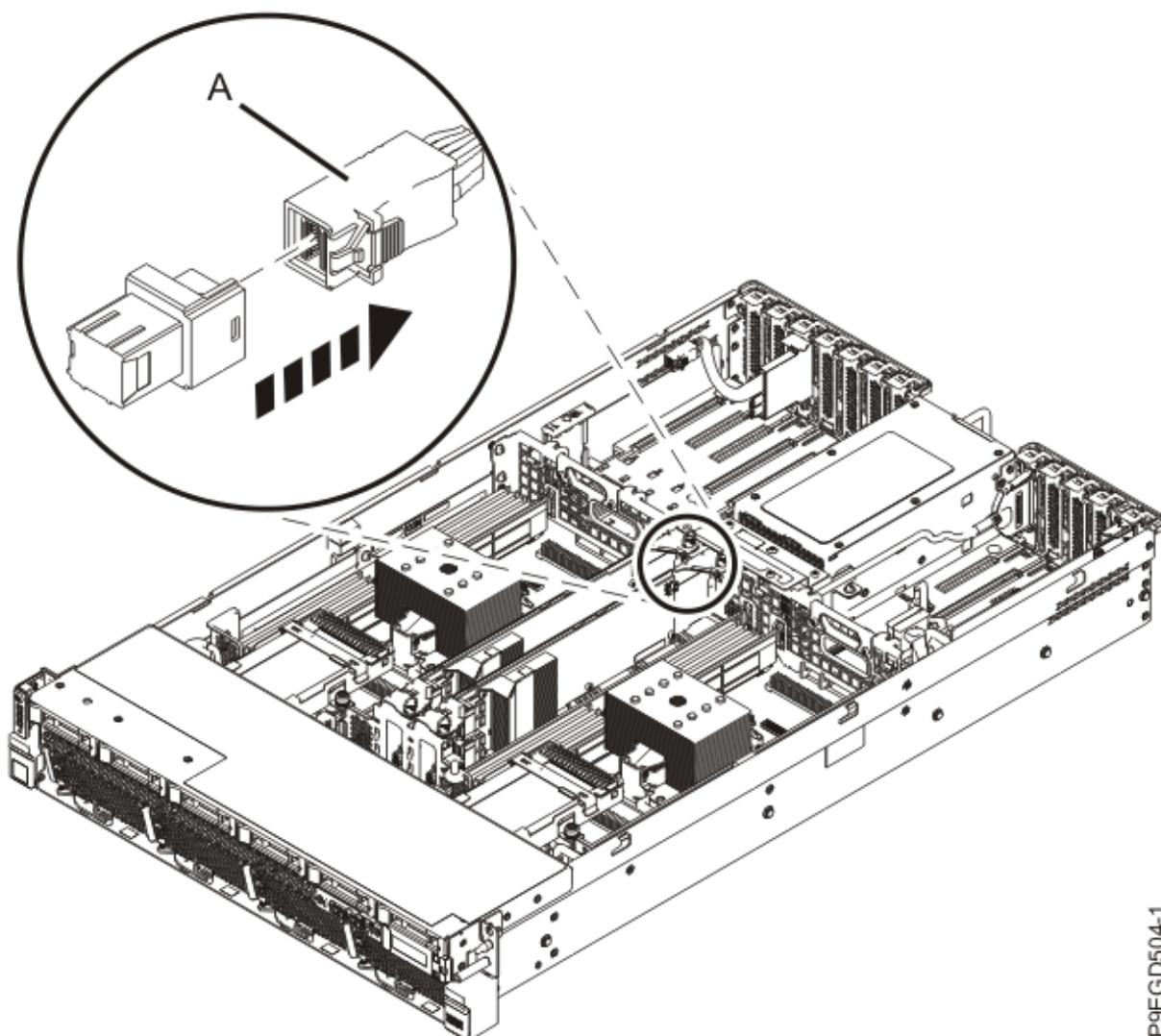
図 21. SAS RAID 内部アダプターからの背面 SAS ケーブルの切り離し
