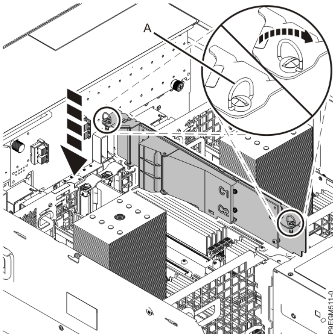
図 35. NVMe M.2 キャリア・カードの装着
