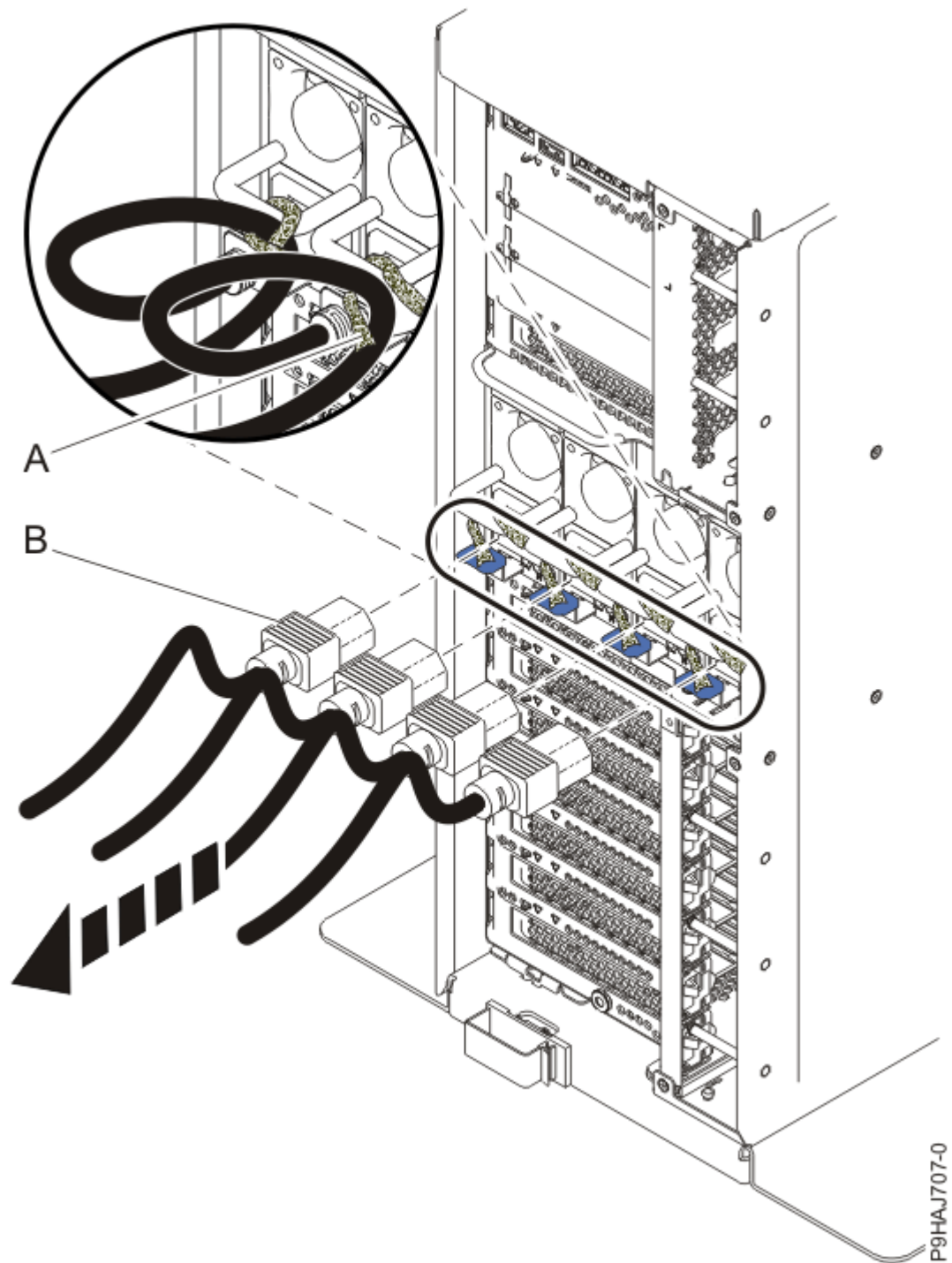
図 24. スタンドアロン型サーバーからの電源コードの取り外し
