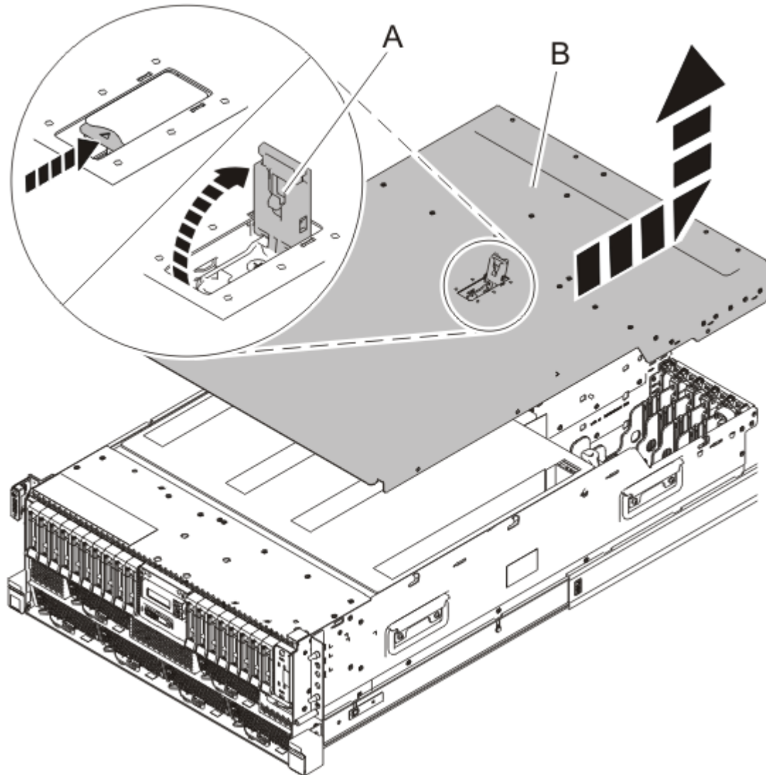
図 26. ラック・マウント型システムからの保守アクセス・カバーの取り外し
