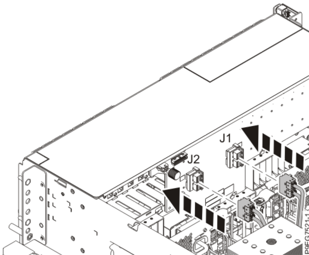
図 14. 基本機能ディスク・ドライブ・バックプレーンの前面 SAS ケーブルの再接続
