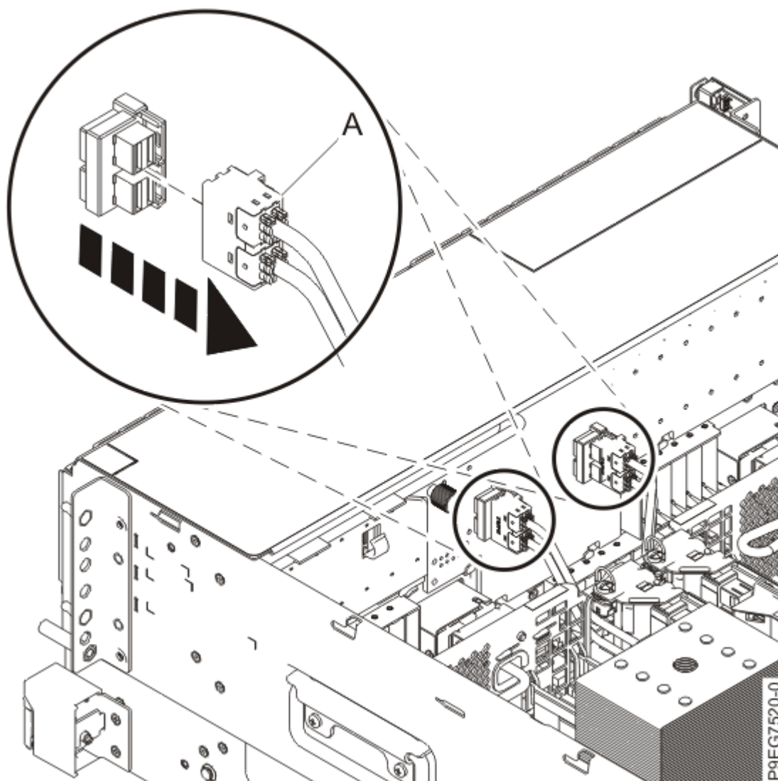
図 30. 前面 SAS ケーブルのプラグを抜く
