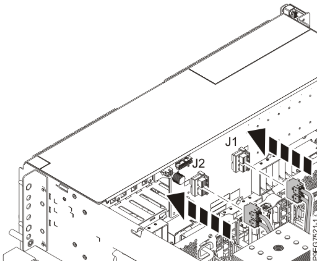
図 39. 基本機能ディスク・ドライブ・バックプレーンの前面 SAS ケーブルの再接続
