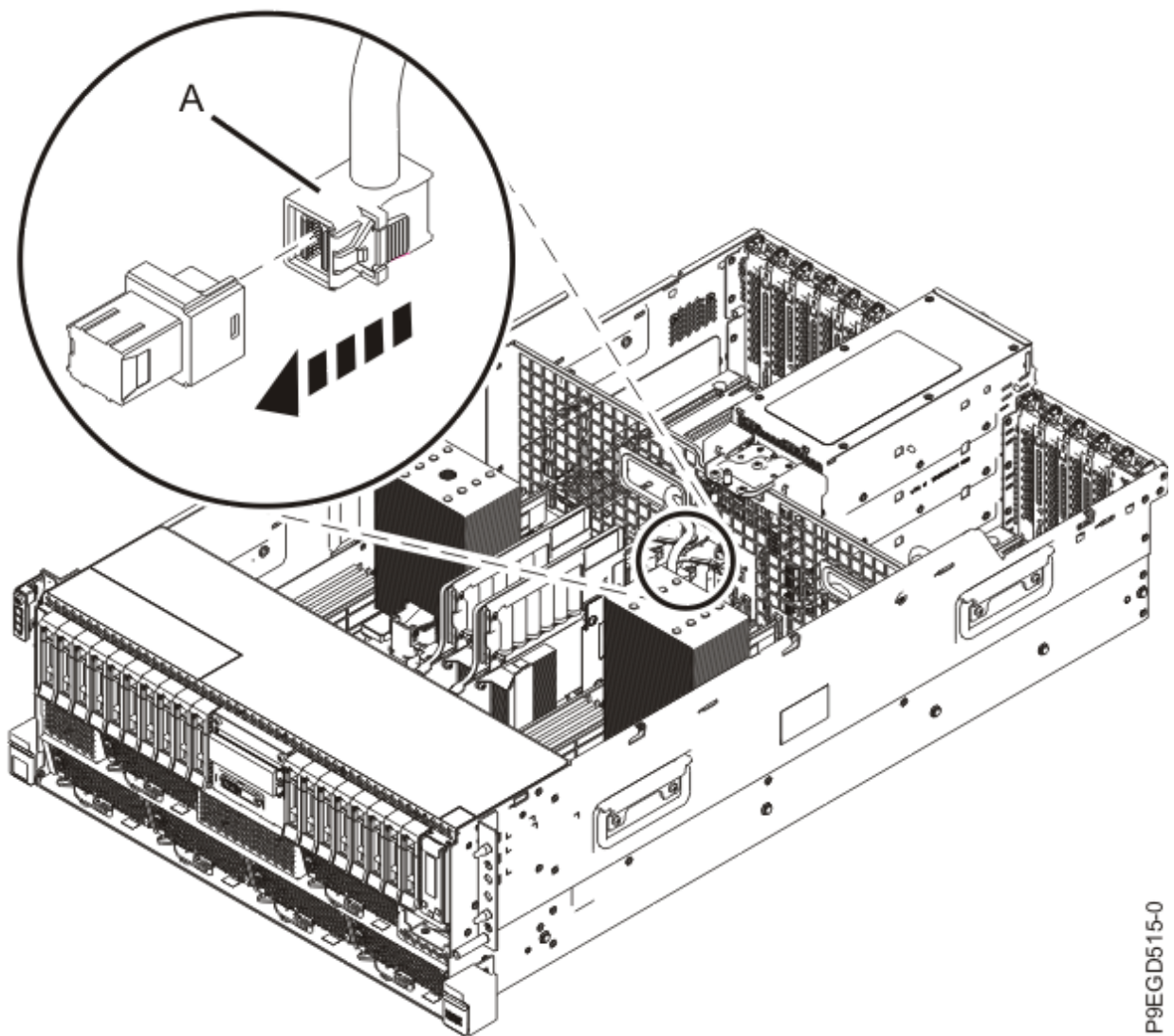
図 13. 背面 SAS ケーブルの再接続
