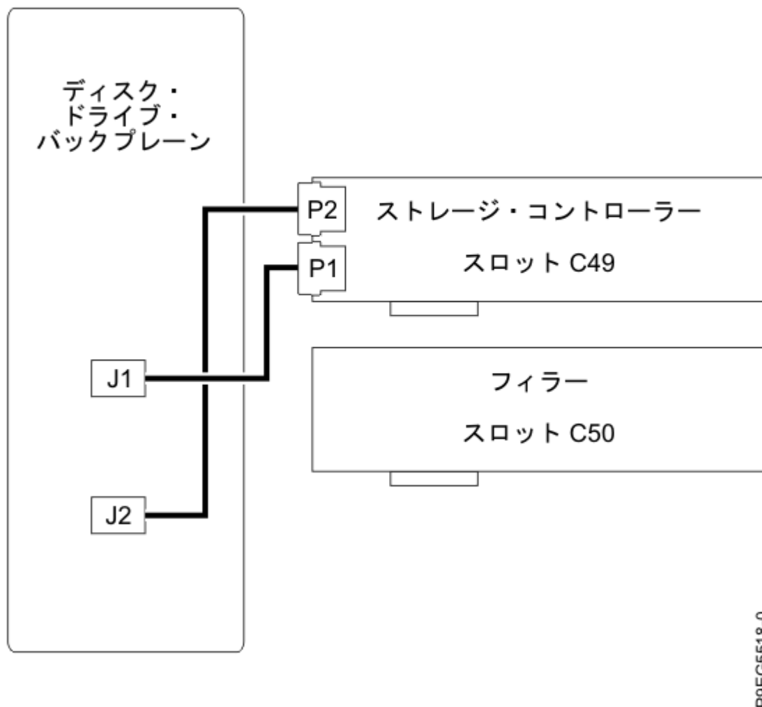
図 8. 基本ストレージ構成での SAS ケーブルの再接続
