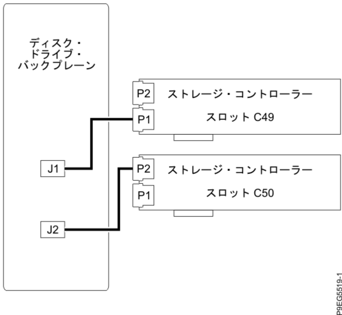
図 34. 分割ディスク構成での SAS ケーブルの再接続
