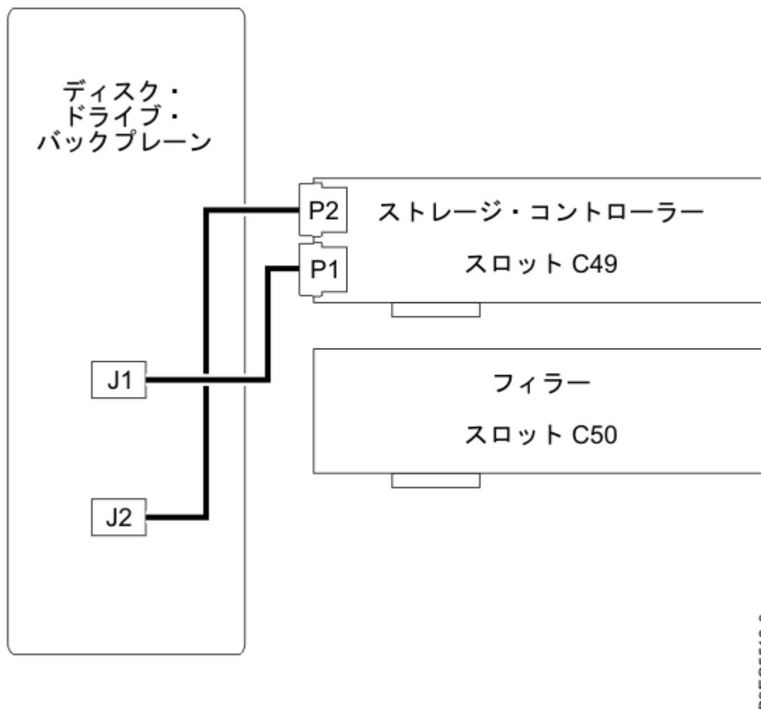
図 33. 基本ストレージ構成での SAS ケーブルの再接続
