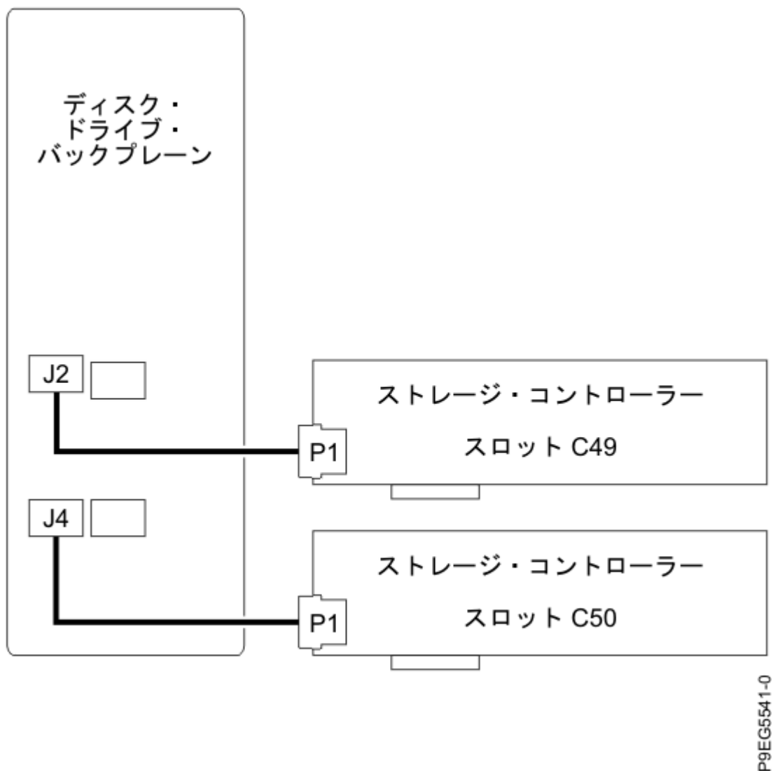
図 36. 18 ドライブ拡張機能 構成での SAS ケーブルの再接続
