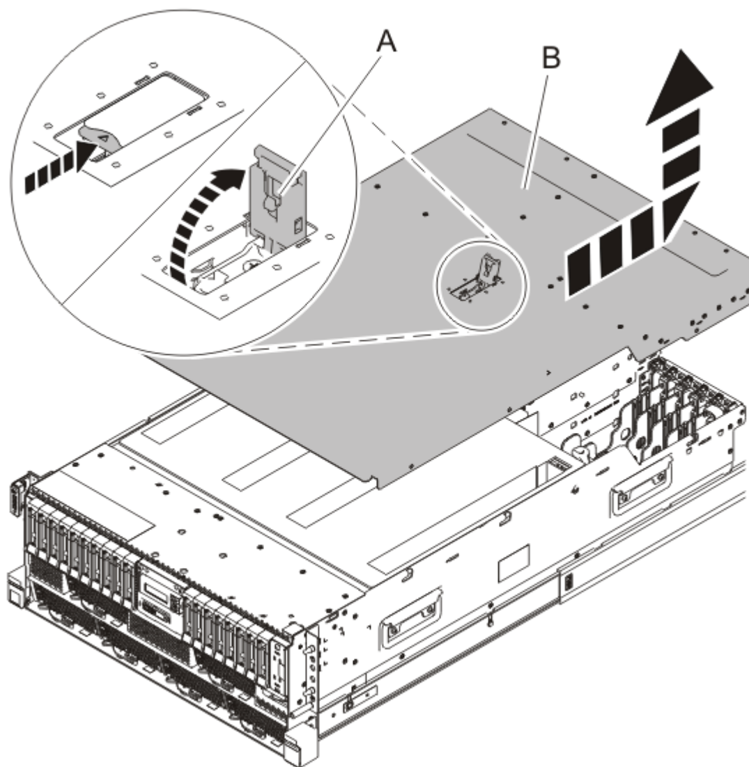
図 4. ラック・マウント型システムからの保守アクセス・カバーの取り外し
