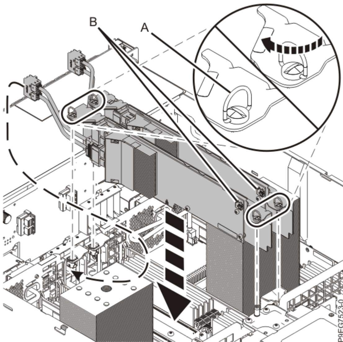
図 12. SAS RAID アダプターの装着
