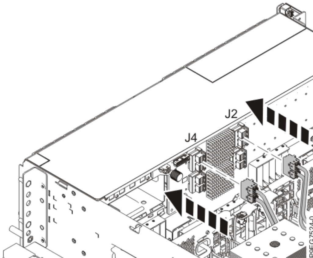
図 15. 12 ドライブ拡張機能ディスク・ドライブ・バックプレーンまたは 18 ドライブ拡張機能ディスク・ドライブ・バックプレーンの前面 SAS ケーブルの再接続
