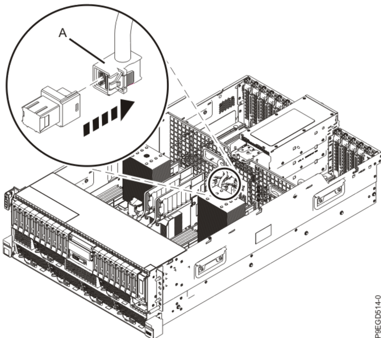
図 31. スロット位置 P1-C49 および P-C50 の SAS RAID 内部アダプターからの背面 SAS ケーブルの切り離し
