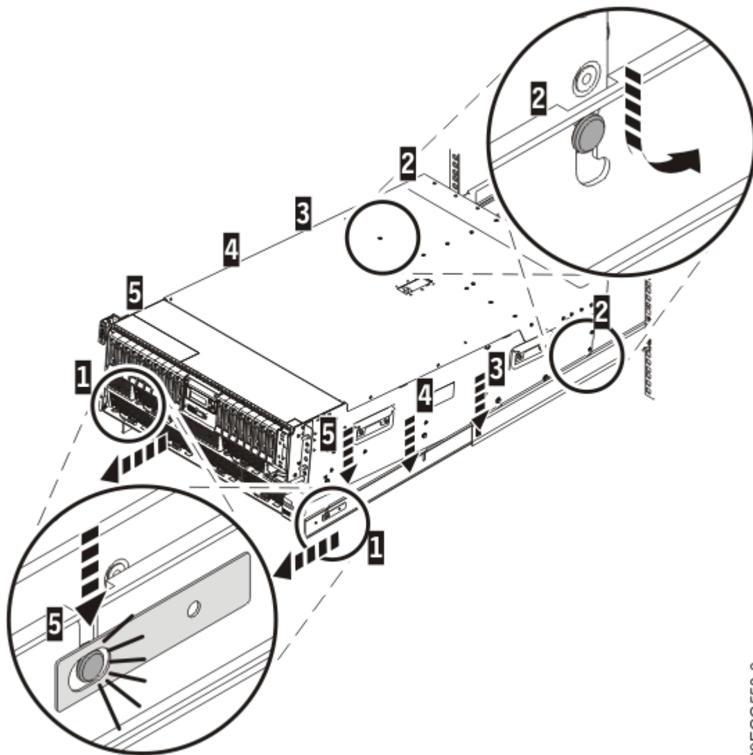
図 7. スライド・レールの延長、およびサーバーのくぎの頭とレールのスロットとの位置合わせ
