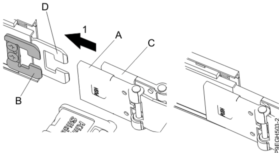
図 11. 取り付けブラケットの挿入
