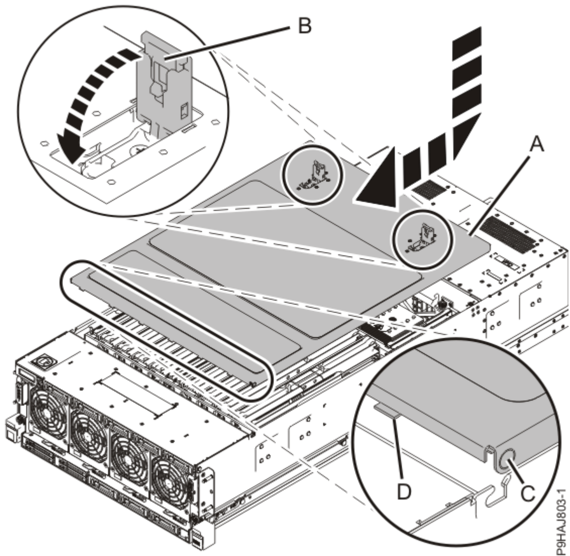
図 13. 保守アクセス・カバーの取り付け
