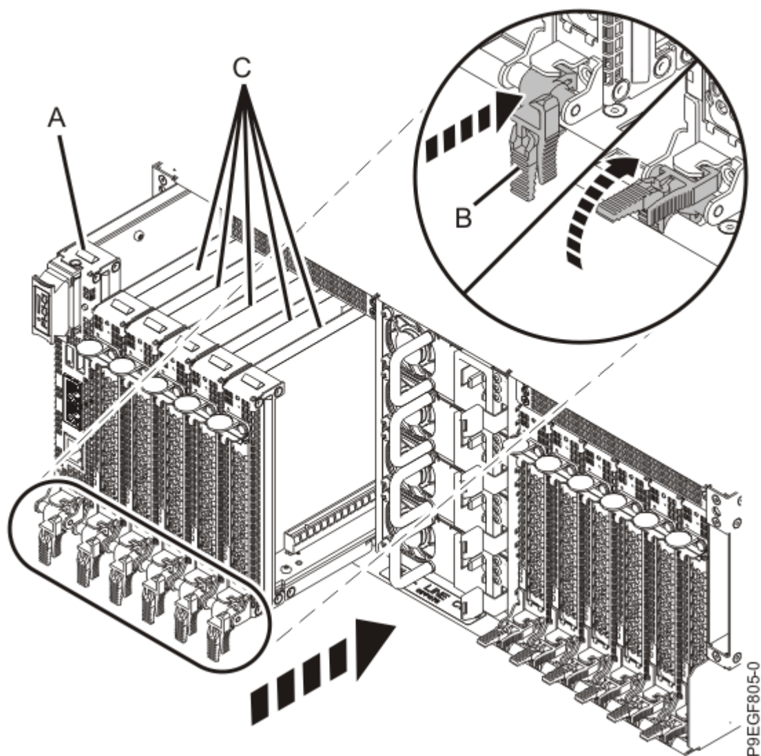
図 15. サービス・プロセッサ・カードおよび PCIe カセットの再取り付け 7. ラベルを使用して電源コード (A) をシステム装置に再接続します (下図を参照)。 次の図に示すように、面ファスナー (B) を使用して、電源コードをシステムに固定します。
