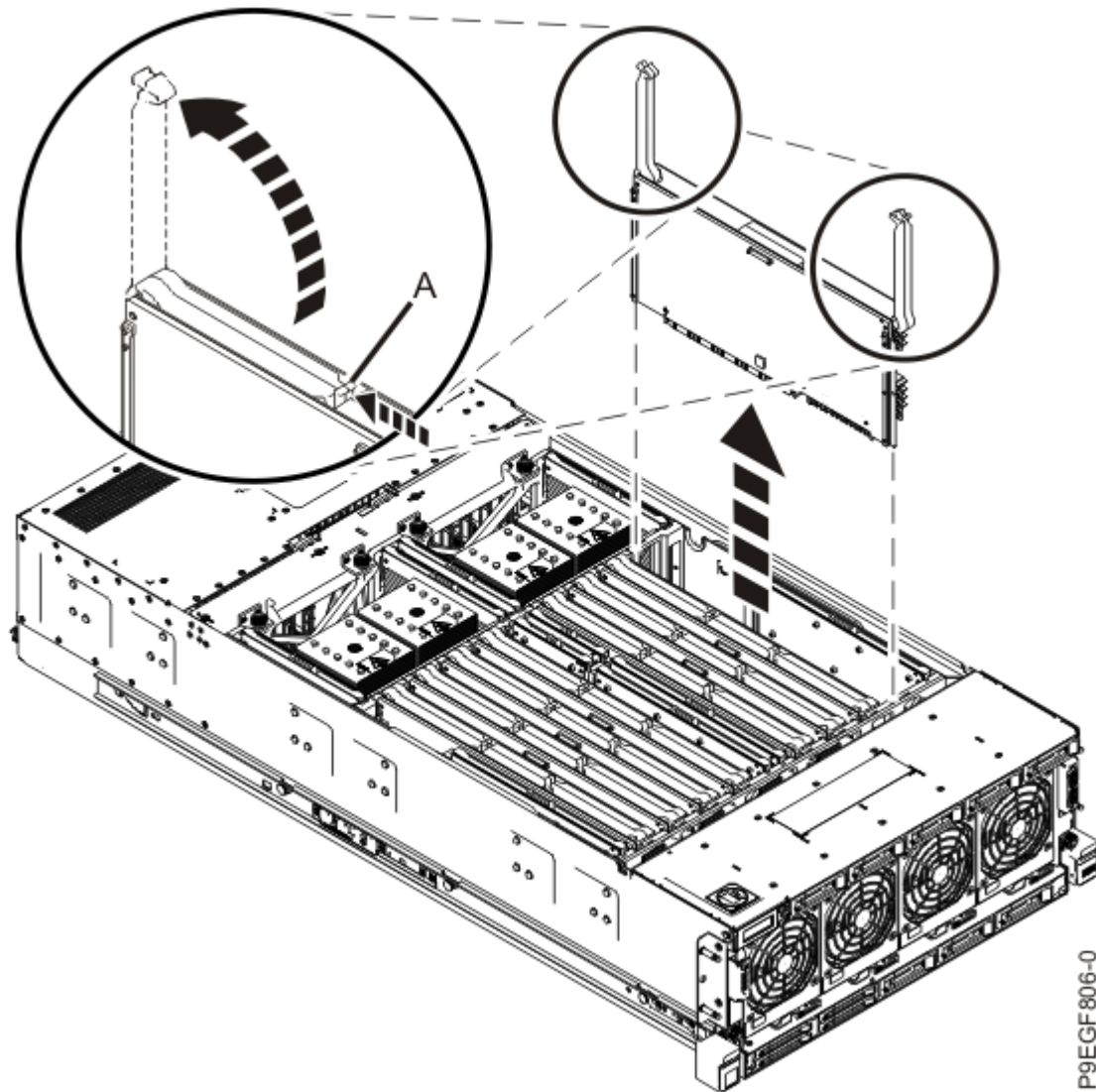
図 5. メモリー・ライザーの取り外し
