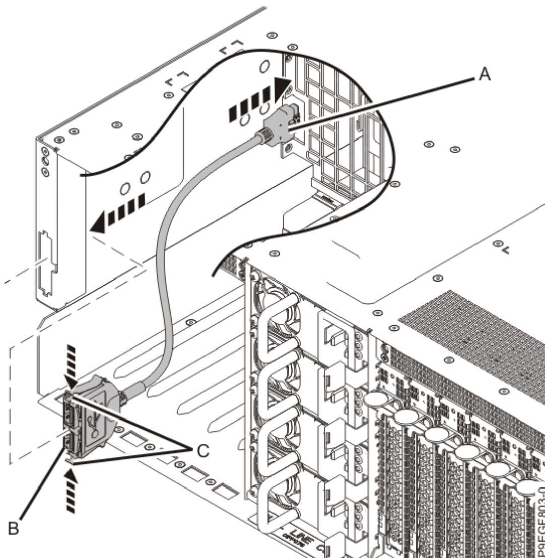
図 9. 背面 USB ポート・コネクタの再取り付け
