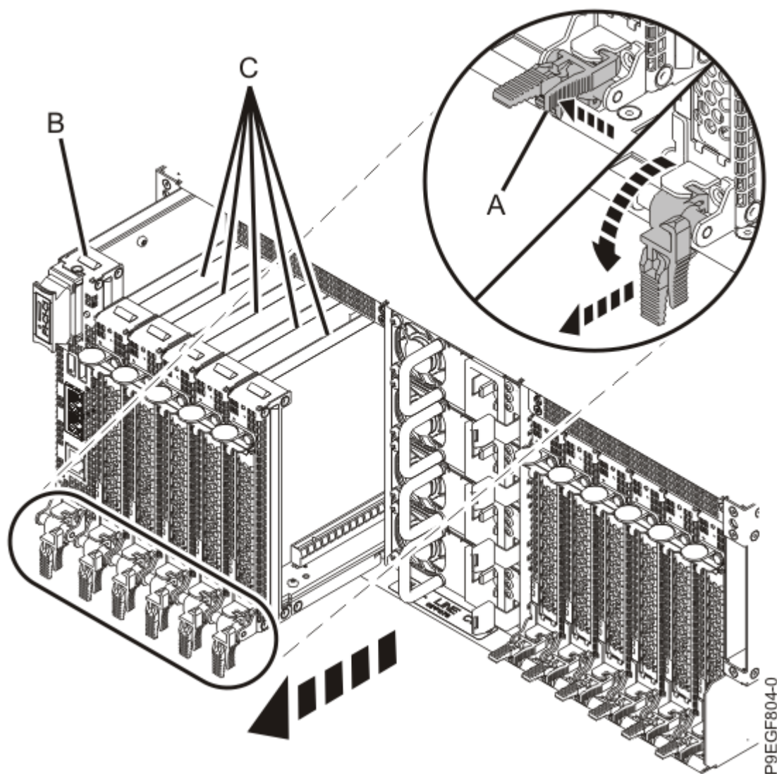
図 2. サービス・プロセッサ・カードおよび PCIe カセットの取り外し
