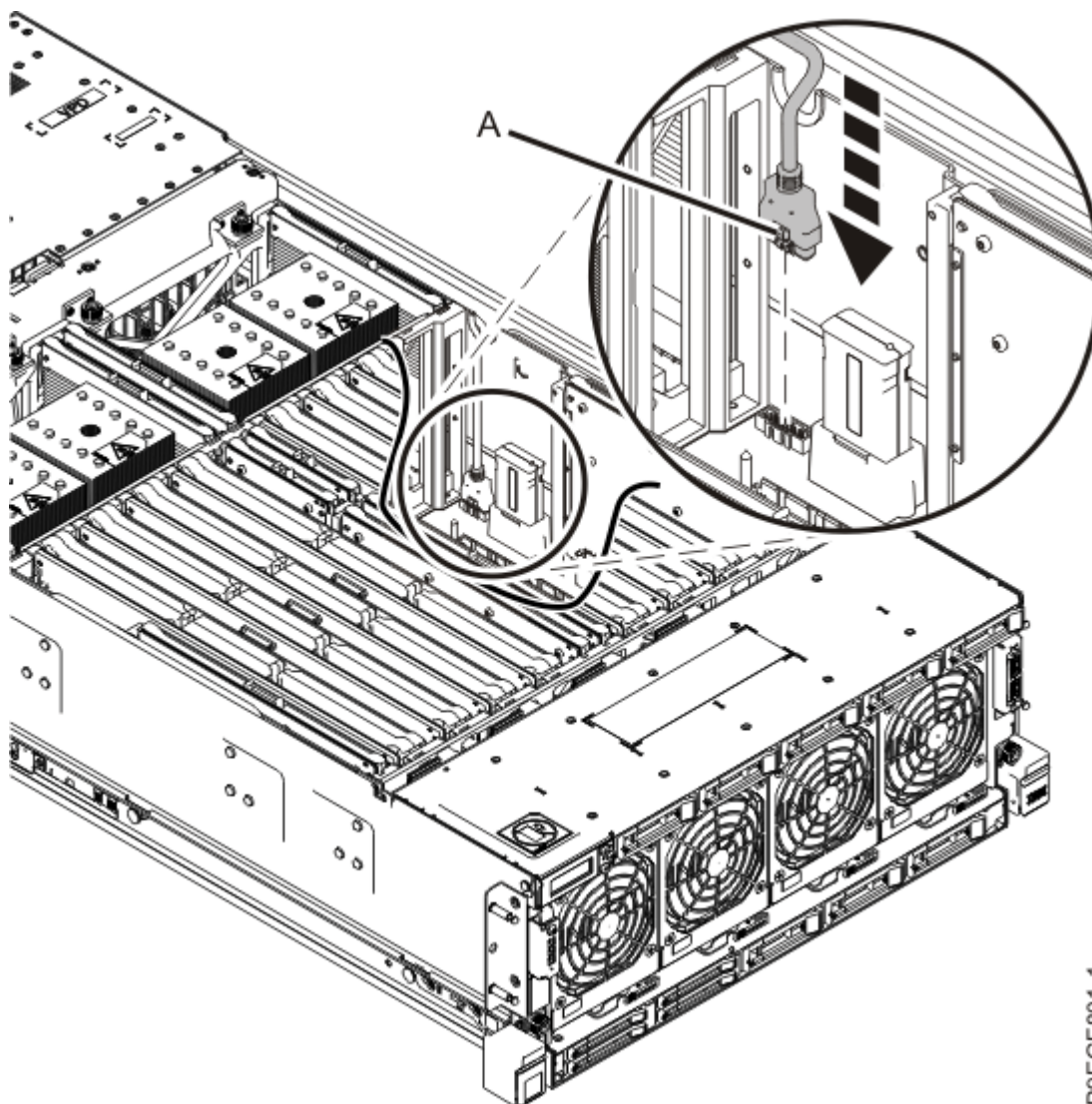
図 11. システム・バックプレーンへの背面 USB ケーブルの再取り付け
