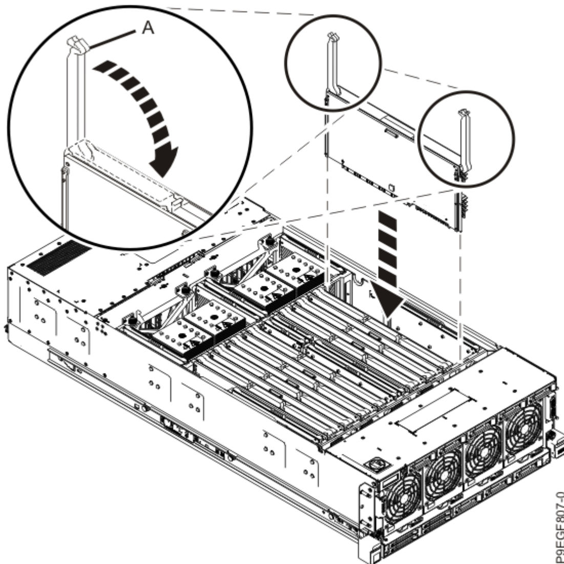
図 12. メモリー・ライザーの取り付け
