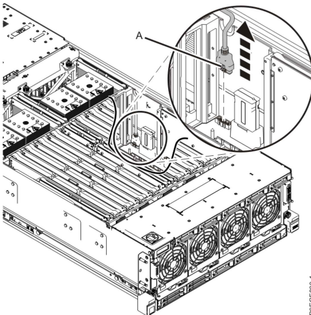
図 6. システム・バックプレーンからの背面 USB ケーブルの取り外し
