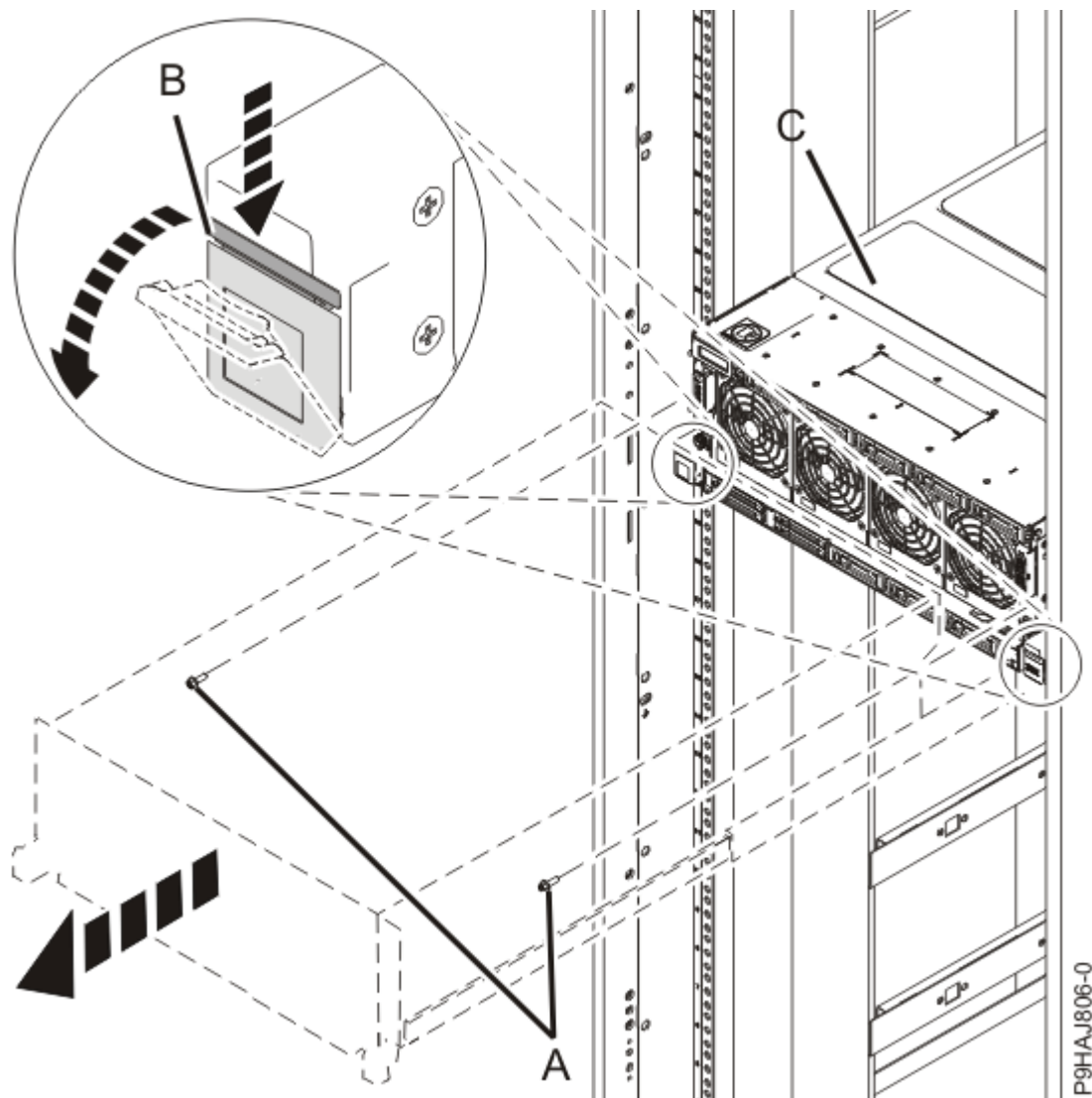
図 10. システムの保守位置への設置
