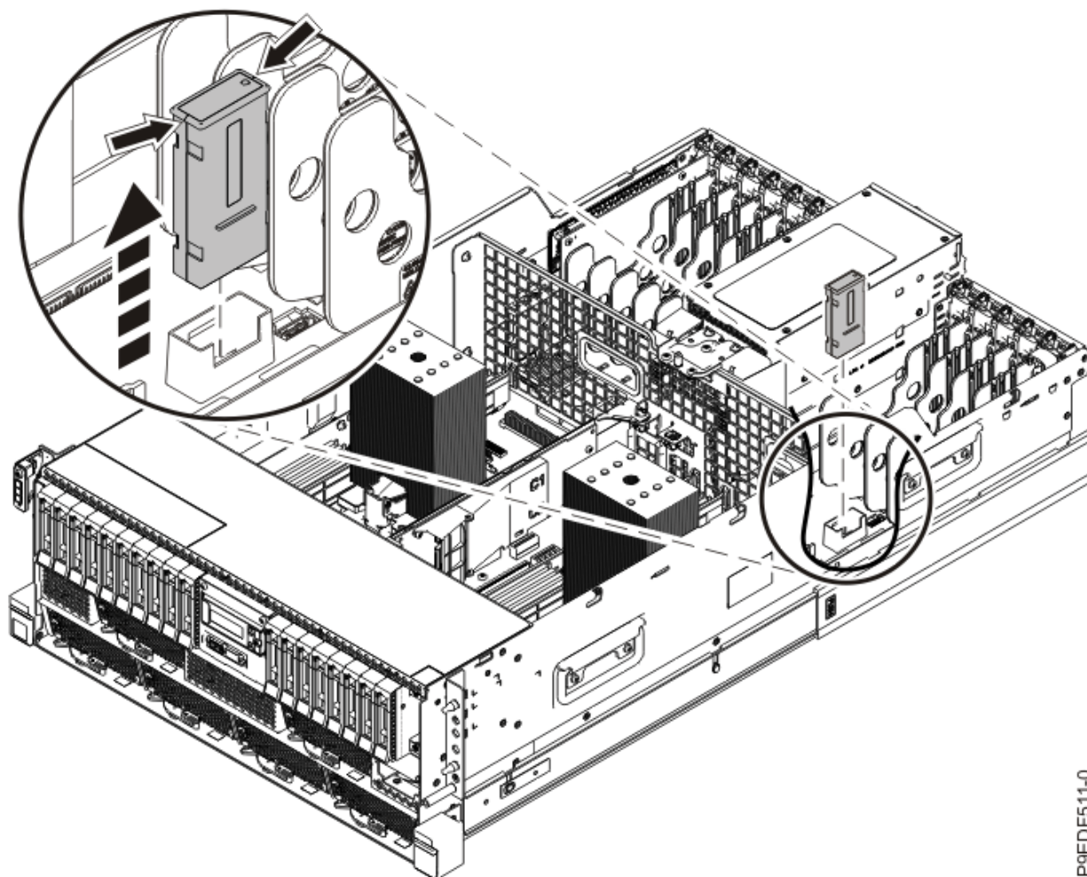
図 7. VPD カードの取り外し
