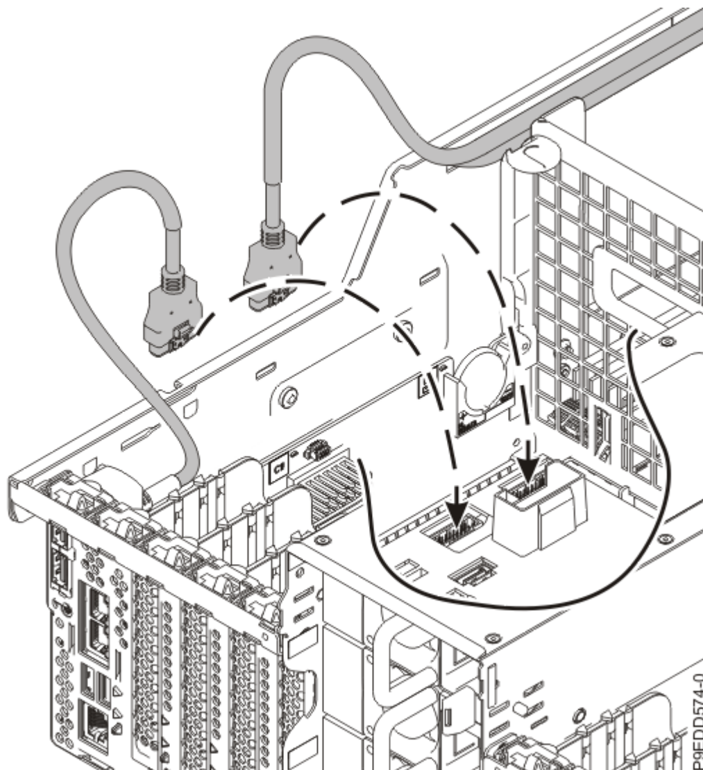
図 13. 前面 USB ケーブルおよび背面 USB ケーブルの再取り付け
