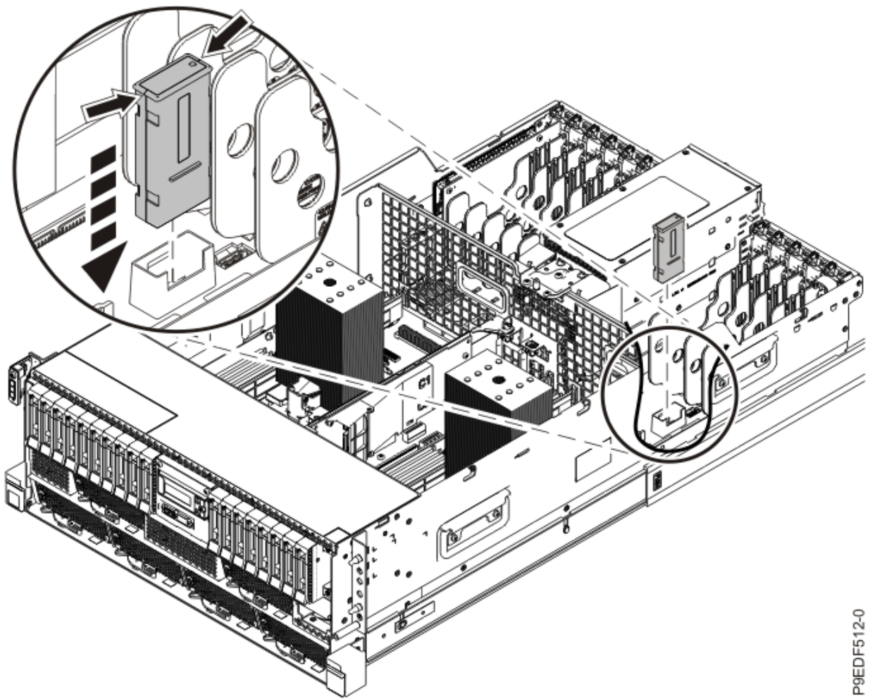
図 14. VPD カードの再取り付け
