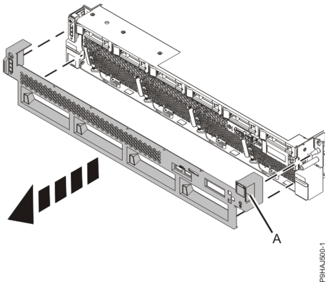
図 2. 前面カバーの取り外し
