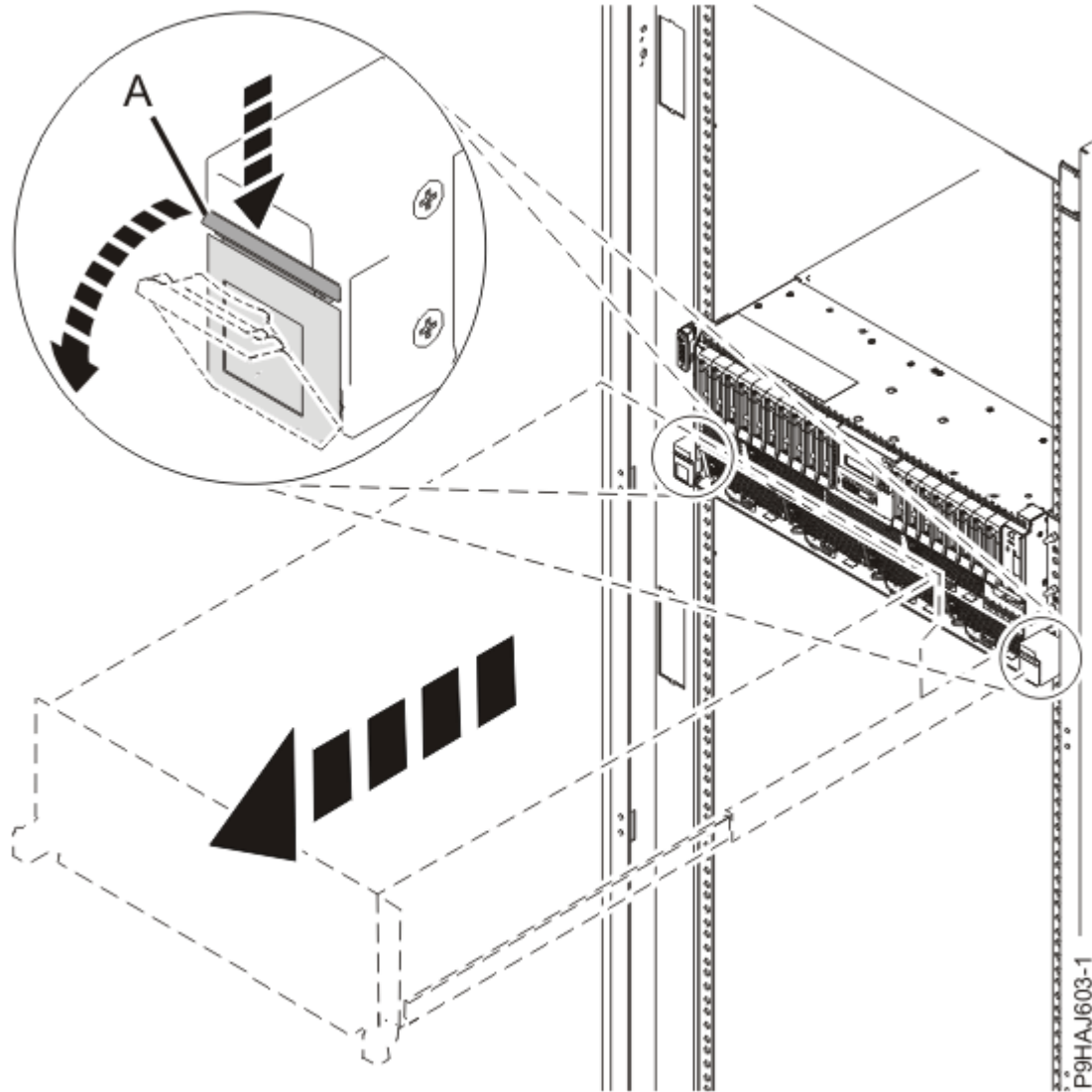
図 7. サイド・ラッチのリリース
