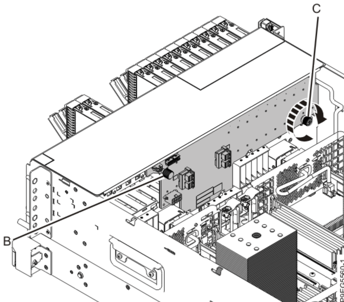
図 28. ディスク・ドライブ・バックプレーンの再取り付け
