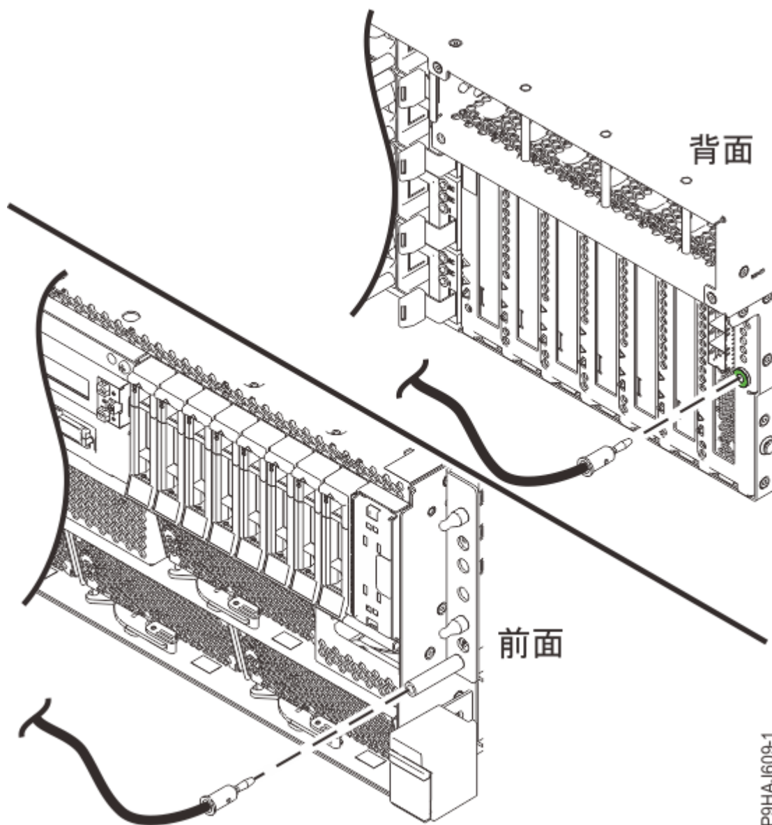
図 8. ESD プラグの位置
