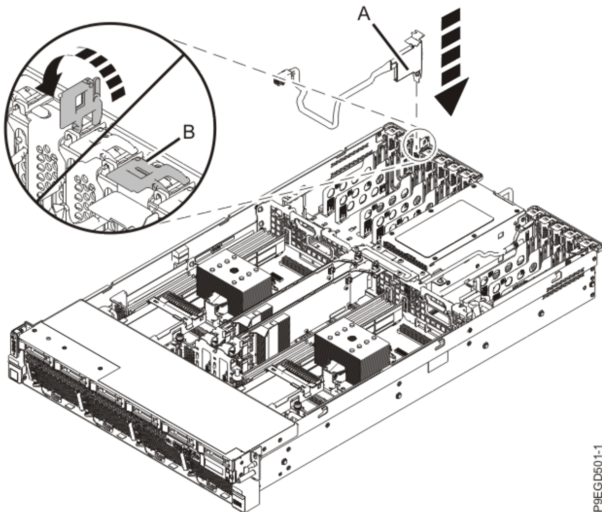
図 8. 背面 SAS ケーブルの取り付け
