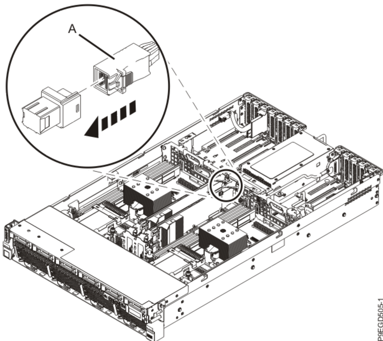
図 10. 背面 SAS ケーブルの取り付け
