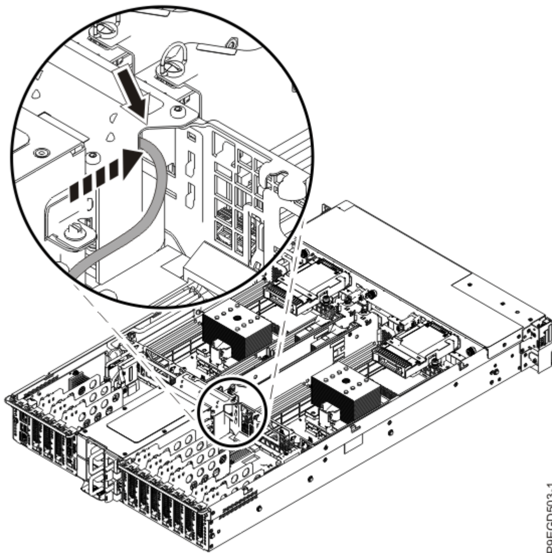
図 9. 背面 SAS ケーブルの配線
