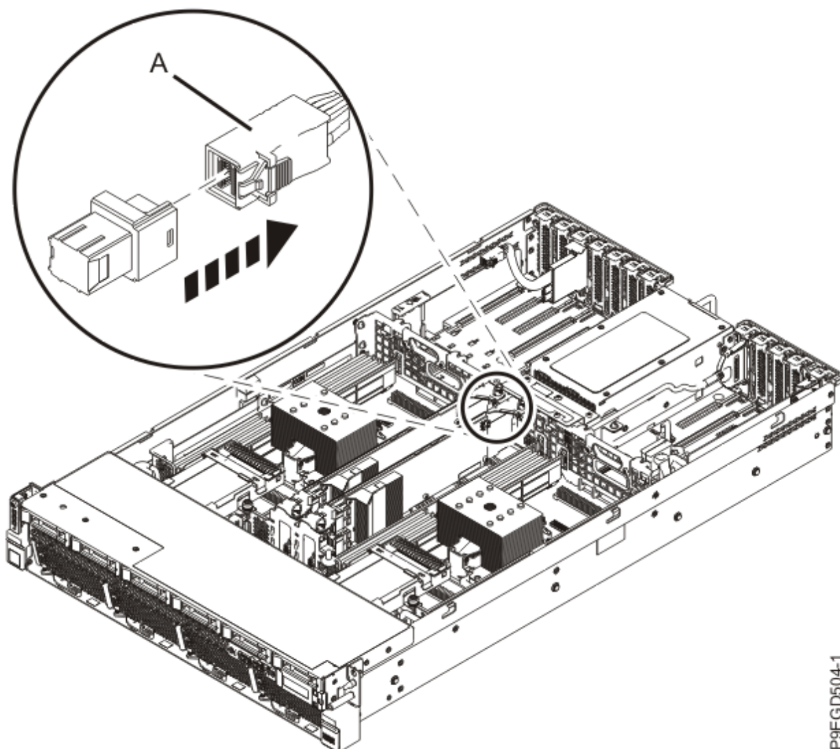
図 6. SAS RAID 内部アダプターからの背面 SAS ケーブルの切り離し
