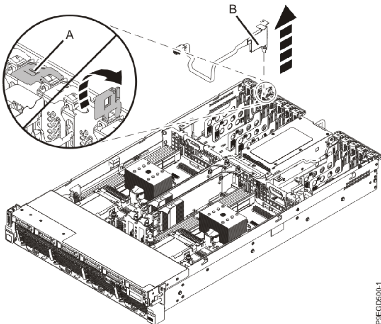
図 7. 背面 SAS ケーブル・アダプターの取り外し
