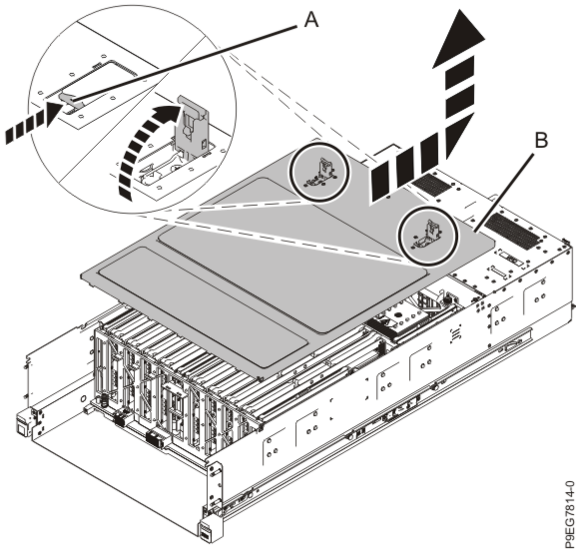
図 33. 保守アクセス・カバーの取り外し
