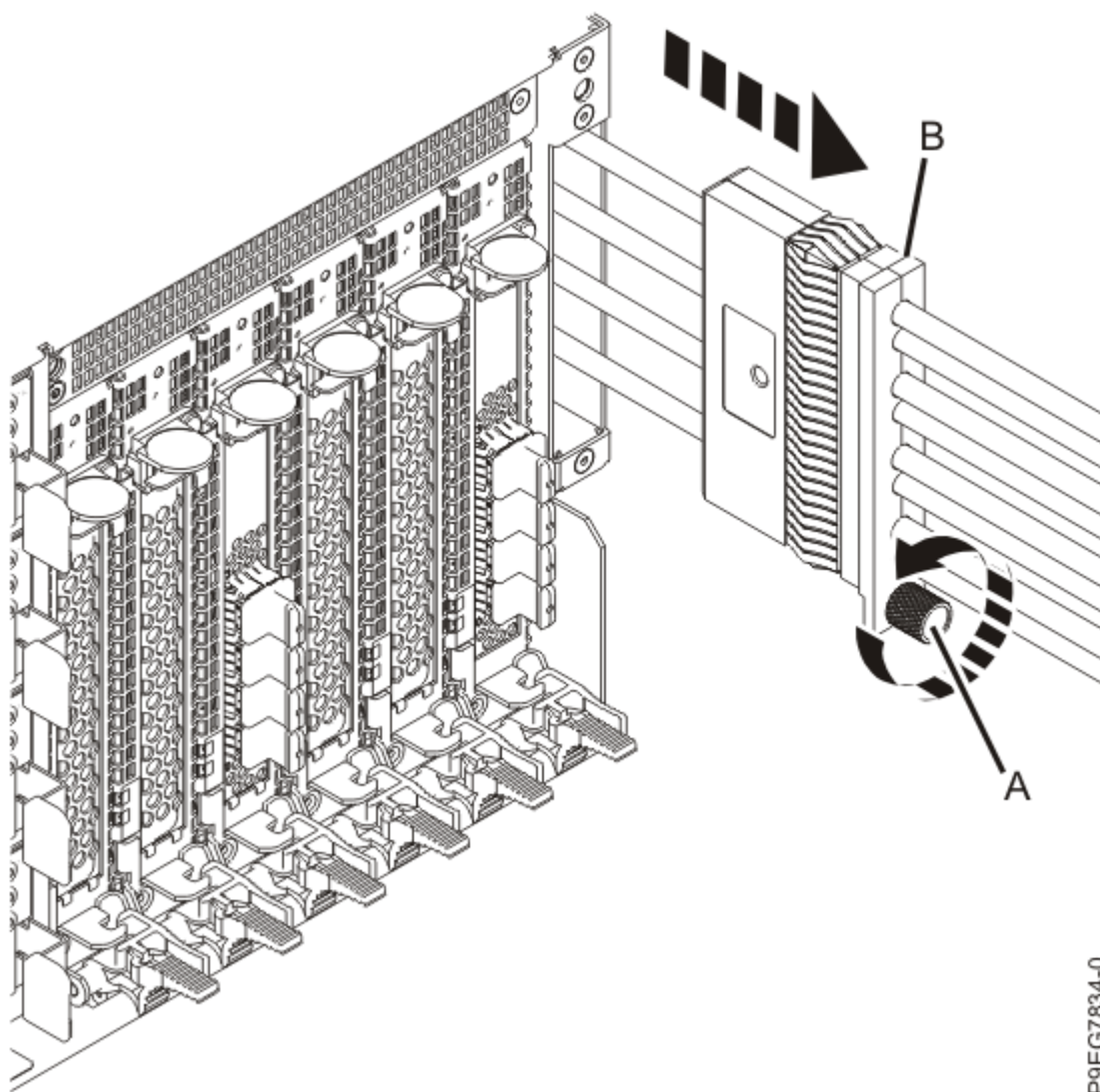
図 26. 拡張機能ディスク・ドライブ・バックプレーンからの SAS ケーブル・ホルダーおよび SAS ケーブルの取り外し
