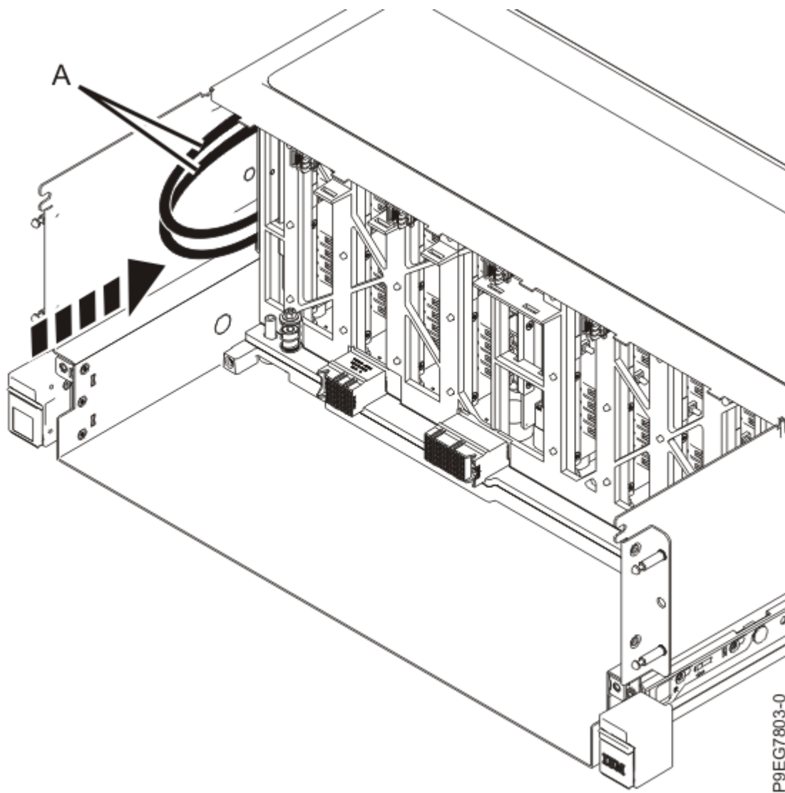
図 19. SAS ケーブルを輪にして、基本機能ディスク・ドライブ・バックプレーンのシステム内へ押し込む
