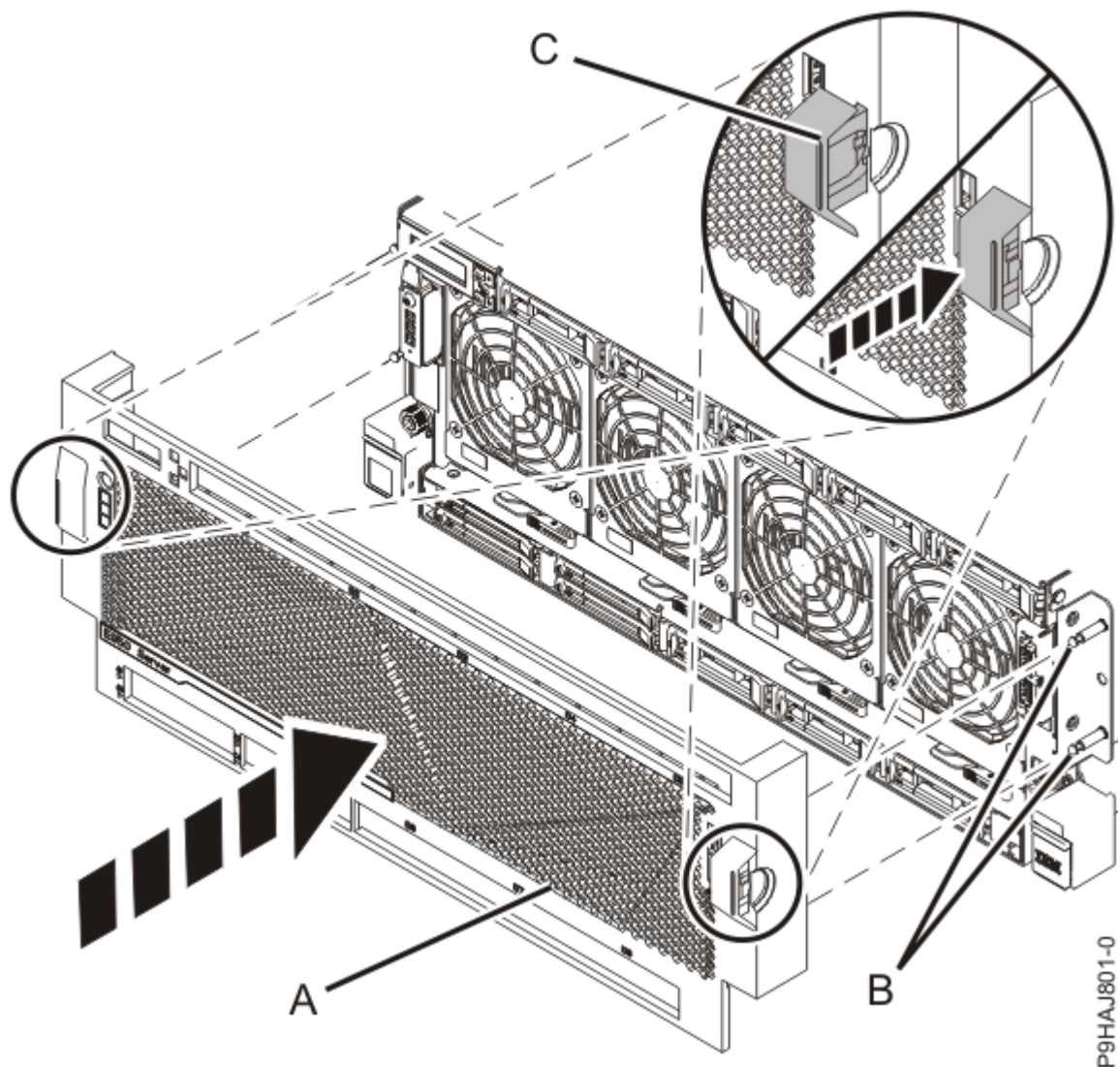
図 46. 前面カバーの取り付け
