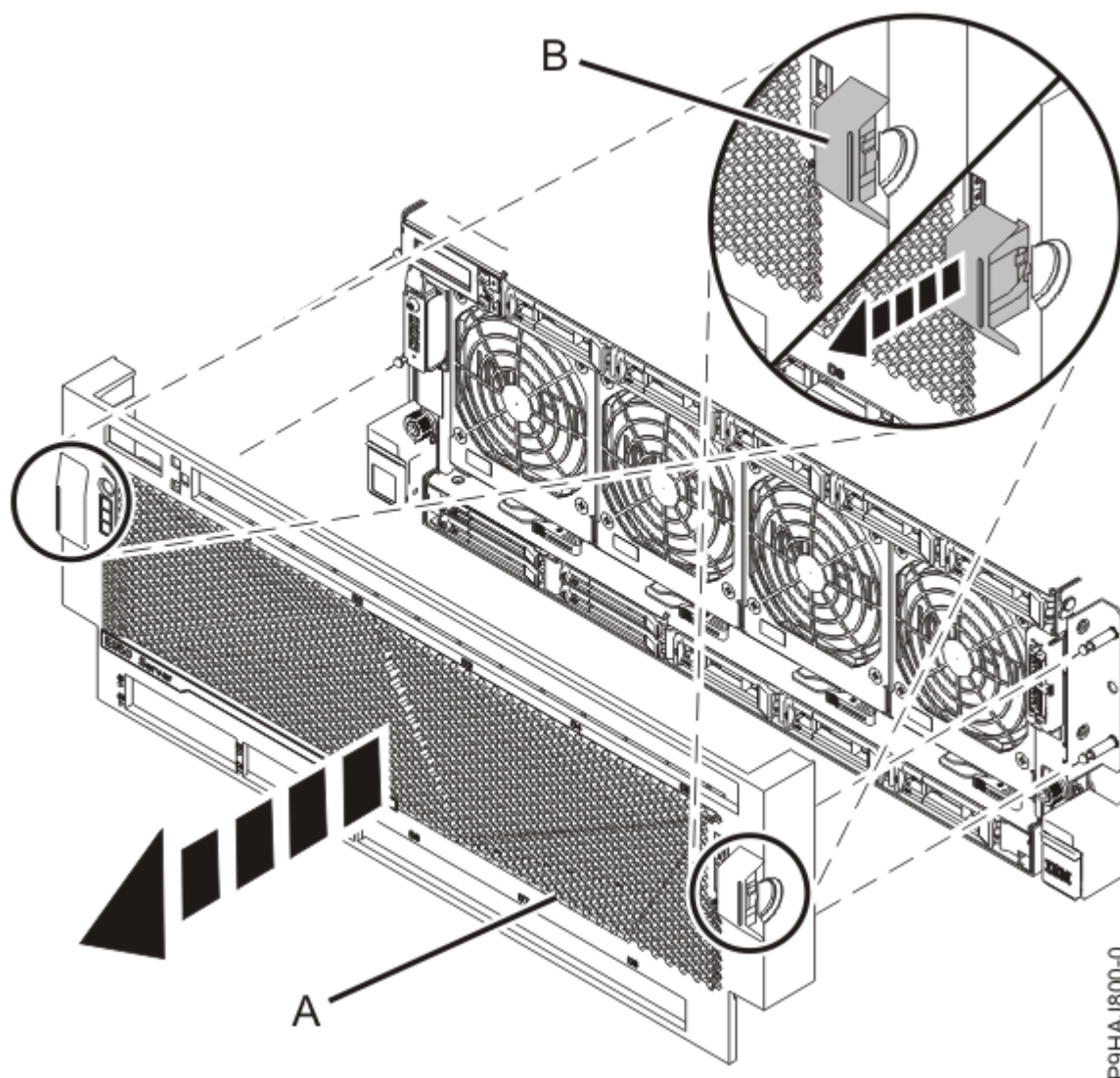
図 4. 前面カバーの取り外し
