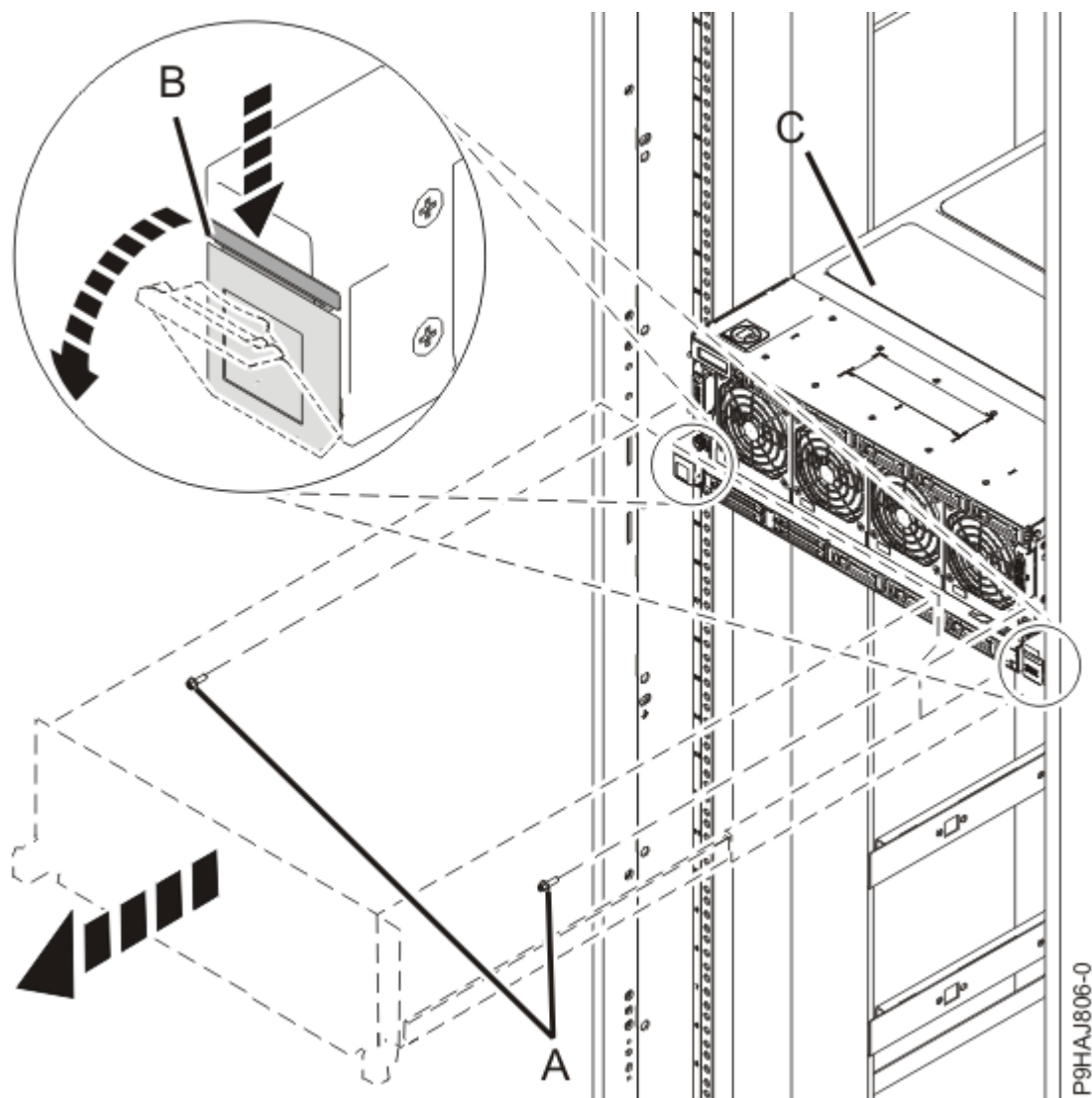
図 5. システムの保守位置への設置 12. 保守アクセス・カバーを取り外します。
