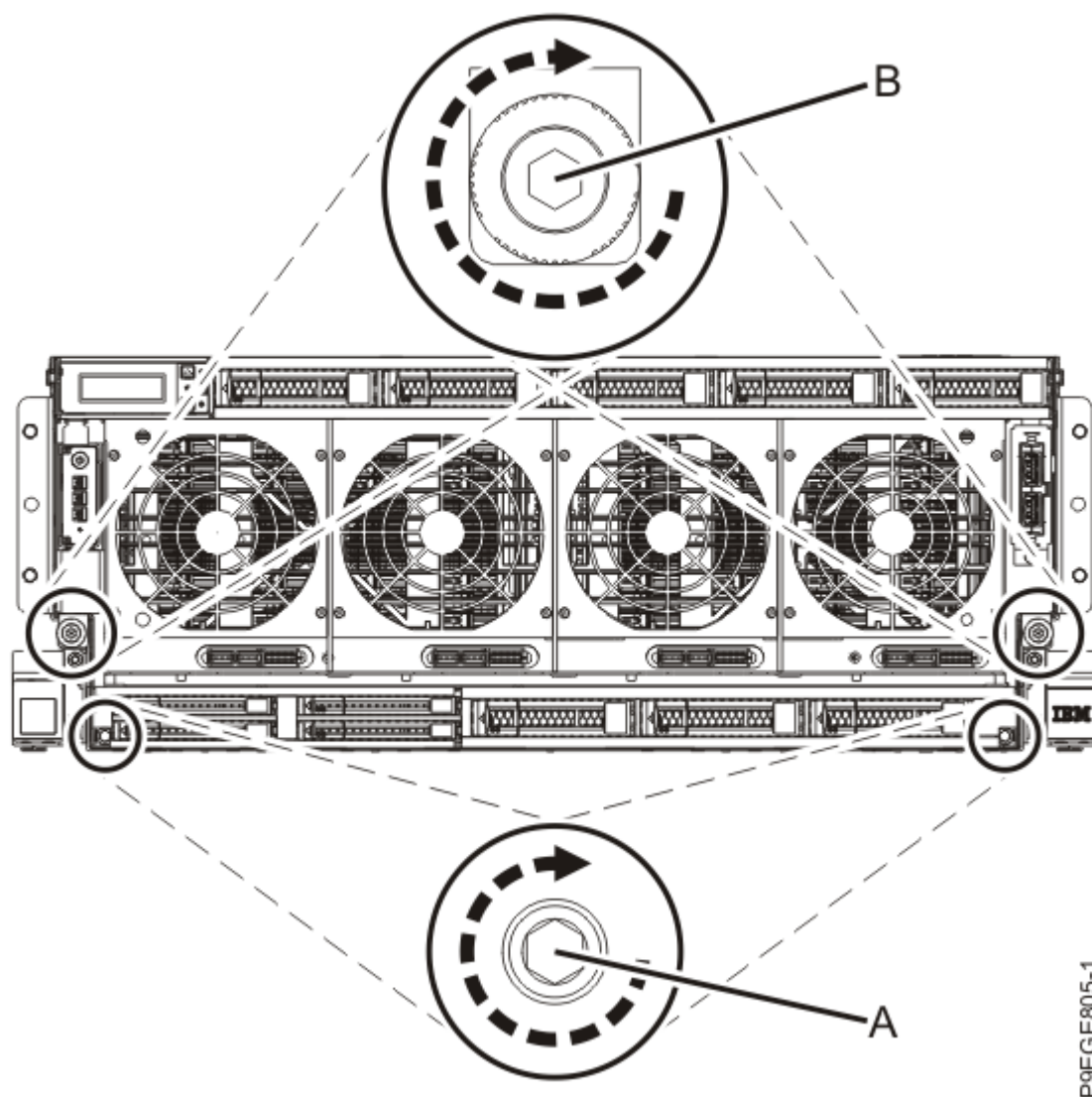
図 44. ディスク・ドライブ・バックプレーンのねじを締める
