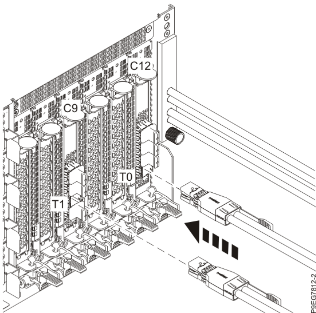
図 30. 基本機能ディスク・ドライブ・バックプレーンの分割構成用の SAS ケーブルのプラグを差し込む
