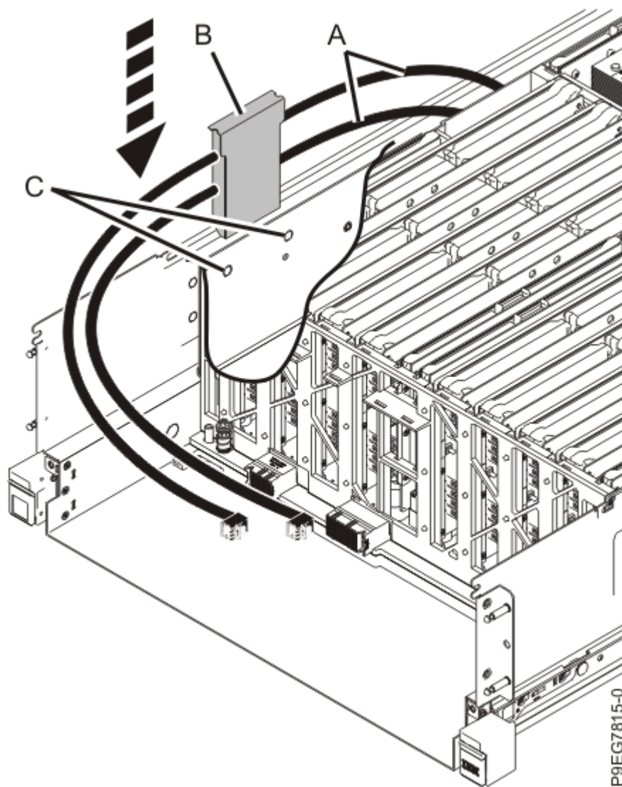
図 34. 基本機能ディスク・ドライブ・バックプレーンの SAS ケーブル・サポートの再取り付け
