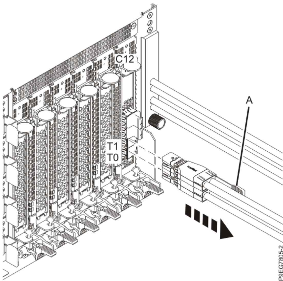
図 22. 基本機能ディスク・ドライブ・バックプレーンの基本構成用の SAS ケーブルの切り離し
