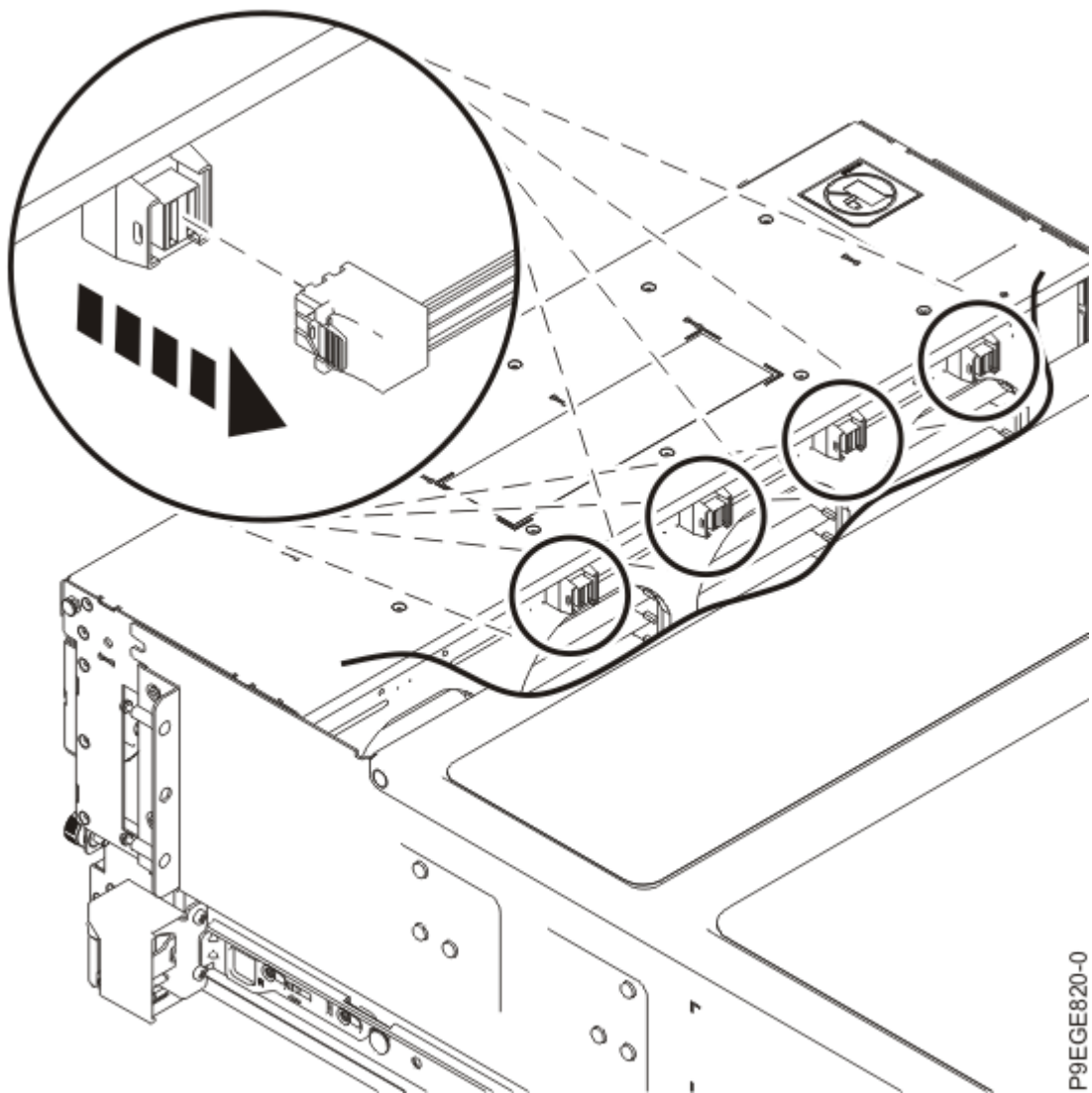
図 13. 拡張機能ディスク・ドライブ・バックプレーンから SAS ケーブルのプラグを引き抜く f) 両手を使用して、ディスク・ドライブ・バックプレーンをシステムから完全に取り外します。
