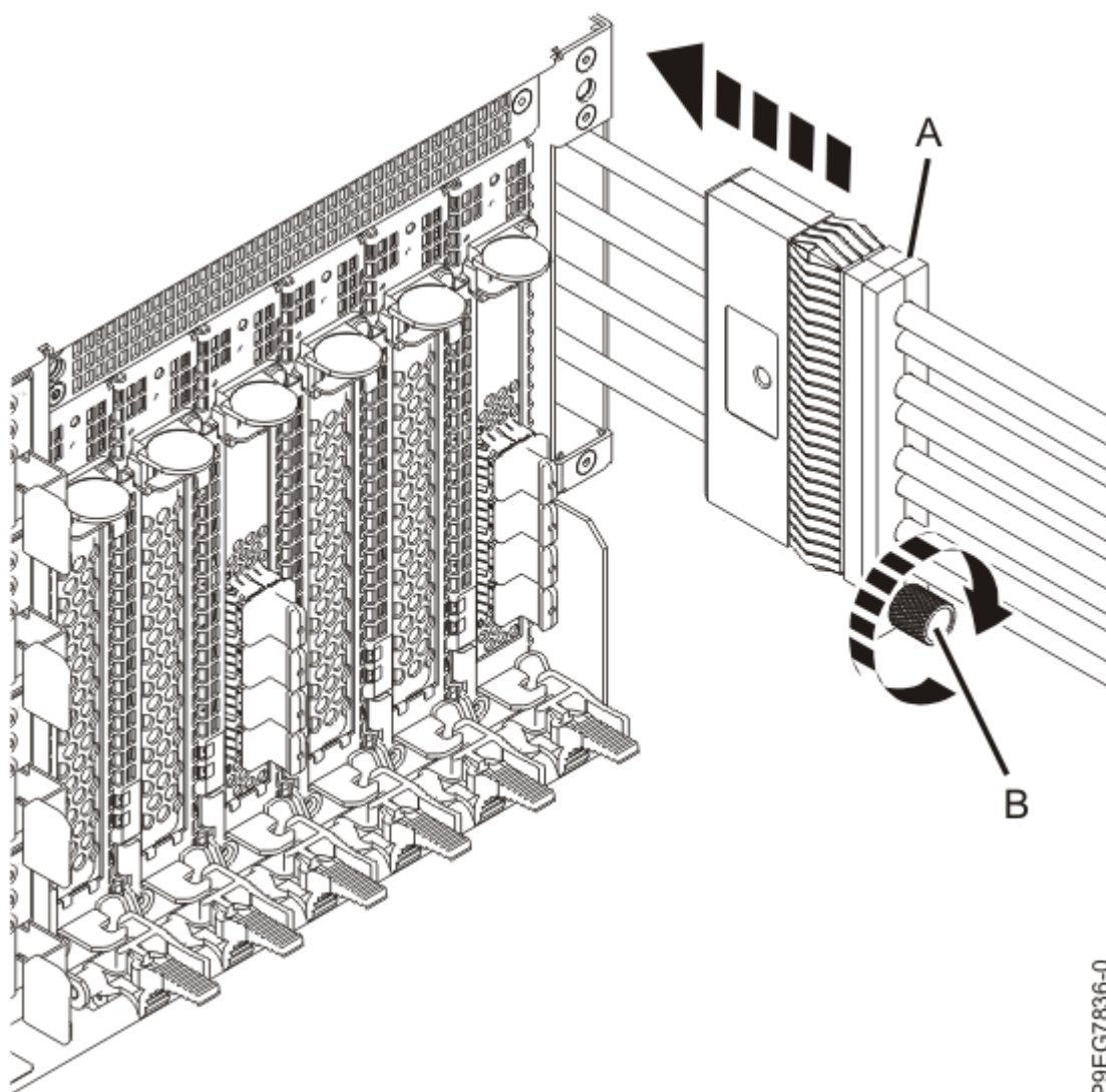
図 28. 拡張機能ディスク・ドライブ・バックプレーンの SAS ケーブルおよび SAS ケーブル・ホルダーの挿入
