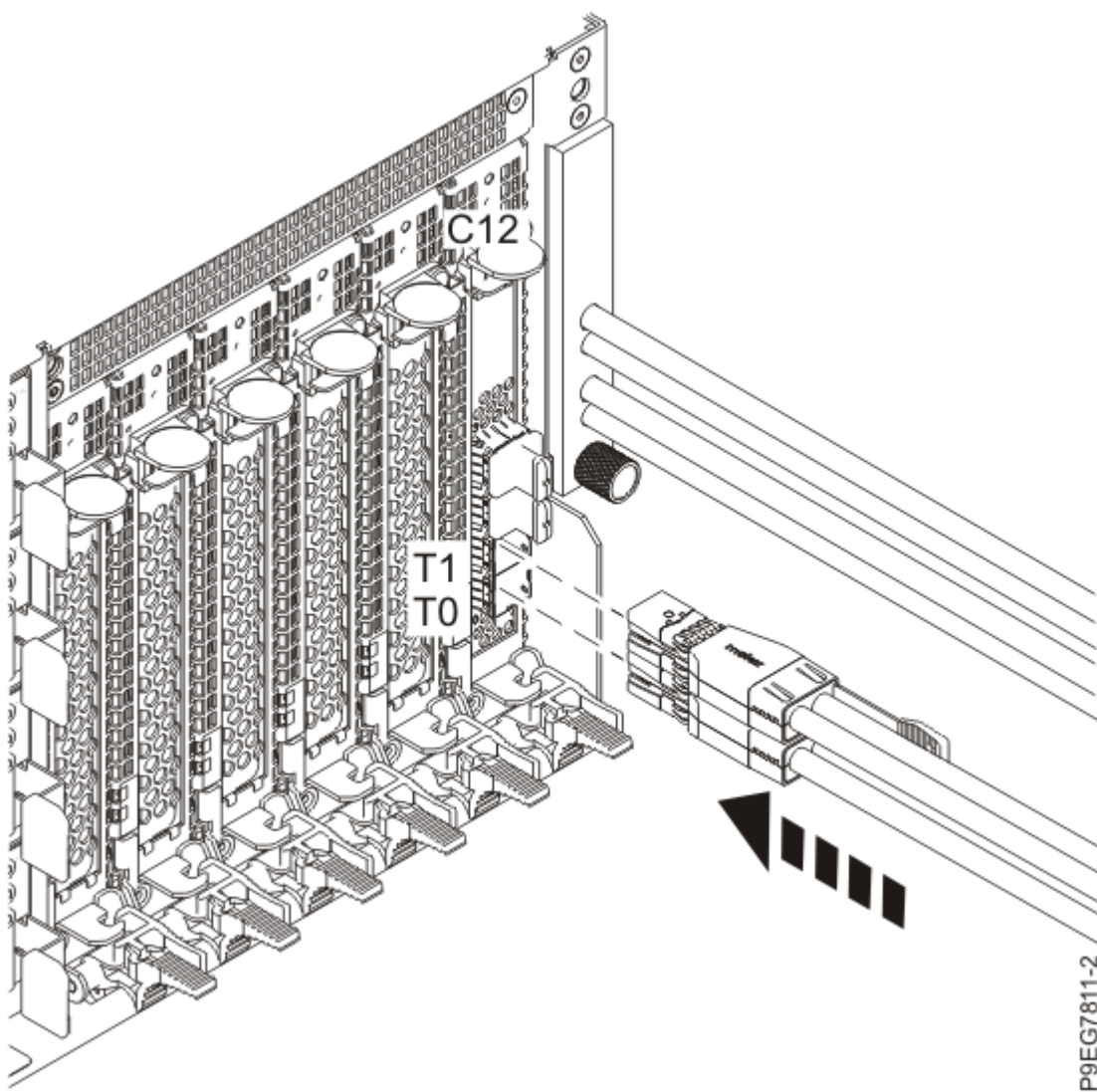
図 29. 基本機能ディスク・ドライブ・バックプレーンの基本構成用の SAS ケーブルのプラグを差し込む
