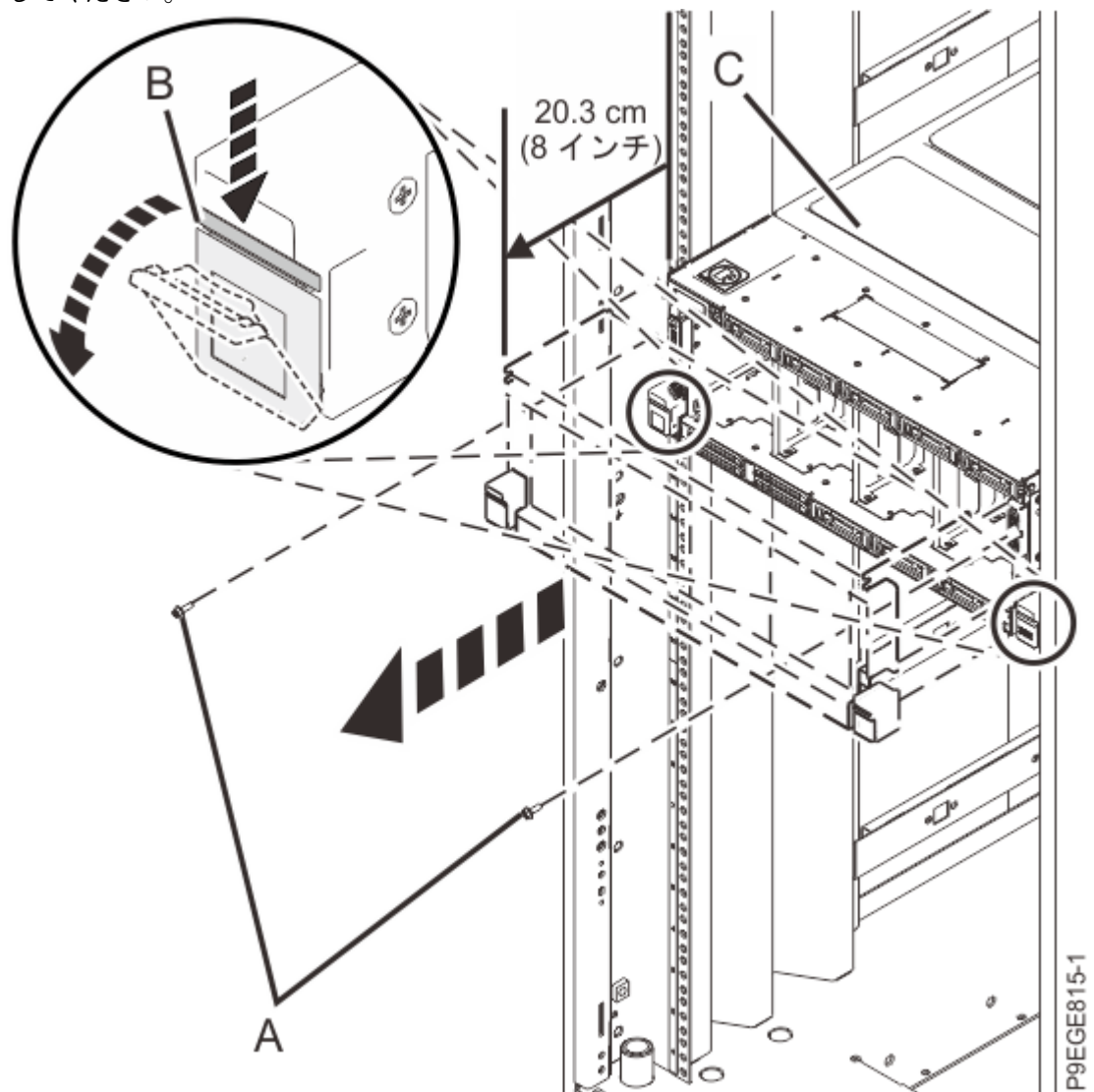
図 11. ラックからの部分的なシステムのスライド
