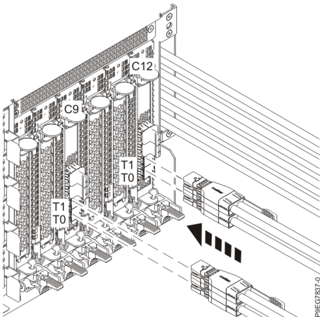
図 31. 拡張機能ディスク・ドライブ・バックプレーンの SAS ケーブルのプラグを差し込む
