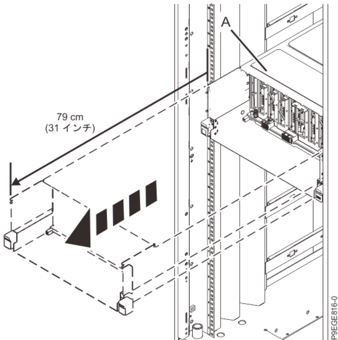
図 15. ラックからの部分的なシステムのスライド
