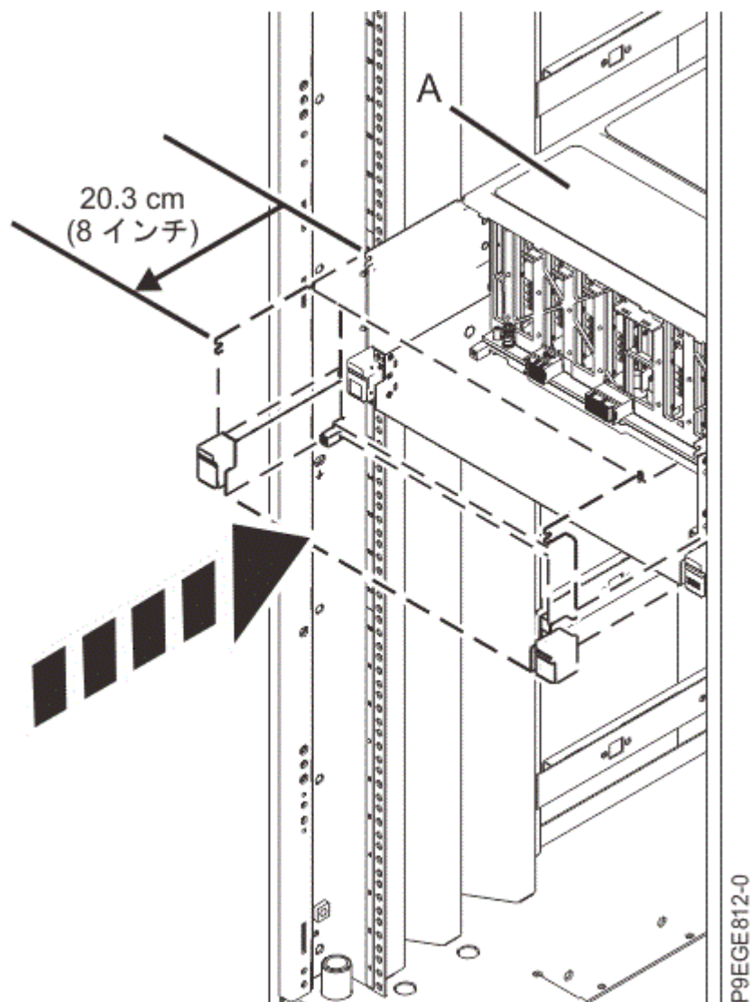
図 39. ラックへの部分的なシステムのスライド
