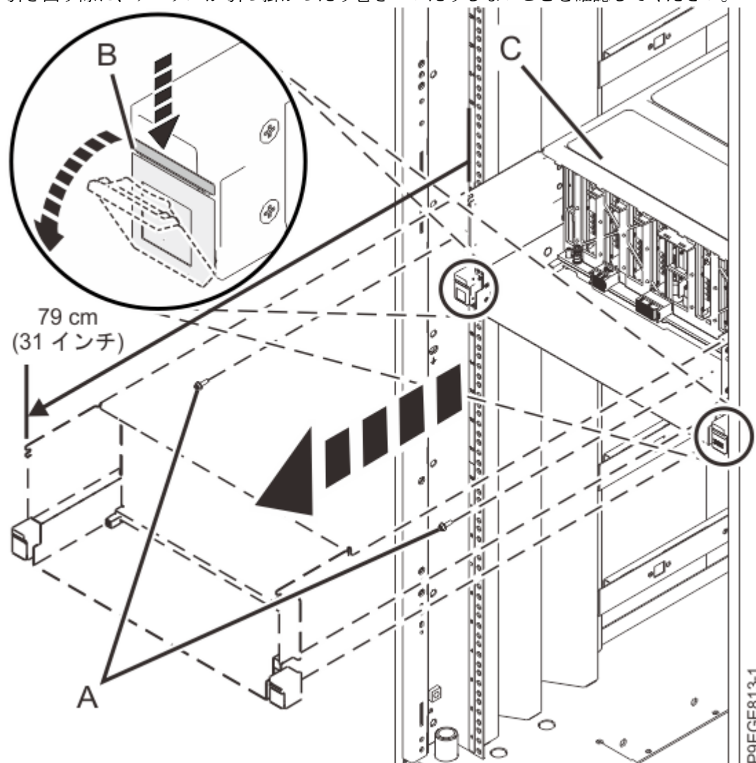
図 32. ラックからの部分的なシステムのスライド
