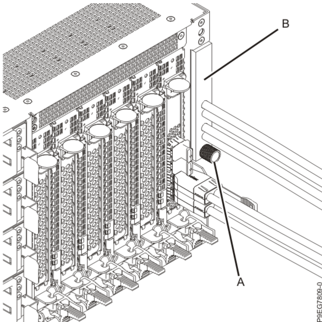
図 2. 外部保護 SAS ケーブルの識別
