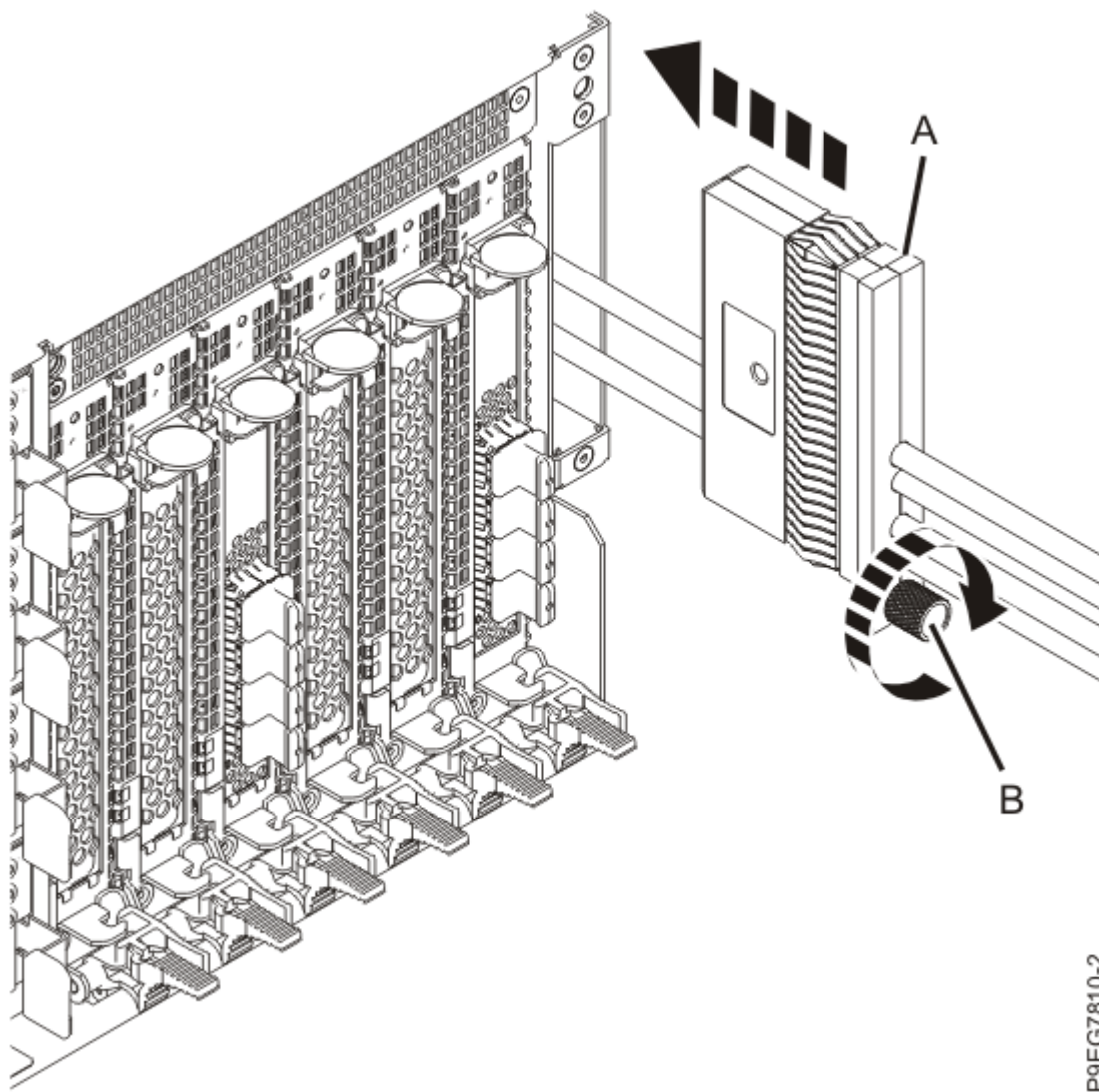
図 27. 基本機能ディスク・ドライブ・バックプレーンの SAS ケーブルおよび SAS ケーブル・ホルダーの挿入
