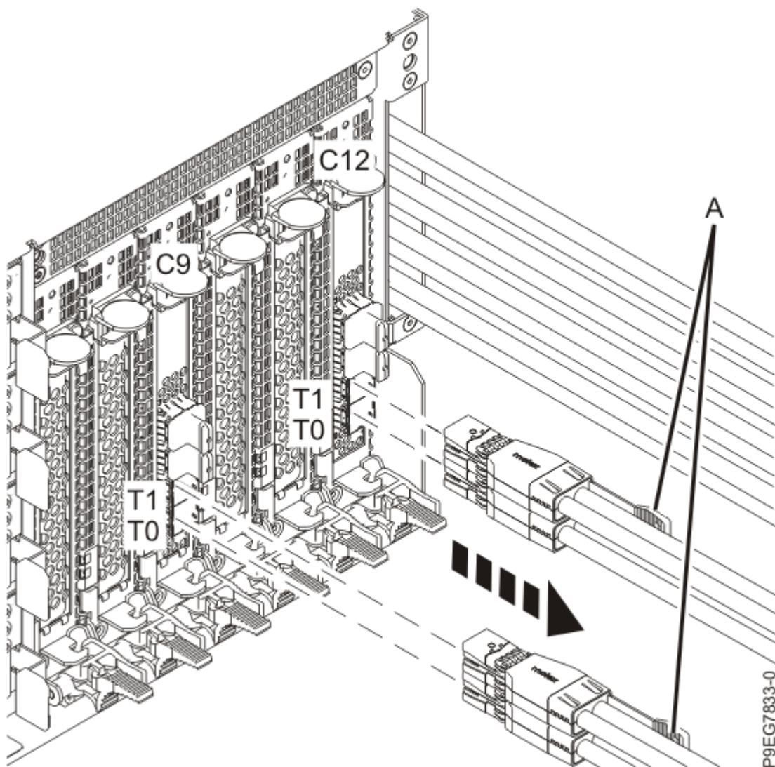
図 24. 拡張機能ディスク・ドライブ・バックプレーンの SAS ケーブルの切り離し 10. SAS ケーブル・ホルダー (B) をシステムの背面に固定しているねじ (A) を緩めます。 システムの背面から SAS ケーブル・ホルダーおよび SAS ケーブルを取り外します。
