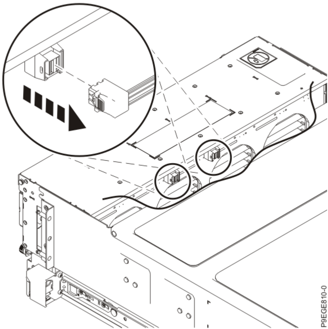
図 12. 基本機能ディスク・ドライブ・バックプレーンから SAS ケーブルのプラグを引き抜く
