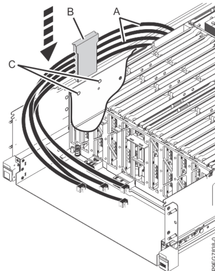
図 35. 拡張機能ディスク・ドライブ・バックプレーンの SAS ケーブル・サポートの再取り付け 7. システムの前面への SAS ケーブルの配線
