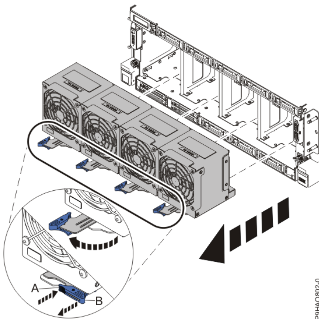
図 8. ファンの取り外し
