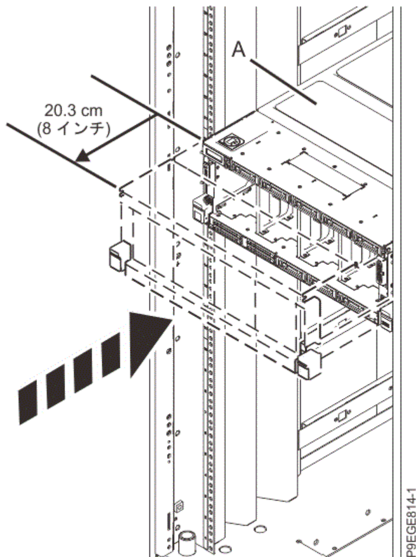
図 43. システムの操作位置への設置
