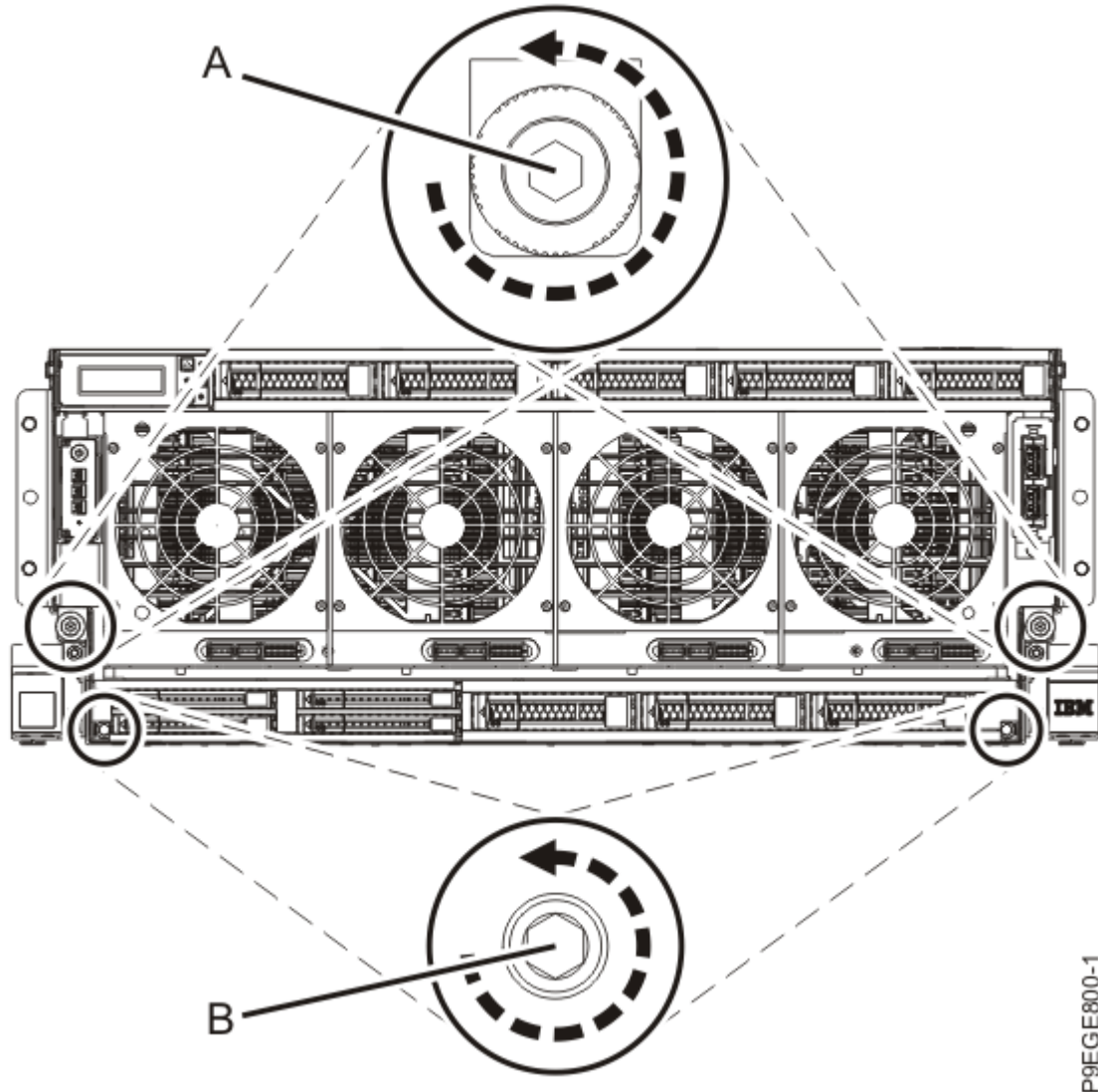
図 9. ディスク・ドライブ・バックプレーンのねじを緩める
