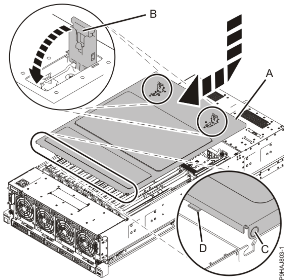
図 48. 保守アクセス・カバーの取り付け
