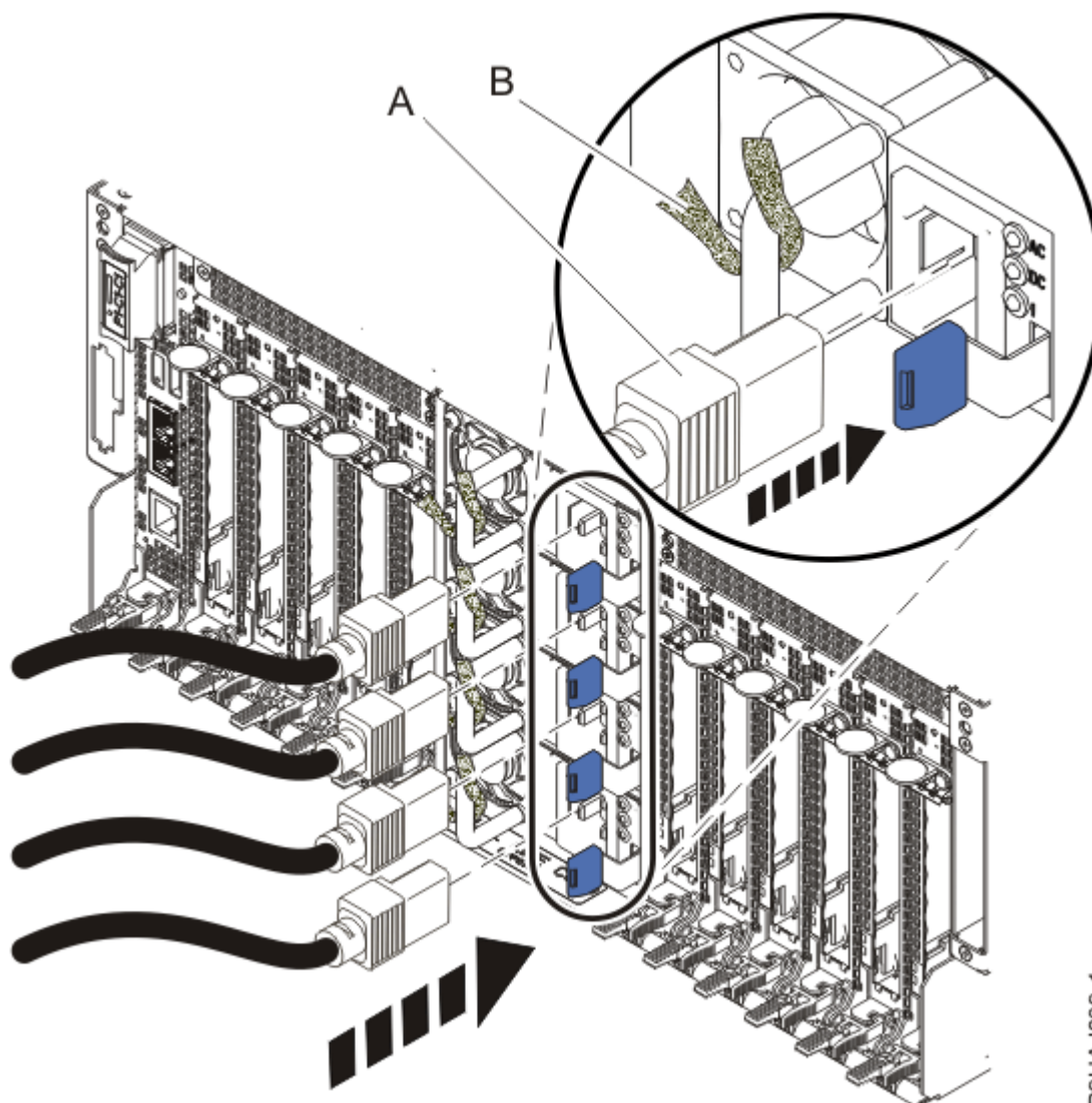
図 50. 電源コードの接続
