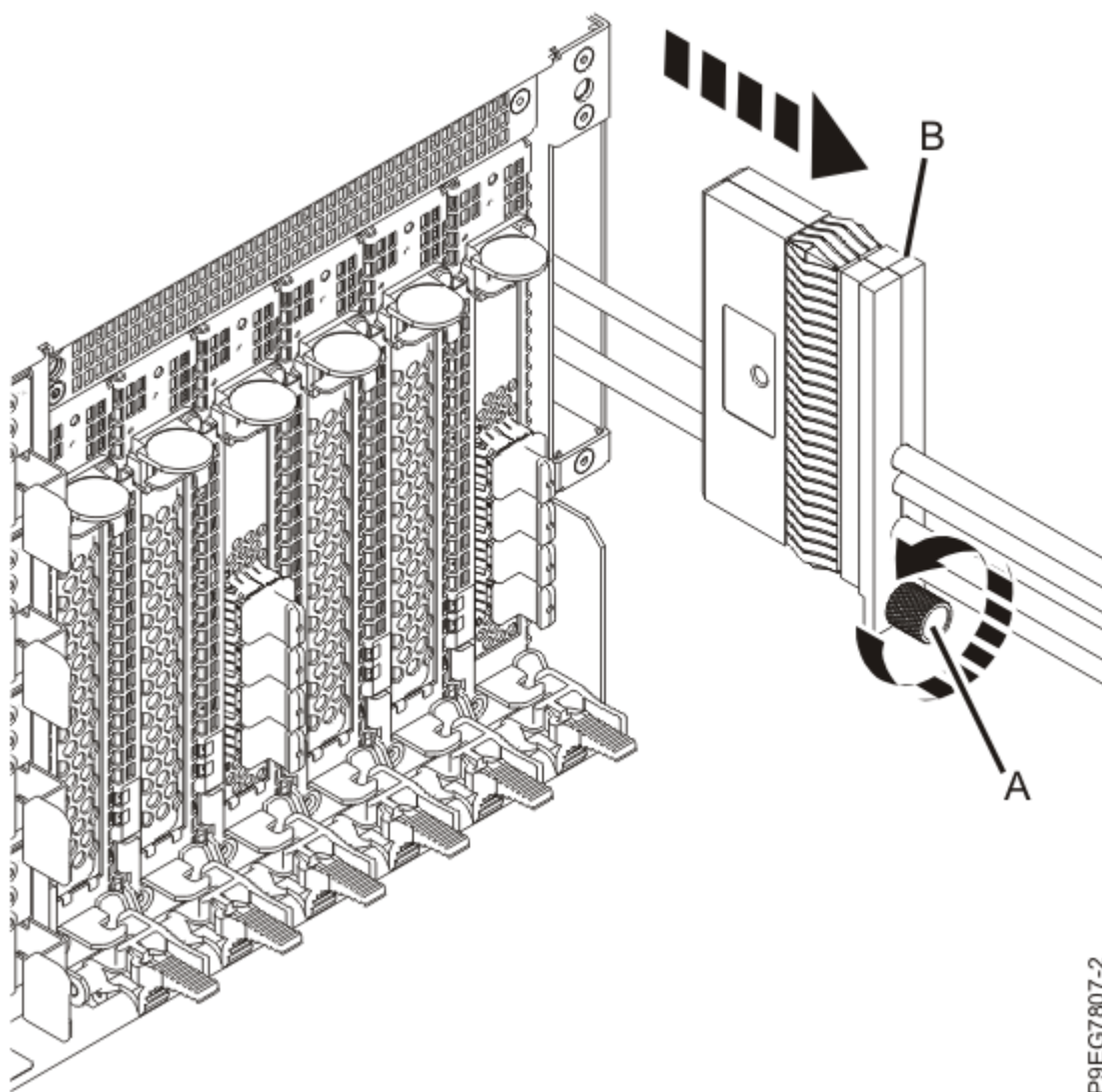
図 25. 基本機能ディスク・ドライブ・バックプレーンからの SAS ケーブル・ホルダーおよび SAS ケーブルの取り外し
