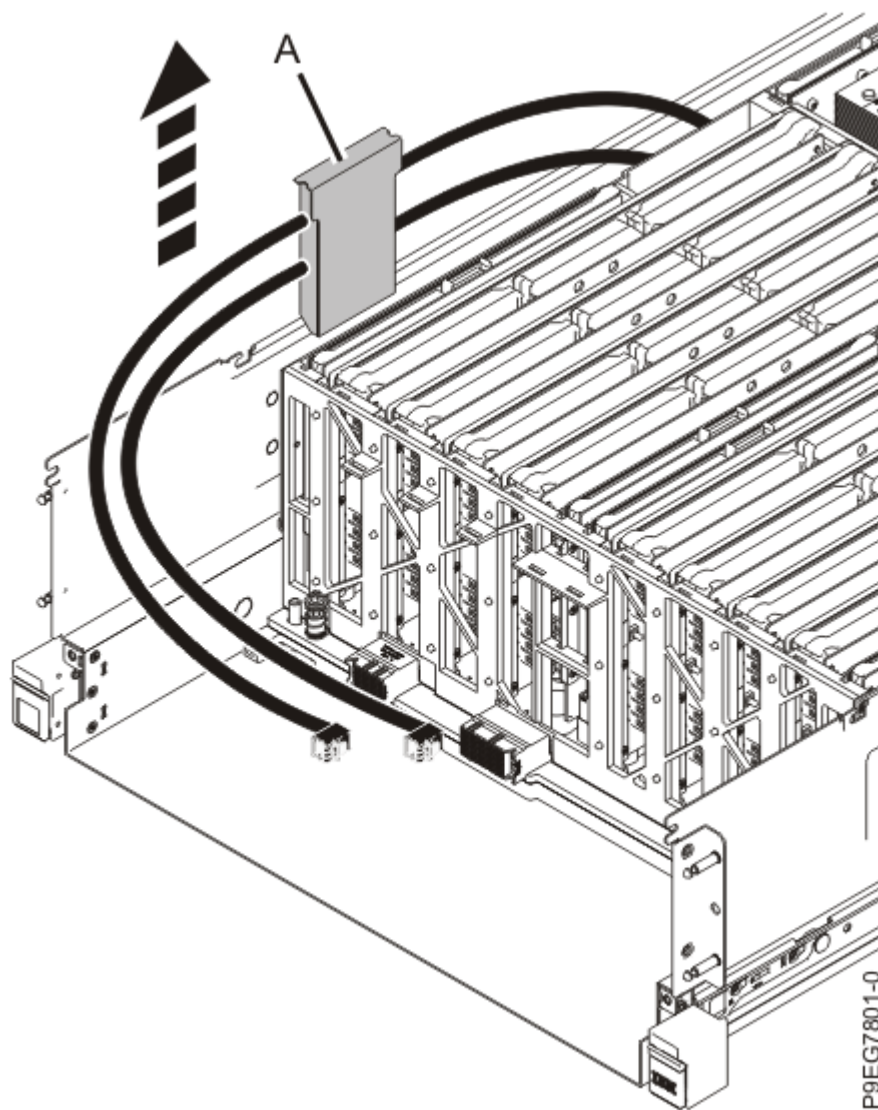
図 16. 基本機能ディスク・ドライブ・バックプレーンの SAS ケーブル・サポートの取り外し
