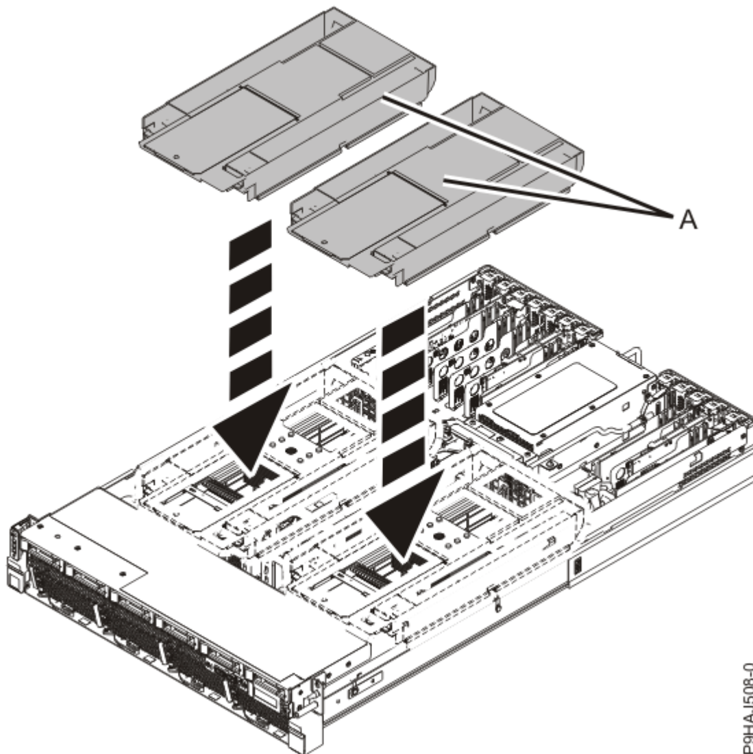
図 21. エア・バッフルの再取り付け
