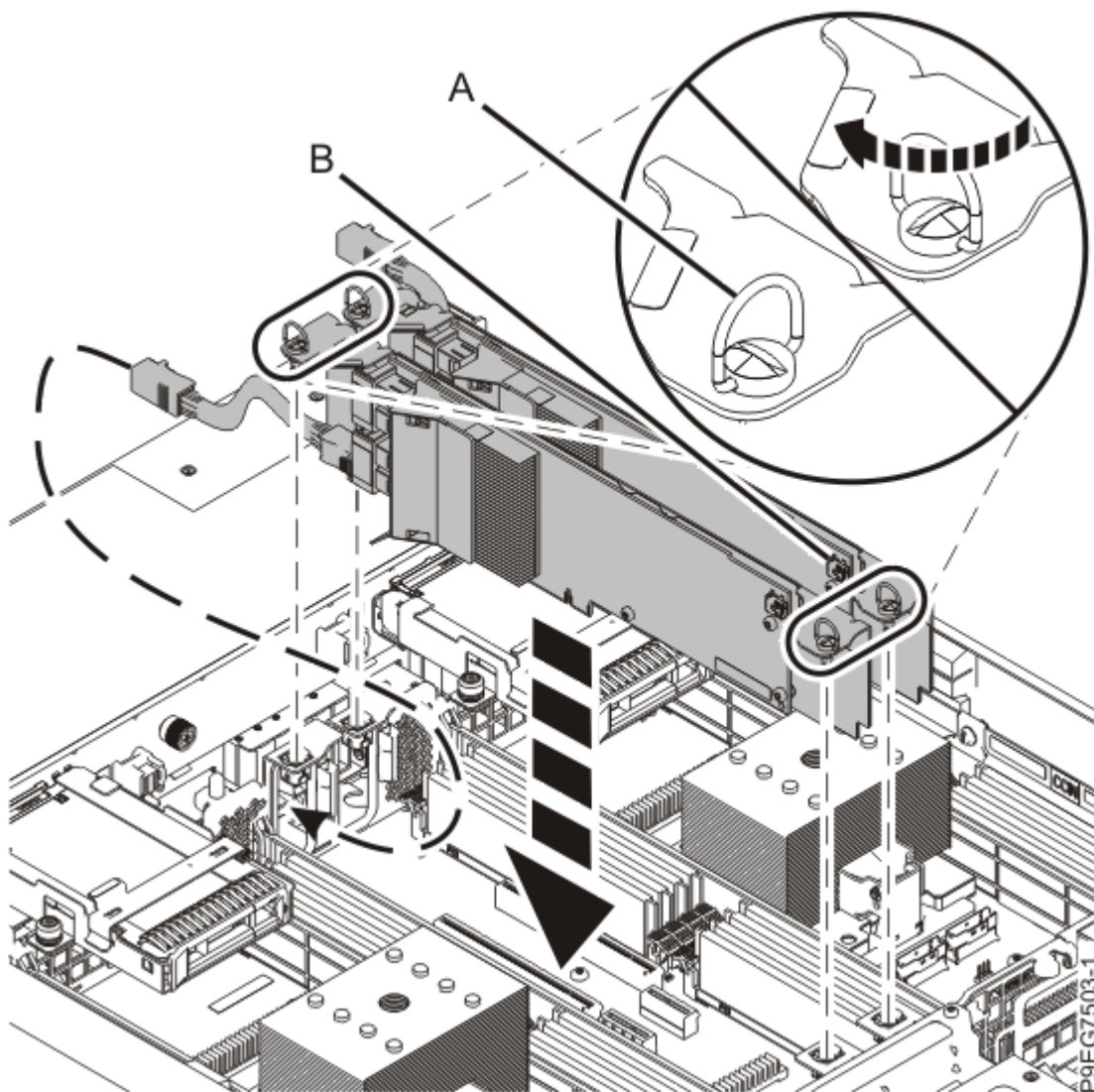
図 15. SAS RAID アダプターの再取り付け
