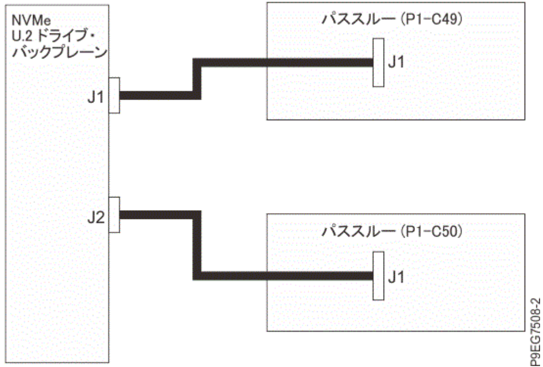
図 18. 2 つの NVMe U.2 パススルー・カードをスロット P1-C49 およびスロット P1-C50 に搭載したシステムの NVMe ケーブルの接続
