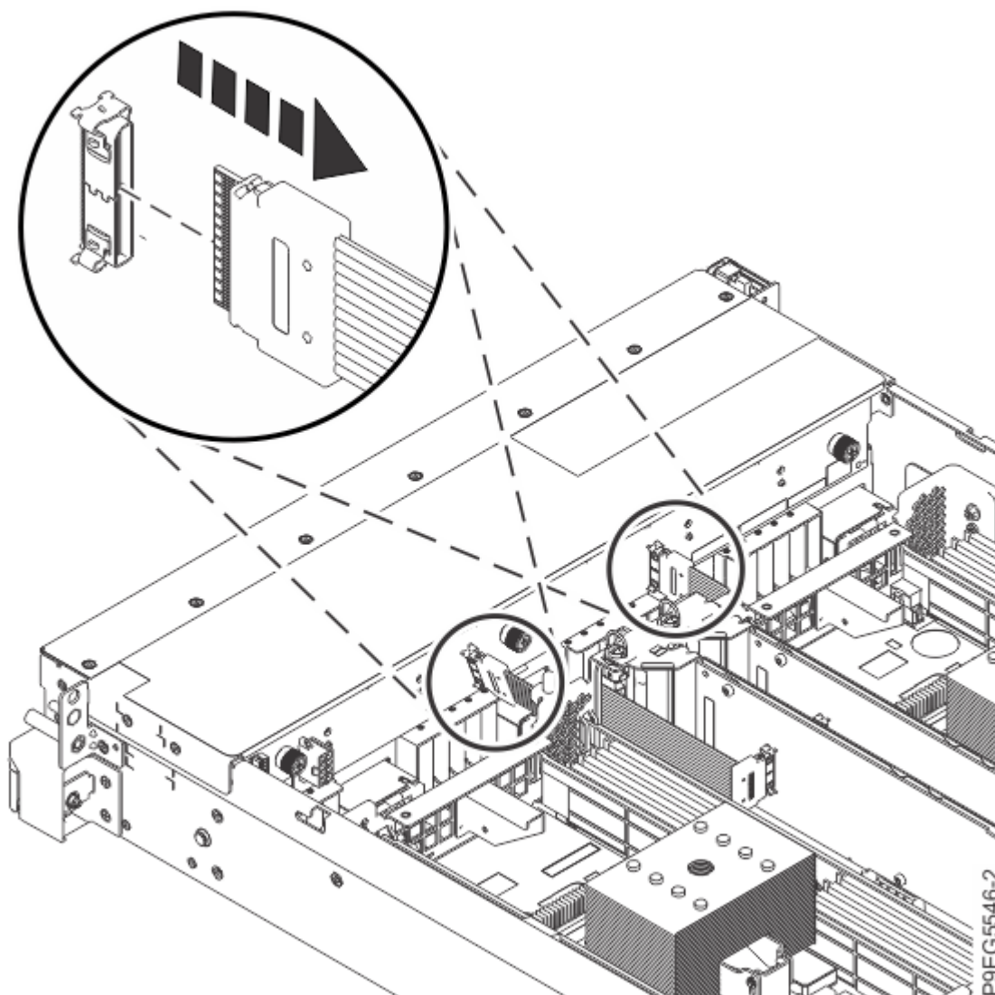
図 8. NVMe ケーブルの切り離し
