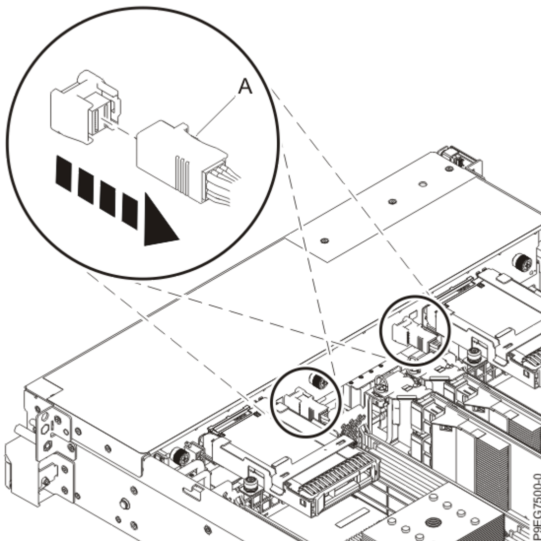
図 6. 前面 SAS ケーブルのプラグを抜く
