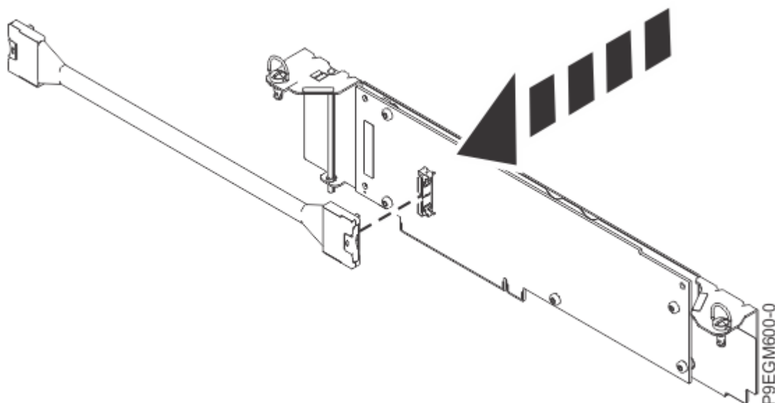
図 10. NVMe U.2 パススルー・カードからの NVMe ケーブルの切り離し
