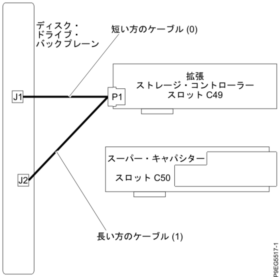
図 14. ハイパフォーマンス・ストレージ・コントローラー構成での「Y」 SAS ケーブルの再接続
