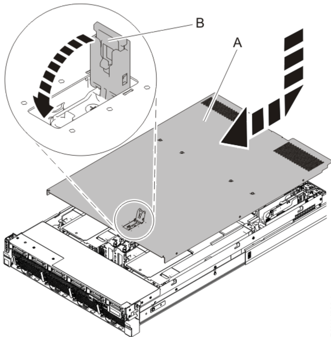
図 22. 保守アクセス・カバーの取り付け
