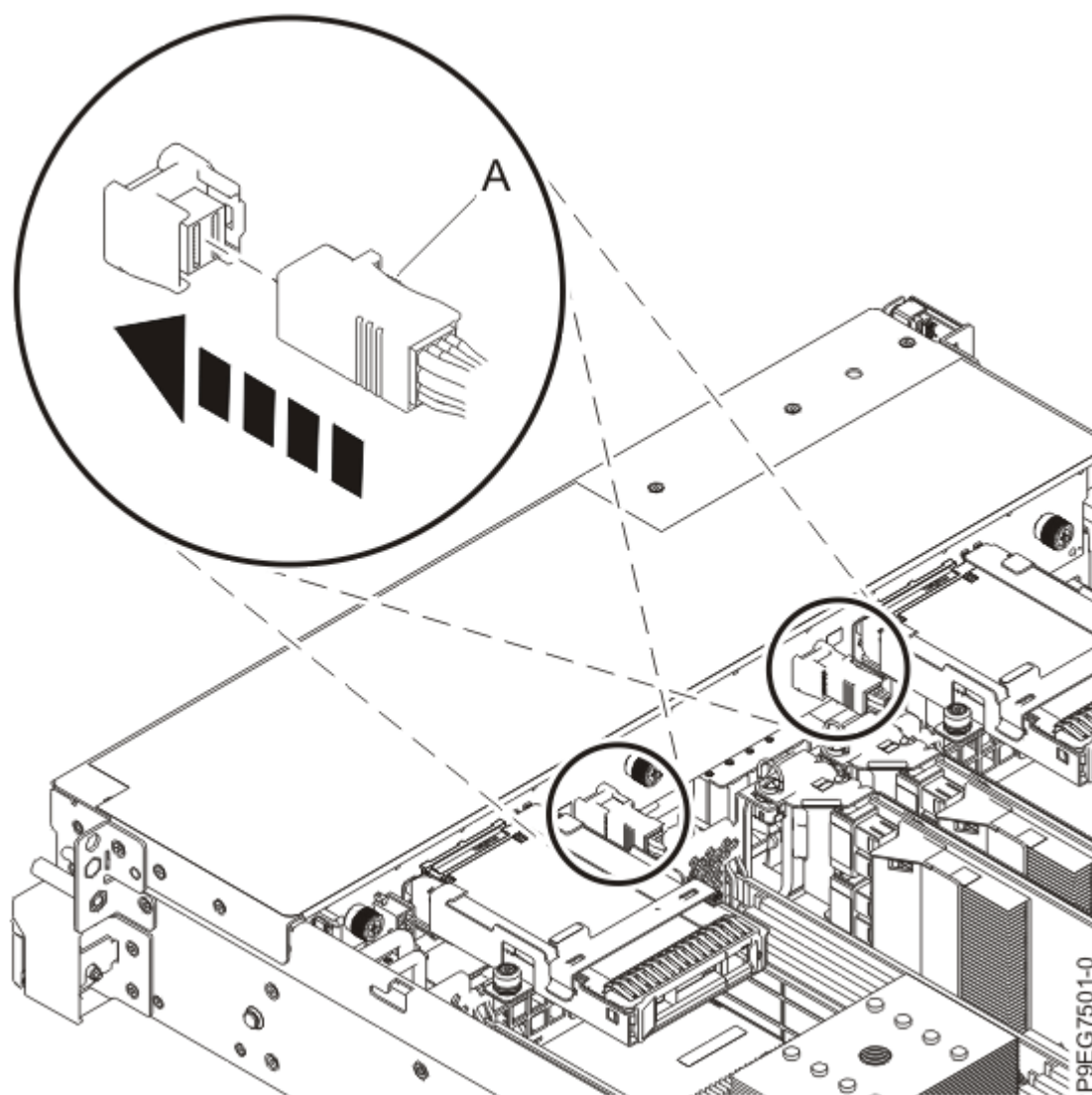
図 11. 前面 SAS ケーブルの再接続
