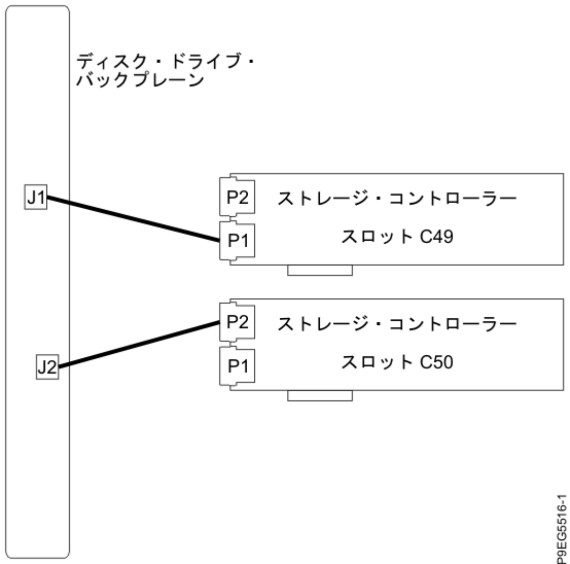
図 13. 分割ディスク構成での SAS ケーブルの再接続
