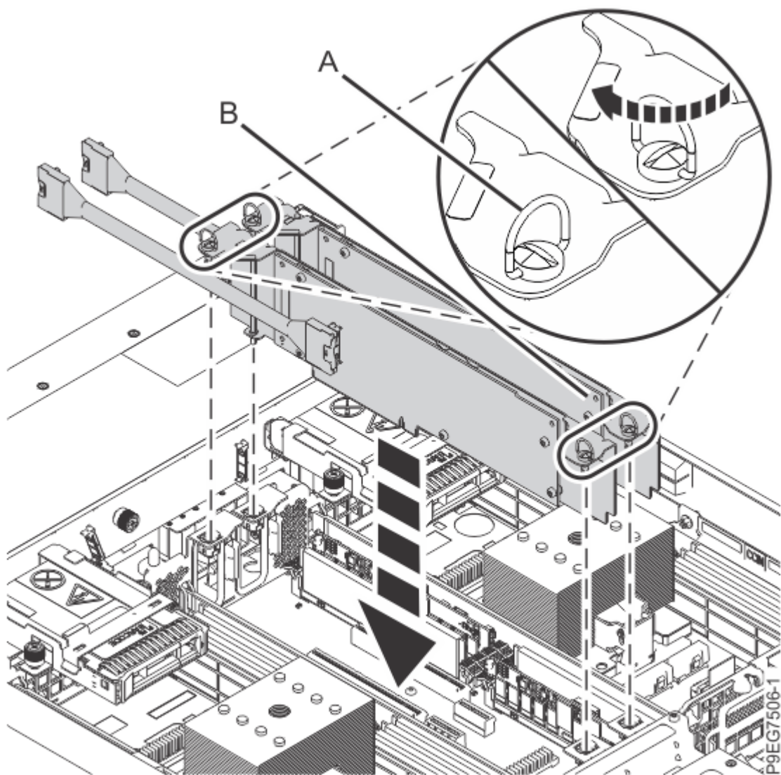
図 19. NVMe U.2 パススルー・カードの装着
