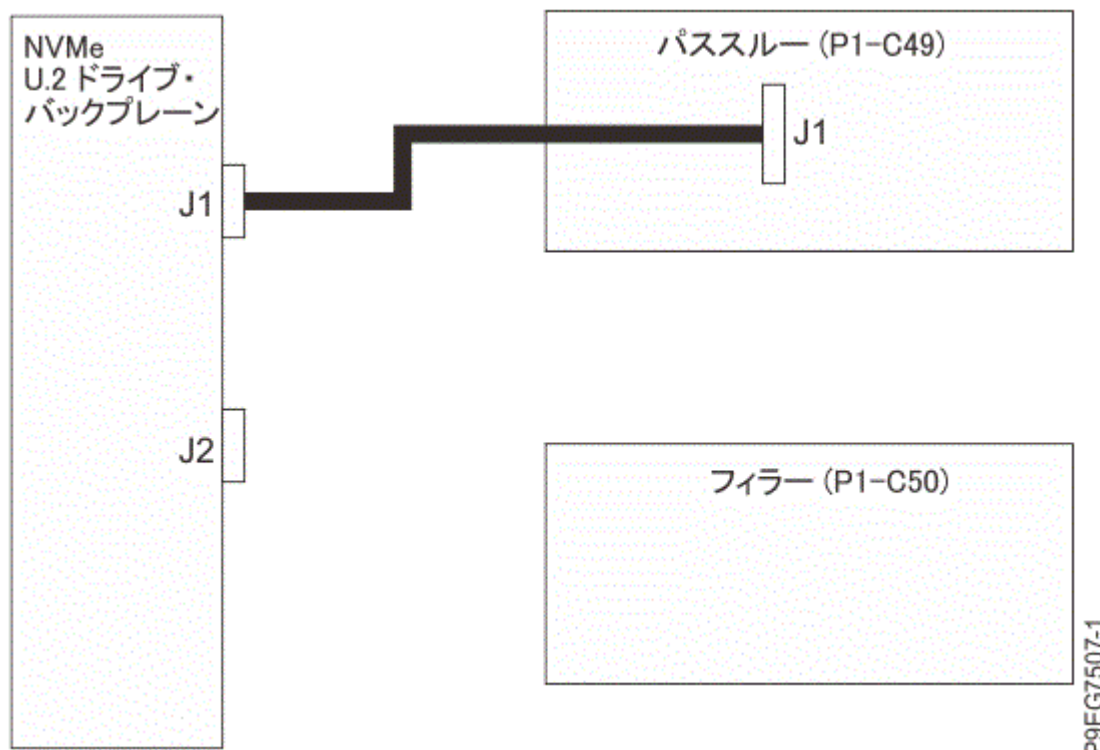
図 17. P1-C49 に 1 つの NVMe U.2 パススルー・カードを搭載し、スロット P1-C50 にフィラーを搭載したシステムの NVMe ケーブルの接続
