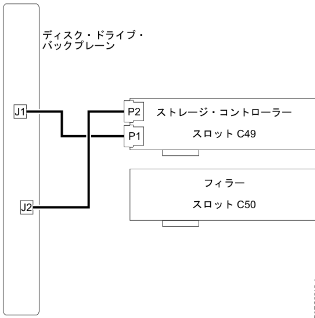
図 12. 基本ストレージ構成での SAS ケーブルの再接続
