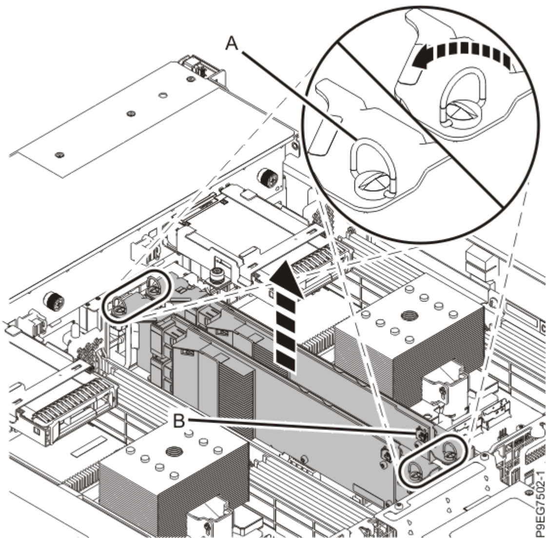
図 7. SAS RAID アダプターの取り外し
