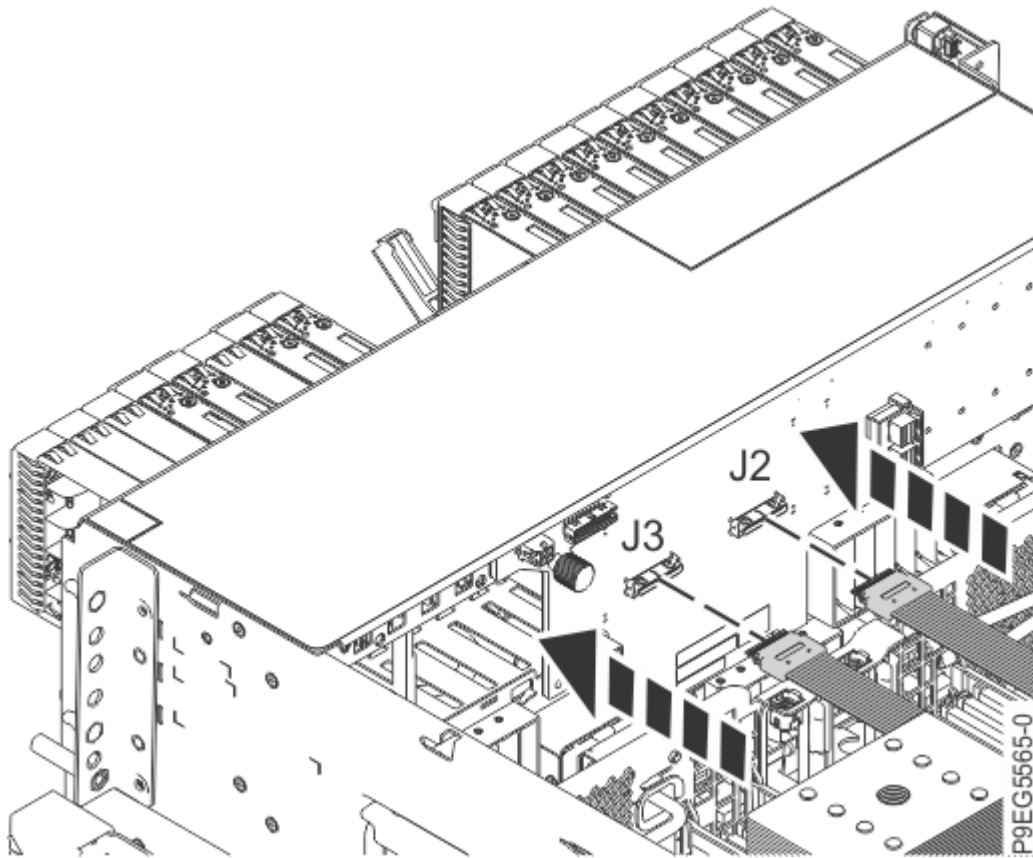
図 31. NVMe ケーブルの再接続
