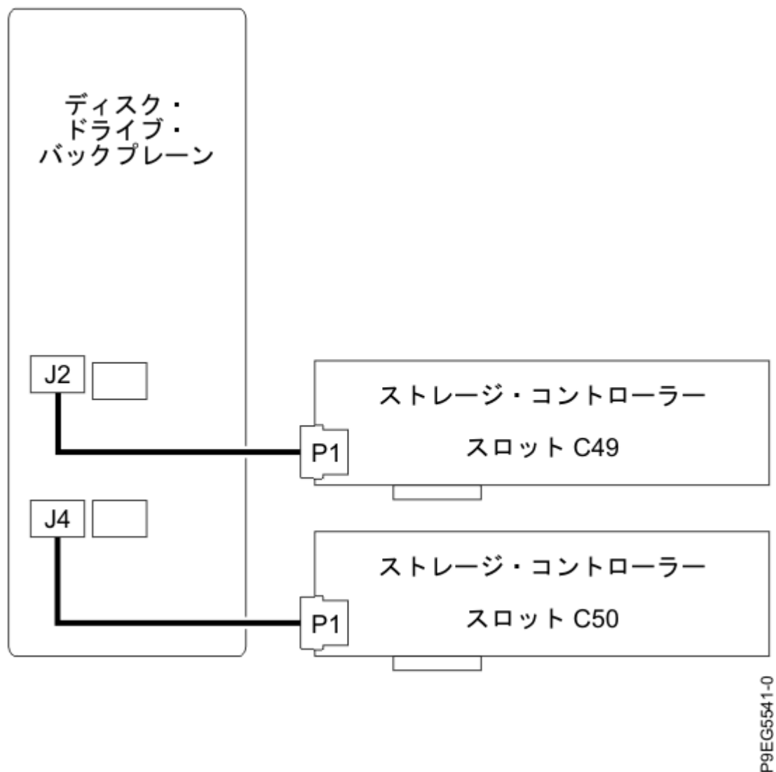
図 23. 18 ドライブ拡張機能 構成での SAS ケーブルの再接続
