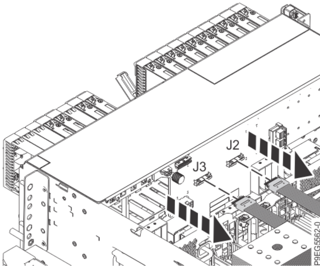
図 14. NVMe ケーブルの切り離し
