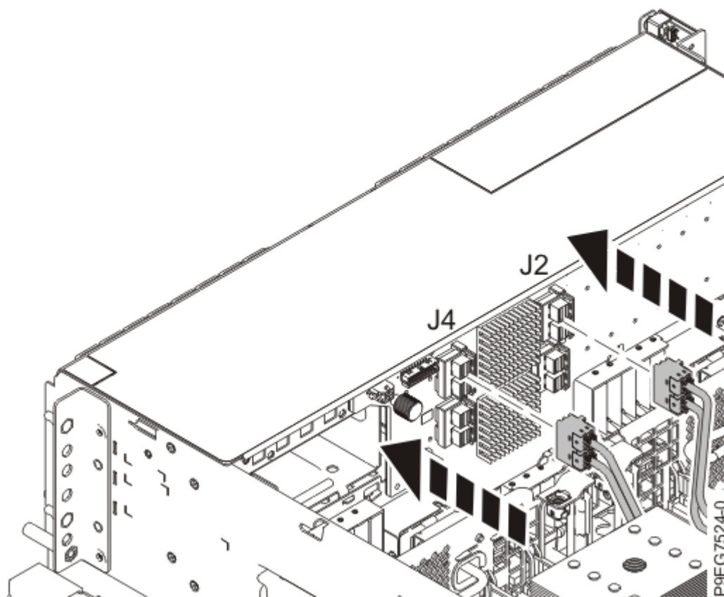
図 18. 12 ドライブ拡張機能ディスク・ドライブ・バックプレーンまたは 18 ドライブ拡張機能ディスク・ドライブ・バックプレーンの前面 SAS ケーブルの再接続
