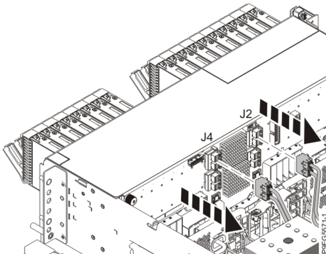
図 11. 18 ドライブ拡張機能 ディスク・ドライブ・バックプレーンから前面 SAS ケーブルを切り離す
