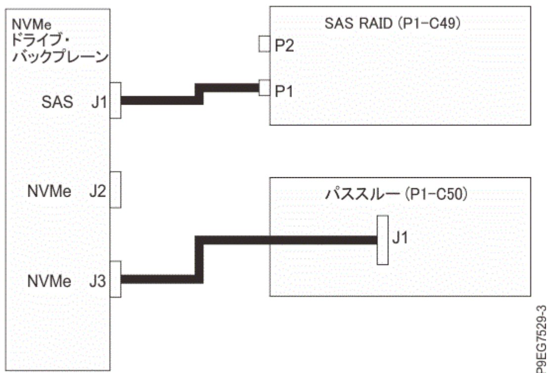
図 29. スロット P1-C49 に 1 つの SAS RAID 内部アダプターを搭載し、スロット P1-C50 に 1 つの NVMe U.2 パススルー・カードを搭載したシステムの NVMe ケーブルの接続
