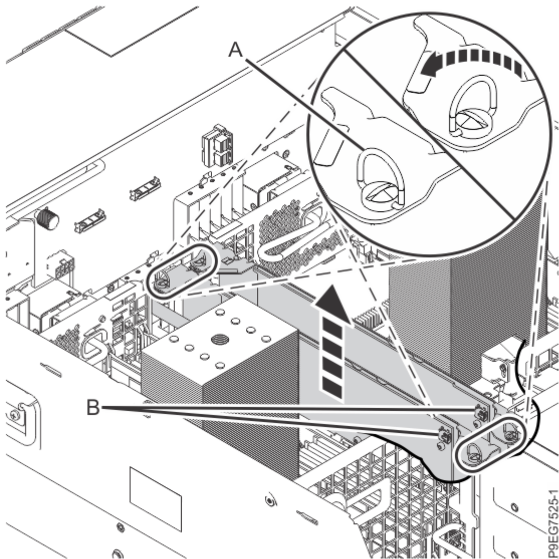
図 15. NVMe U.2 パススルー・カードの取り外し
