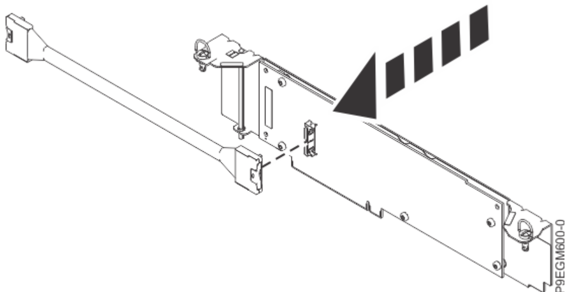
図 16. NVMe U.2 パススルー・カードからの NVMe ケーブルの切り離し
