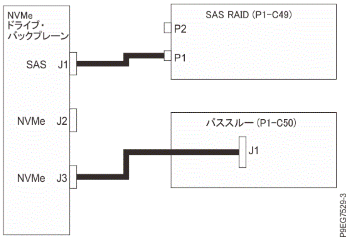
図 24. NVMe ドライブ・バックプレーン構成での SAS ケーブルの再接続
