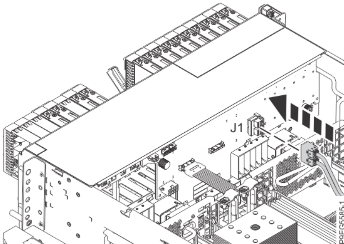
図 19. NVMe ドライブ・バックプレーンの前面 SAS ケーブルの再接続
