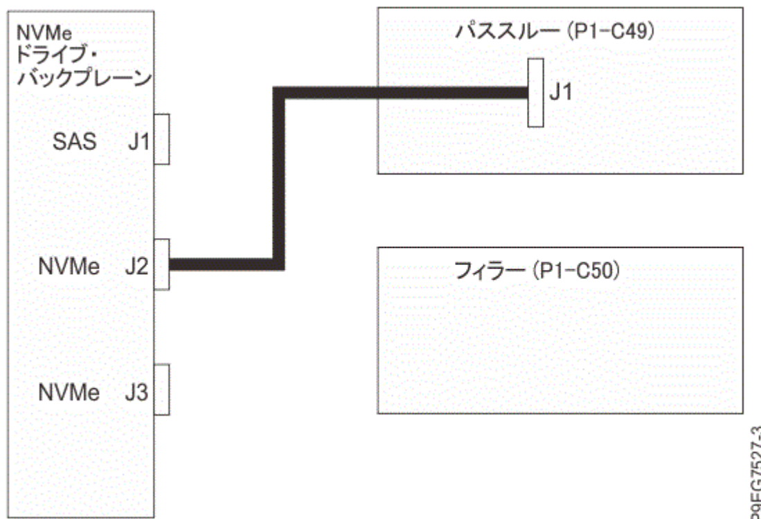
図 27. P1-C49 に 1 つの NVMe U.2 パススルー・カードを搭載し、スロット P1-C50 にフィラーを搭載したシステムの NVMe ケーブルの接続
