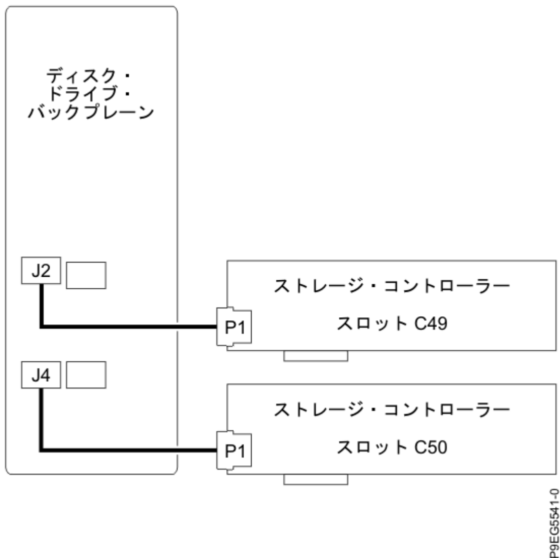
図 22. 12 ドライブ拡張機能 構成での SAS ケーブルの再接続
