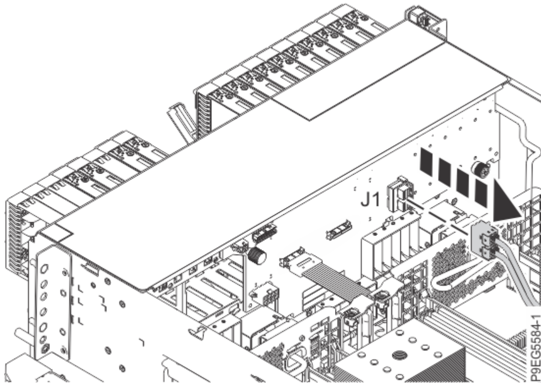
図 12. NVMe バックプレーンから前面 SAS ケーブルを切り離す
