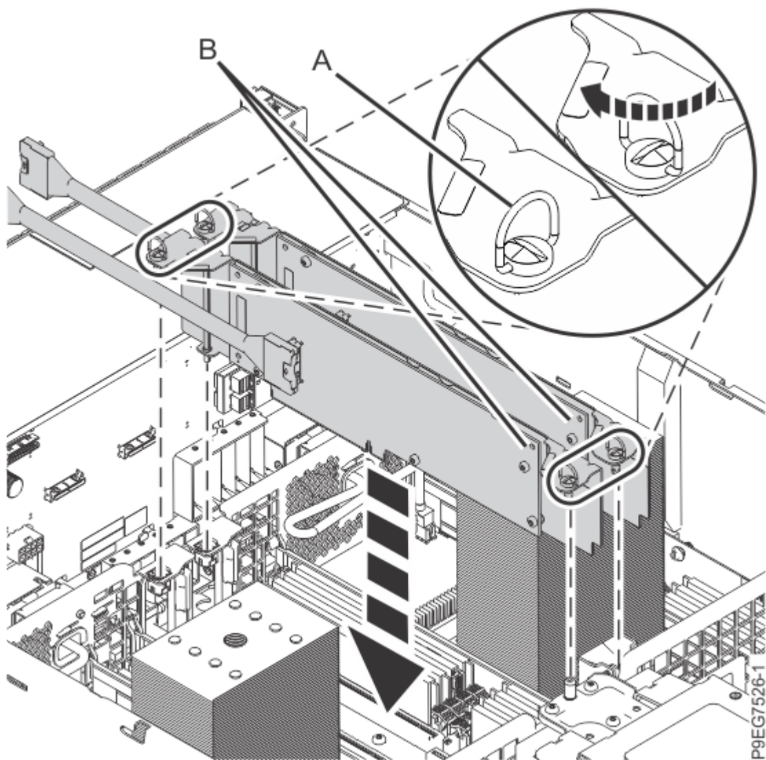
図 30. NVMe U.2 パススルー・カードの装着
