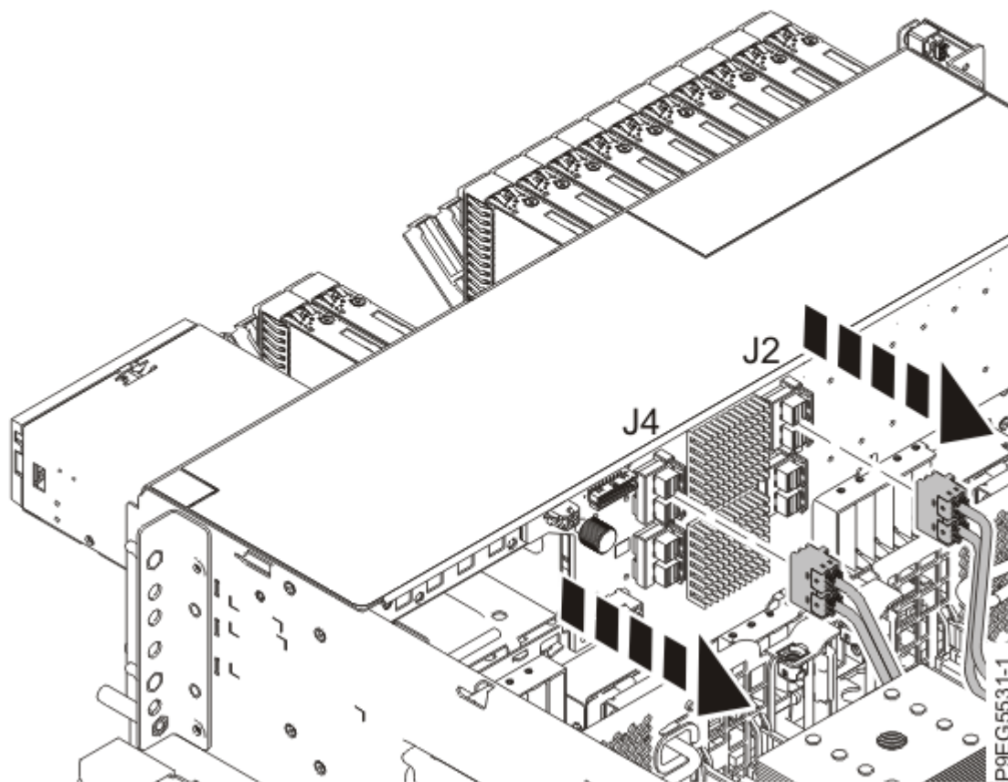
図 10. 12 ドライブ拡張機能 ディスク・ドライブ・バックプレーンから前面 SAS ケーブルを切り離す
