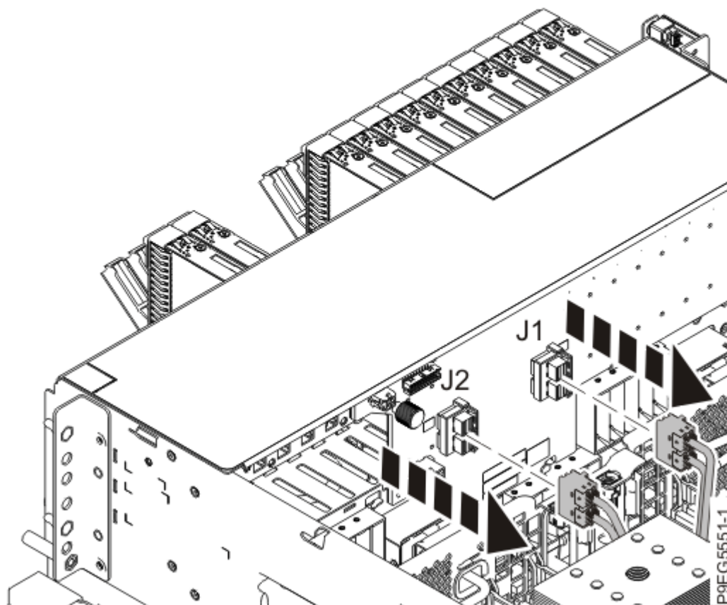
図 9. 基本機能 ディスク・ドライブ・バックプレーンから前面 SAS ケーブルを切り離す
