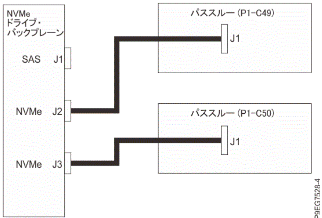
図 28. 2 つの NVMe U.2 パススルー・カードをスロット P1-C49 およびスロット P1-C50 に搭載したシステムの NVMe ケーブルの接続
