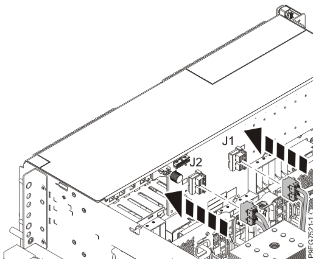
図 17. 基本機能ディスク・ドライブ・バックプレーンの前面 SAS ケーブルの再接続
