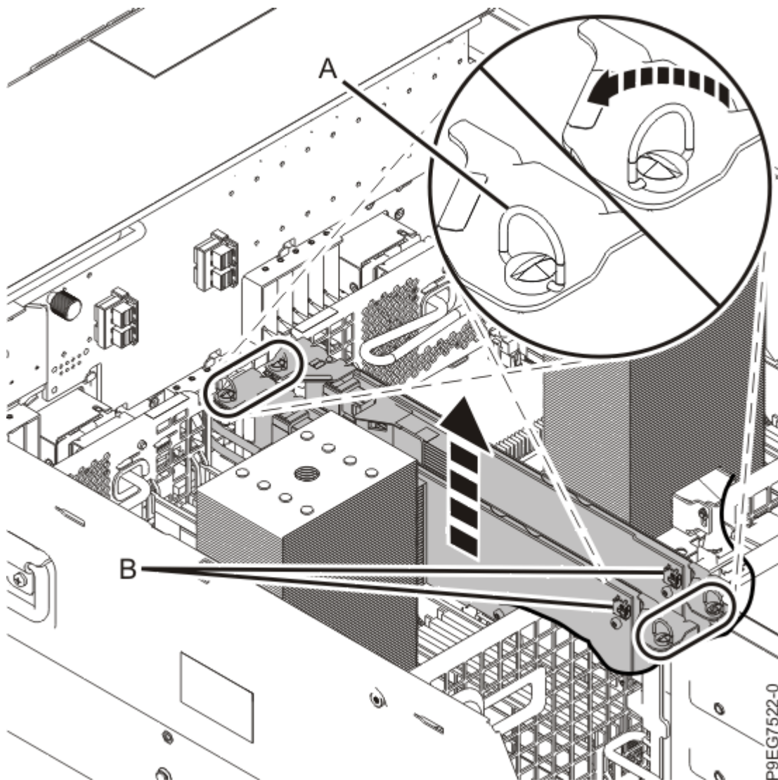
図 13. SAS RAID アダプターの取り外し
