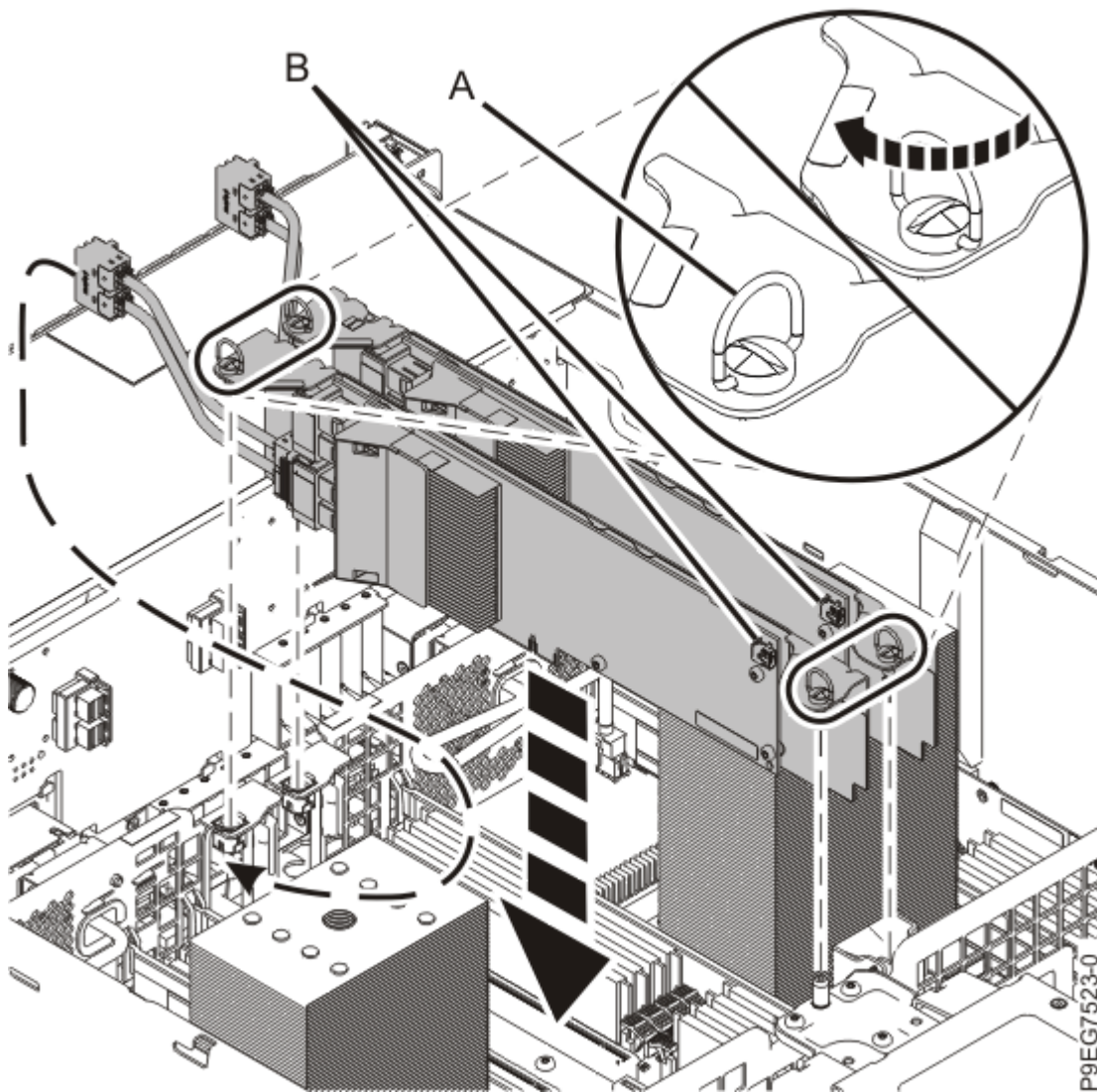
図 25. SAS RAID アダプターの取り替え
