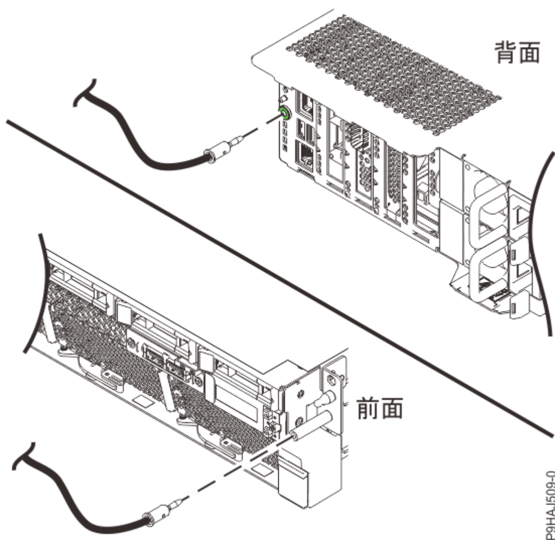
図 3. ESD プラグの位置
