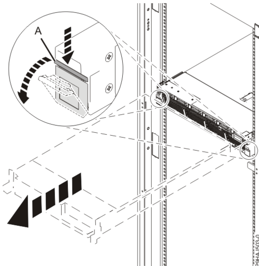
図 28. サイド・ラッチのリリース
