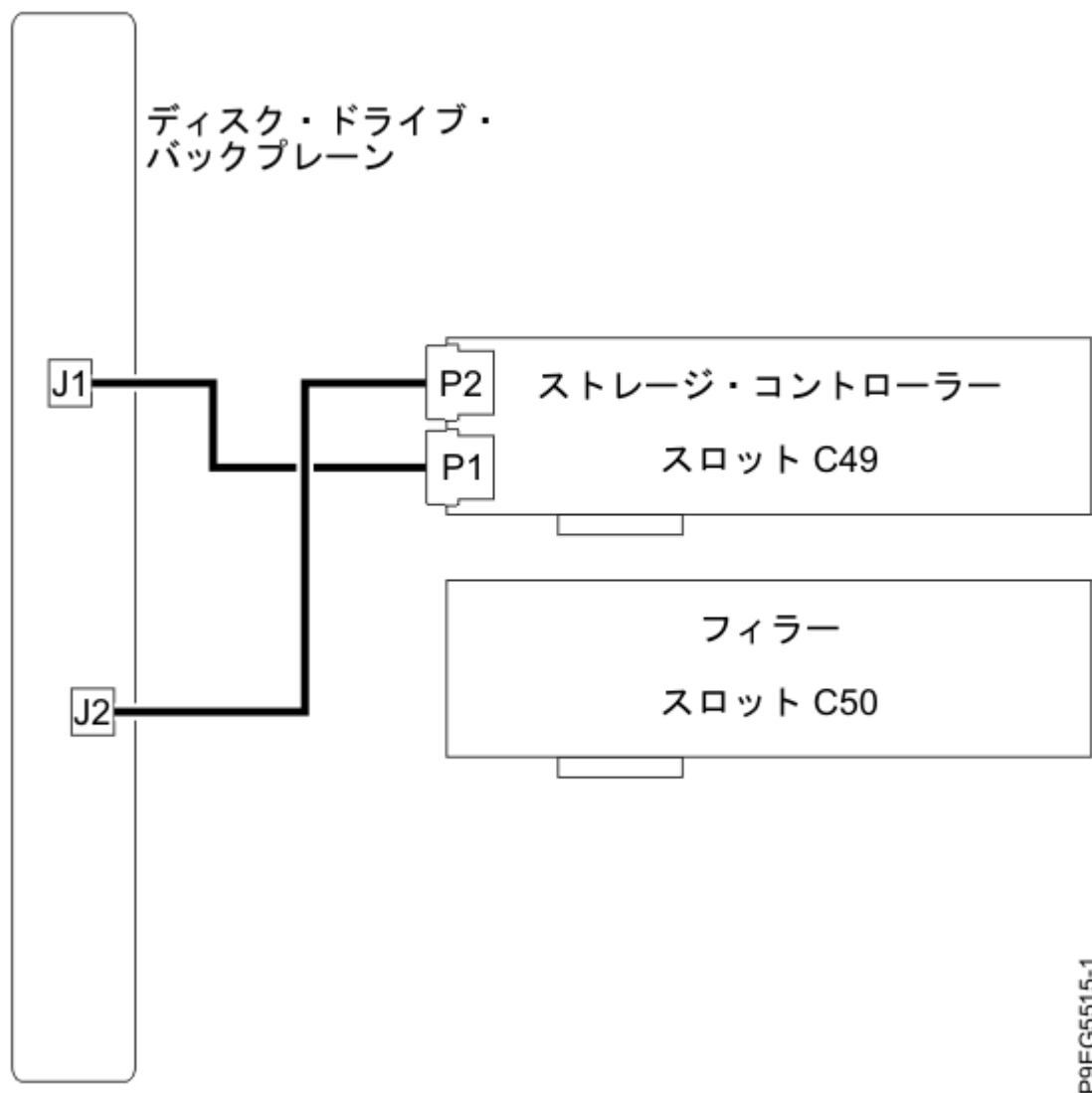
図 17. 基本ストレージ構成での SAS ケーブルの再接続
