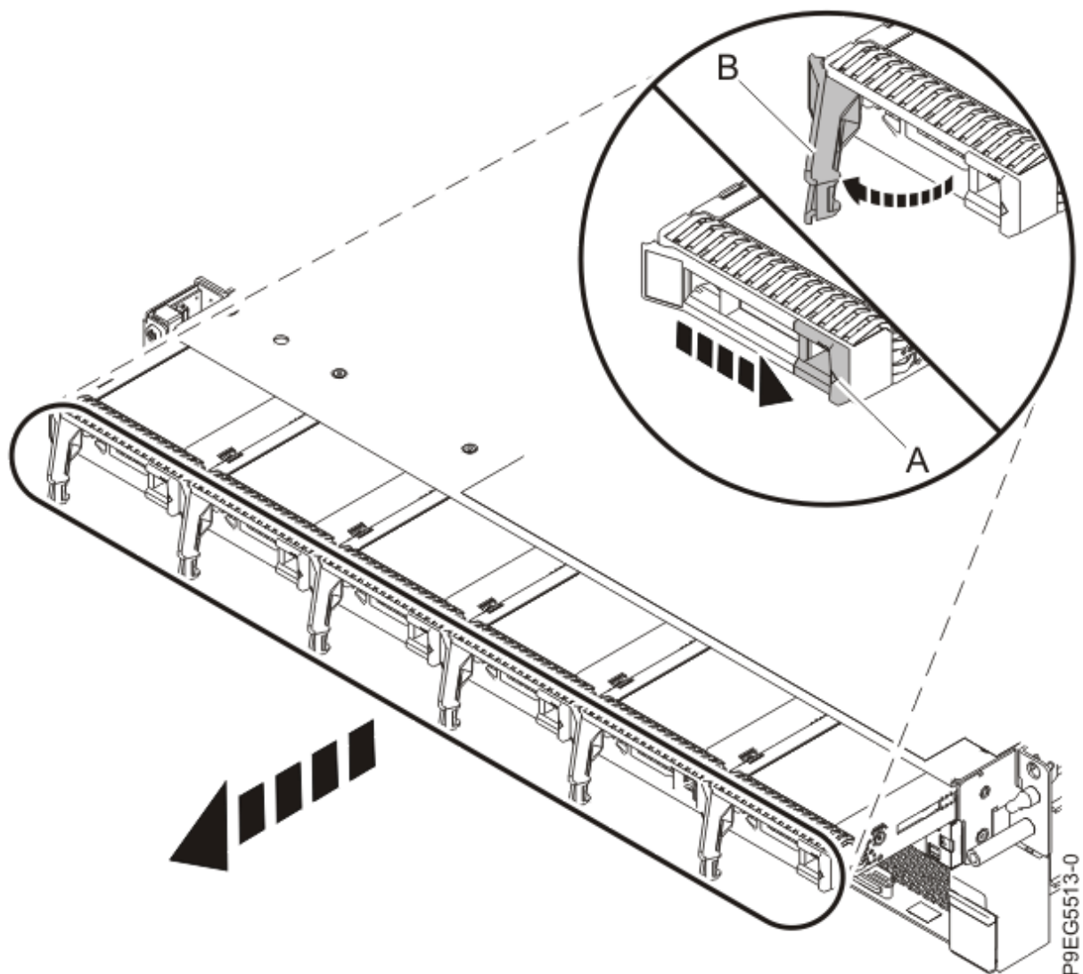
図 10. 前面ドライブの部分的な取り外し
