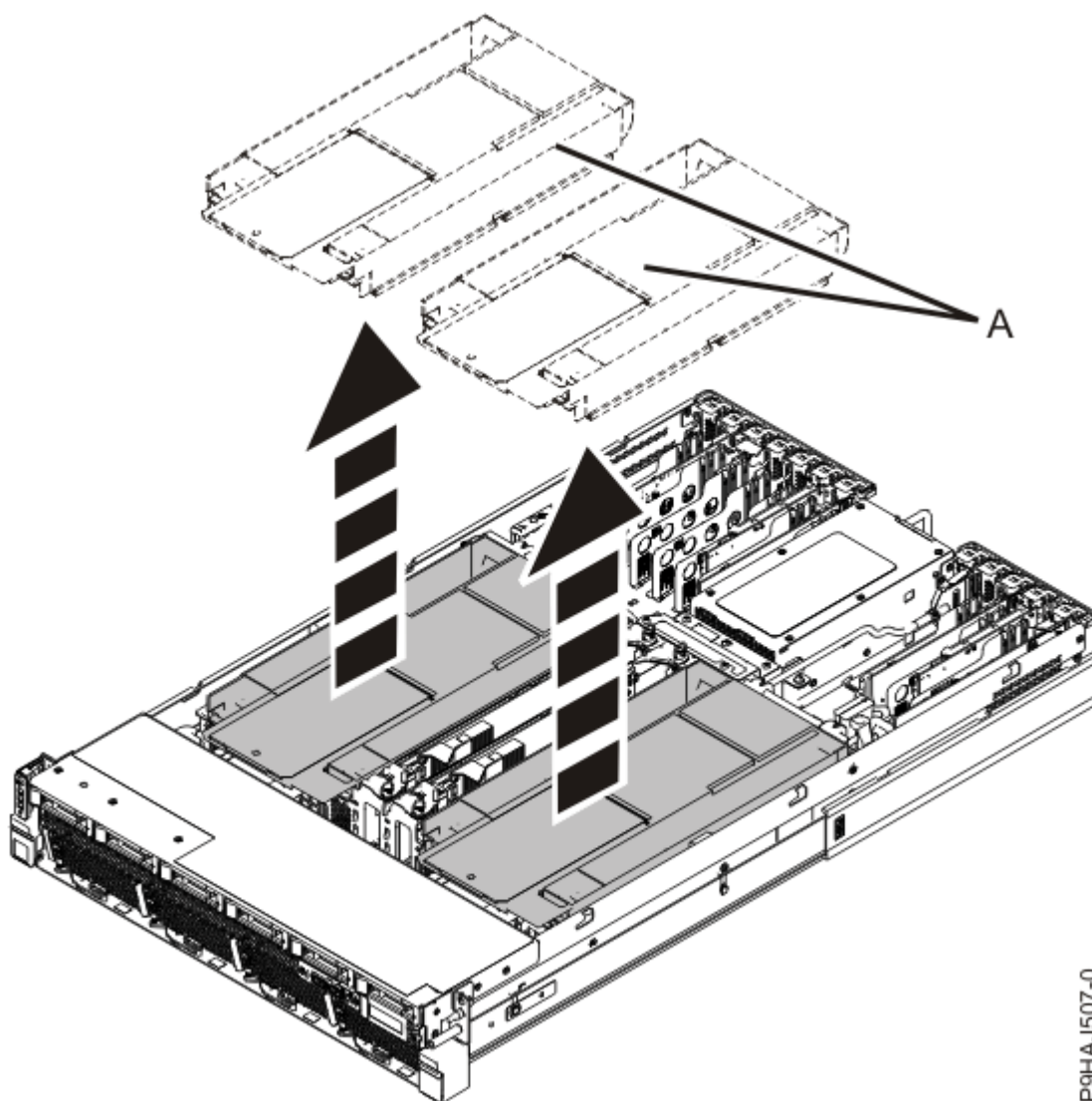
図 31. エア・バッフルの取り外し
