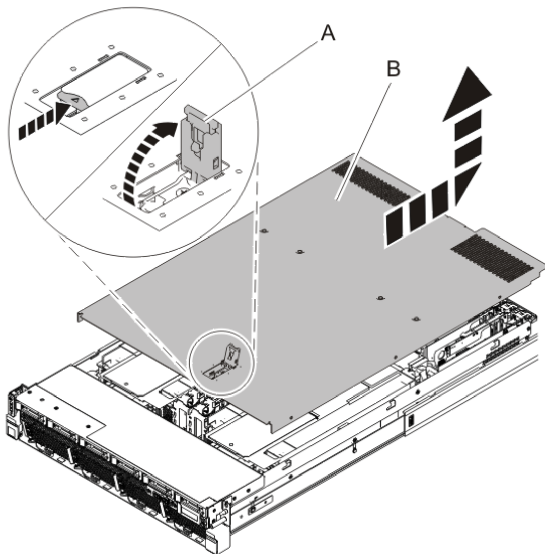
図 39. 保守アクセス・カバーの取り外し
