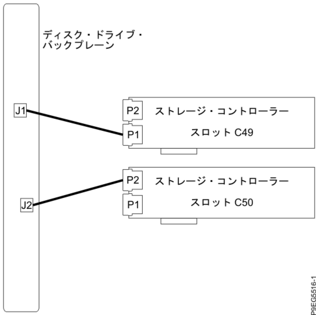
図 18. 分割ディスク構成での SAS ケーブルの再接続
