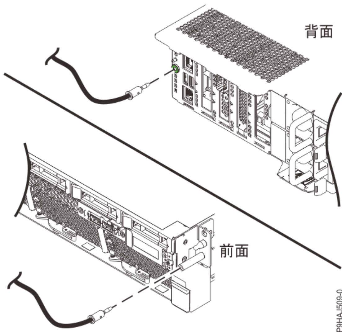
図 29. ESD プラグの位置
