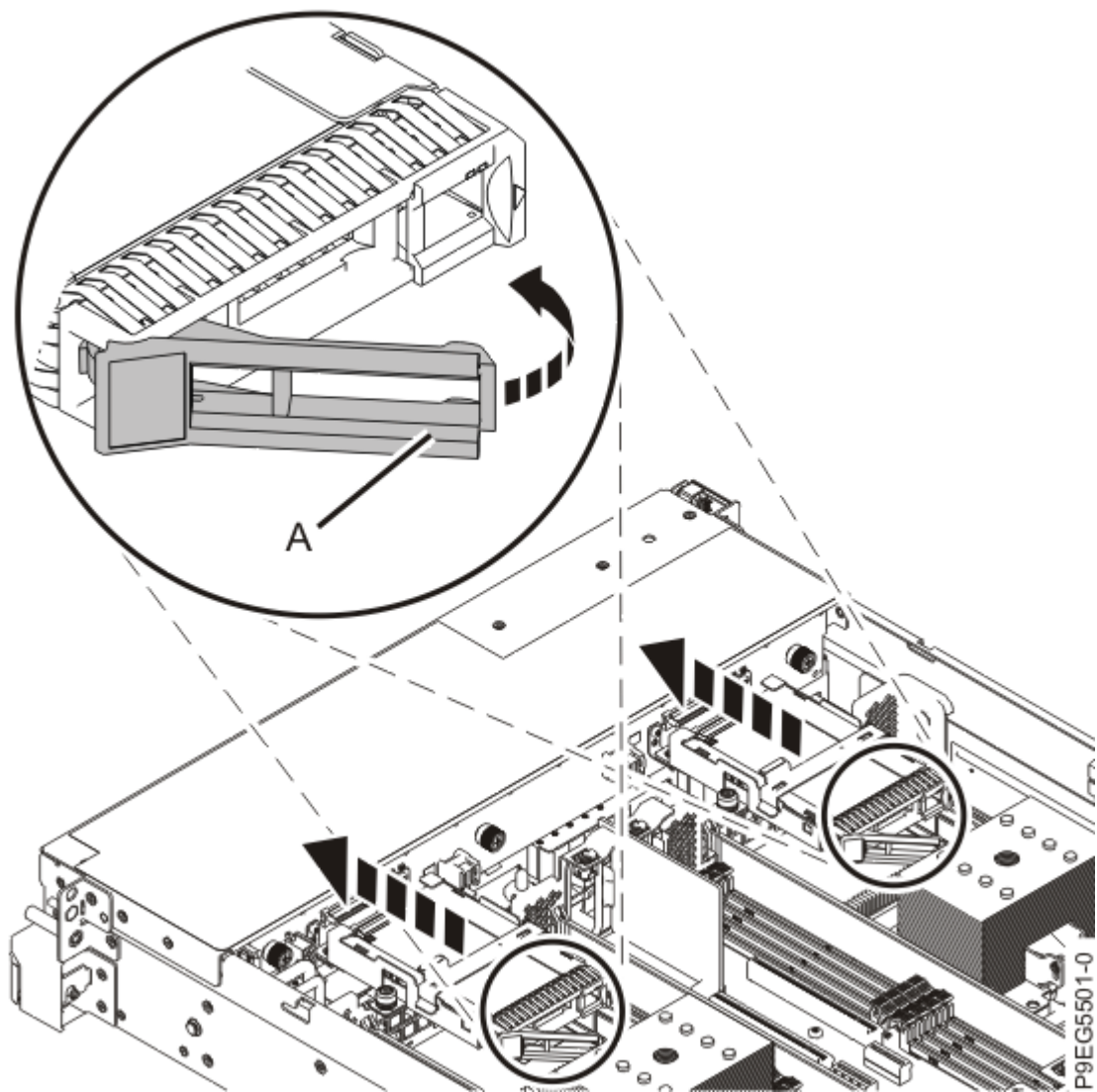
図 23. ドライブのラッチの固定
