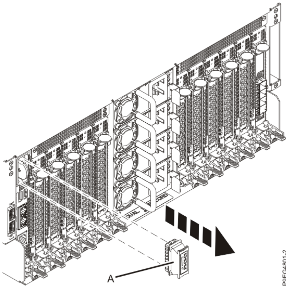
図 1. 時刻バッテリーのカバーの取り外し
