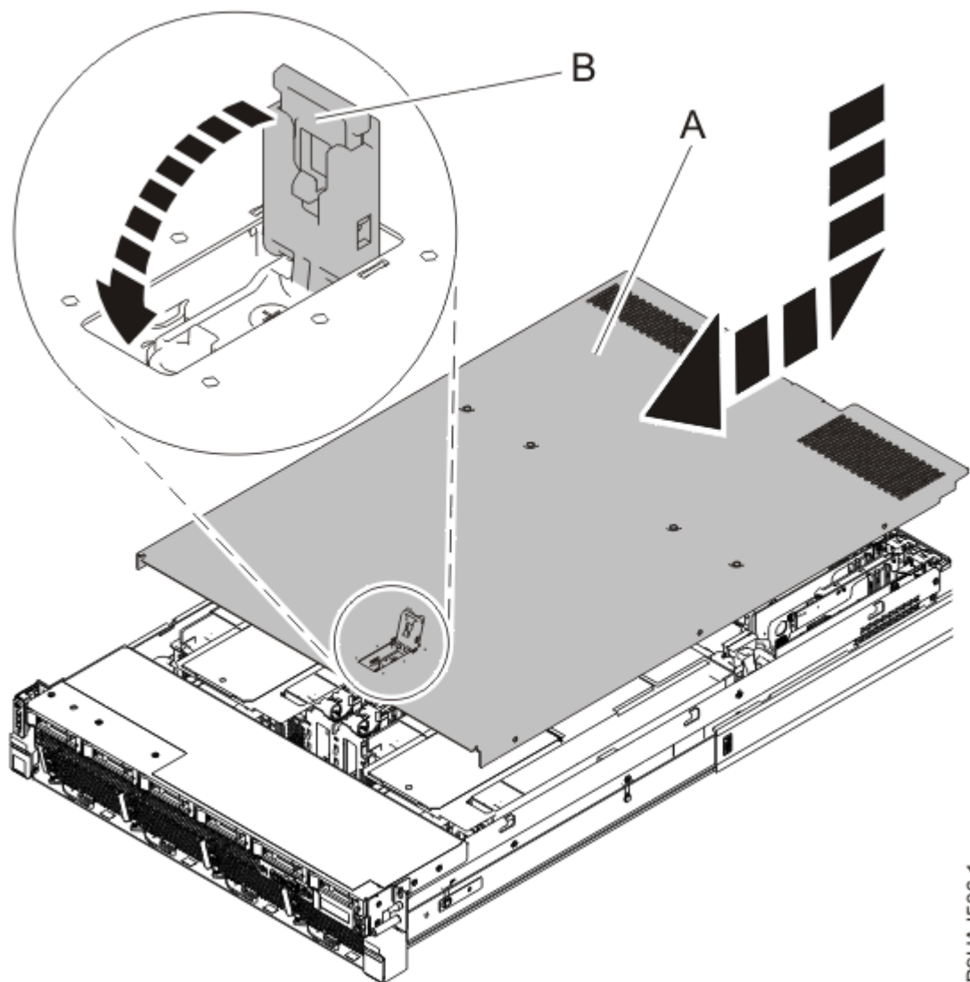
図 7. 保守アクセス・カバーの取り付け
