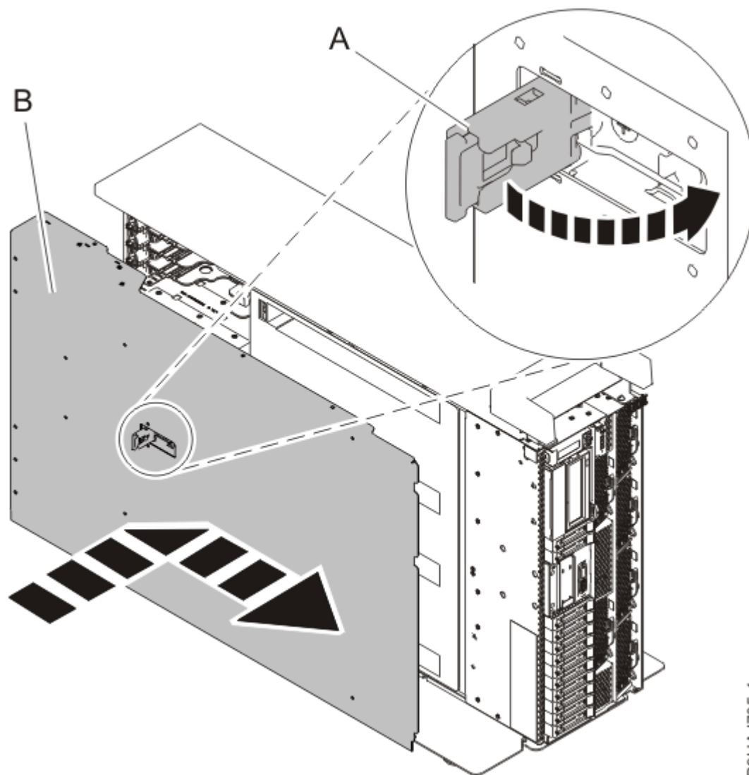
図 12. 保守アクセス・カバーの取り付け
