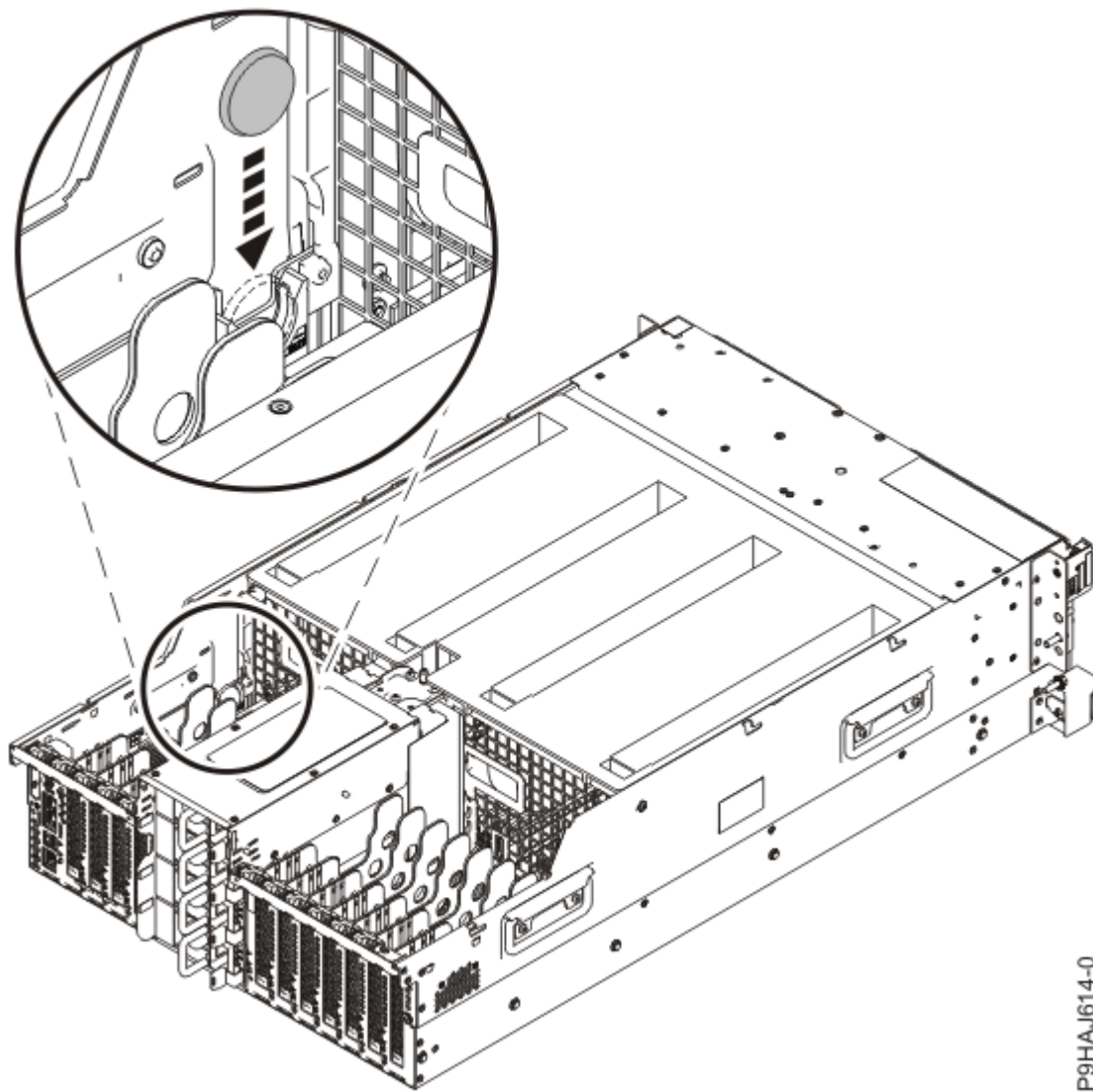
図 9. ラック・マウント型システムの時刻バッテリーの取り付け
