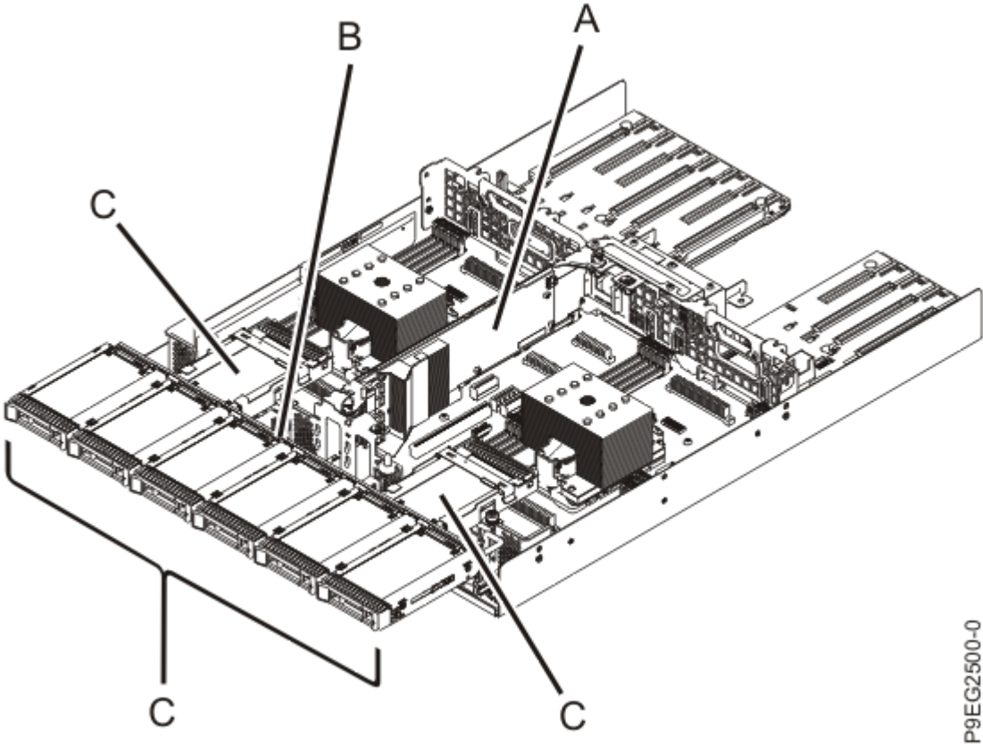
図 1. 基本機能ストレージ構成 9008-22L、9009-22A、または 9223-22H システムの SAS サブシステム部品
