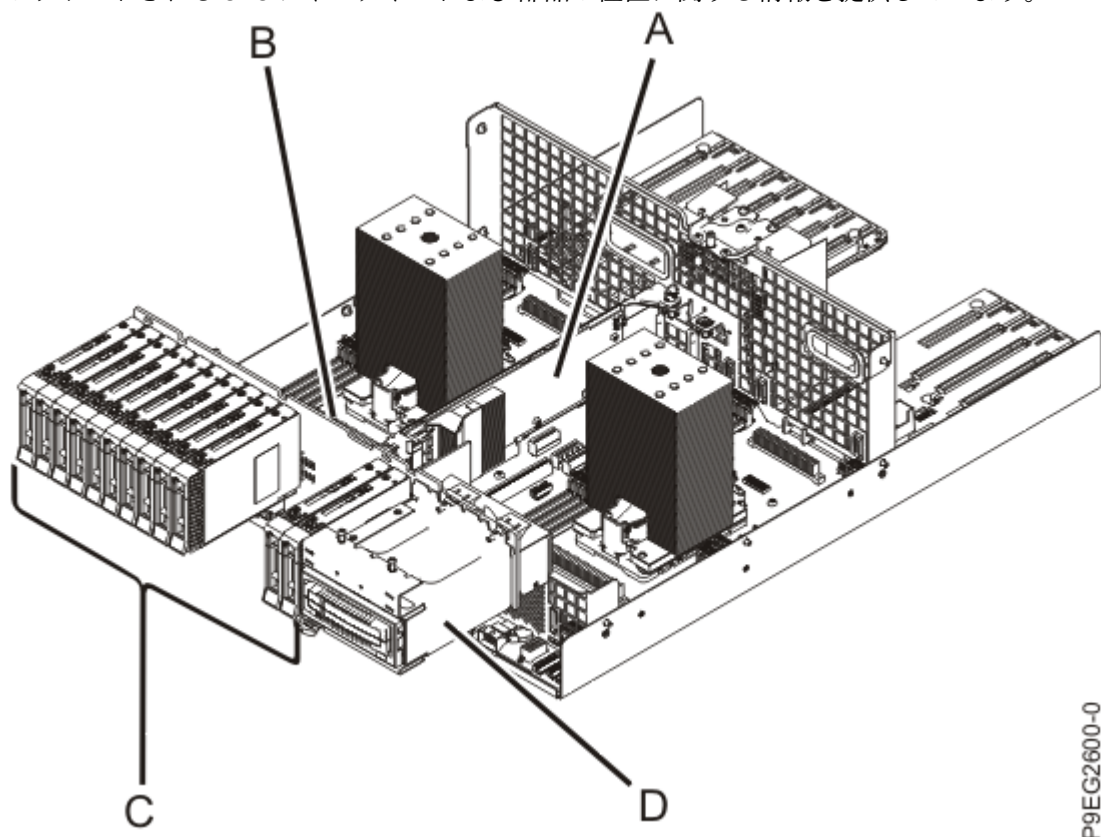
図 2. 基本機能ストレージ構成 9009-41A、9009-42A、または 9223-42H システムの SAS サブシステム部品
