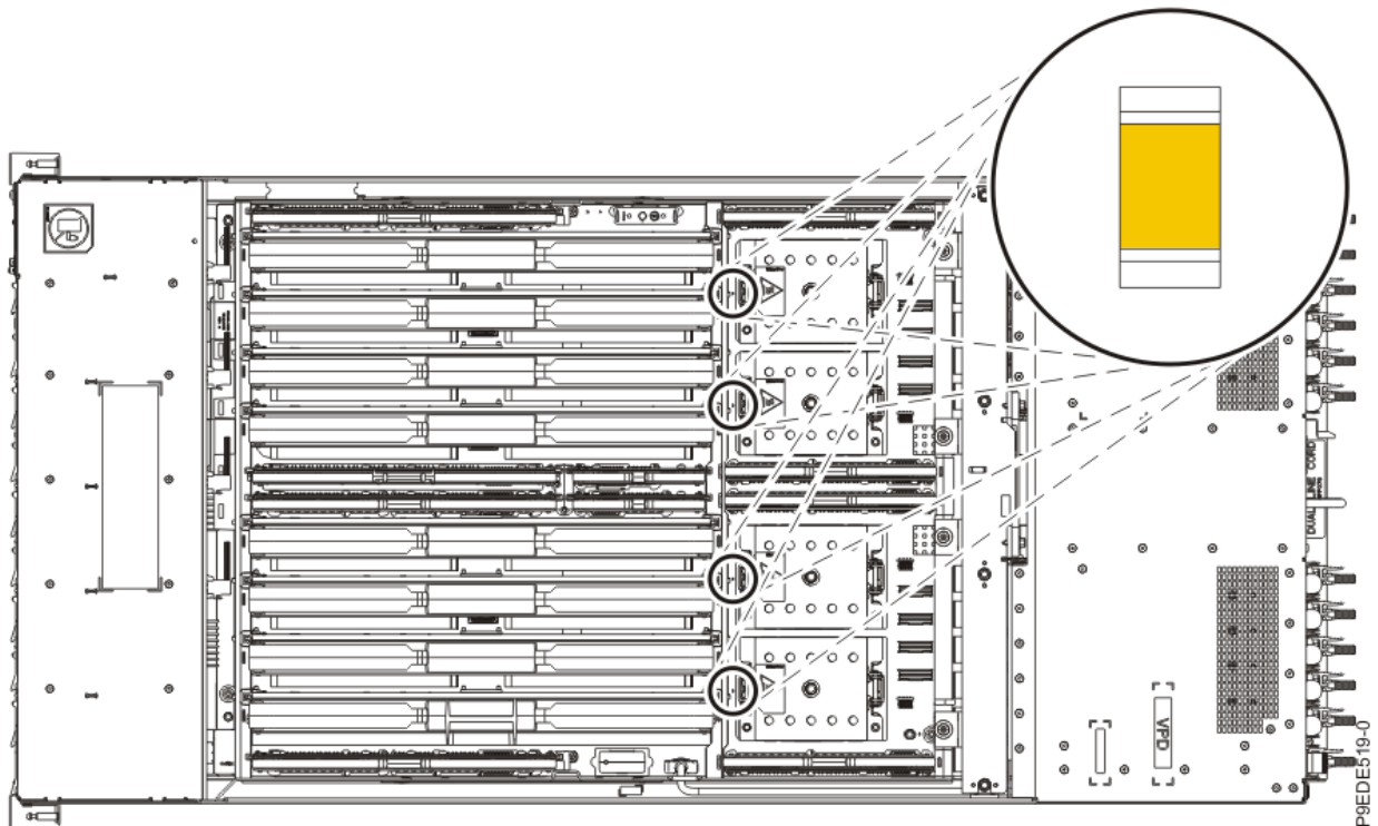
図 5. システム・プロセッサ・モジュールの LED
