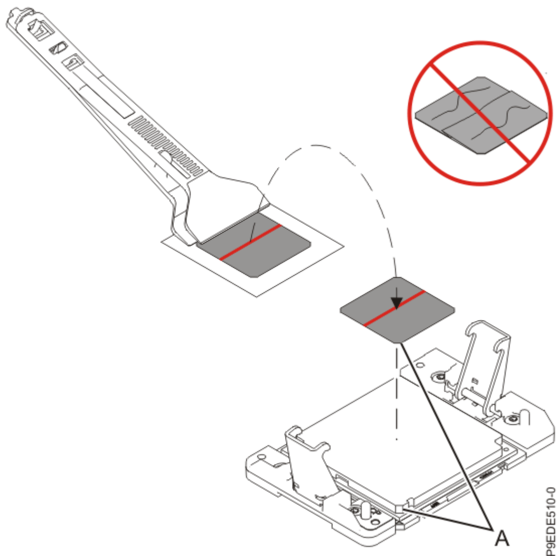
図 19. システム・プロセッサ・モジュールへの銀色の TIM の取り付け e) ヒート・シンクを TIM の上に置きます (23 ページの図 20 を参照)。
