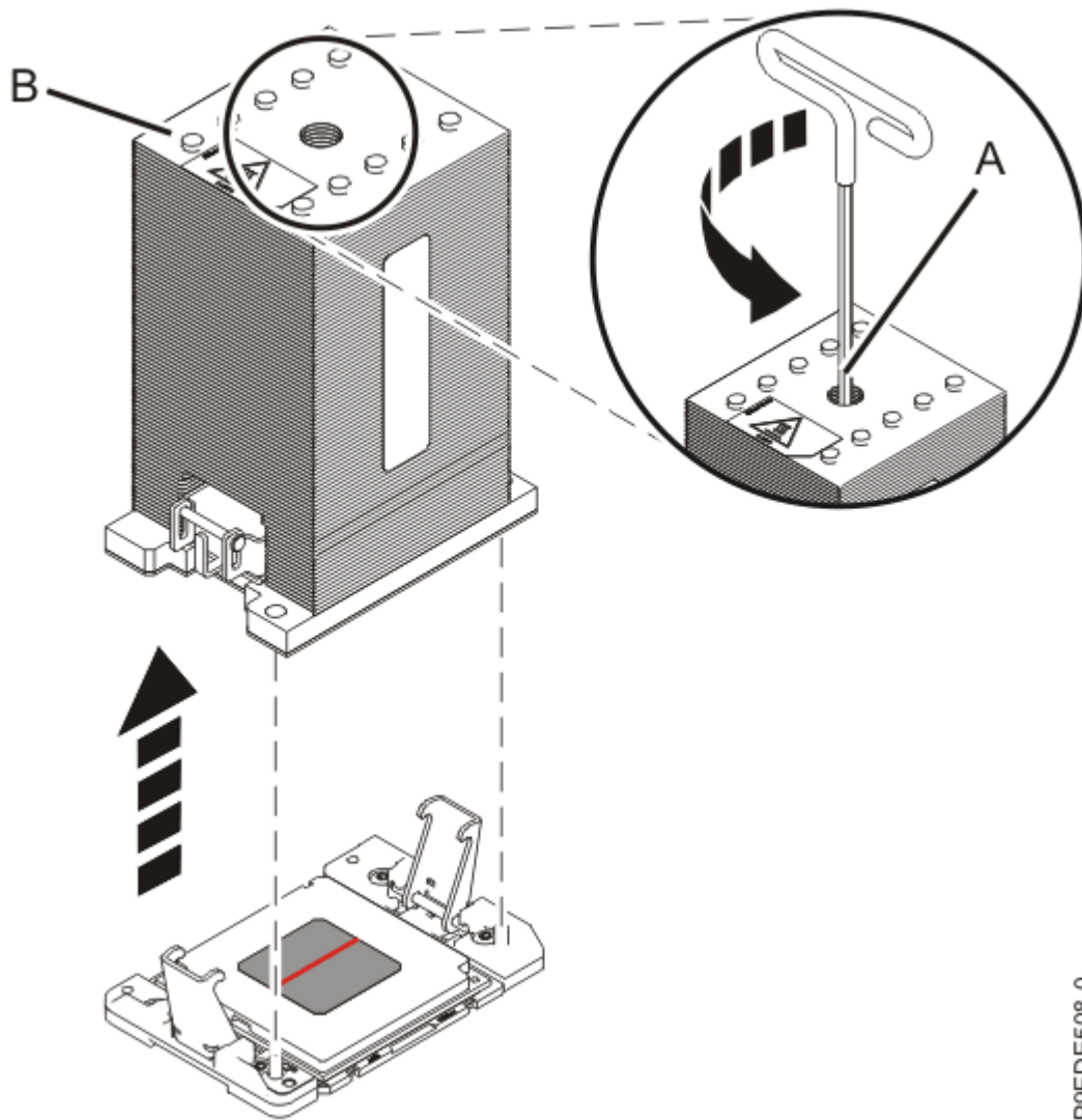
図 7. ヒート・シンクの取り外し
