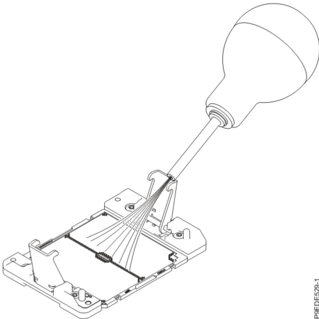
図 16. システム・プロセッサ・ソケットからほこりやごみを除去
