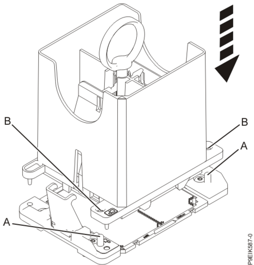
図 17. システム・プロセッサ・モジュールの取り付け
