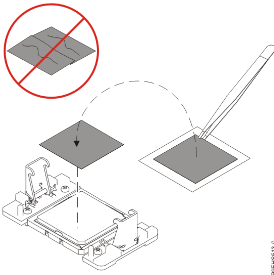
図 21. システム・プロセッサ・モジュールへの新規 TIM の取り付け
