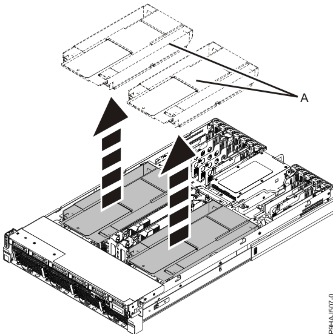
図 4. エア・バッフルの取り外し
