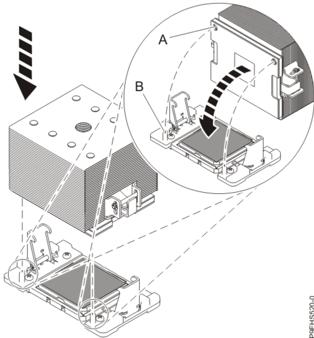
図 22. TIM へのヒート・シンクの取り付け
