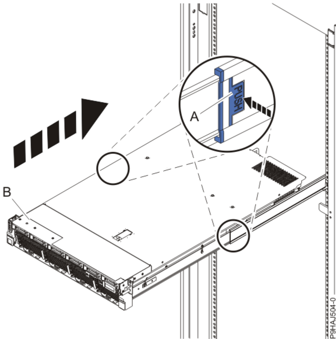
図 29. システムの操作位置への設置
