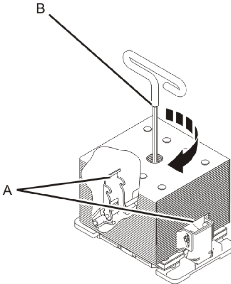
図 25. ヒート・シンク上の中央にあるロードねじの締め付け
