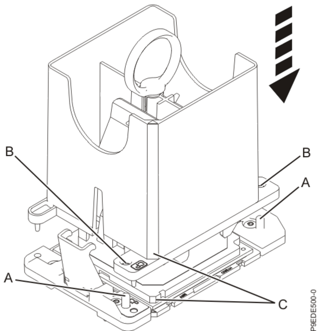
図 10. 取り外しツールをシステム・プロセッサ・モジュールの上に下ろす
