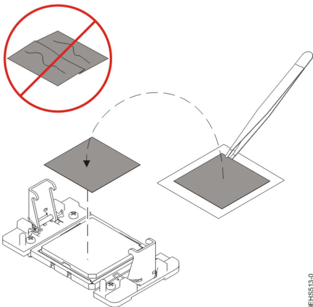
図 23. システム・プロセッサ・モジュールへの TIM の移動 b) ヒート・シンクを TIM の上に置きます (26 ページの図 24 を参照)。
