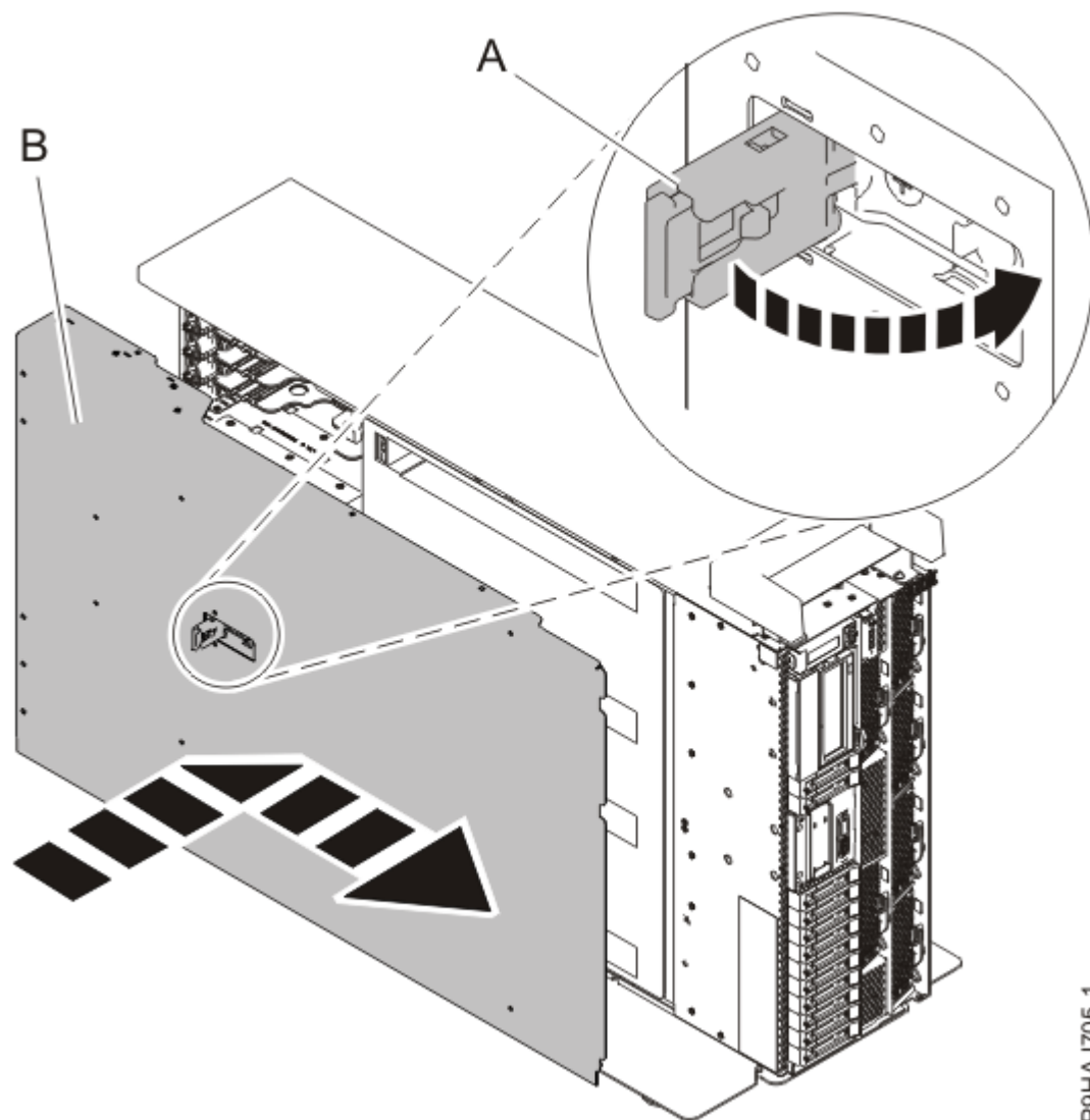
図 34. 保守アクセス・カバーの取り付け
