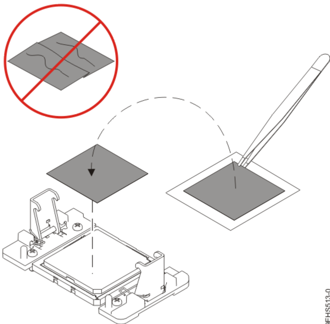
図 28. システム・プロセッサ・モジュールへの TIM の移動 b) ヒート・シンクを TIM の上に置きます (31 ページの図 29 を参照)。
