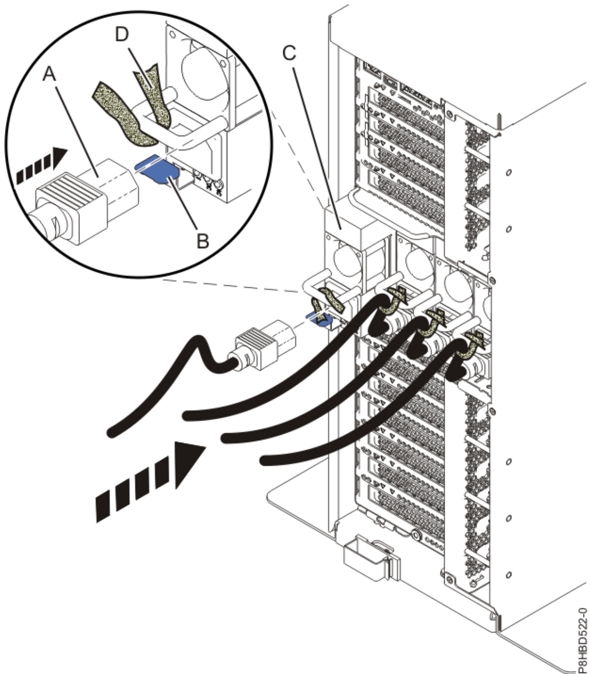
図 35. 電源装置の再取り付け
