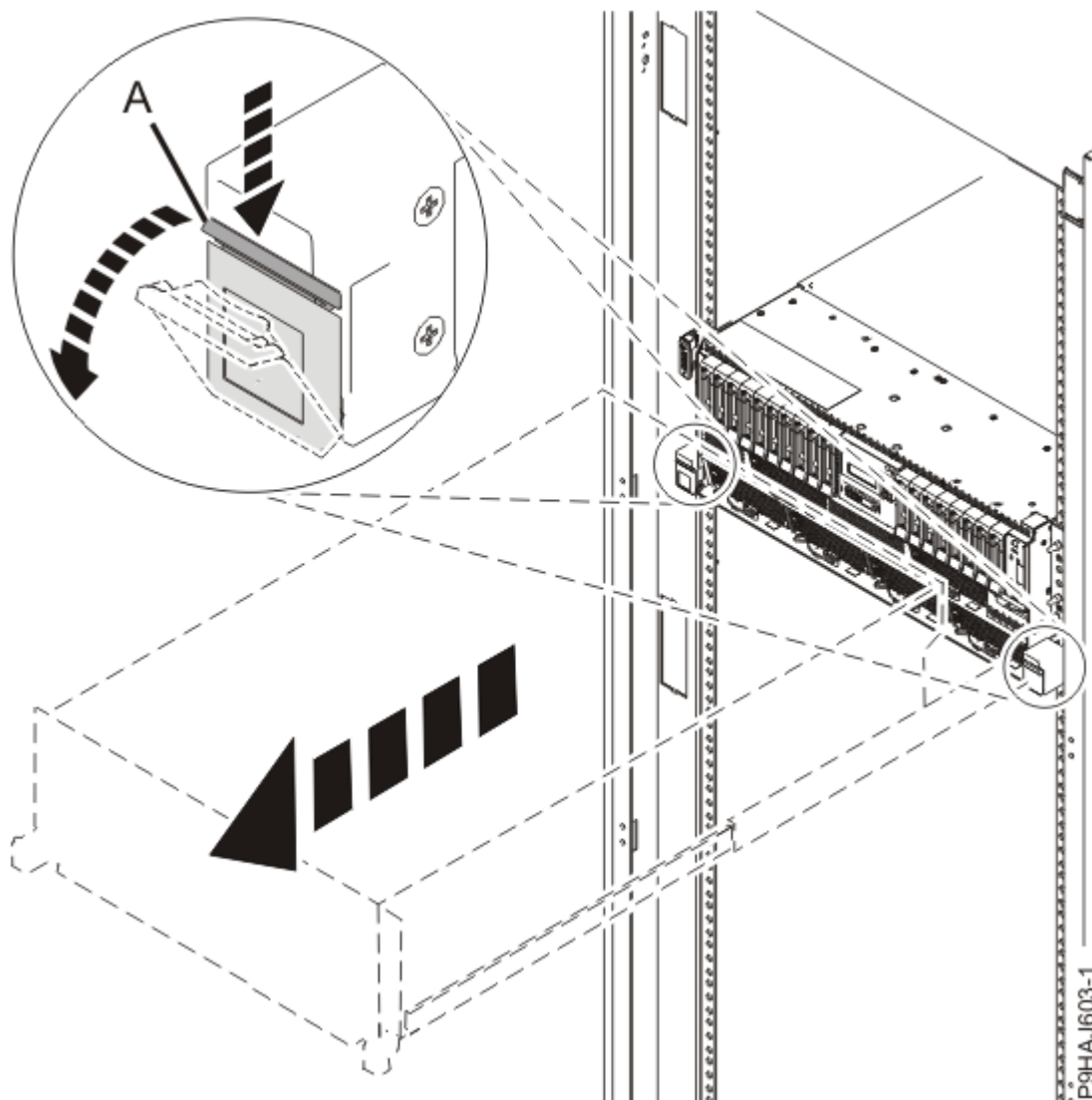
図 3. サイド・ラッチのリリース
