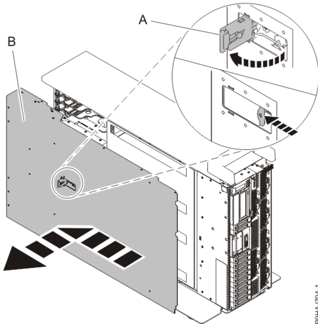
図 7. 保守アクセス・カバーの取り外し
