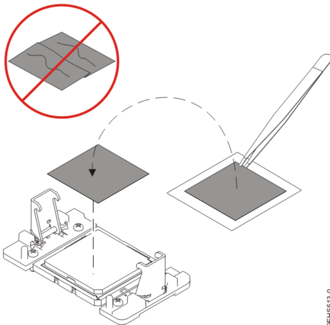
図 26. システム・プロセッサ・モジュールへの新規 TIM の取り付け
