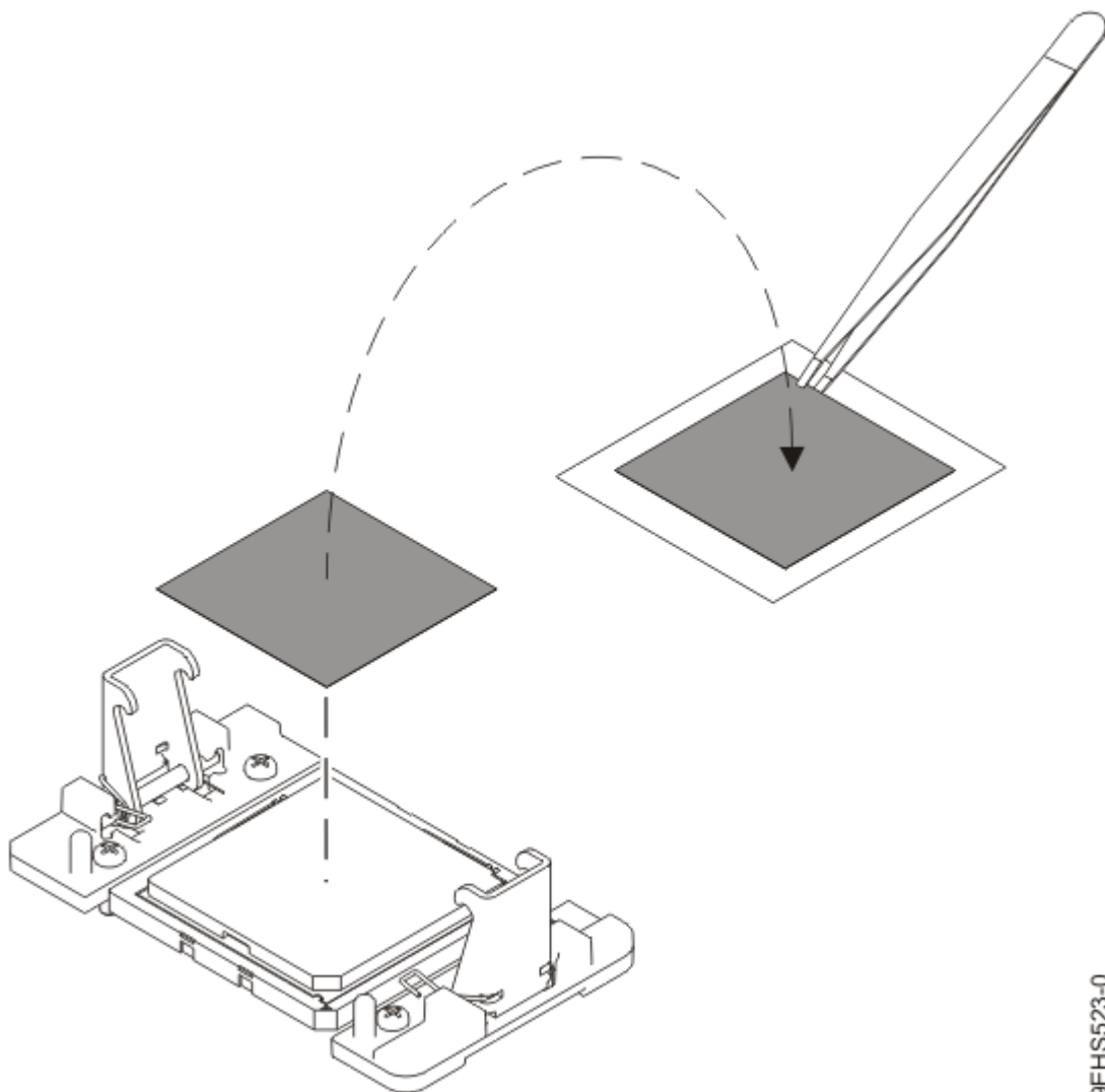
図 13. システム・プロセッサ・モジュールからの TIM の取り外し
