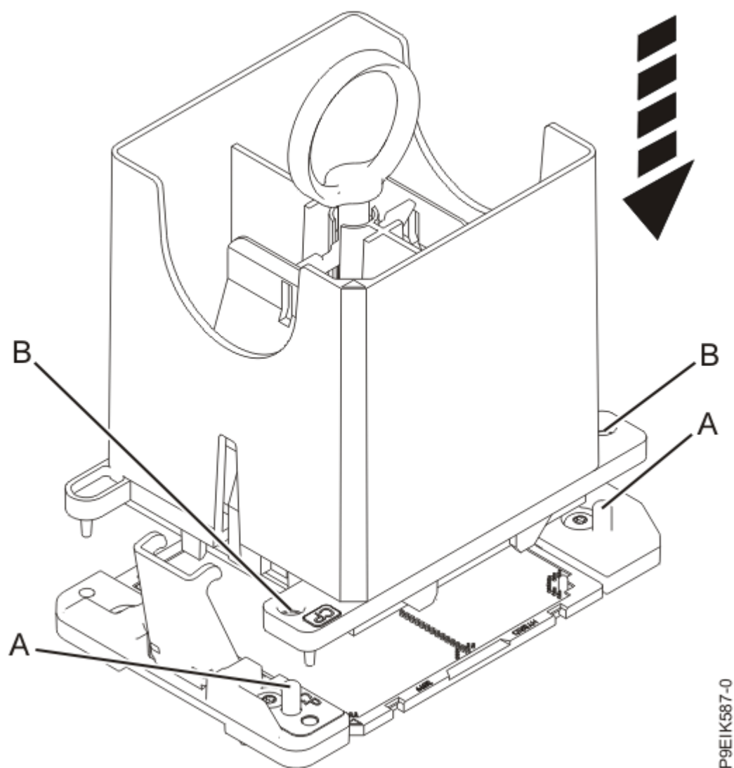
図 23. システム・プロセッサ・モジュールの取り付け
