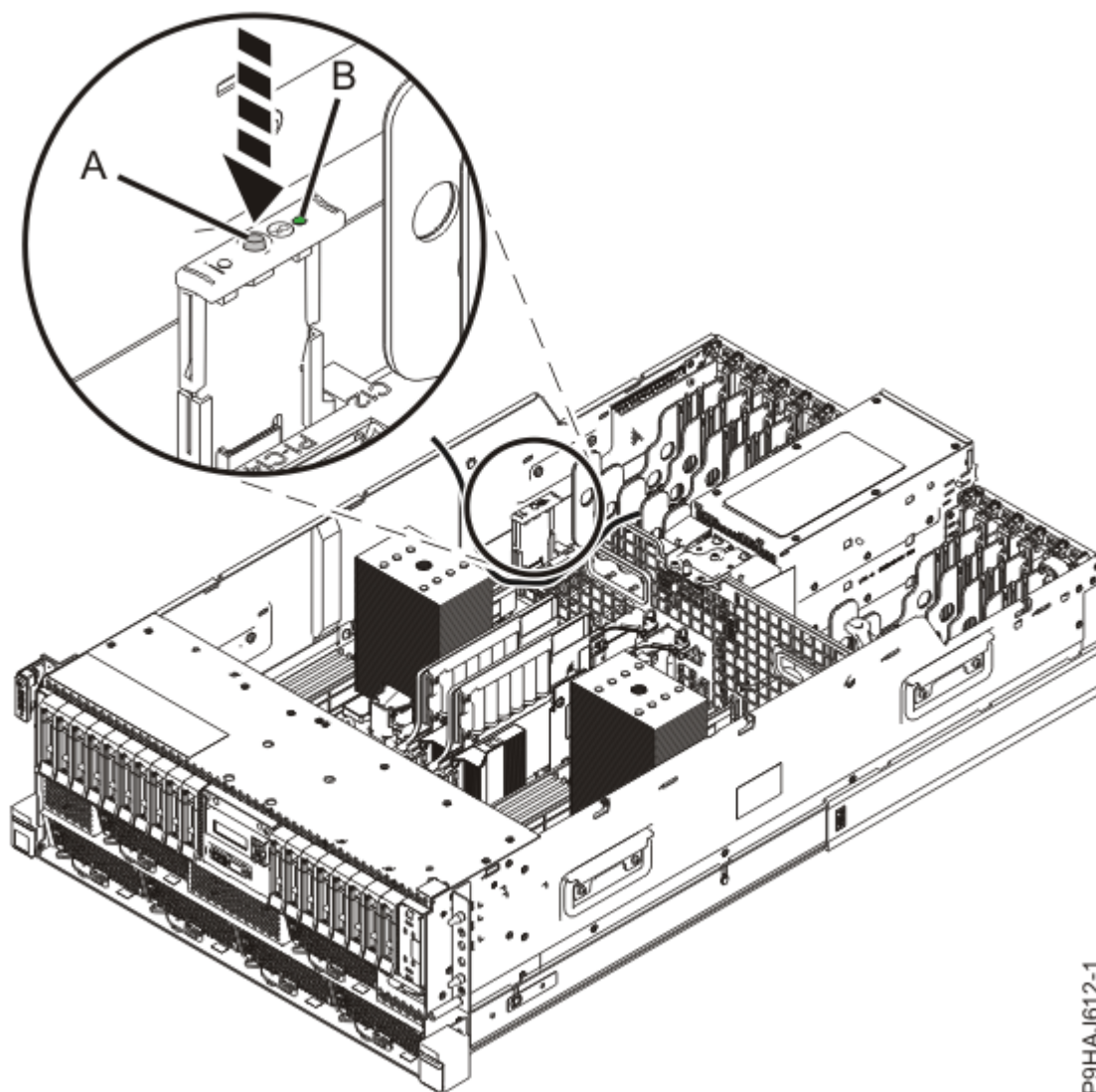
図 10. 識別 LED の活動化
