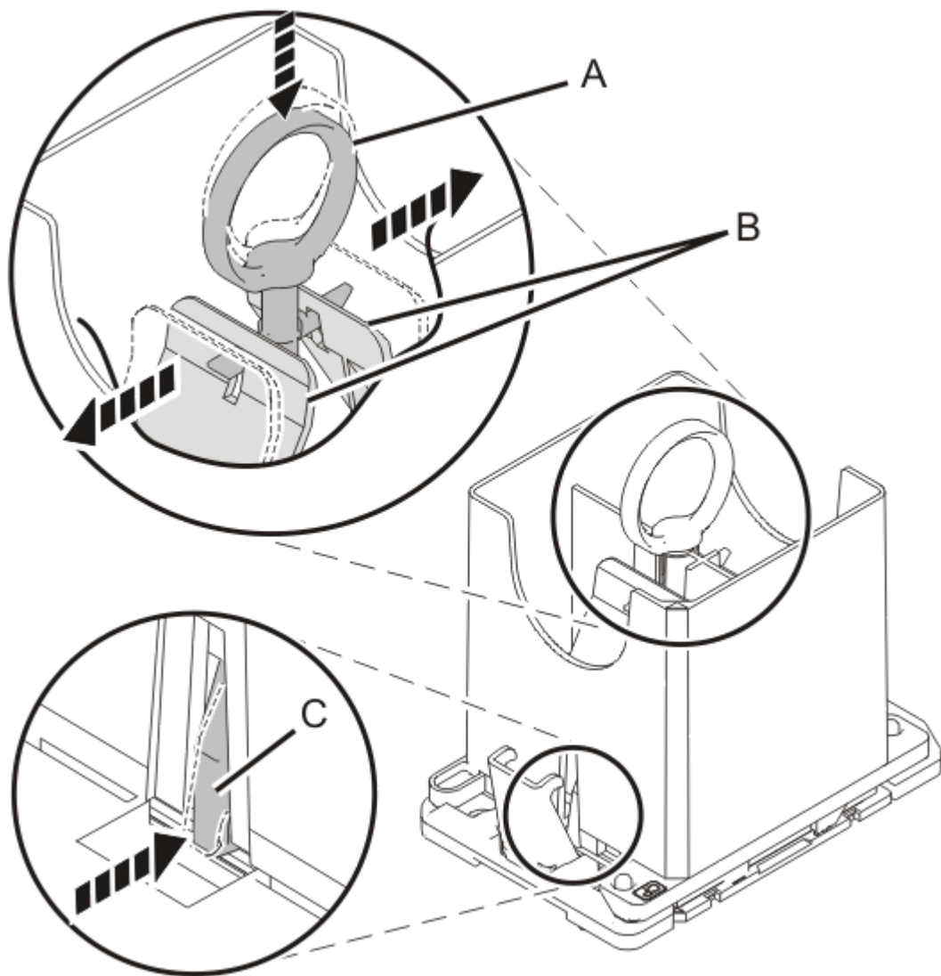
図 16. システム・プロセッサ・モジュールをツールにロック
